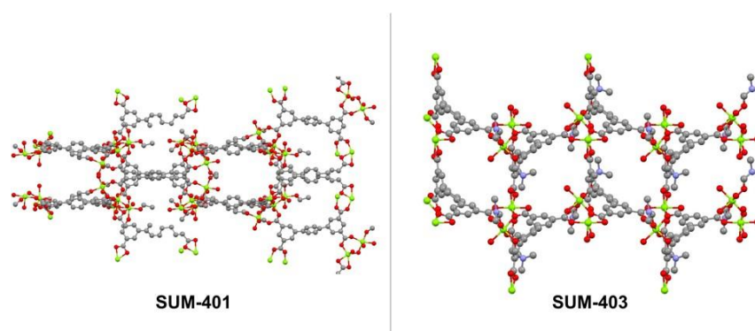
Figure 6. MOF de Mg vue selon l'axe b. Les groupes latéraux ont été éliminés pour une meilleure visualisation.
