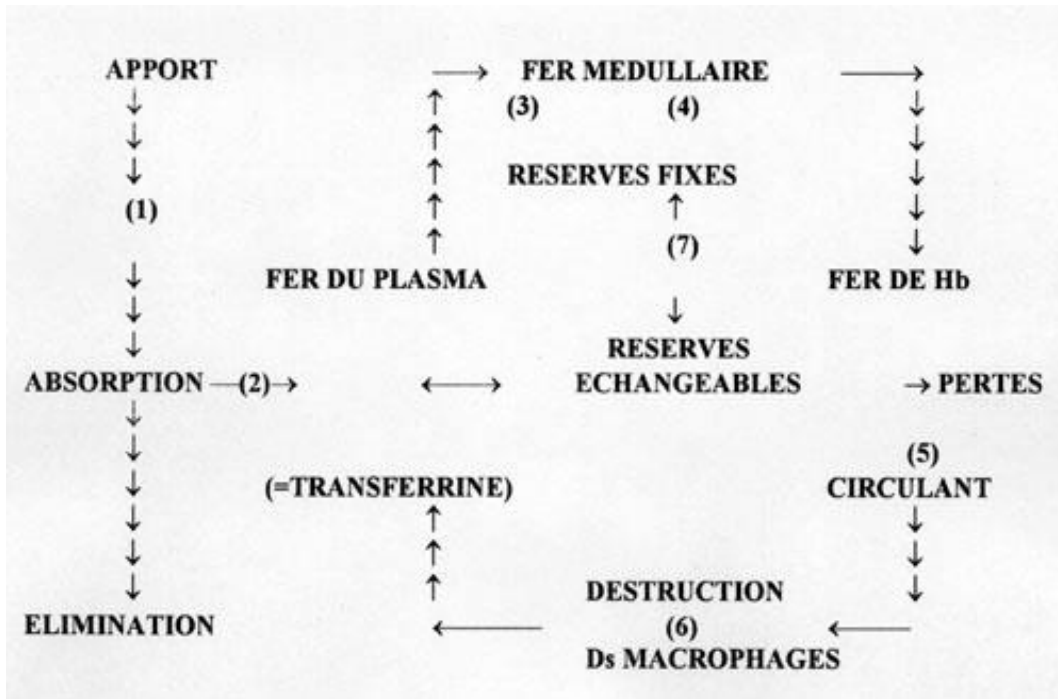
Figure 3a : Cycle du fer
