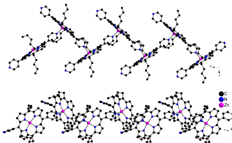
Figure II-23 : Portion du réseau monodimensionnel formé par T1 en présence d'acétate dans le plan ab (en haut) et dans le plan bc (en bas). Les atomes d'hydrogène sont omis pour plus de clarté.
