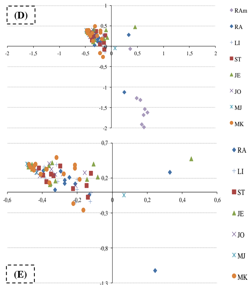
Figure 4.5 (D) et (E) - Analyse factorielle des correspondances sur les profils génétiques, montrant les individus des 8 populations de B. splendens (+ B. mollis en (D)) de la Nouvelle-Calédonie. Labels des sites et espèces : cf. Figures 4.1 et 4.2 p. 187-188.
