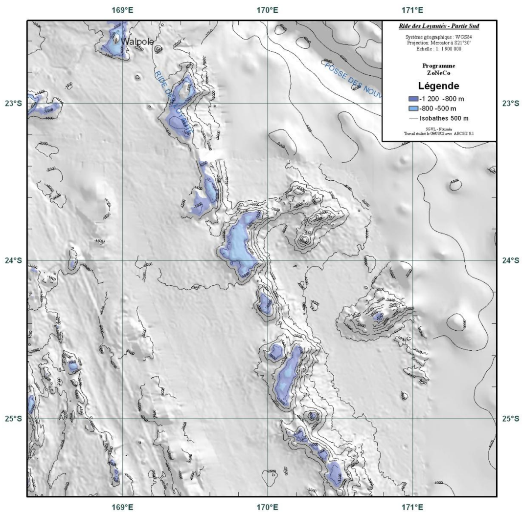
Figure 1.20 – La Ride des Loyauté : segment sud immergé (carte ZoNeCo).
