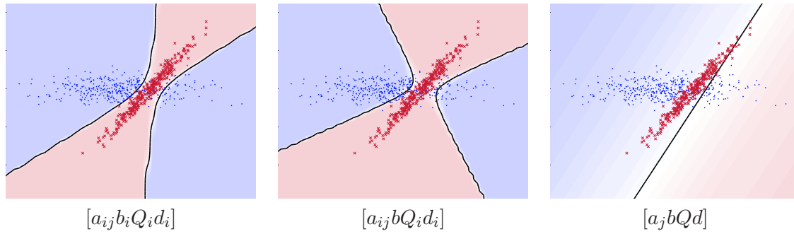
FIG. 5.2 – Frontières de décision de l’HDDA avec les modèles [a_{ij}b_i Q_i d_i] , [a_{ij}b Q_i d_i] et [a_j b Q d] sur les données simulées. Les données sont projetées sur deux des axes originaux pour la représentation uniquement.
