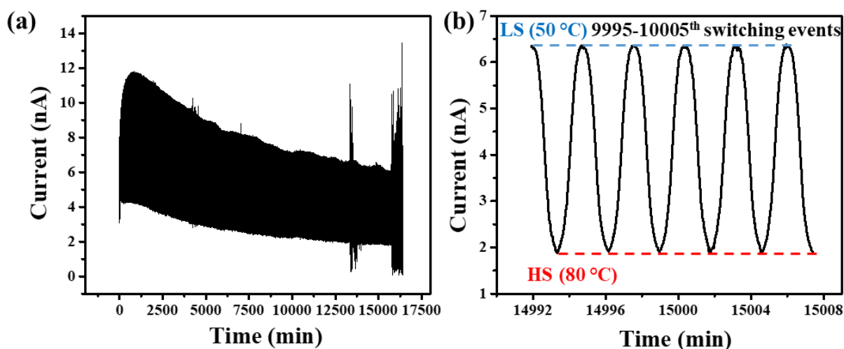
Figure 2.5 : (a) Cycles de commutation actuels entre le HS et le LS dans la jonction pendant >10.000 commutations. Des zooms sont également montrés sur les 9995ème - 10005ème (b) événements de commutation.
