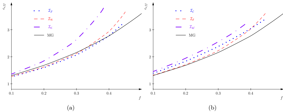
FIGURE 20 – Comparaisons des simulations avec la loi de Maxwell-Garnett pour diverses fraction volumiques f
