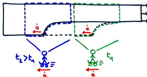
Figure 8 Principe de l'approche en régime stationnaire : l'observateur suit l'avancée du front de fissure à la vitesse \dot{a} .
