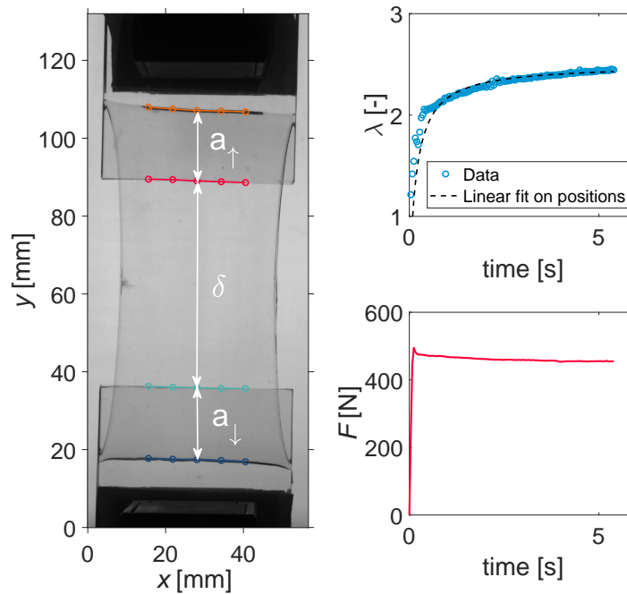
Figure 3 Exemple de test TCTT : après une traction \delta à la vitesse \dot{\delta} = 10 \text{ mm} \cdot \text{s}^{-1} , l'intercalaire s'est décollé d'une longueur 2a . L'élongation est \lambda = 1 + \delta/2a .
