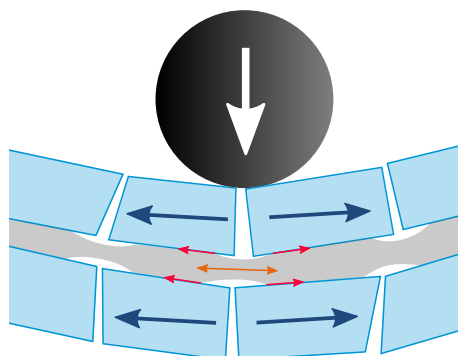
Figure 2 Schéma d'un verre feuilleté sous impact : tension entre fragments ( \leftarrow \rightarrow ), élongation ( \leftrightarrow ) et délamination ( \rightarrow ) de l'intercalaire.
