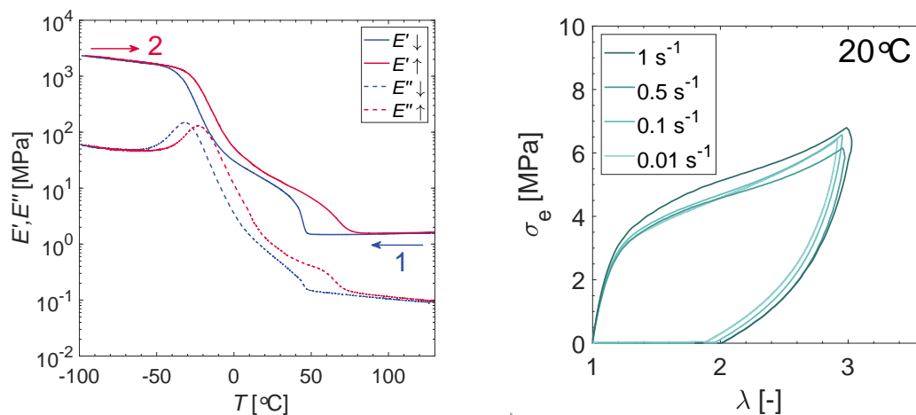
(a) DMTA en petites déformations : module de stockage E' et module de perte E'' of EVA en fonction de la température ( \varepsilon = 0.1\% , f = 1 \text{ Hz} , \beta = 1^{\circ}\text{C}\cdot\text{min}^{-1} )
