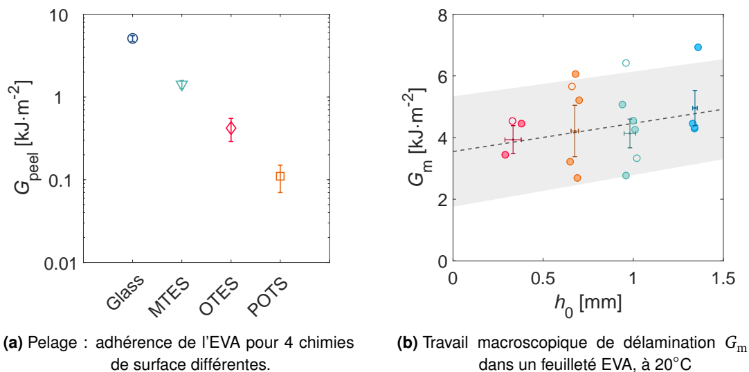
Figure 6 Délamination de l'EVA : (a) contrôle de l'adhésion par la chimie de surface, (b) énergie de délamination dans le TCTT.
