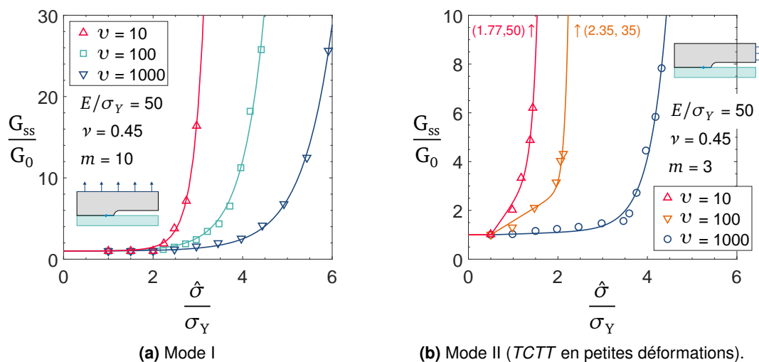
Figure 9 Énergie de fracture en régime stationnaire vs. contrainte cohésive, dans un matériau visco-plastique : effet de la vitesse de propagation v .
