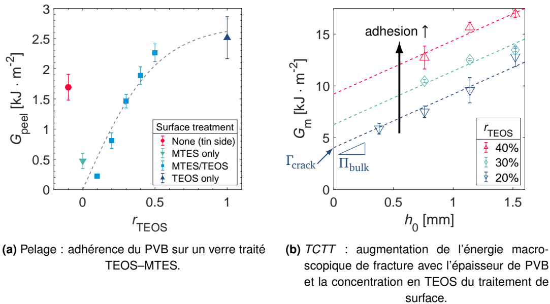
Figure 4 Modification d'adhésion dans le verre feuilleté avec du PVB.
