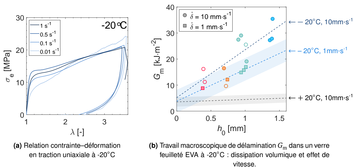
Figure 7 Intercalaire EVA à sa T_g : (a) comportement mécanique dissipatif et (b) TCTT.
