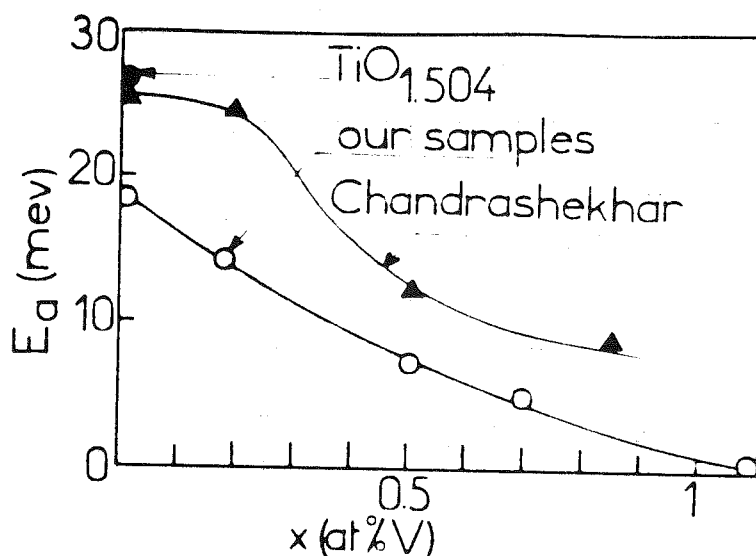
Fig. 52 : Variation de l'énergie d'activation E_a en fonction de x pour différents cristaux de \text{Ti}_2\text{O}_3 .
