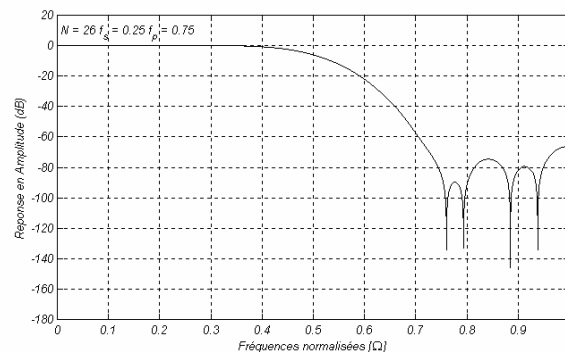
Figure IV- 29 : Effet de la troncature des coefficients du HB1.
