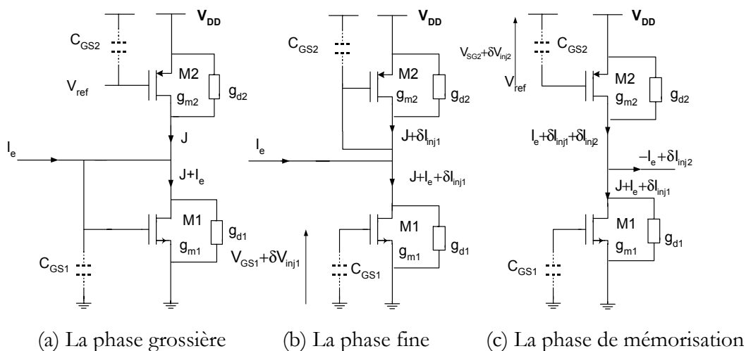
Figure I- 12 : La cellule mémoire S 2 I durant la phase d'acquisition (la phase grossière-la phase fine) et durant la phase de mémorisation.
