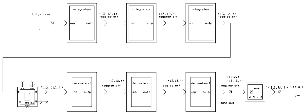
Figure IV- 58 : Filtre sinus cardinal.
