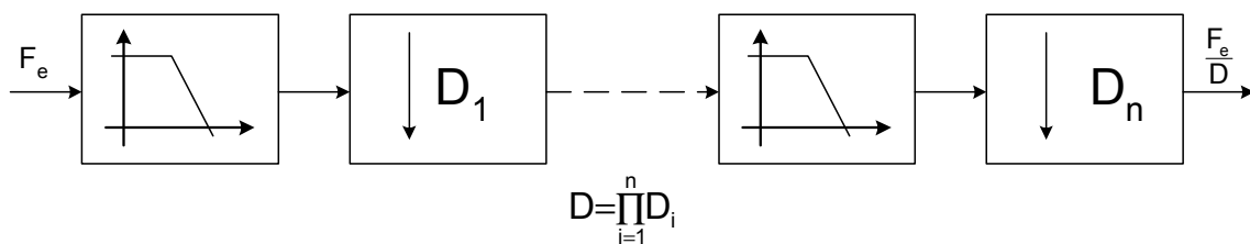
Figure II- 38 : Décimation à plusieurs étages.
