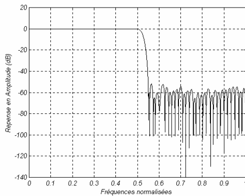
Figure IV- 23 : Réponse en fréquence du filtre H_{32}(z) avec des coefficients quantifiés en 13 bits.
