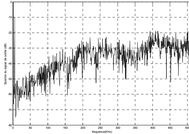
Figure III- 47 : Spectre de sortie du modulateur \Sigma\Delta S^2I .
