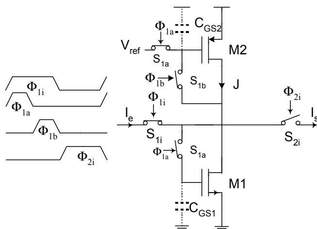
Figure I- 11 : La cellule mémoire de courant de base S 2 I.
