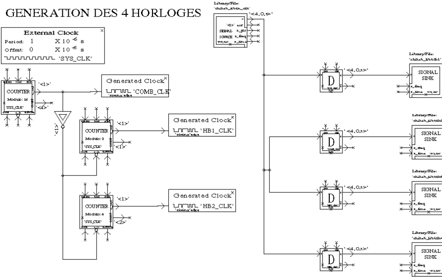
Figure IV- 55 : Génération des 4 horloges.
