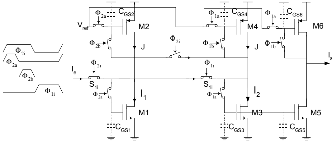
Figure III- 16 : Principe de l'intégrateur S 2 I à courants commutés.
