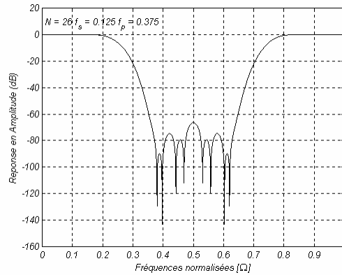
Figure IV- 39 : Réponse totale du Sinc compensée après décimation.
