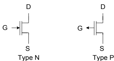
Figure I- 1 : Les symboles du transistor à enrichissement.
