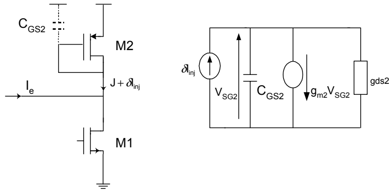
Figure I- 29 : Circuit équivalent en petits signaux de la cellule mémoire S 2 I en deuxième phase d'acquisition.
