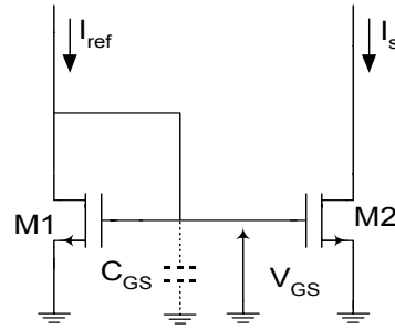
Figure I- 7 : Miroir de courant.
