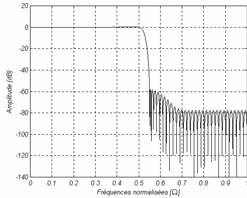
Figure IV- 22 : Réponse en fréquence composées du filtre H_3(z) = H_{31}(z) * H_{32}(z) .
