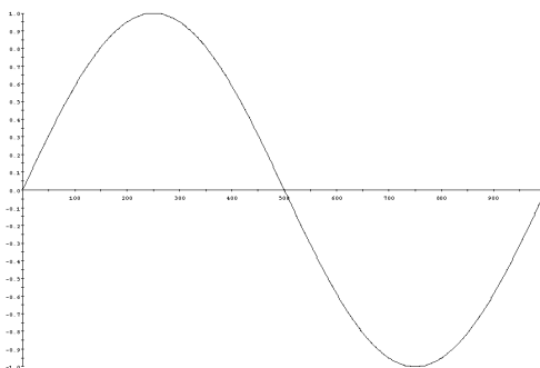
Figure IV- 50 : Entrée sinusoidale du dérivateur.
