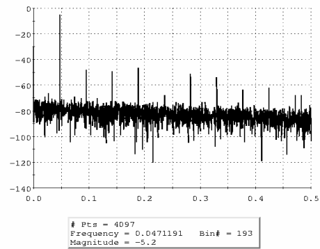
Figure IV- 79 : FFT de la sortie.
