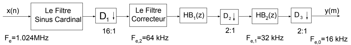
Figure IV- 25 : La structure 3, le filtre sinc suivi de deux demi-bande.
