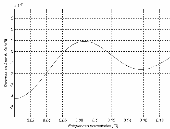
Figure IV- 27 : Ondulation dans la bande passante du filtre HB 1 .
