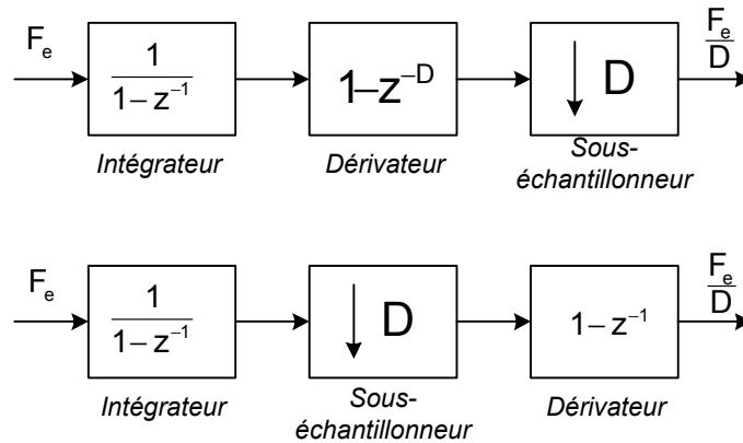
Figure II- 40 : Amélioration de la structure du sinus cardinal.
