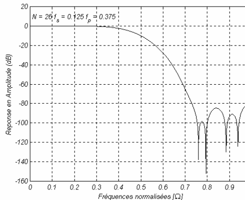
Figure IV- 41 : Réponse en fréquence composée et normalisée après le filtre HB1.
