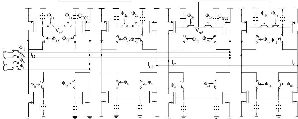
Figure III- 23 : Intégrateur différentiel S 2 I bilinéaire.
