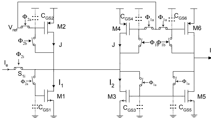
Figure III- 17 : Principe d'un intégrateur S 2 I non inverseur.
