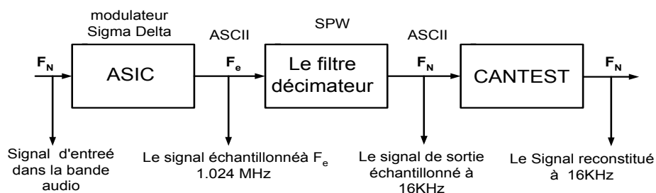
Figure IV- 86 : Schéma bloc du test.
