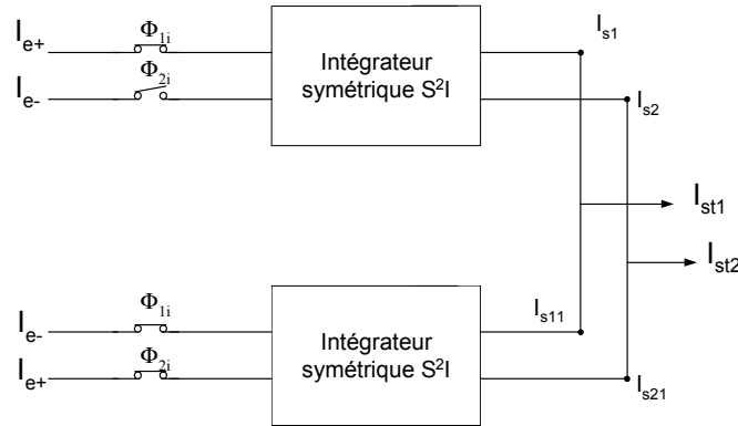
Figure III- 24 : Schéma synoptique de l'intégrateur différentiel S 2 I bilinéaire.
