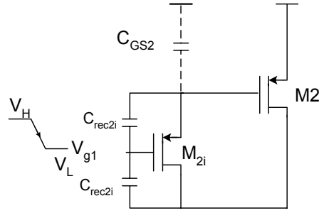
Figure I- 21 : Cellule mémoire S 2 I durant la phase fine avec les capacités parasites.
