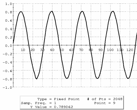
Figure IV- 74 : Sortie du premier filtre demi -bande.
