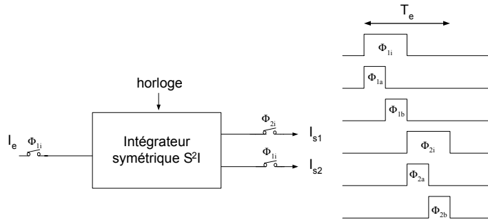
Figure III- 22 : Schéma synoptique de l'intégrateur S 2 I symétrique en mode courant.
