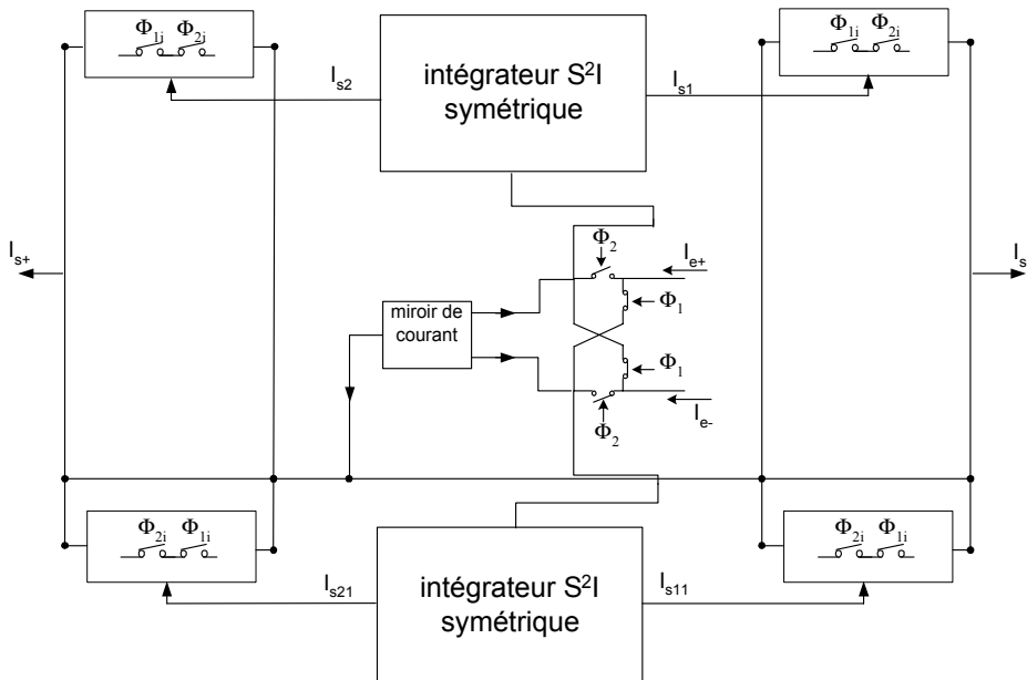
Figure III- 27 : Schéma synoptique de l'intégrateur S 2 I pseudo bilinéaire.
