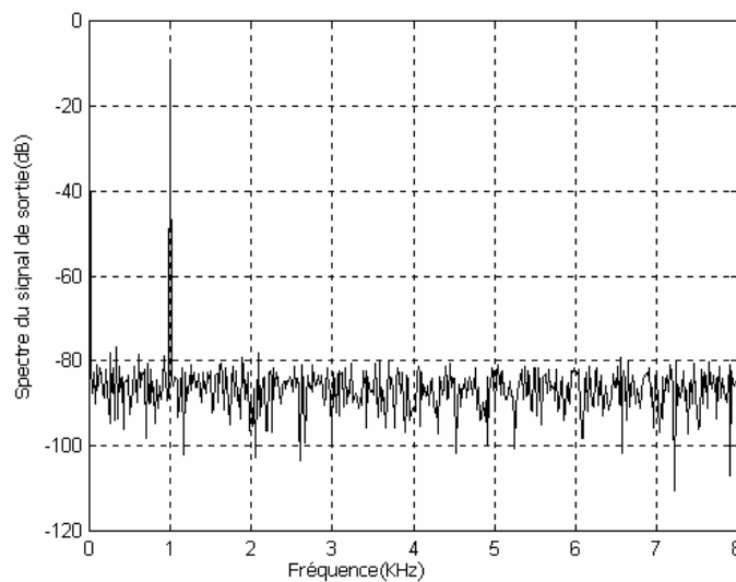
Figure III- 11 : Spectre de sortie pour le model S 2 I.
