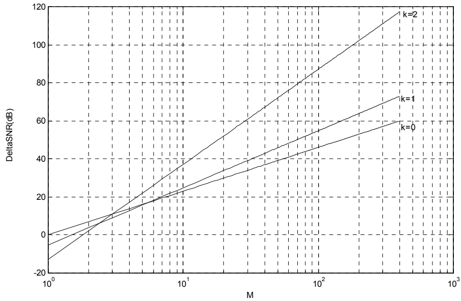
Figure II- 18 : Evolution du \Delta SNR pour différentes valeurs de k (0, 1, 2) en fonction de M.
