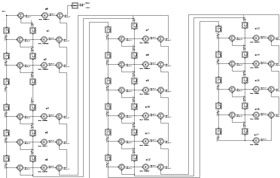
Figure IV- 65 : Filtre compensateur.
