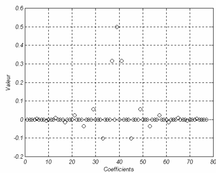
Figure IV- 32 : Effet de la troncature des coefficients du HB_2 .
