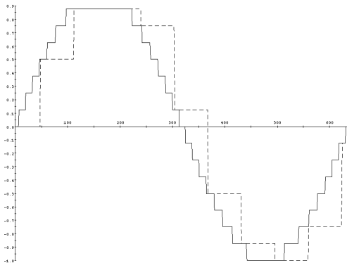
Figure IV- 56 : La décimation par 32.
