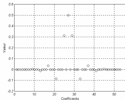
Figure IV- 28 : Réponse impulsionnelle du filtre HB 1 .
