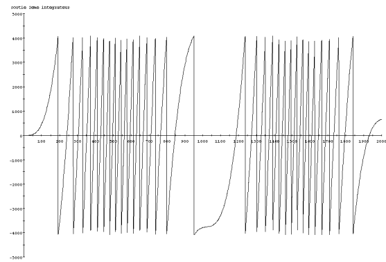
Figure IV- 60 : Sortie du deuxième intégrateur.
