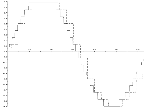
Figure IV- 57 : La décimation par 16.
