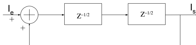
Figure I- 14 : Le schéma bloc en Z de l'intégrateur.
