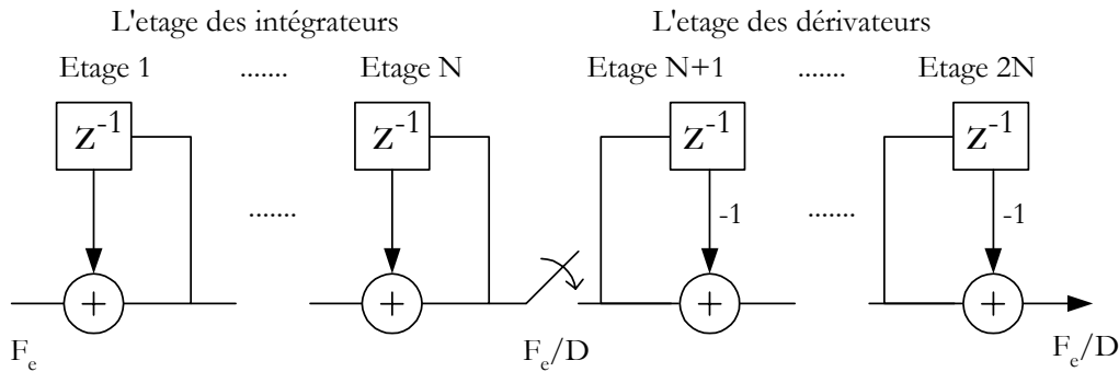
Figure IV- 45 : Structure sinus cardinal du filtre de décimation.
