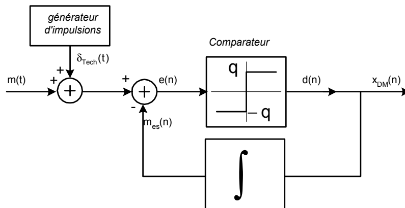
Figure II- 9 : Structure du modulateur Delta modifié.
