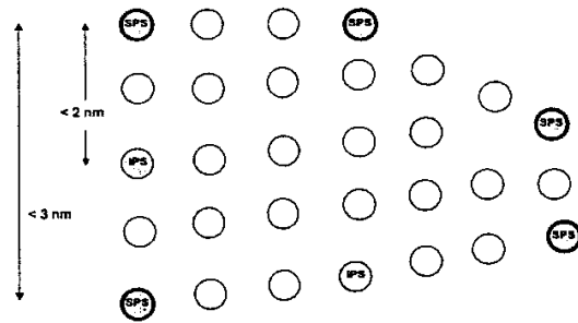
Hình 5a. Ví dụ về phương án bố trí báo hiệu khu vực nhóm điện gió ngoài khơi.
