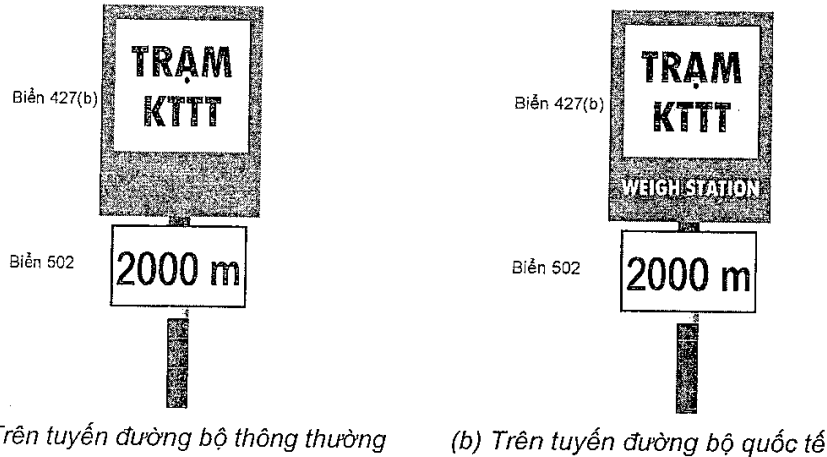
Hình 2. Mẫu biển báo cự ly đến trạm KTTTX
