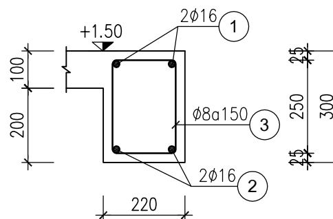
DẦM D4-220X300 - L=6.38M - SL:01
