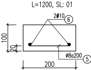
LANH TÔ CỦA ĐI D1
