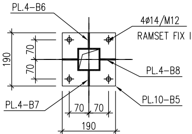
MẶT CẮT 5-5
