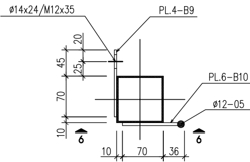
MẶT CẮT 2-2
