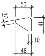
BẢN MÃ B7
