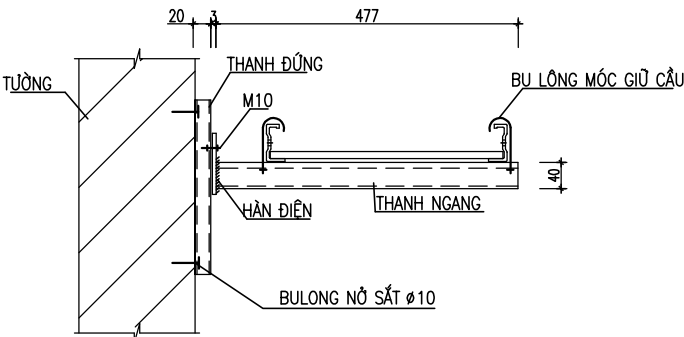
CHI TIẾT I-I: GIA CỐ CONSOL ĐỖ CẦU VÀO TƯỜNG (12 THANH)
