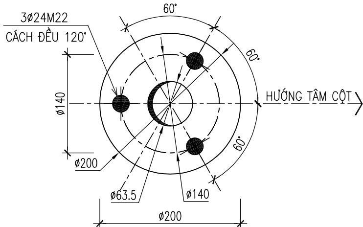
BẢN D3
