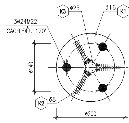
CHI TIẾT K1 \delta=16 ; SL=1
