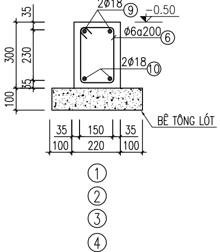
MẶT CẮT 9-9 (GM3 220X300, SL=04)
