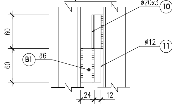
MẶT CẮT 5-5
