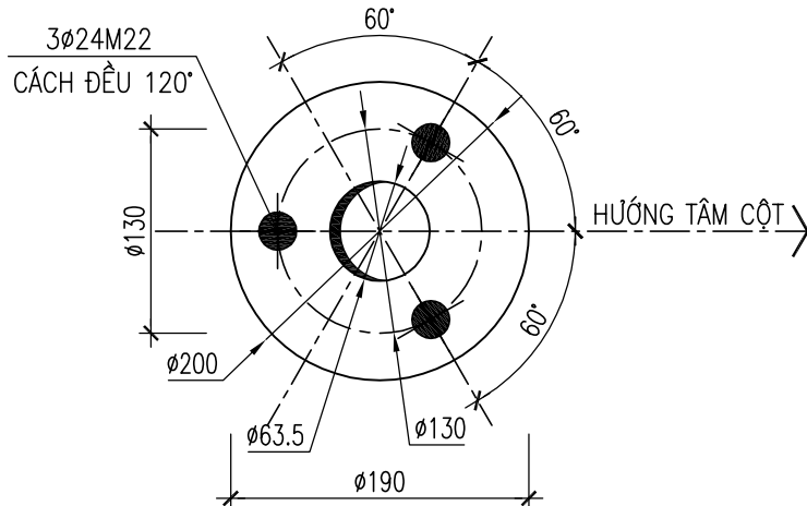
BẢN D1
