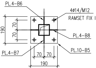
MẶT CẮT 5-5
