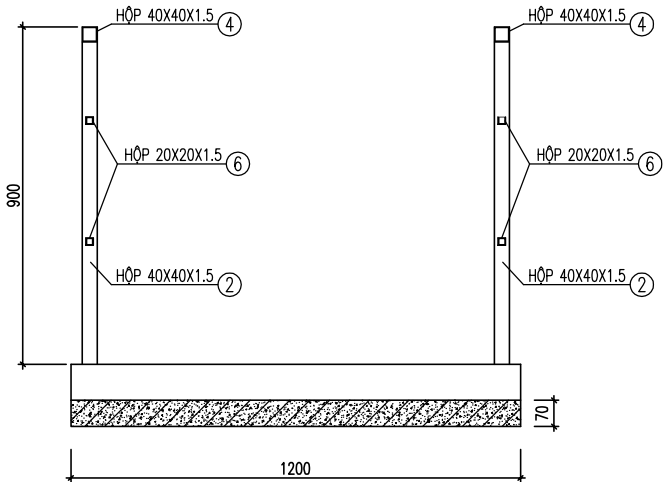
MẶT CẮT 1-1
