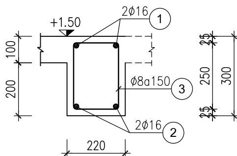
DẦM D3-220X300 - L=1.32M - SL:02
