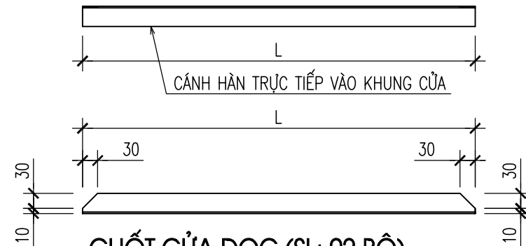
CHỐT CỬA DỌC (SL: 02 BỘ)
