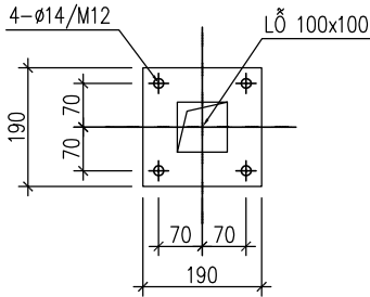
BẢN MÃ B1, B5
