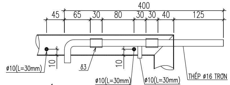
MẶT CẮT 3-3
