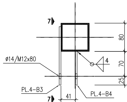
MẶT CẮT 7-7
