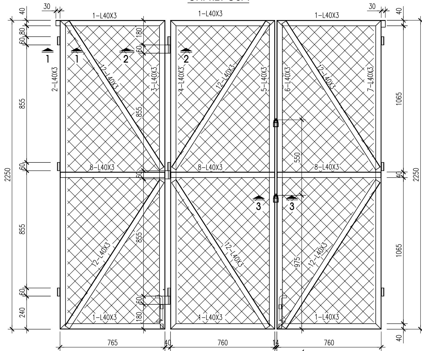
MẮT CẮT 2-2
