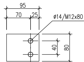
BẢN MÃ B4
