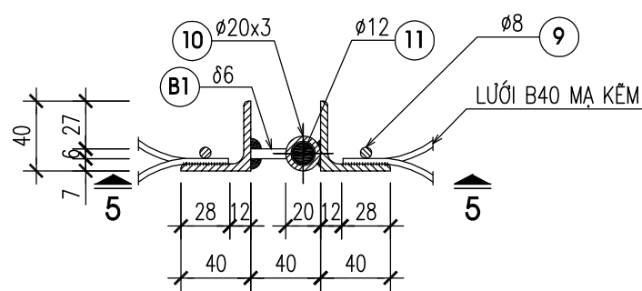
MẶT CẮT 5-5
