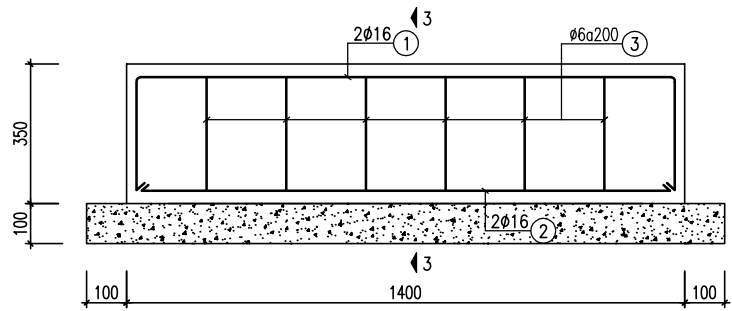
DẦM CHÂN THANG
