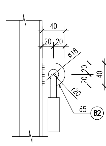
MẶT CẮT 7-7
