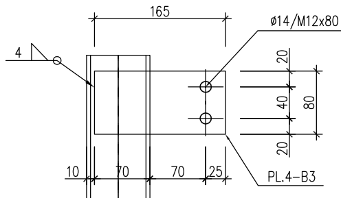
MẶT CẮT 7-7
