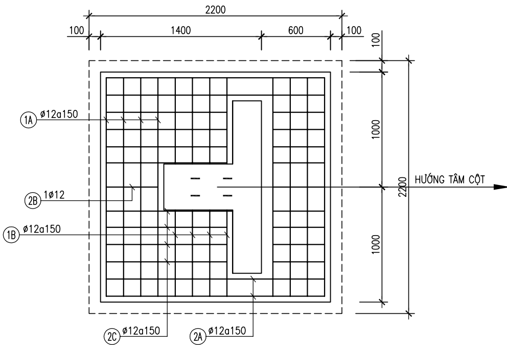
MẶT BẰNG BỐ TRÍ THÉP GIA CỐ
