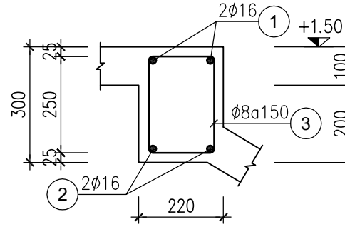
DẦM D5 220X300 - L=1.32M - SL:01
