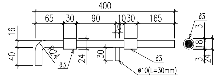
CHỐT CỬA DỌC (SL: 02 BỘ)
