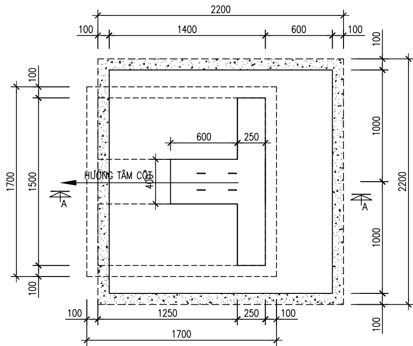
MẶT BẰNG GIA CỐ MÓNG CO M2, M3
