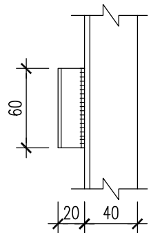
MẶT CẮT 4-4
