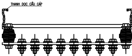
CHI TIẾT I-I: GIA CỐ CONSOL ĐỖ CẦU VÀO TƯỜNG (12 THANH)
