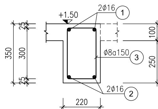
DẦM D2-220X350 - L=4.05 - SL:03
