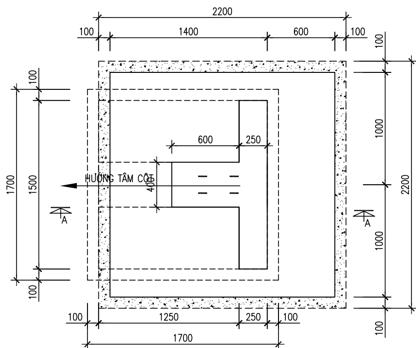
MẶT BẰNG GIA CỐ MÓNG CO M1
