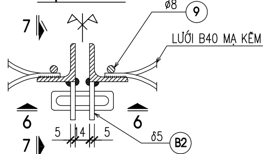
MẮT CẮT 6-6
