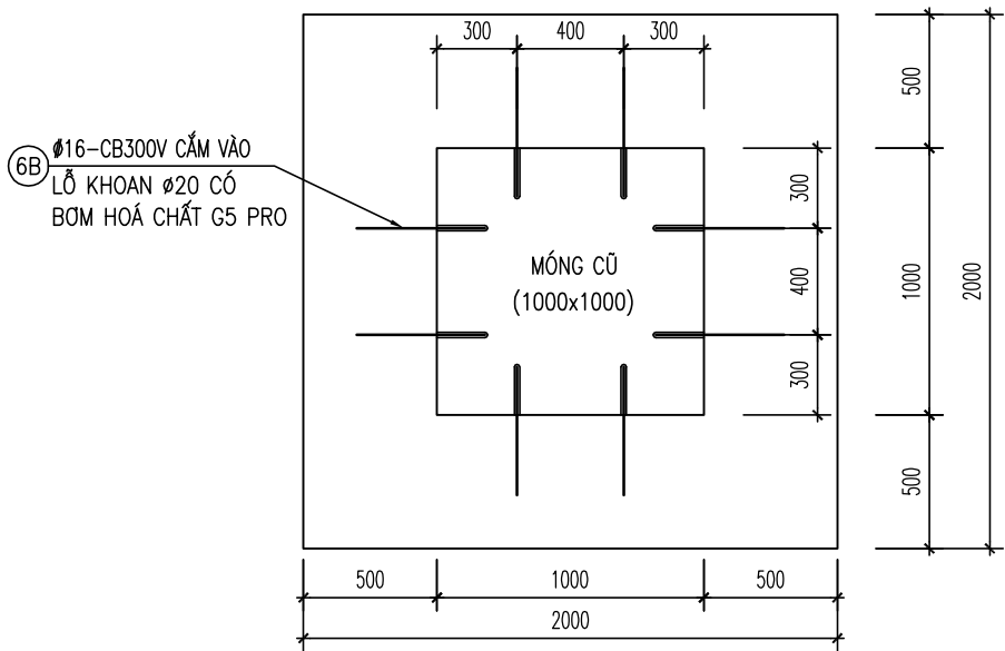
MẶT CẮT E - E
