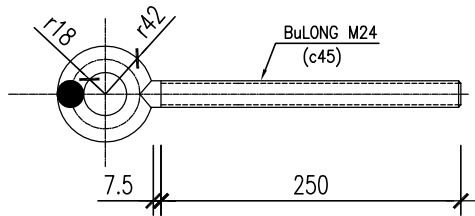
CHI TIẾT BULÔNG M24 (BL) sl: 2c
