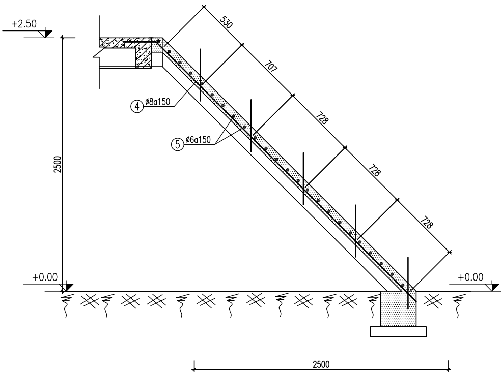
MẶT CẮT 1-1
