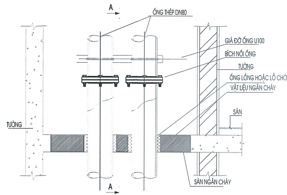
CHI TIẾT LẮP ĐẶT ĐƯỜNG ỐNG TRỰC ĐỨNG
