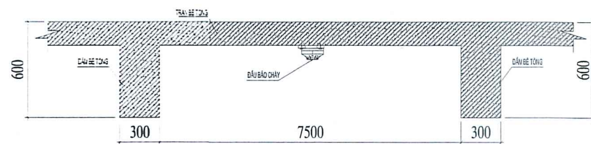
CHI TIẾT LẮP ĐẦU BẢO CHÁY GIỮA CÁC DẦM BÊ TÔNG
