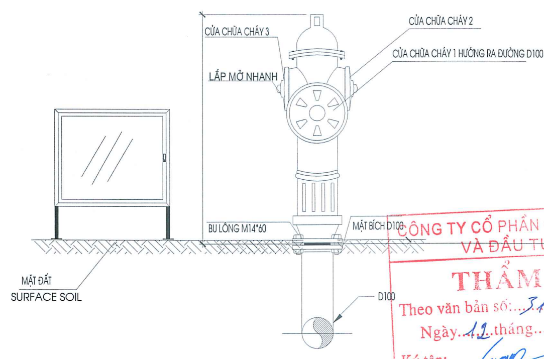
HỌNG NƯỚC CHỮA CHÁY 3 CỬA THEO TCVN 6379:2024
