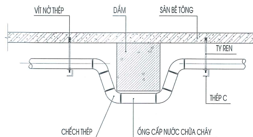
CHI TIẾT LẮP ĐẶT ỐNG CHỮA CHÁY TRÁNH DẦM
