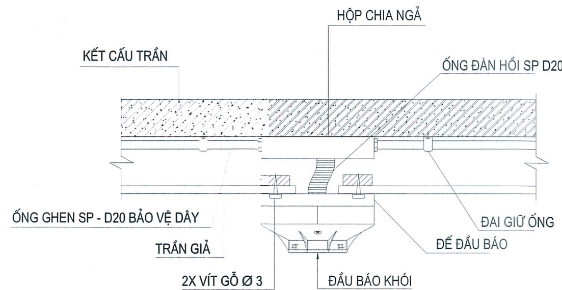
LẮP ĐẶT ĐẦU BẢO KHÓI DƯỚI TRẦN GIẢ
