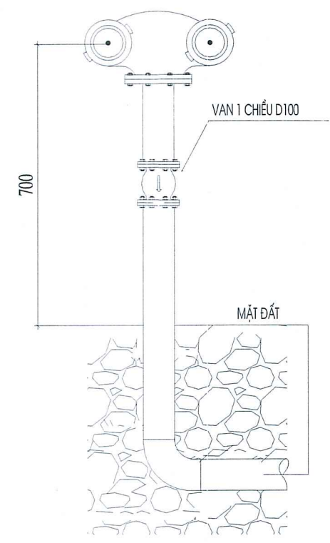
CHI TIẾT LẮP ĐẶT TRỤ TIẾP NƯỚC 2 CỬA DN65
