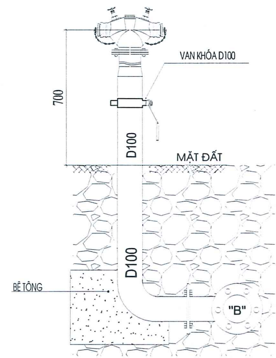
LẮP ĐẶT TRỤ CHỮA CHÁY 2 CỬA D100
