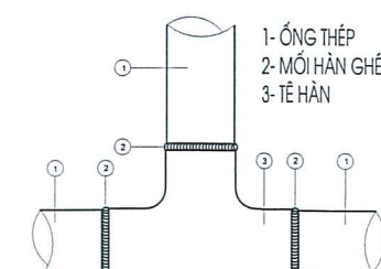
CHI TIẾT LẮP ĐẶT ỐNG VÀ PHỤ KIỆN TỪ BẢNG PHƯƠNG PHÁP REN
