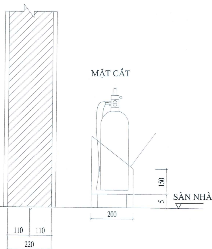
GIÁ ĐỰNG BÌNH CHỮA CHÁY
