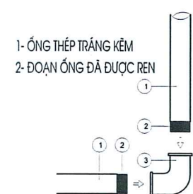
CHI TIẾT LẮP CÚT
