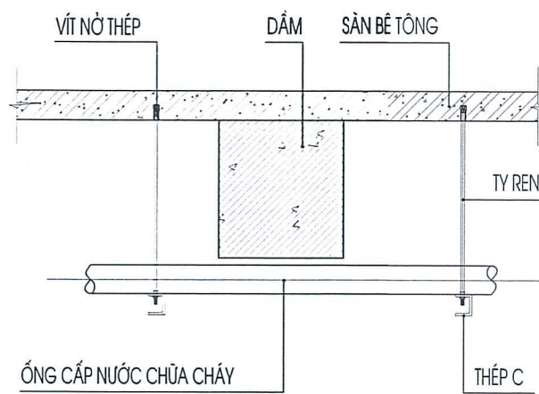
CHI TIẾT LẮP ĐẶT ỐNG CHỮA CHÁY QUA DẦM
