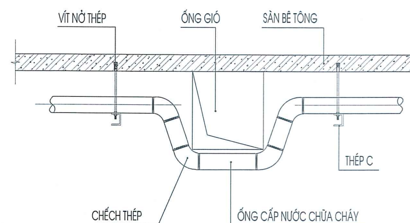
CHI TIẾT LẮP ĐẶT ỐNG CHỮA CHÁY TRÁNH ỐNG GIÓ
