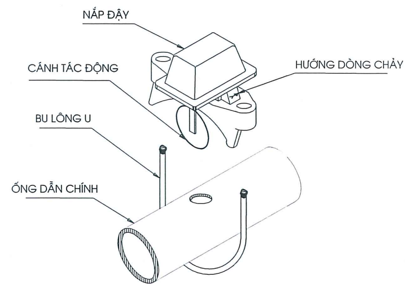
CHI TIẾT CÔNG TẮC DÒNG CHẢY
