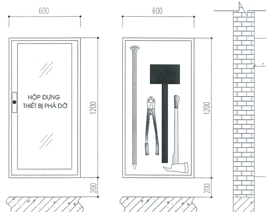
HỘP ĐỰNG THIẾT BỊ PHÁ ĐỠ:
