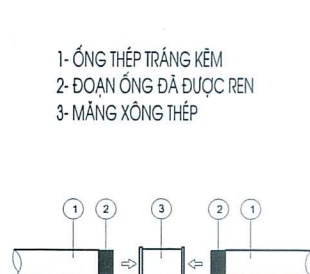
CHI TIẾT LẮP MĂNG XÔNG NỐI ỐNG
