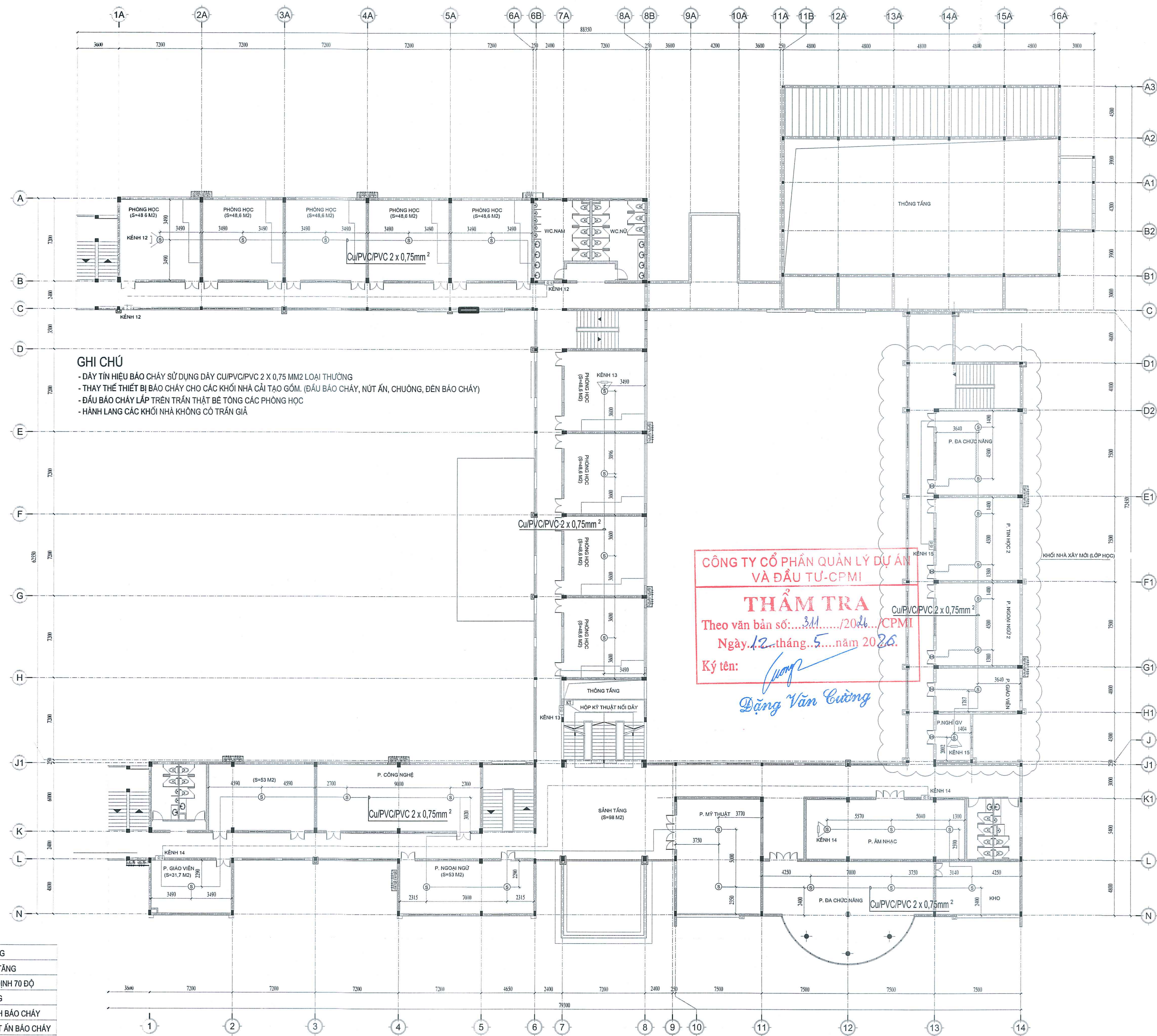
MẶT BẰNG BÁO CHÁY TẦNG 3
