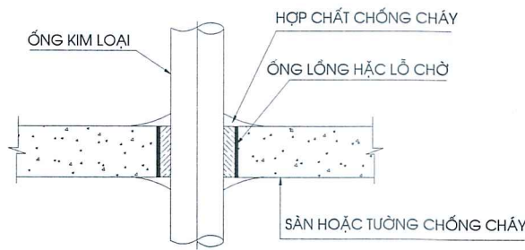
3-CHI TIẾT LẮP ĐẶT ỐNG XUYÊN SÀN CHỐNG CHÁY
