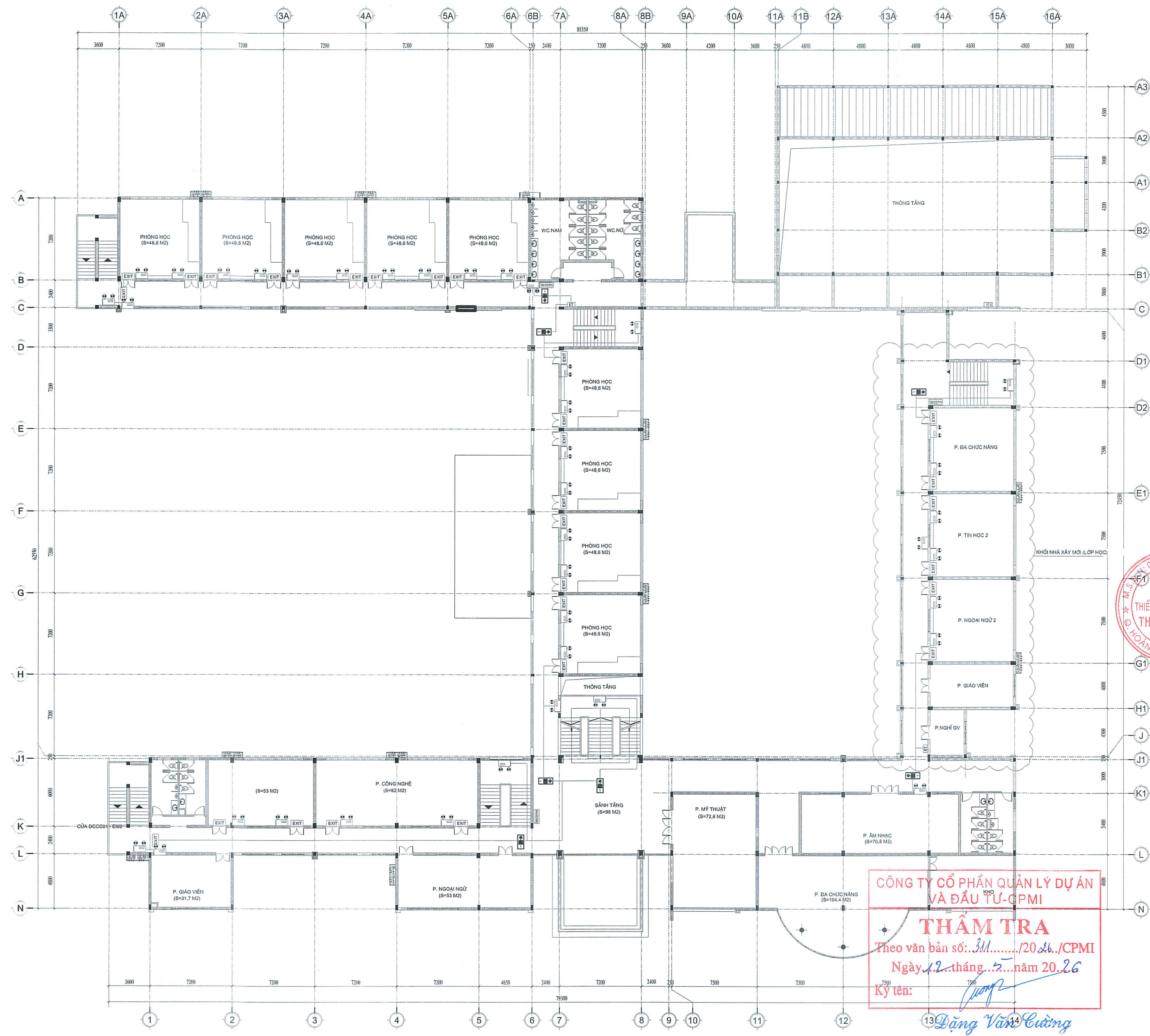
MẶT BẰNG ĐÈN EXIT & ĐÈN SỰ CỐ TẦNG 3
