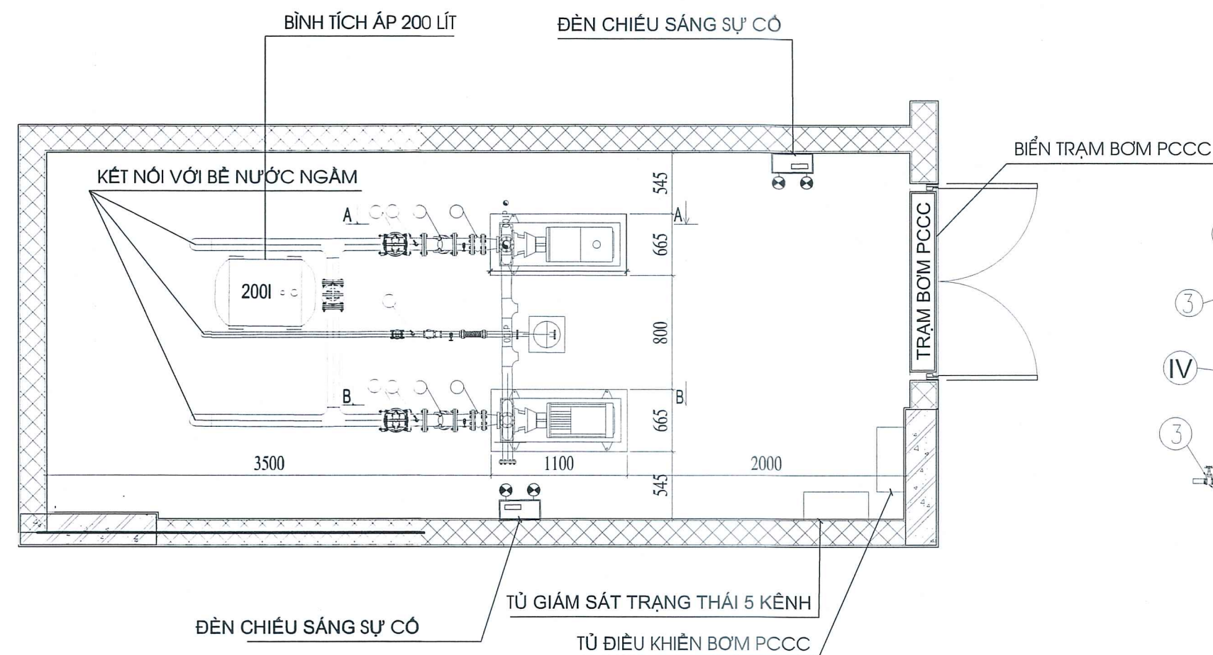
MẶT BẰNG TRẠM BƠM
