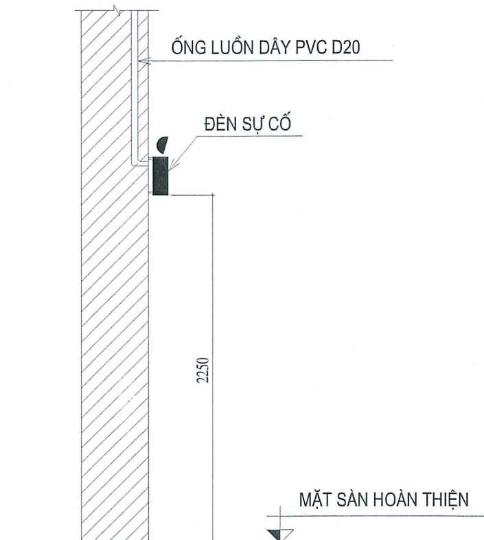
CHI TIẾT LẮP ĐẶT ĐÈN CHIẾU SÁNG SỰ CỐ
