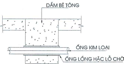
2-CHI TIẾT LẮP ĐẶT ỐNG XUYÊN DẦM
