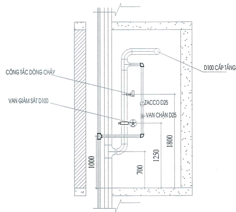
CHI TIẾT LẮP ĐẶT VAN TRỤC KỸ THUẬT
