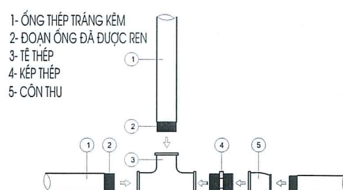
CHI TIẾT LẮP CÚT HÀN
