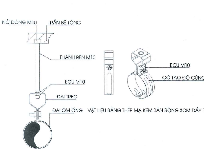
CHI TIẾT TREO ỐNG CHO 1 ỐNG D65 TRỞ XUỐNG
