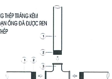
CHI TIẾT LẮP MĂNG XÔNG NỐI ỐNG
