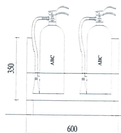
GIÁ ĐỰNG BÌNH CHỮA CHÁY
