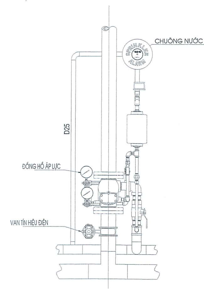
CHI TIẾT LẮP ĐẶT ALARM VALVE
