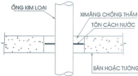
1-LẮP ĐẶT ỐNG XUYÊN SÀN, TƯỜNG CHỐNG THẨM
