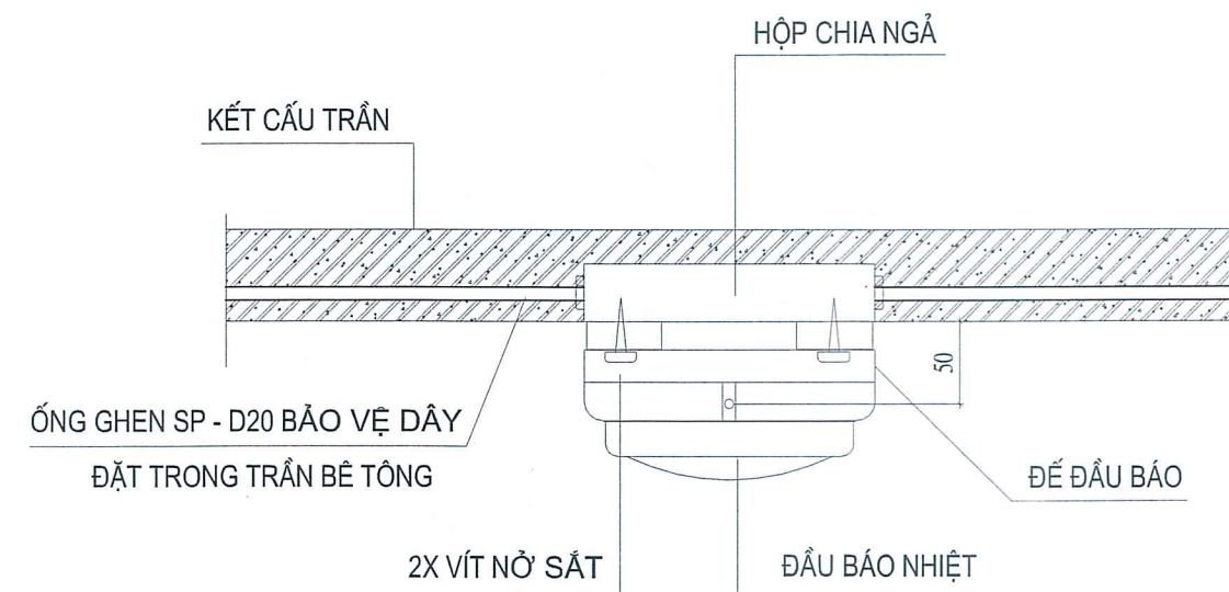
LẮP ĐẶT ĐẦU BẢO NHIỆT DƯỚI TRẦN BTCT
