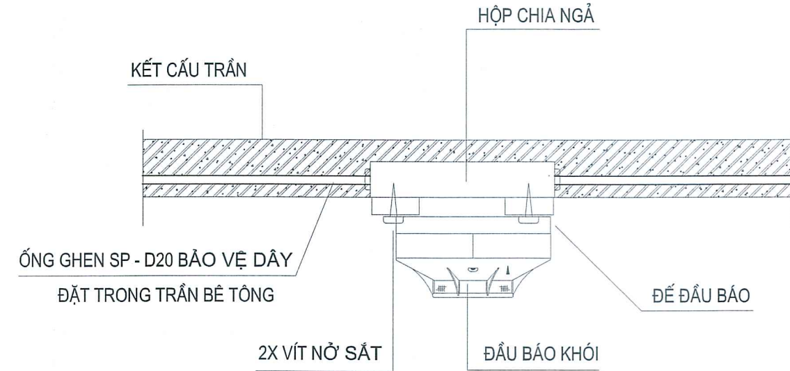
LẮP ĐẶT ĐẦU BẢO KHÓI DƯỚI TRẦN BTCT
