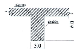
MẶT CẮT DẦM BÊ TÔNG
