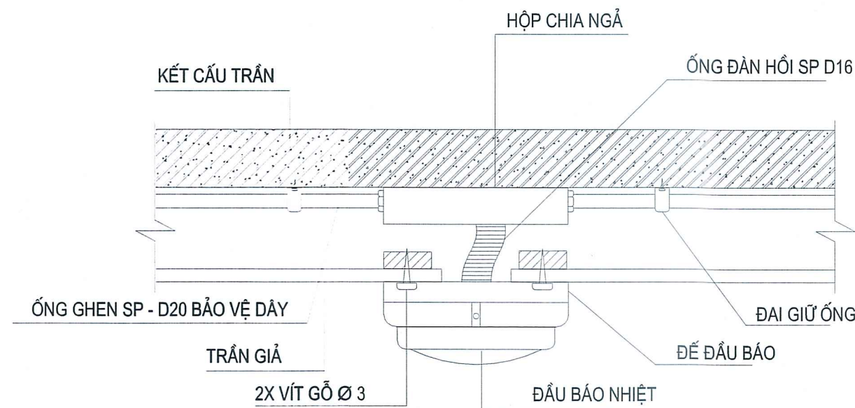
LẮP ĐẶT ĐẦU BẢO NHIỆT DƯỚI TRẦN GIẢ
