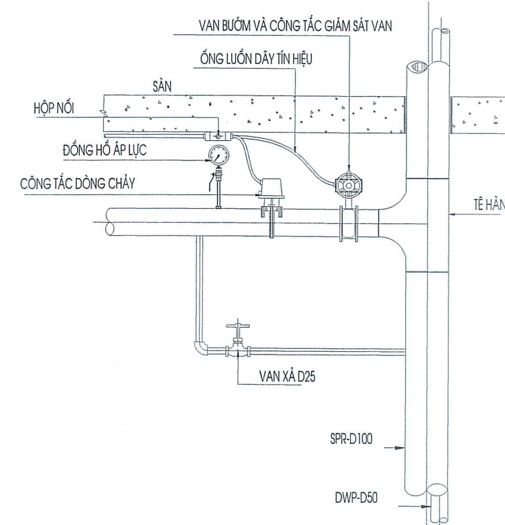
CHI TIẾT LẮP ĐẶT NHÁNH
