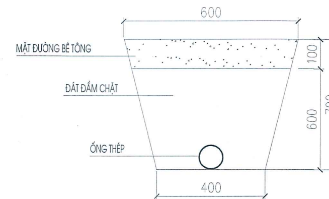
MẶT CẮT ĐƯỜNG ỐNG CHÔN NGOÀI NHÀ
