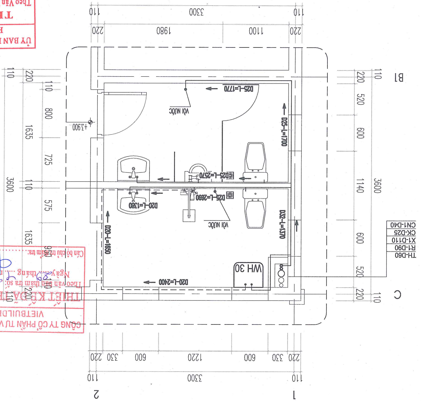
CHI TIẾT CẤP NƯỚC WC03
