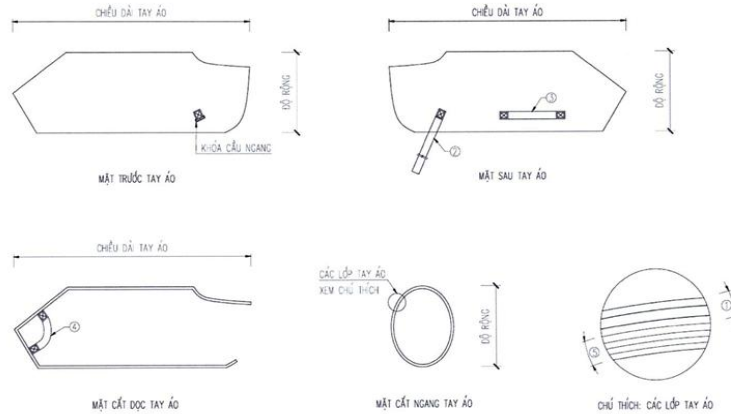
Hình 1 – Sơ đồ cấu tạo Tay áo bông bảo hiểm trong huấn luyện chó nghiệp vụ
