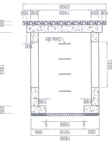
MẬT CẮT 2 - 2
