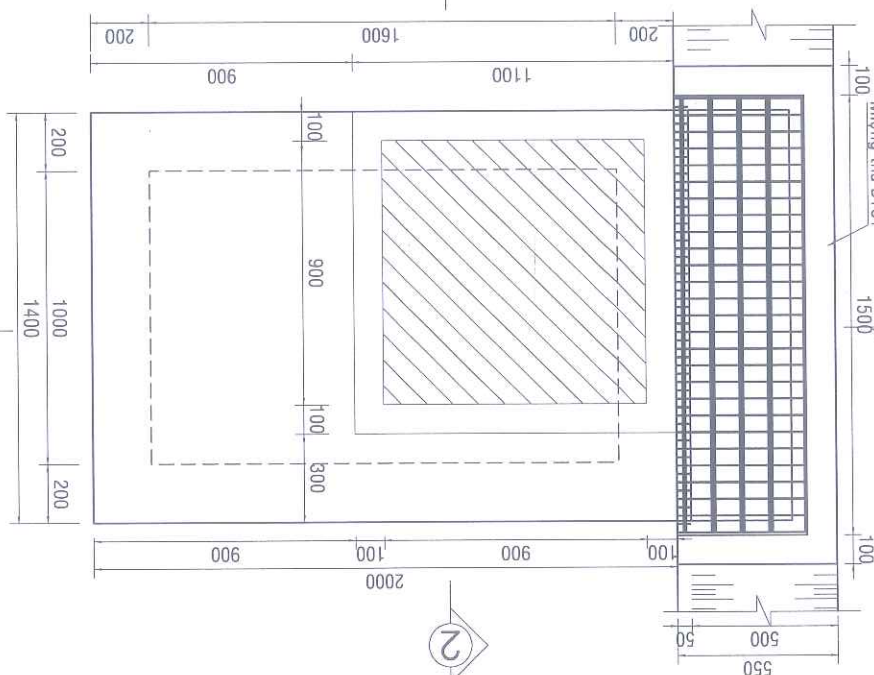
MẶT CẮT 1-1 TỶ LỆ: 1/25
