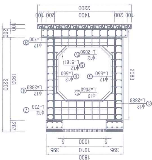
CỘT THÉP THÀNH
