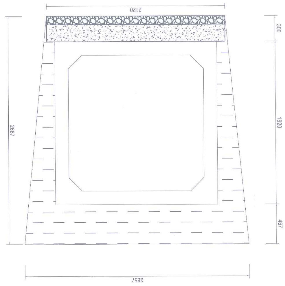
PHỤ ĐỒ CÔNG 1.6X1.6 Tỷ lệ: 1/25
