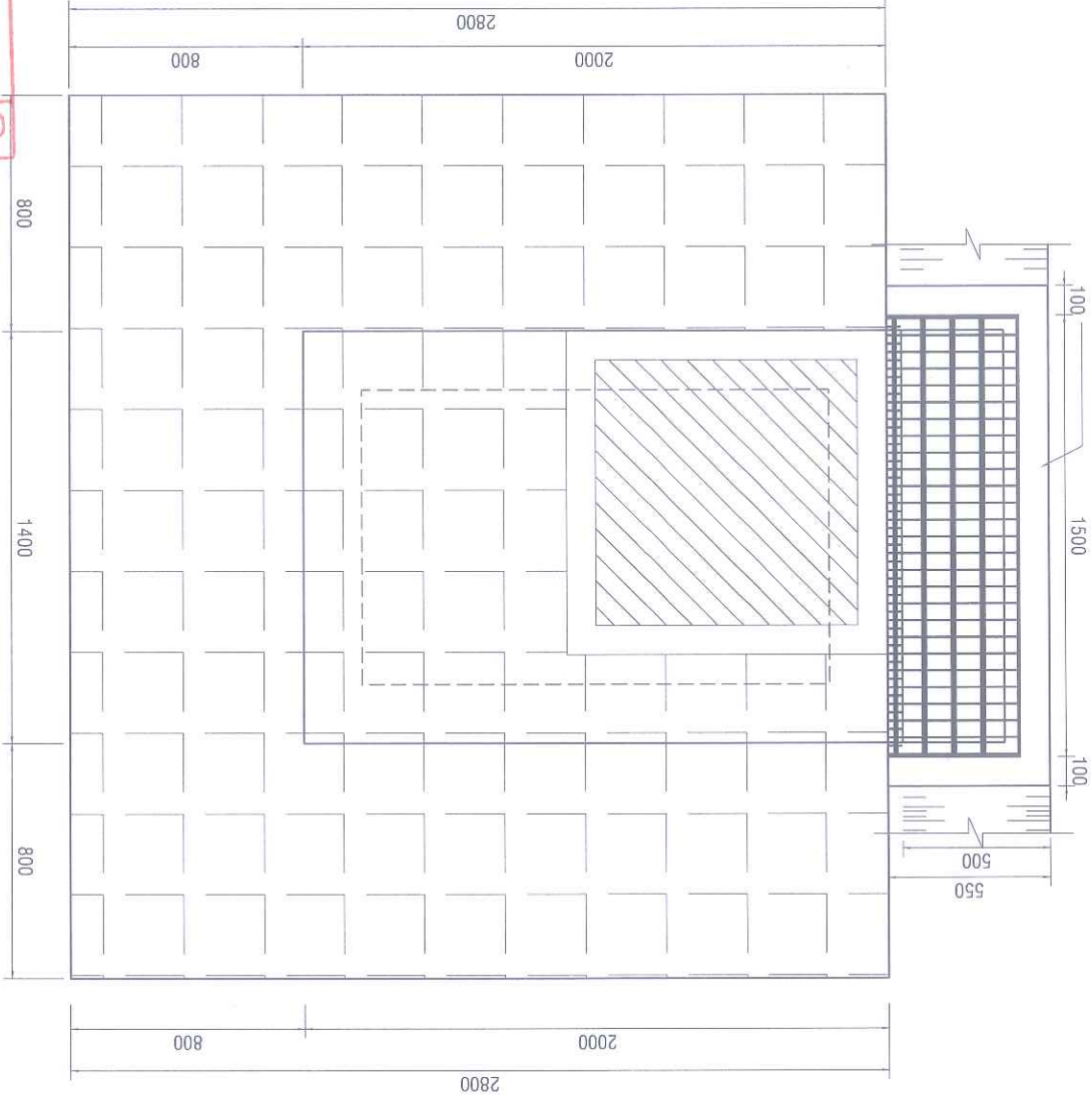
MẶT BẰNG CẢI TẠO VÍA HÈ ĐƯỜNG PHỤ RIỀNG ĐỎ TỶ LỆ: 1/25
