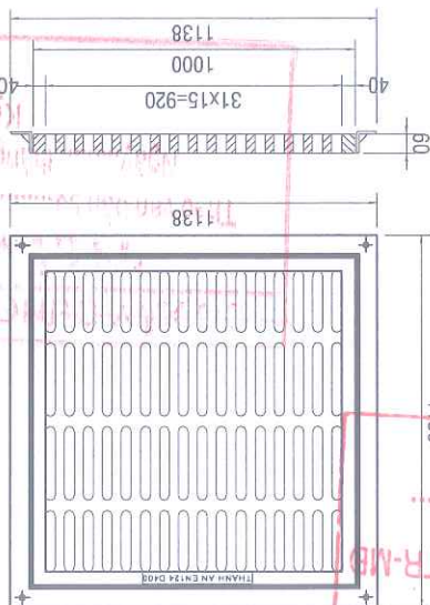
CHI TIẾT NÁP THU NƯỚC
