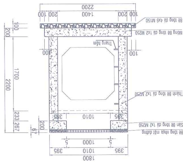
MẶT CẮT 1 - 1
