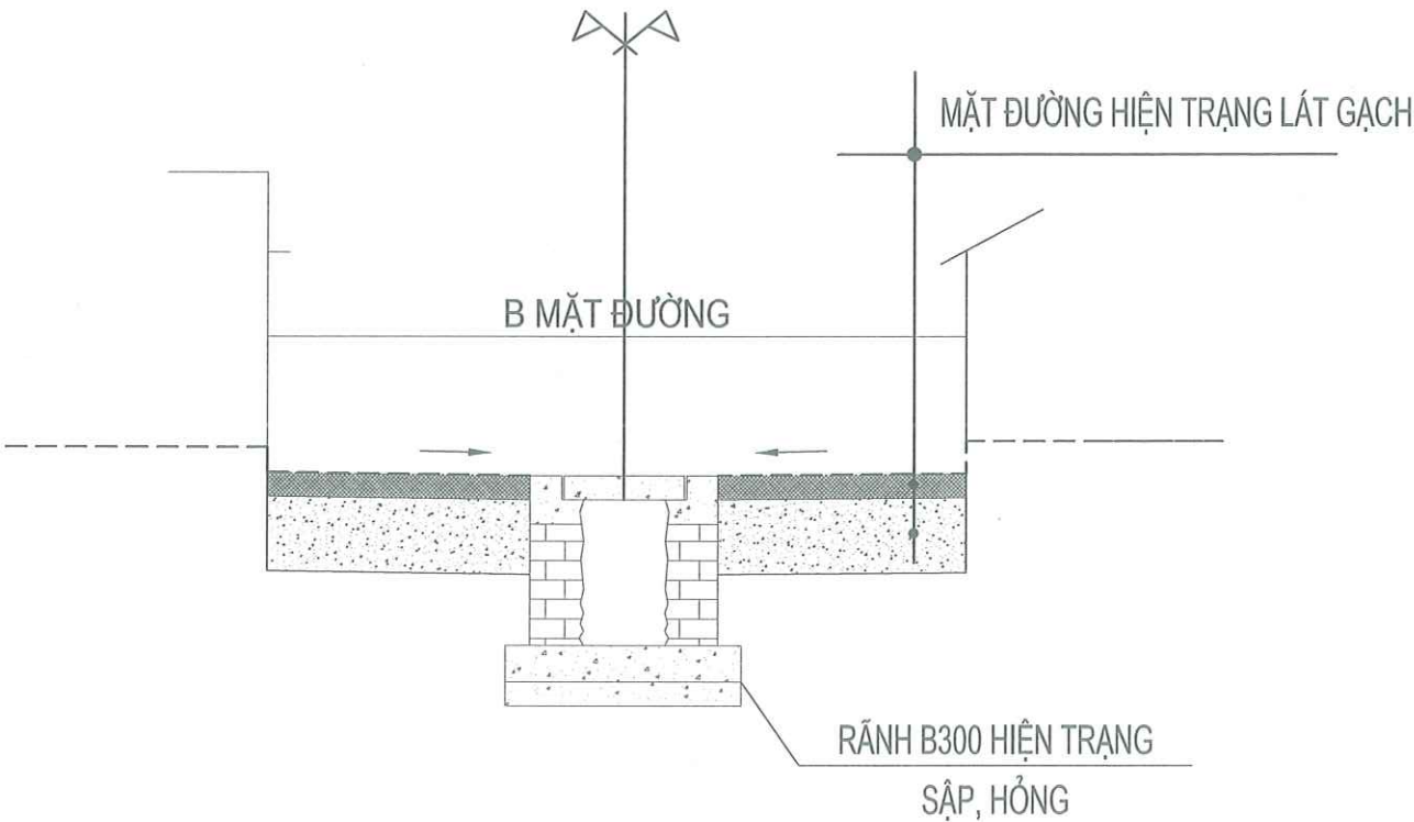
MẶT ĐƯỜNG HIỆN TRẠNG
