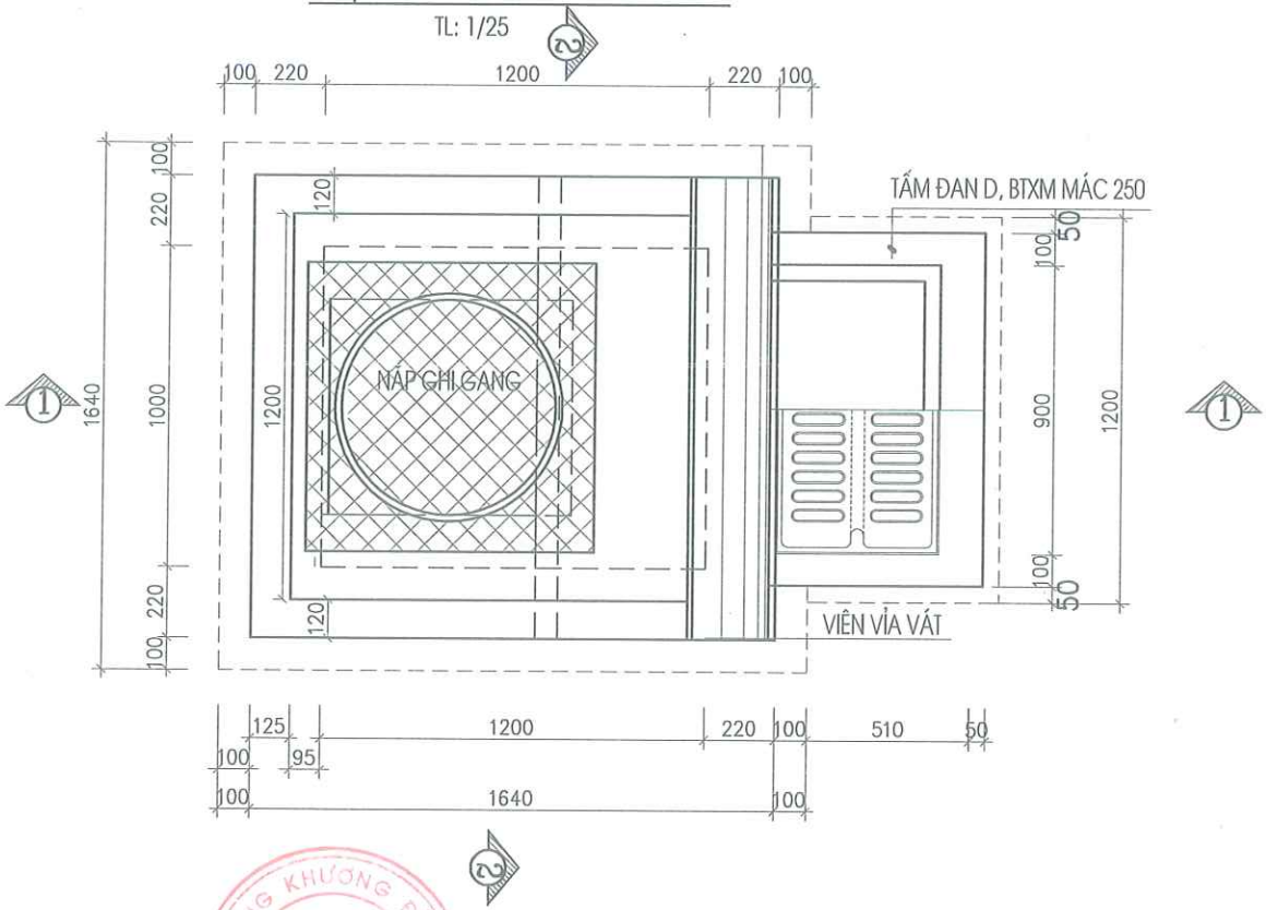
MẶT BẰNG GA HÀM ÉCH
