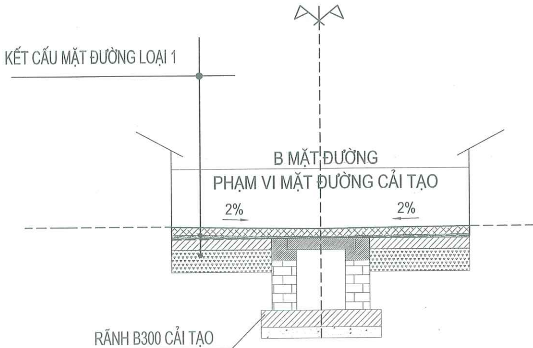
MẶT ĐƯỜNG CẢI TẠO Dặng văn Tuyên
