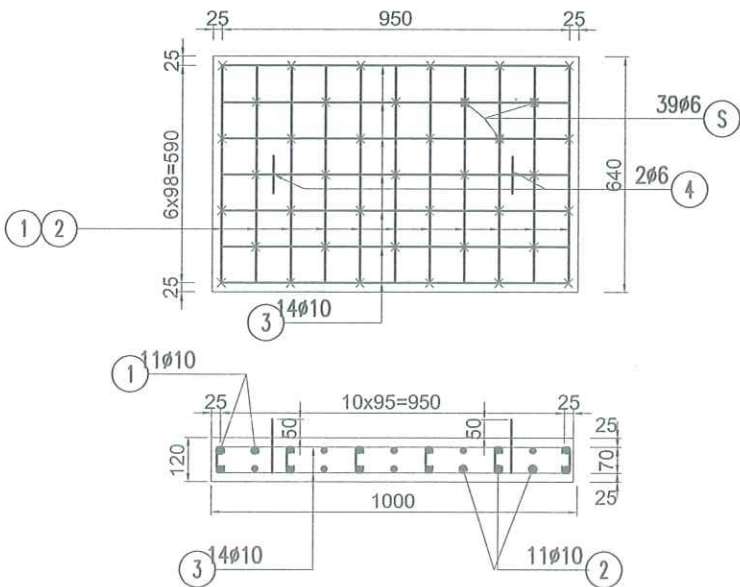
CHI TIẾT TẤM ĐƠN RÃNH
