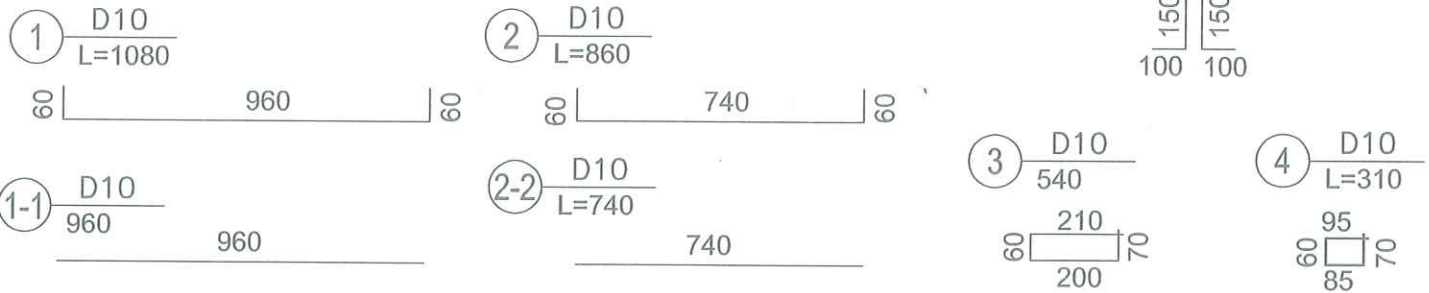
QUY CÁCH CỐT THÉP
