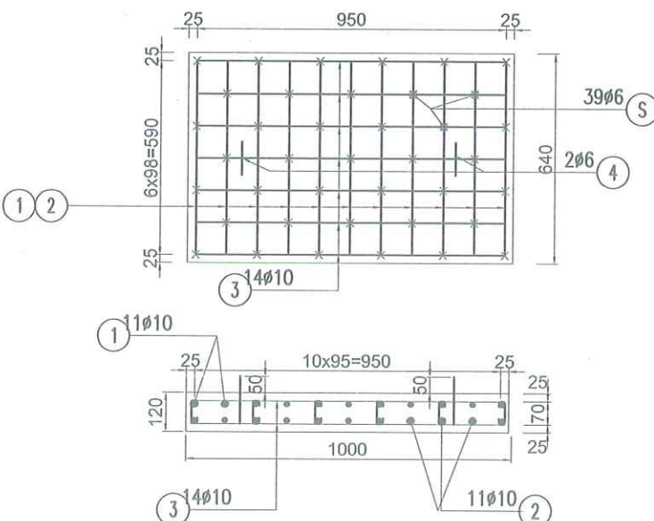
CHI TIẾT TẮM ĐƠN RÃNH
