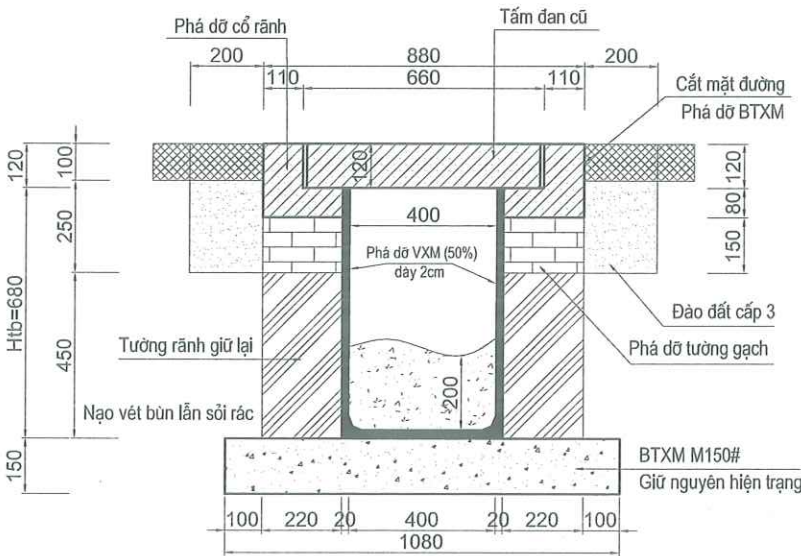
CHI TIẾT RÃNH THOÁT NƯỚC HIỆN TRẠNG
