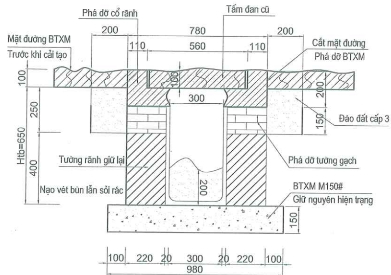
CHI TIẾT TẮM ĐƠN RÃNH
