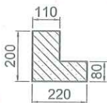
CHI TIẾT CỔ RÃNH
