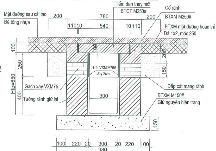
CHI TIẾT RÃNH THOÁT NƯỚC CẢI TẠO
