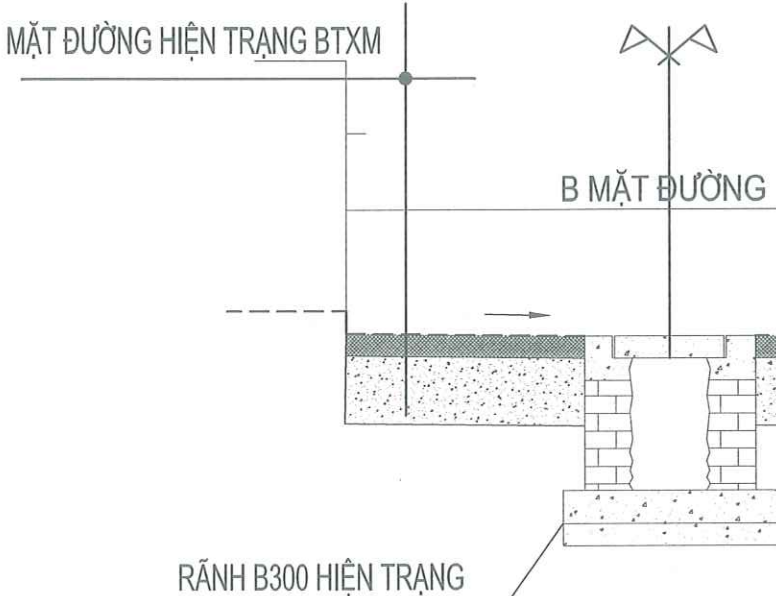
MẶT ĐƯỜNG CẢI TẠO ÁP DỤNG TỪ CỌC T11 ĐẾN CỌC D4
