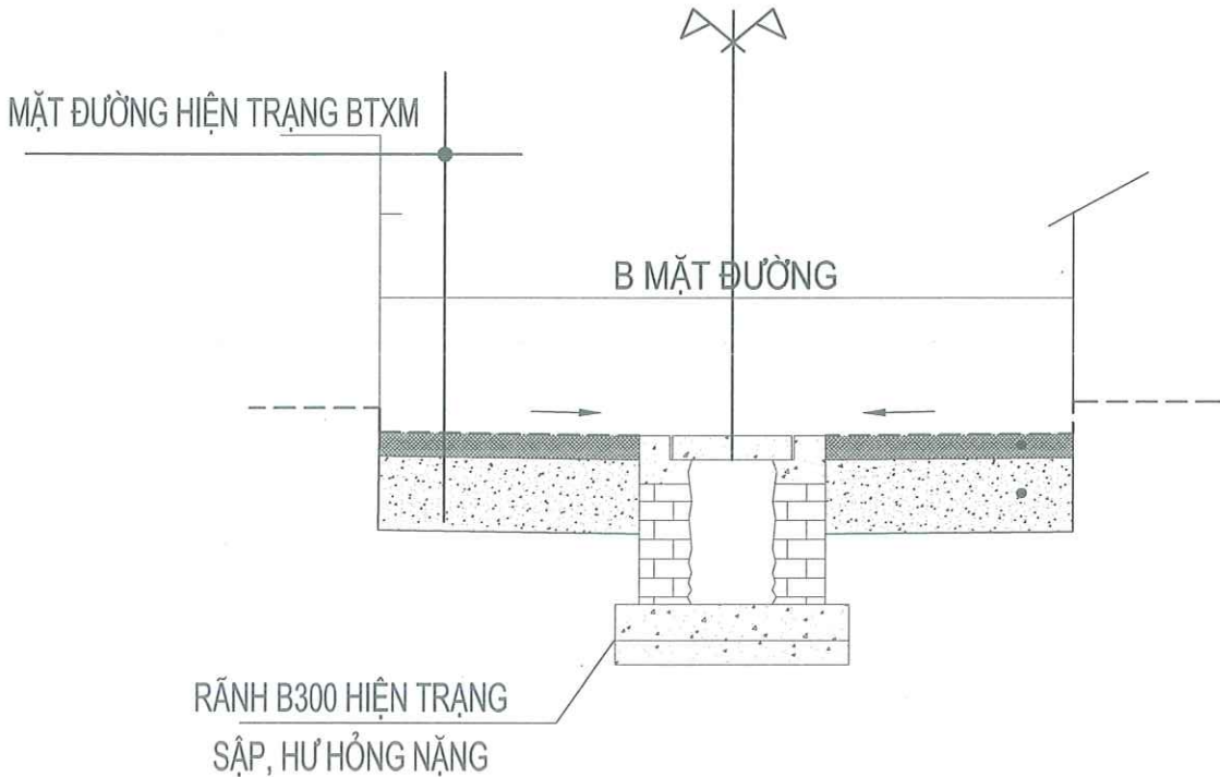
MẶT ĐƯỜNG HIỆN TRẠNG
