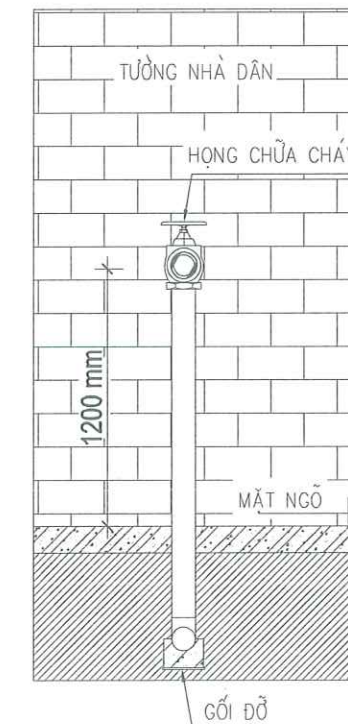
MẶT ĐÚNG HỌNG CHỮA CHÁY
