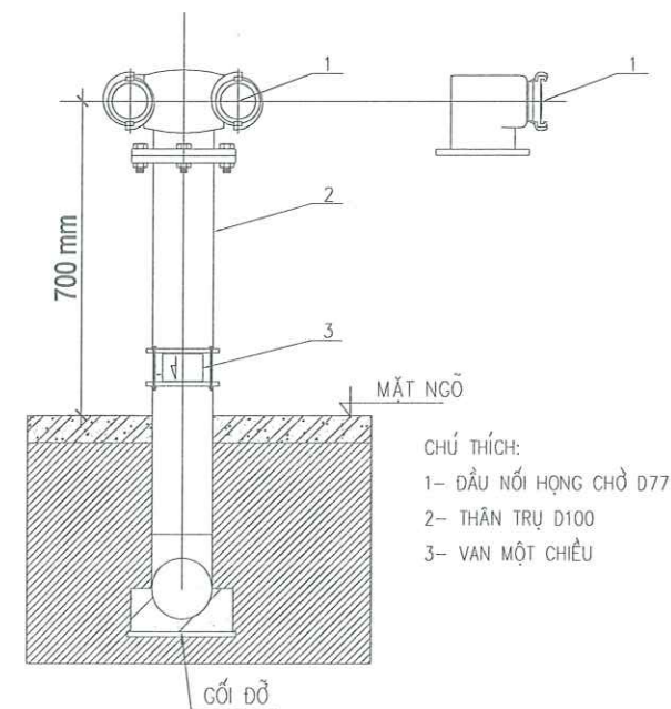
CHI TIẾT HỌNG LẤY NƯỚC O2
