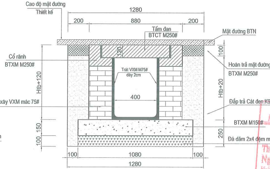
MẶT CẮT ĐÀO ĐẮP RÃNH
