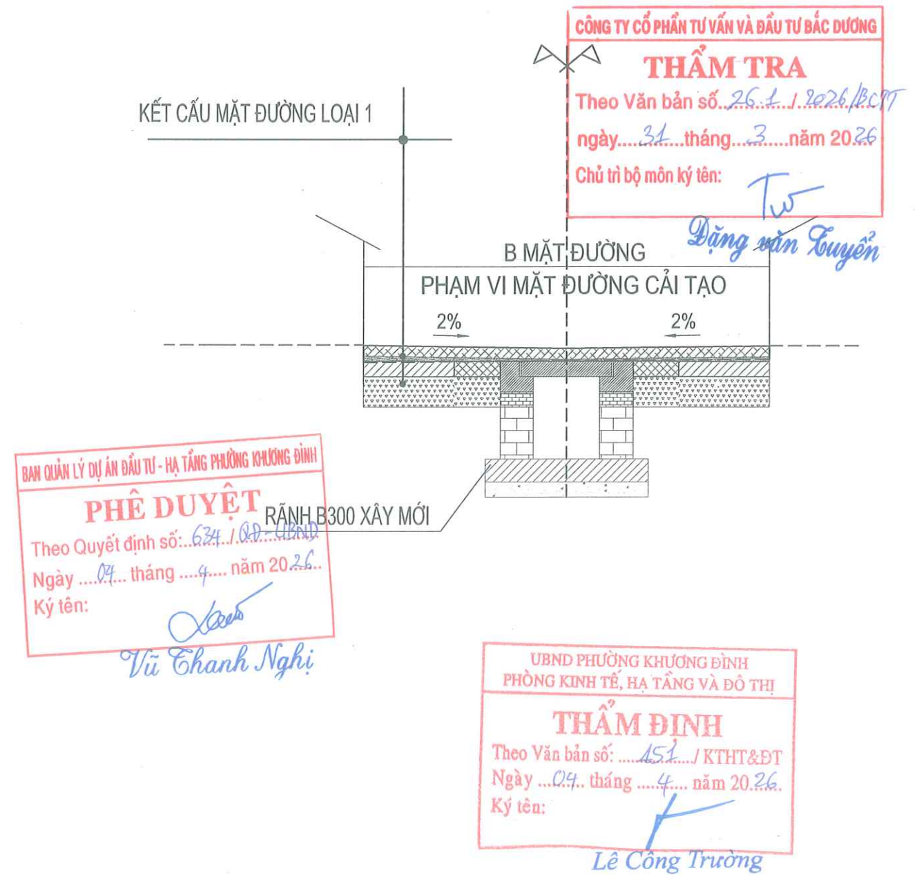
MẶT ĐƯỜNG CẢI TẠO
