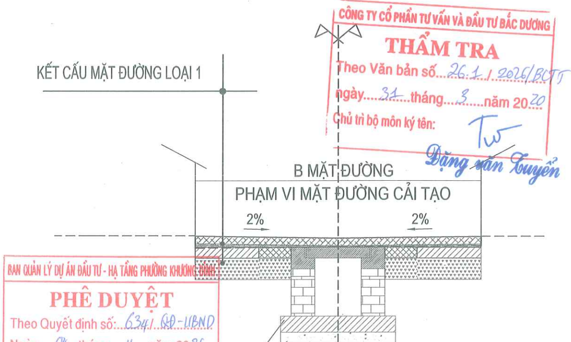
MẶT ĐƯỜNG CẢI TẠO
