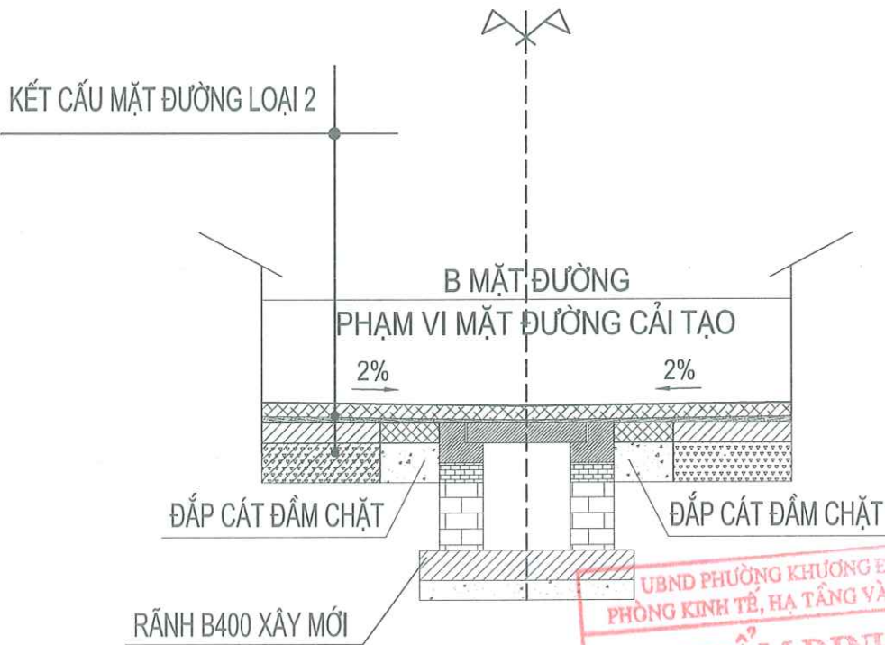
MẶT ĐƯỜNG CẢI TẠO
