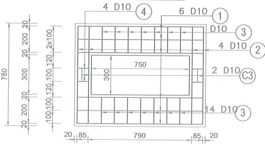
CHI TIẾT TẤM ĐAN D
