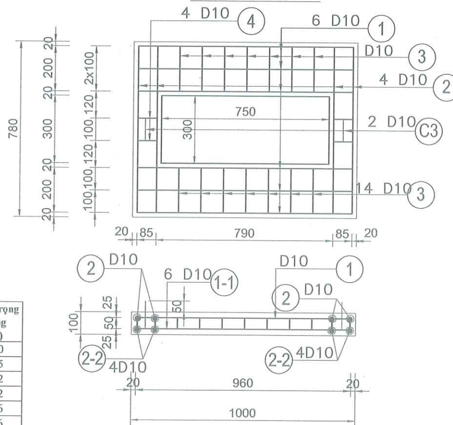
CHI TIẾT TẮM ĐẠN D
