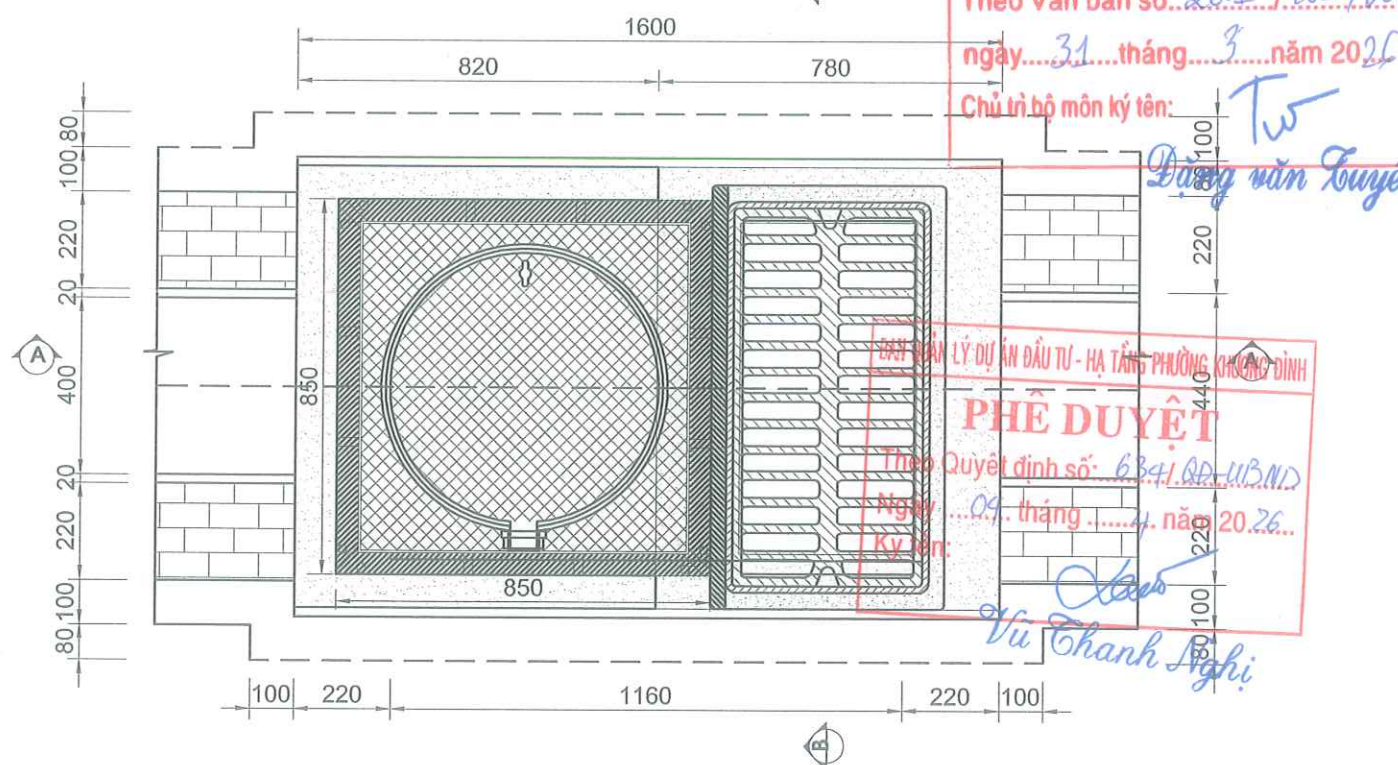
MẶT BẰNG HỒ GA TL: 1/25
