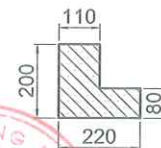
CHI TIẾT CỔ RÃNH
