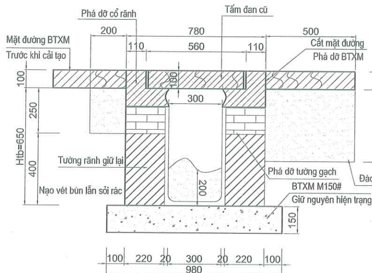
CHI TIẾT TẤM ĐAN RÃNH
