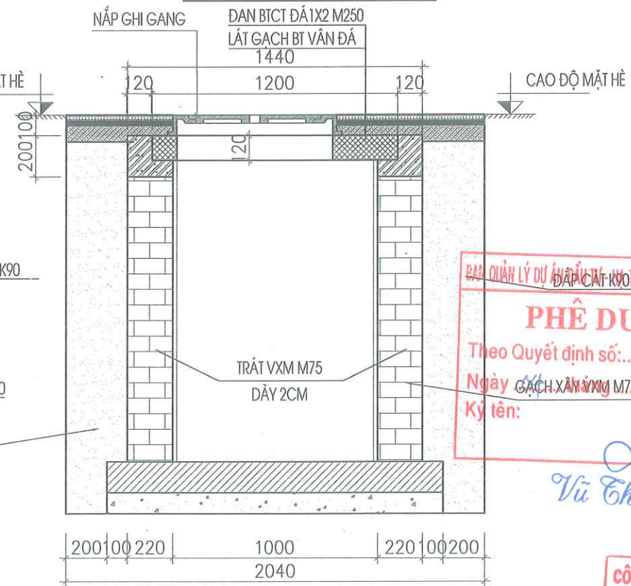
MẶT CẮT ĐÀO ĐẮP 2-2
