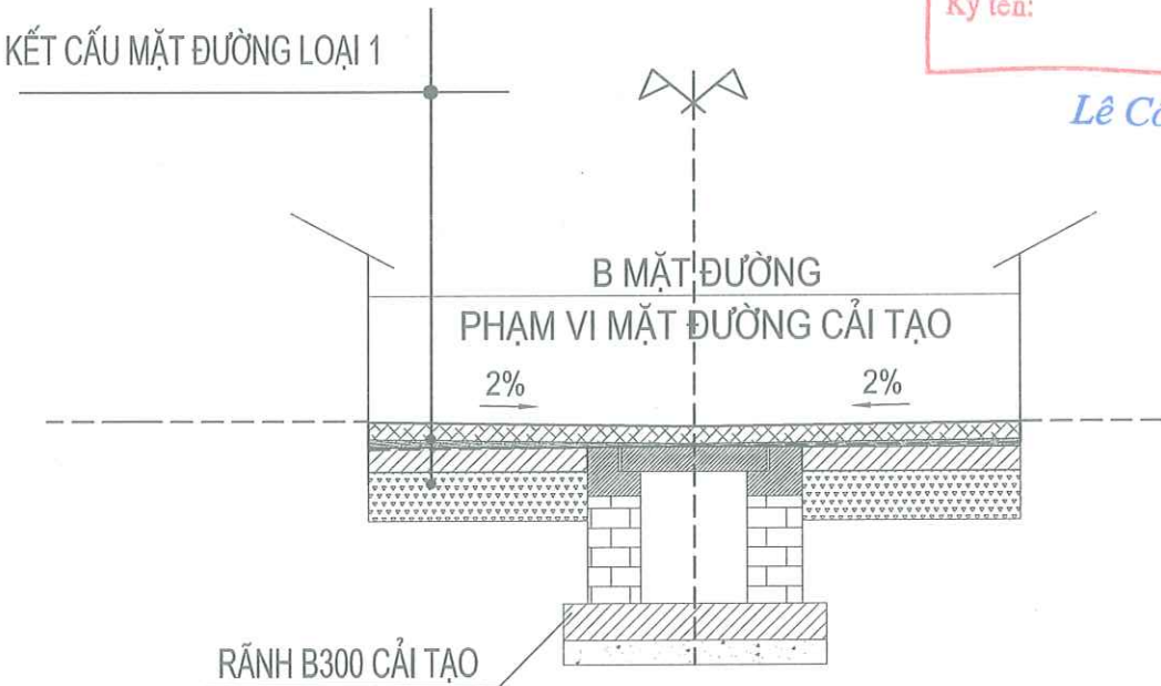
MẶT ĐƯỜNG CẢI TẠO ÁP DỤNG TỪ CỌC T11 ĐẾN CỌC D4
