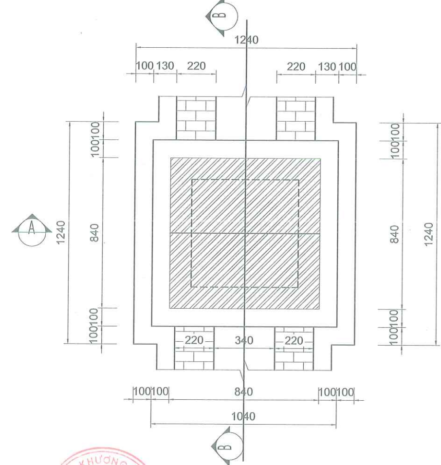
MẶT BẰNG HỒ GA TL: 1/25
