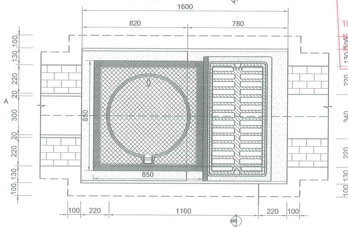
MẶT BẰNG HỐ GA TL: 1/25
