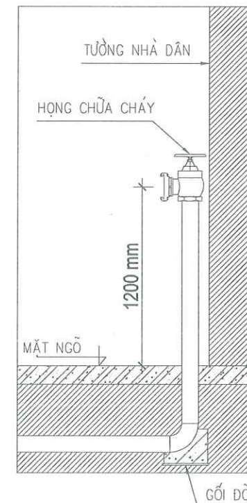
MẶT CẮT HỌNG CHỮA CHÁY
