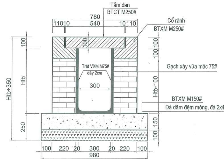
CHI TIẾT RÃNH THOÁT NƯỚC B300
