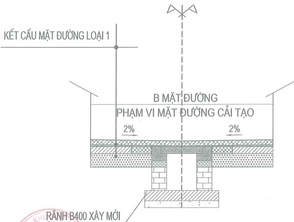
MẶT ĐƯỜNG CẢI TẠO ÁP DỤNG TỪ CỌC DT9 ĐẾN CỌC T11
