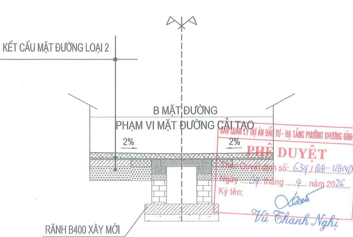
MẶT ĐƯỜNG CẢI TẠO
