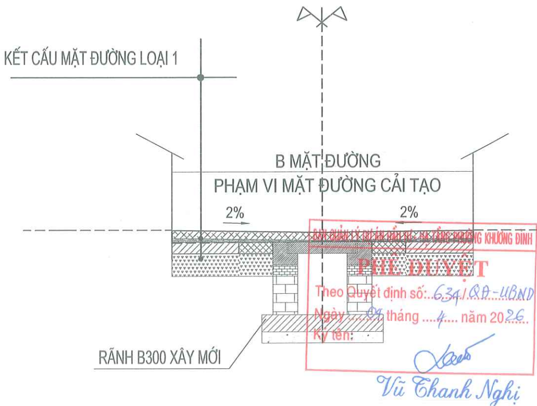
MẶT ĐƯỜNG CẢI TẠO Dặng văn Tuyên
