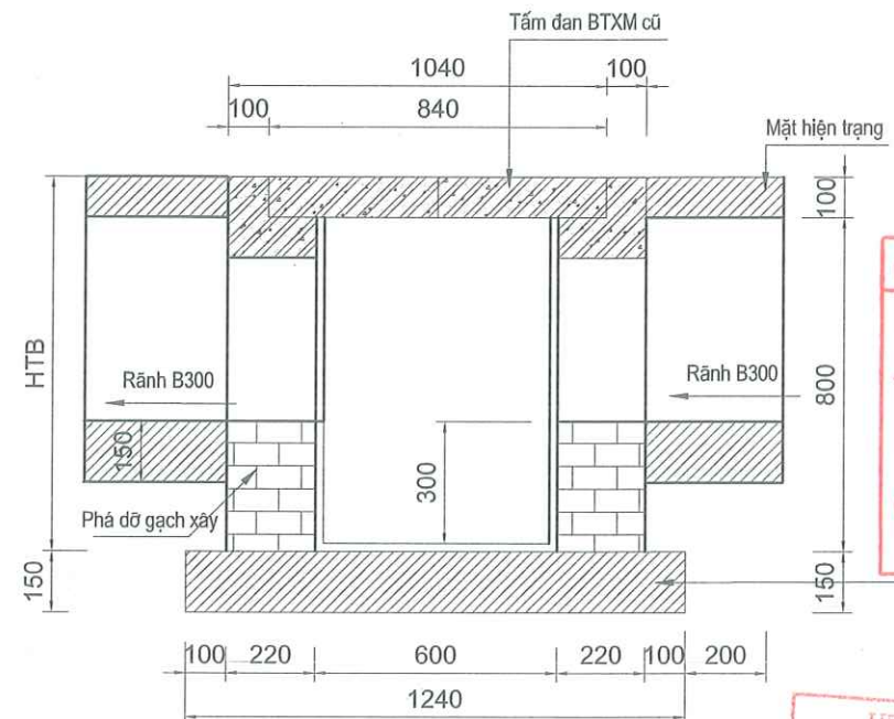
MẶT CẮT B-B TL: 1/25
