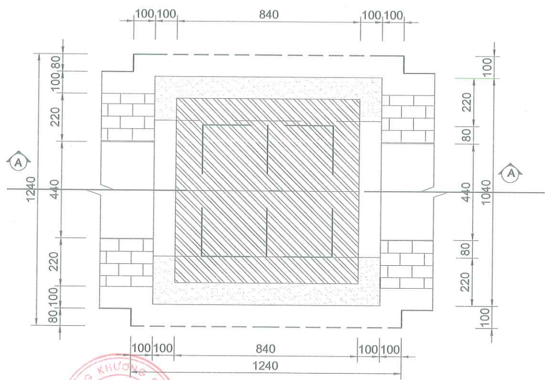
MẶT BẰNG HỒ GA HIỆN TRẠNG TL: 1/25
