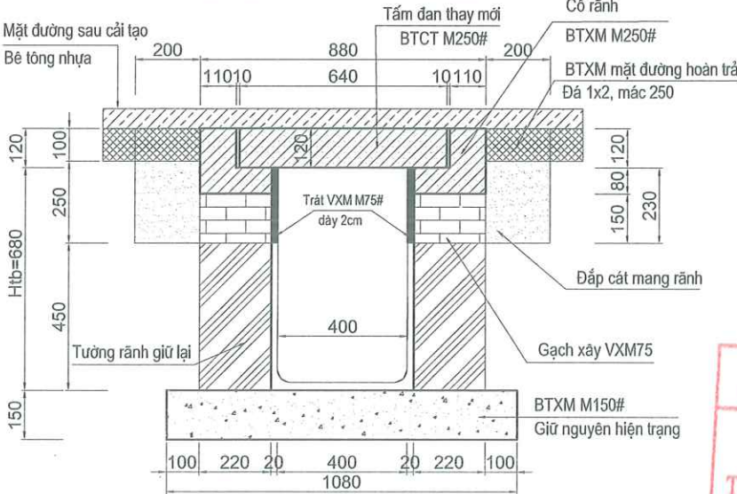
CHI TIẾT RÃNH THOÁT NƯỚC CẢI TẠO
