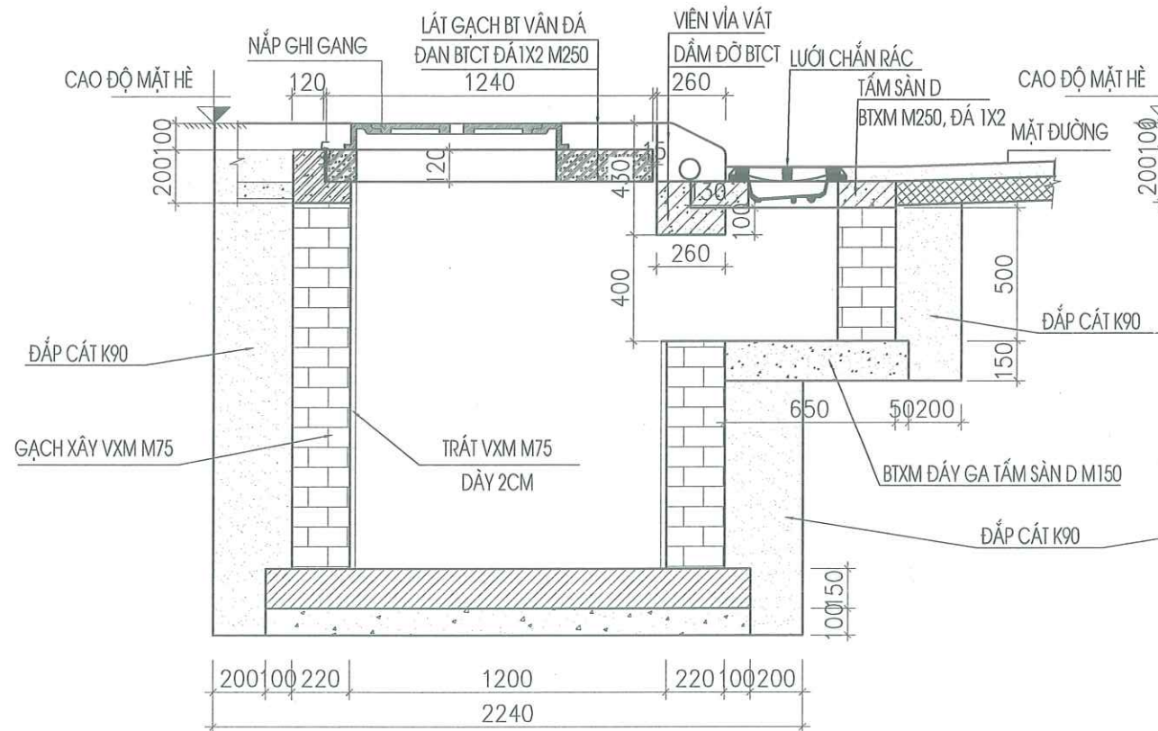
MẶT CẮT ĐÀO ĐẮP 1-1
