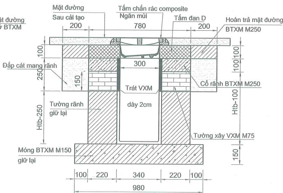
CHI TIẾT RÃNH CẢI TẠO
