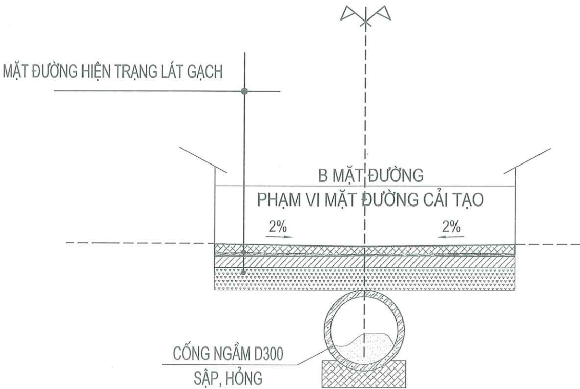
MẶT ĐƯỜNG HIỆN TRẠNG
