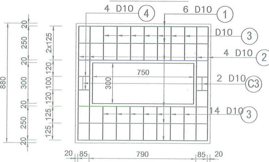
CHI TIẾT TẮM ĐẠN D
