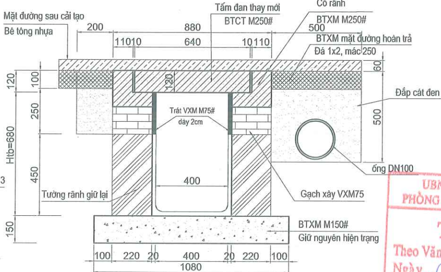
CHI TIẾT RÃNH THOÁT NƯỚC CẢI TẠO
