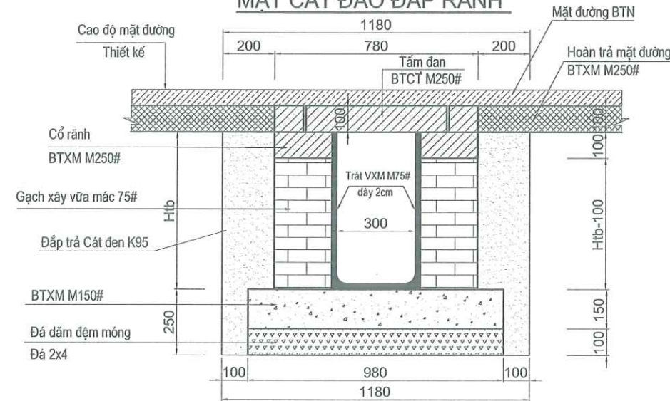
MẶT CẮT ĐÀO ĐẮP RÃNH
