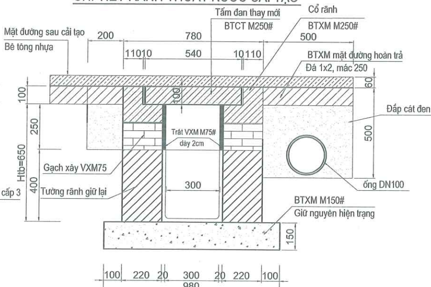
CHI TIẾT RÃNH THOÁT NƯỚC CẢI TẠO
