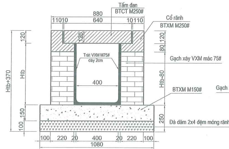
CHI TIẾT TẤM ĐAN RÃNH
