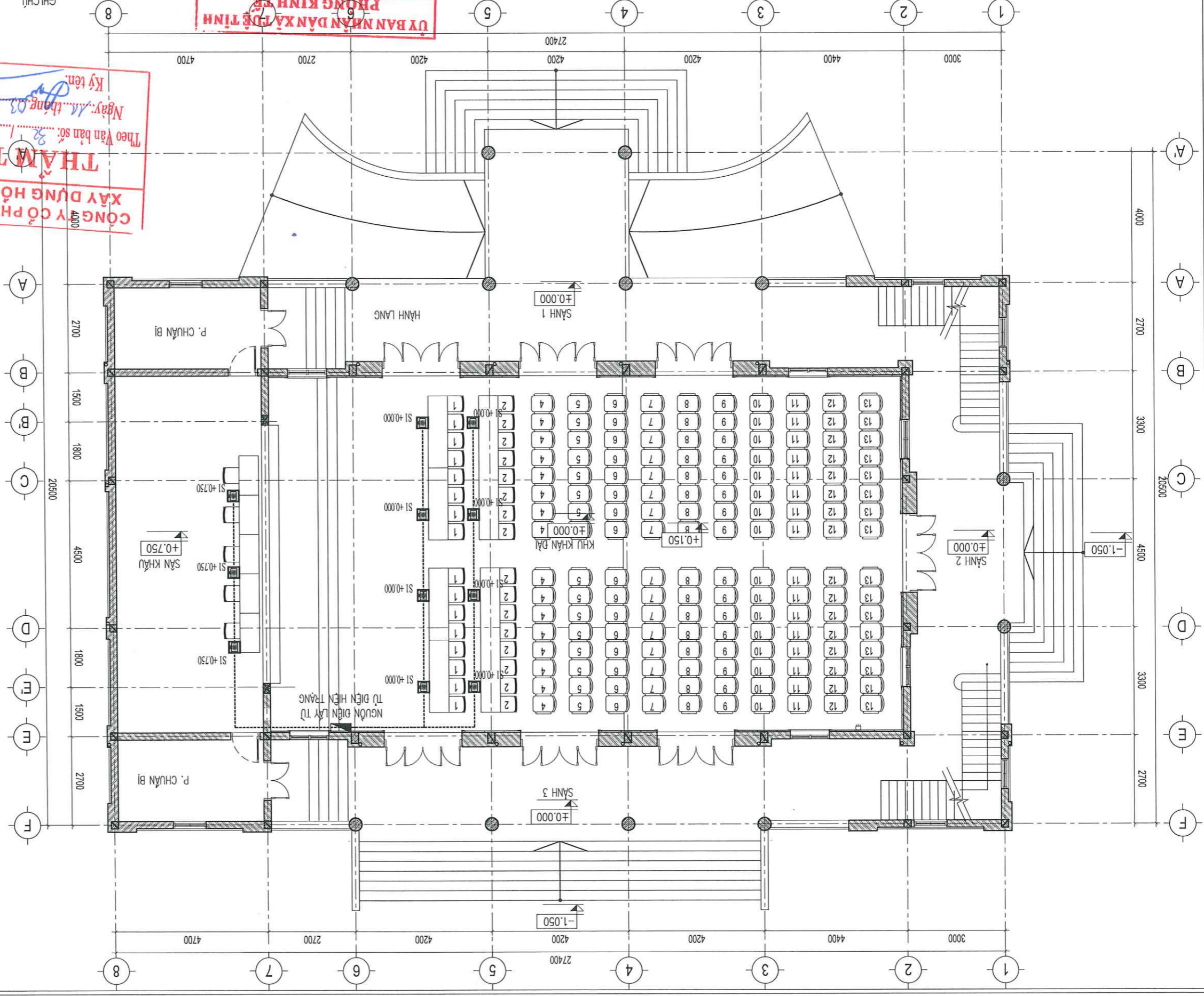
MẶT BẰNG Ồ CẦM
