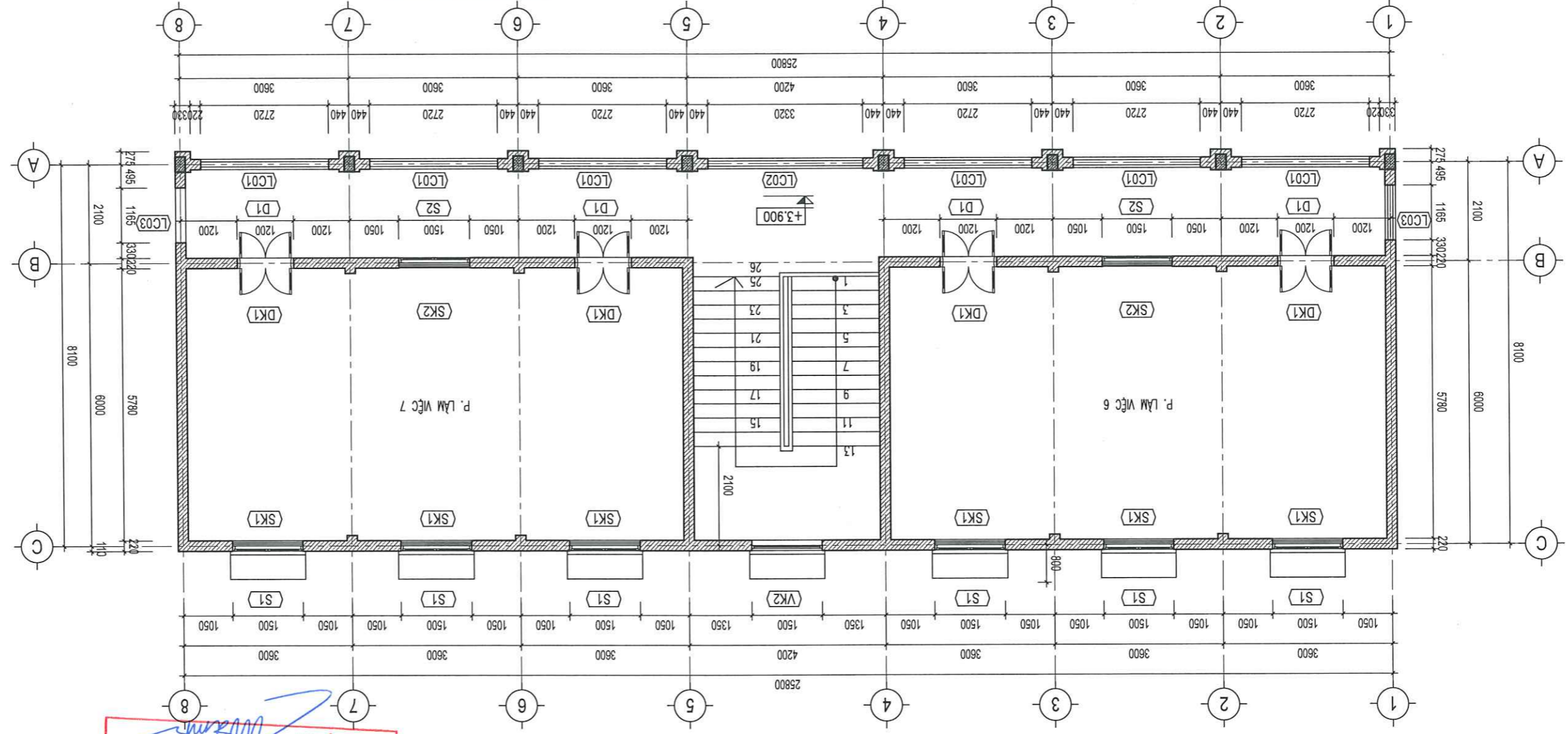
MẶT BẰNG HIỆN TRẠNG TẦNG 2
