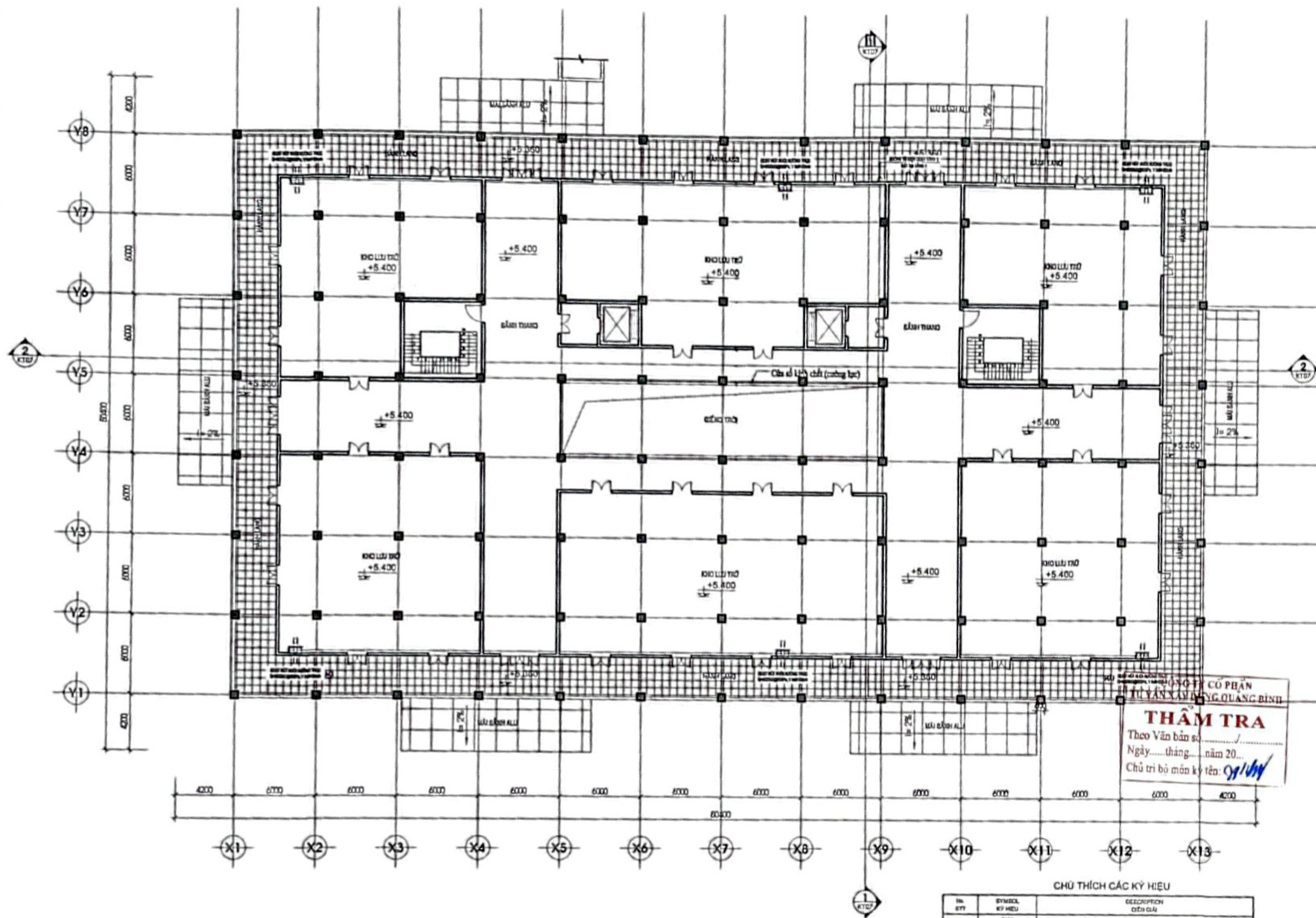
1 MẶT BẰNG TẦNG 2 T/L: 1/100
