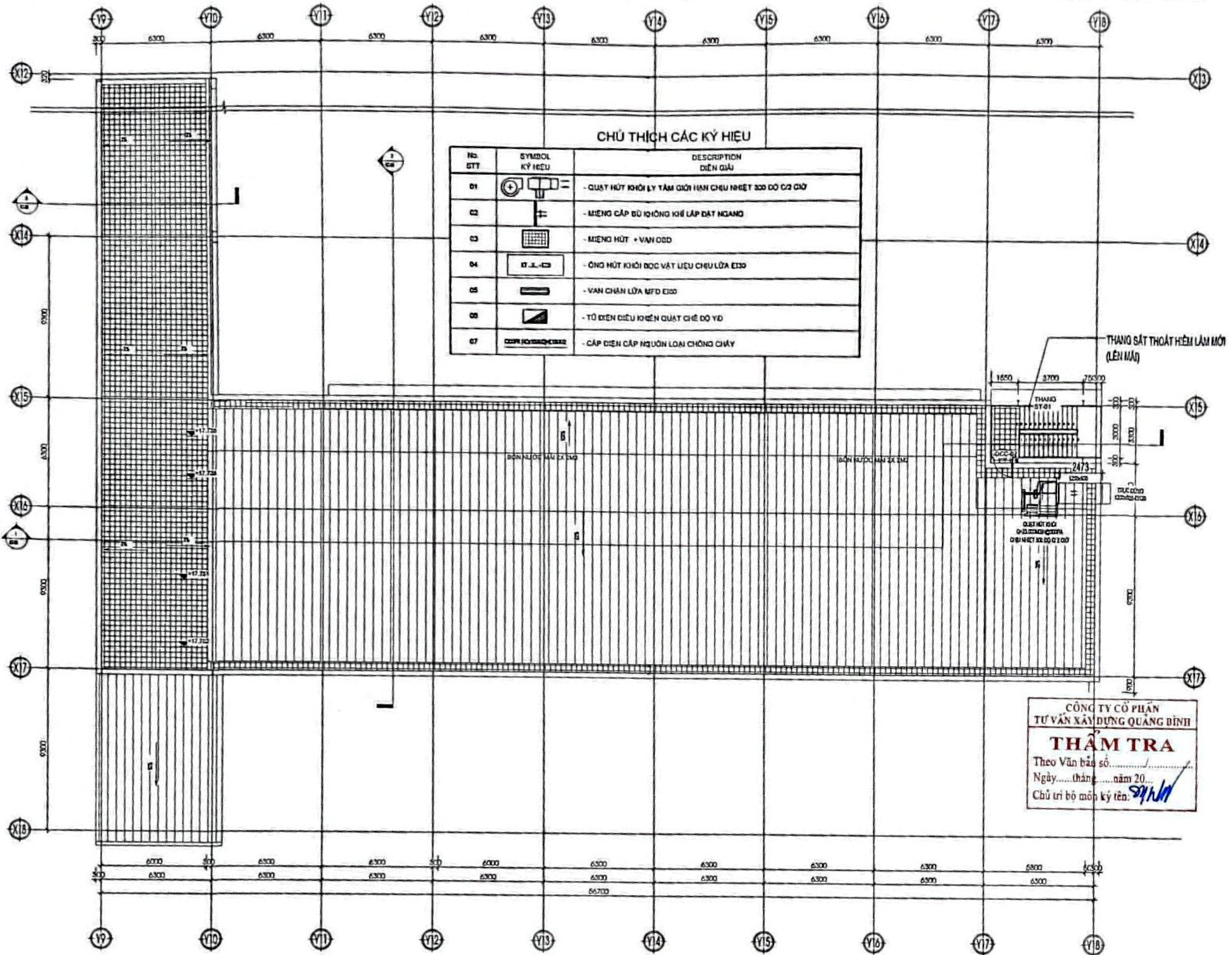
MẶT BẰNG TẦNG TUM (LÀM MỚI) T.L 1:100
