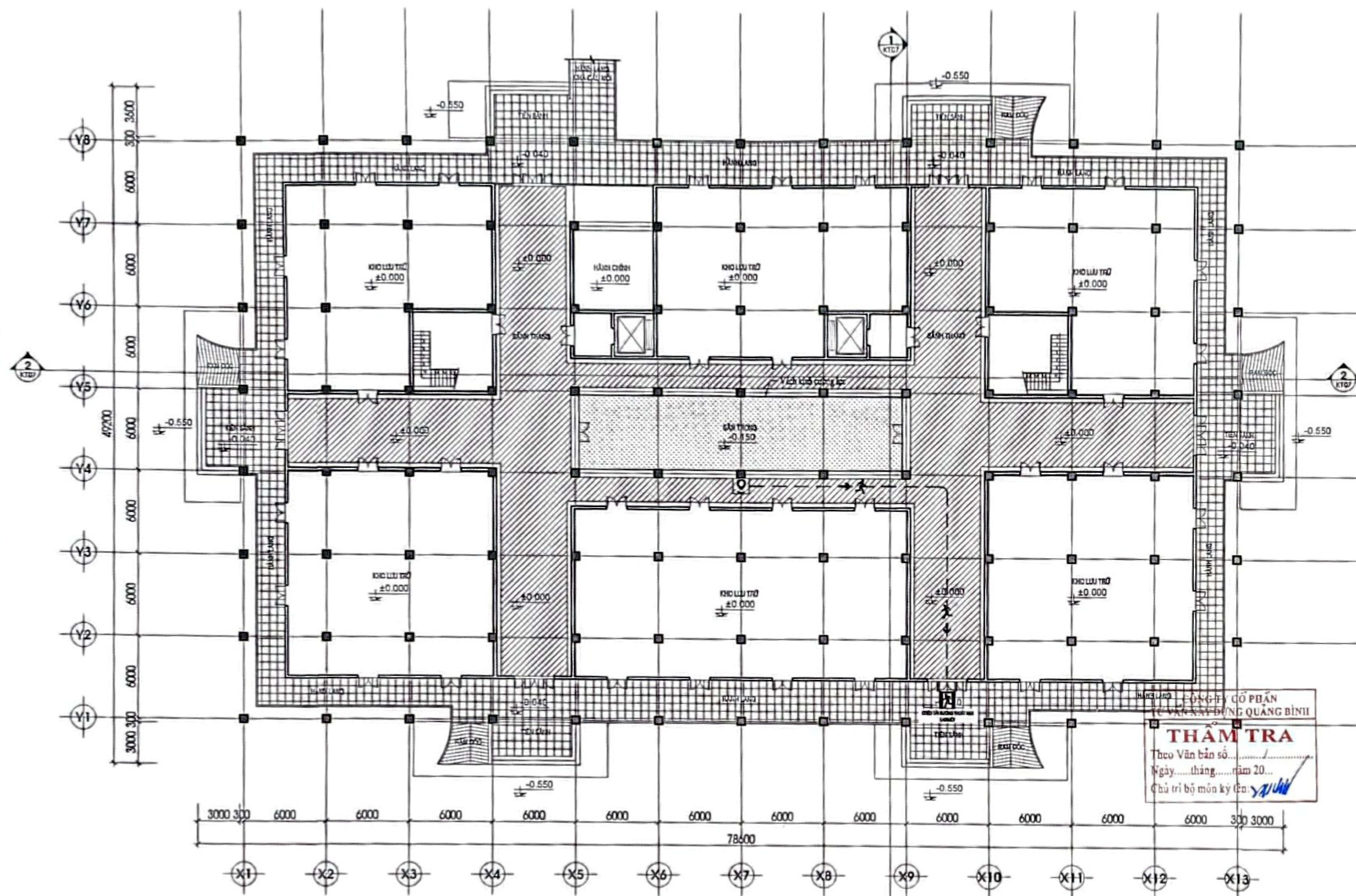
1 MẶT BẰNG TẦNG 1 T/L: 1/100
