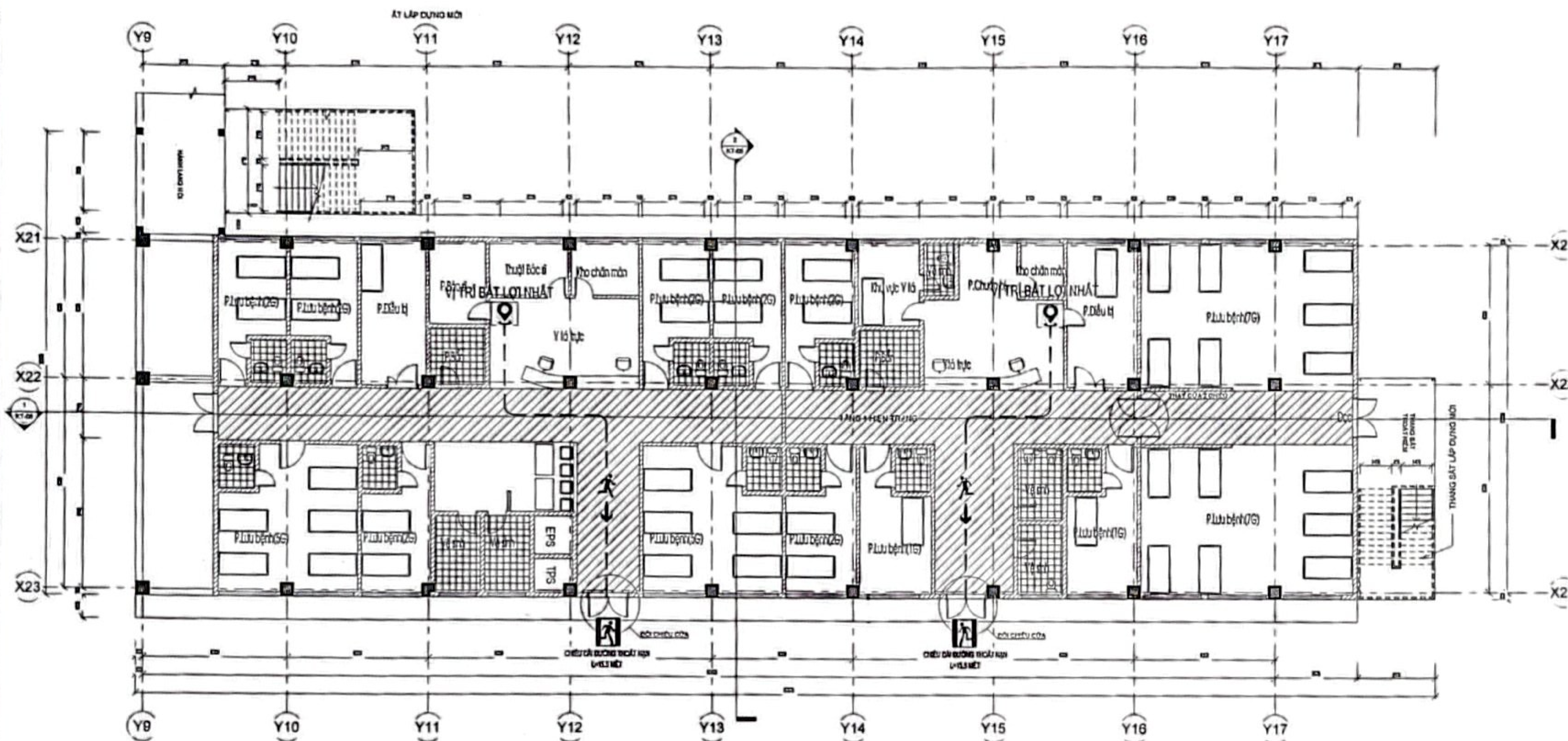
MẶT BẰNG TẦNG 1 (HIỆN TRẠNG) TL 1:100
