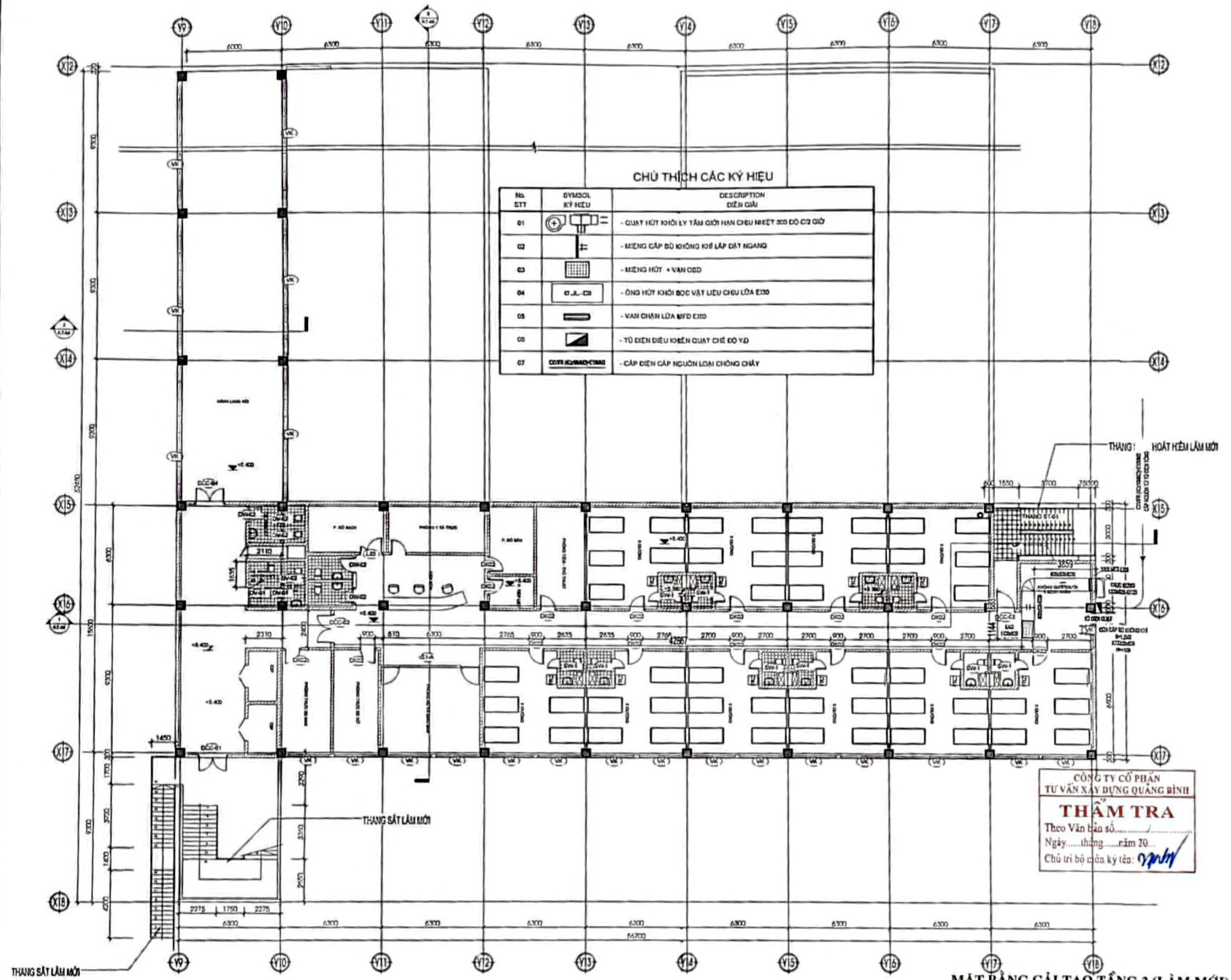
MẶT BẰNG CẢI TẠO TẦNG 2 (LÀM MỚI) TL 1:100
