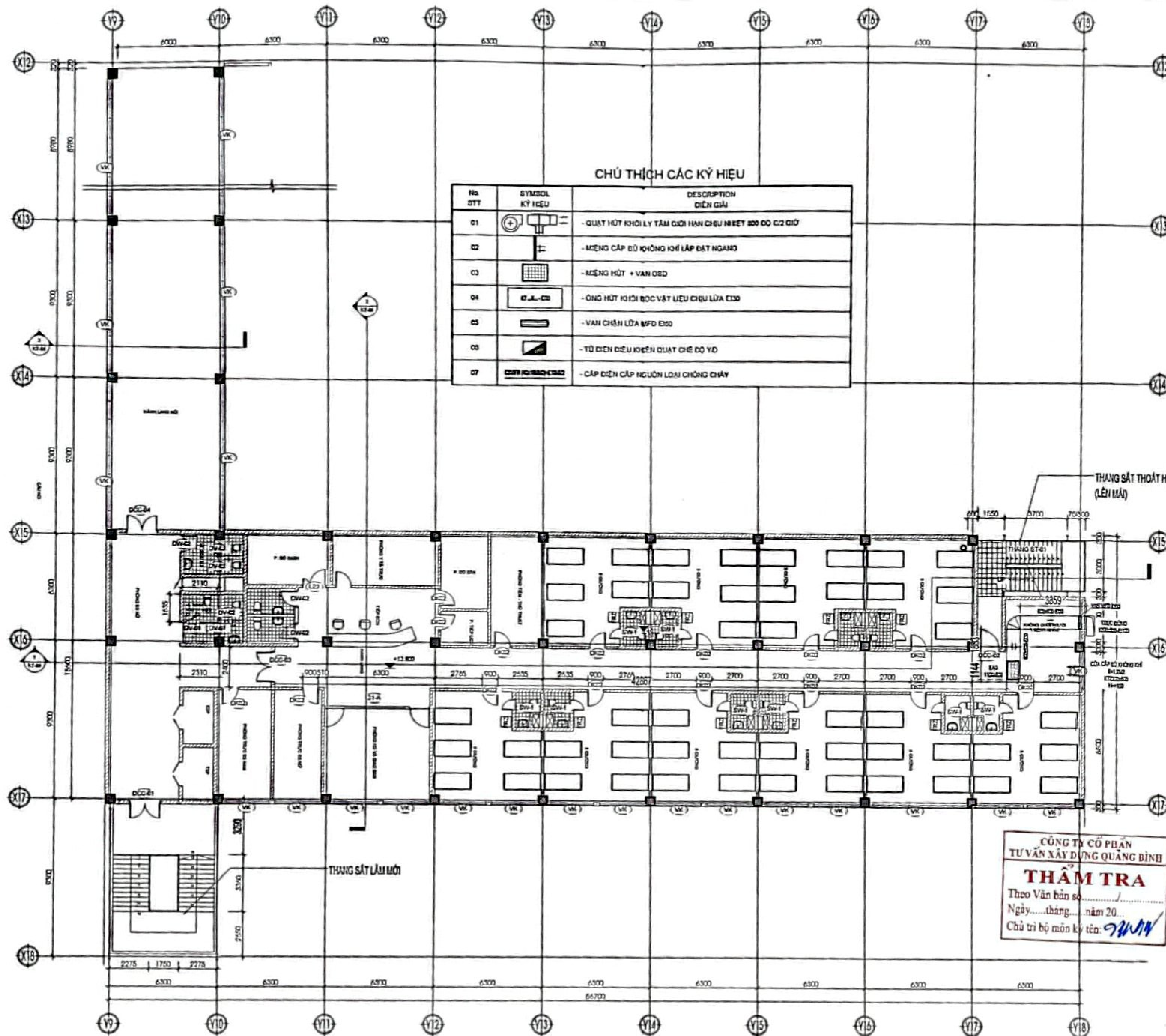
MẶT BẰNG TẦNG 4 (LÀM MỚI) T.L 1:100
