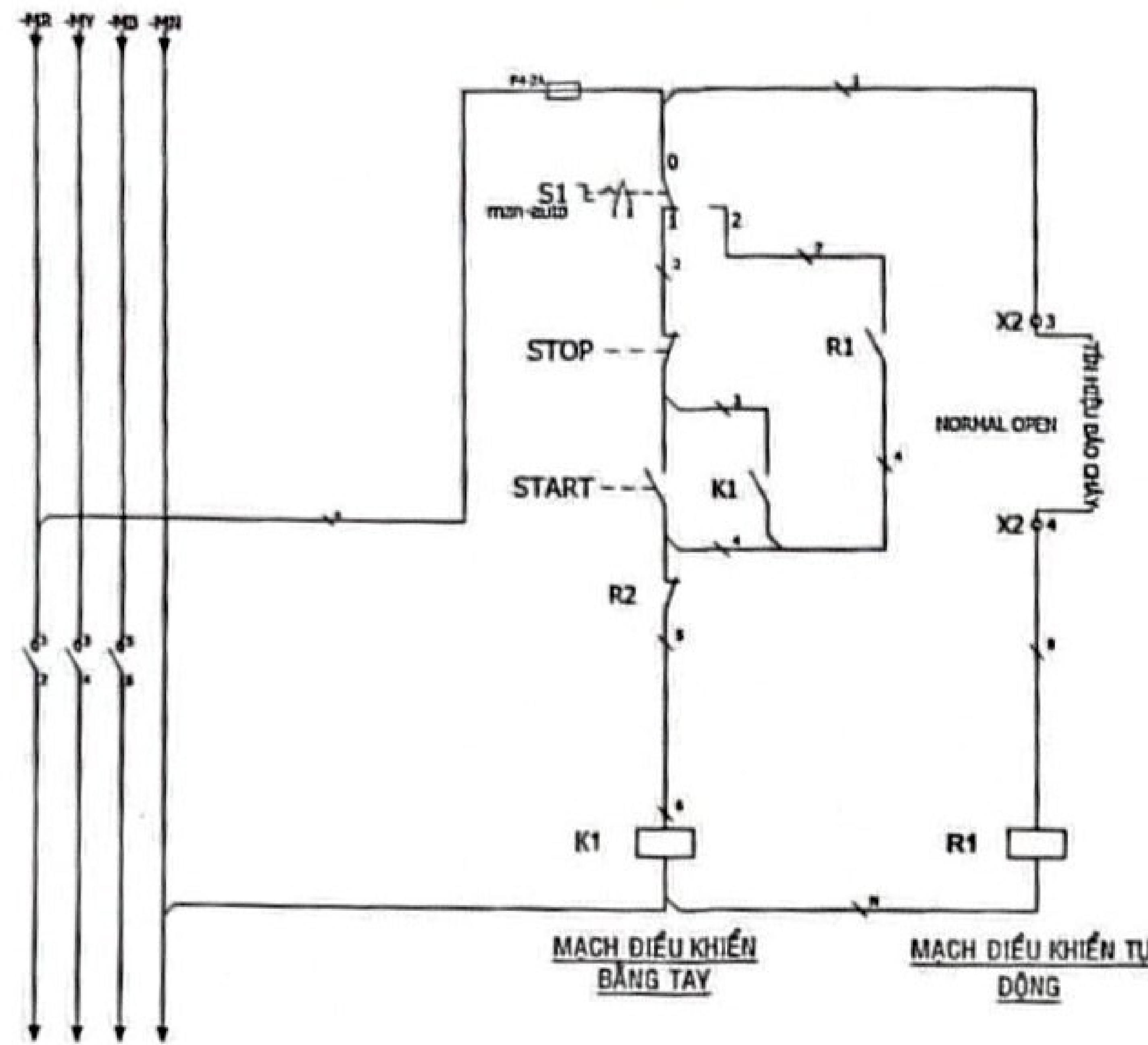
SƠ ĐỒ NGUYÊN LÝ MẠCH ĐIỀU KHIỂN ĐIỂN HÌNH QUẠT HÚT KHÓI
