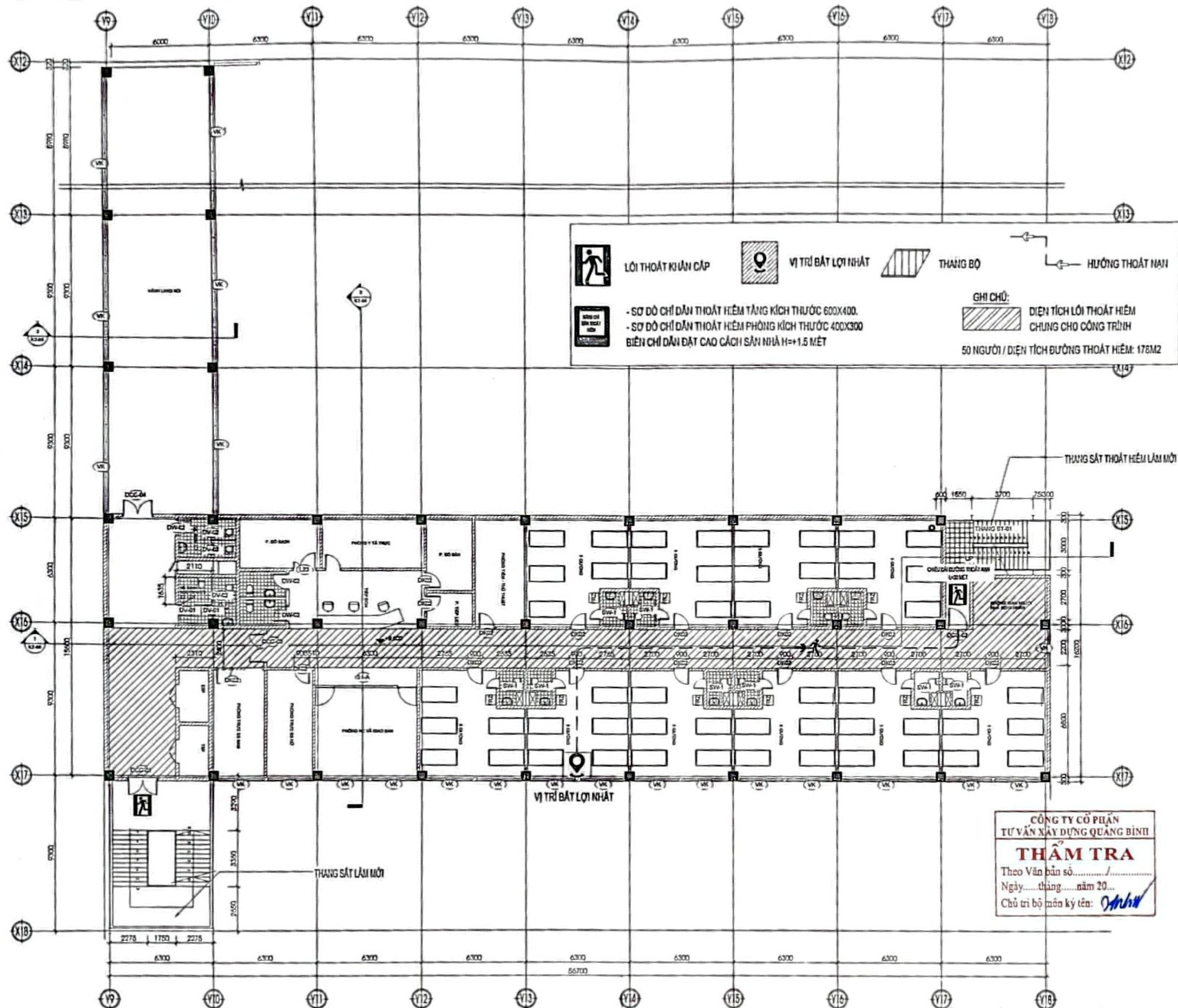
MẶT BẰNG TẦNG 3 (LÀM MỚI) TL 1:100
