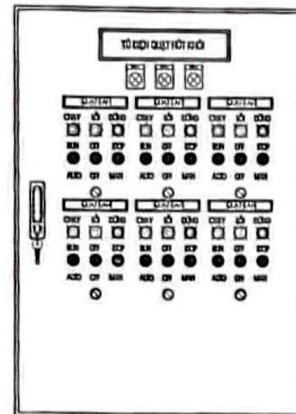
TỦ ĐIỆN ĐIỀU KHIỂN QUẠT HÚT KHÓI TẦNG 1 NHÀ KHO
