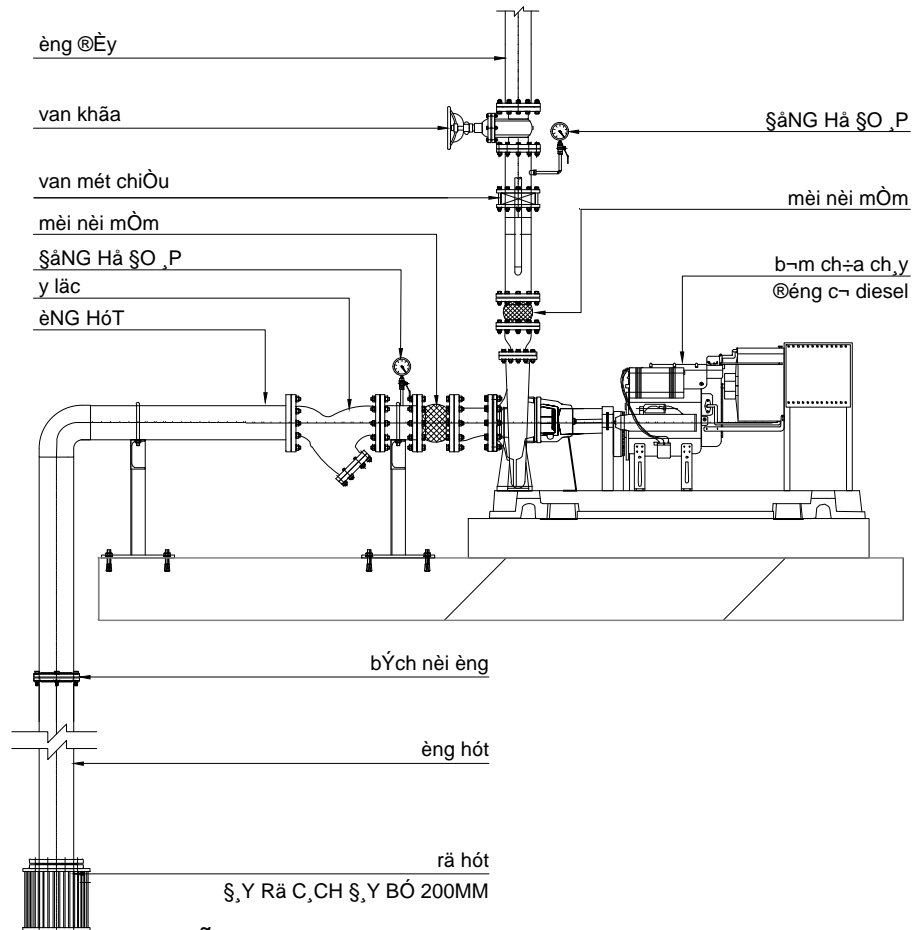
chi tiÕt 1/4p @Æt b-m tróc ngang şéNG C¥ DIESEL
