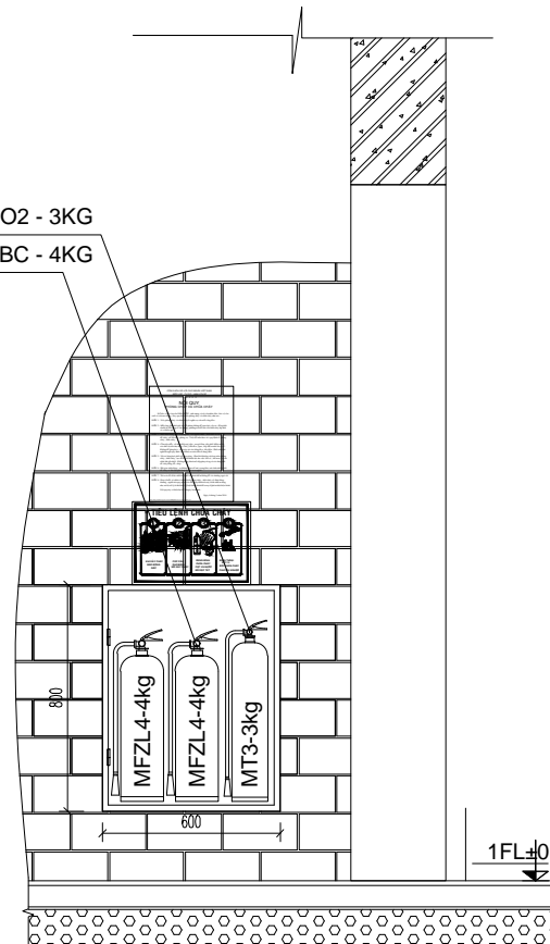
CHI TI T L P I N HÌNH T T NG BÌNH CH A CHÁY
