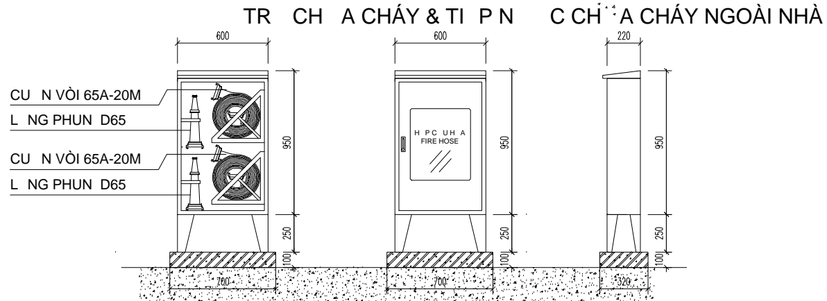
CHI TI T T CH A CHÁY NGOÀI NHÀ
