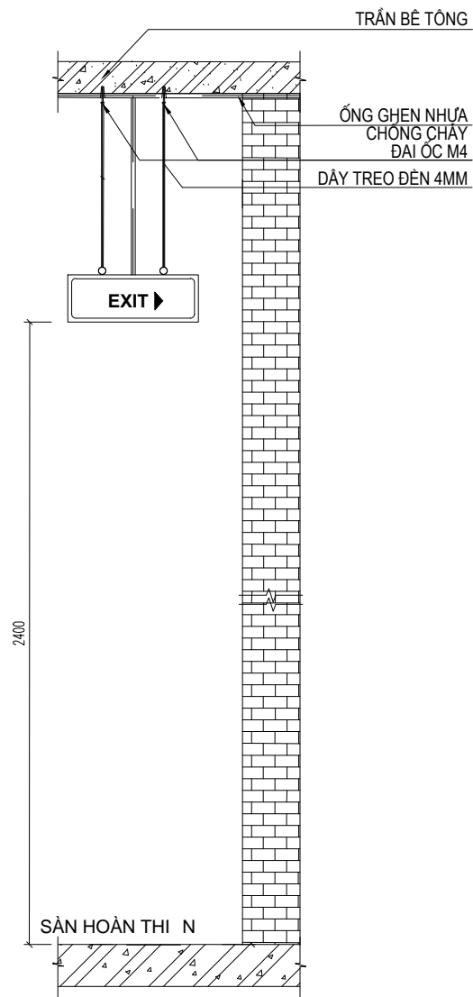
CHI TIẾT LẮP ĐẶT ĐÈN CHỈ LỐI THOÁT NẠN EXIT KHU VỰC KHÔNG CÓ TRẦN GIẢ
