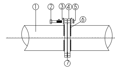
chi tiÕt 1/4p bÝch
