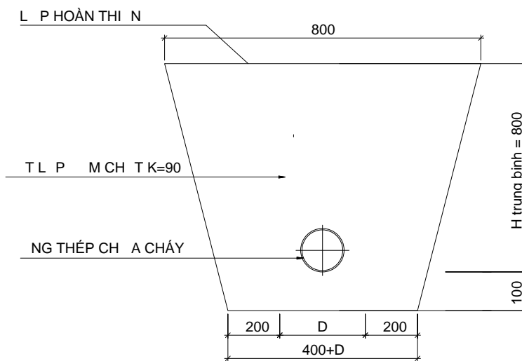
M T C T I N HÌNH M NG T NG THÉP
