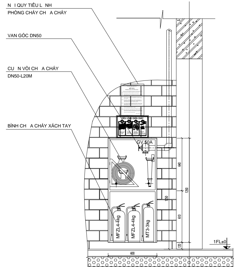
CHI TI TL P I N HÌNH TT CH A CHÁY VÁCH T NG
