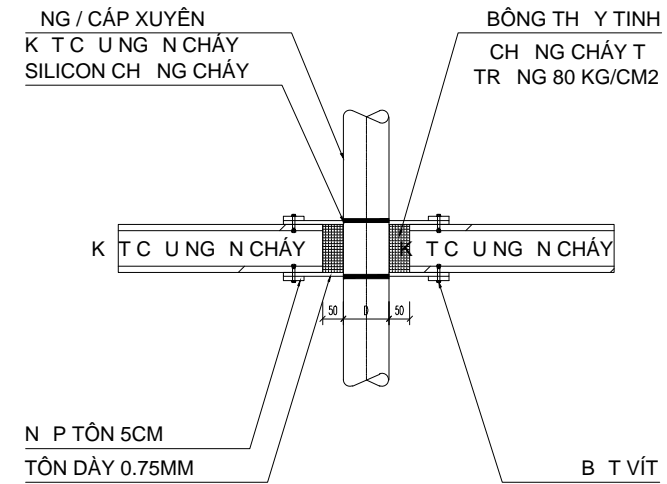
CHI TI T NG I QU A VÁCH NG N CHÁY
