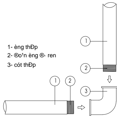
chi tiÕt 1/4p cõt ren
