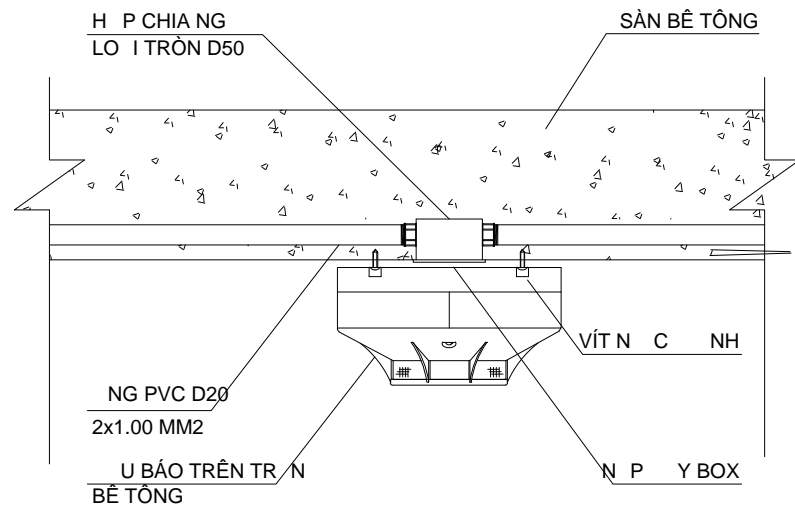
CHI TI T L P T U BẢO D I TR N BÊ TÔNG
