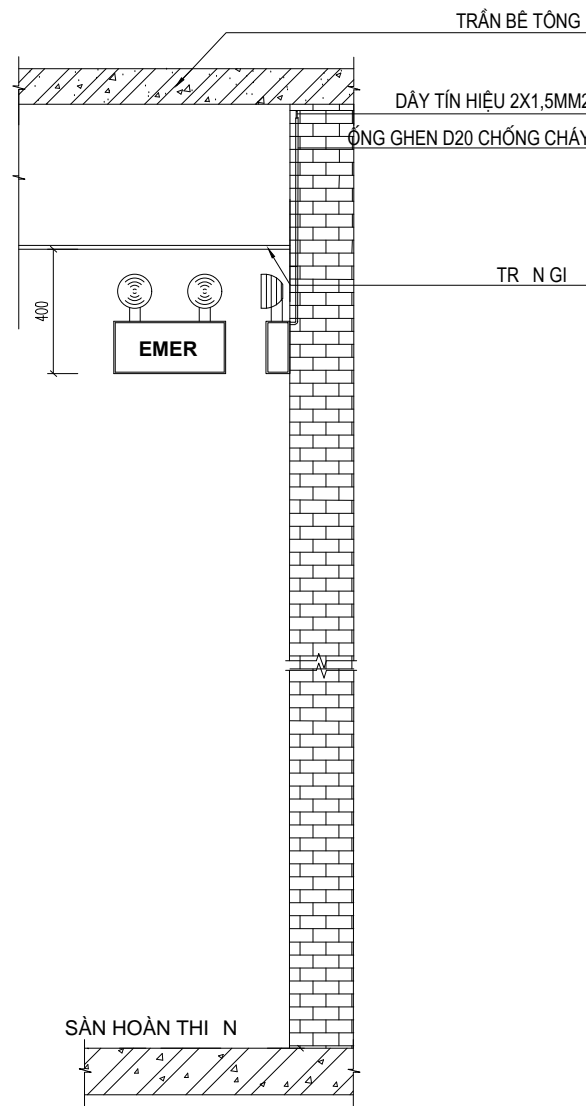
CHI TIẾT LẮP ĐẶT ĐÈN CHIẾU SÁNG SỰ CỐ KHU VỰC CÓ TRẦN GIẢ
