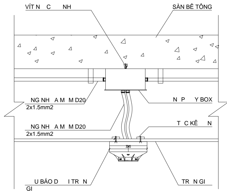
CHI TI T L P T U BẢO D I TR N BÊ TÔNG
