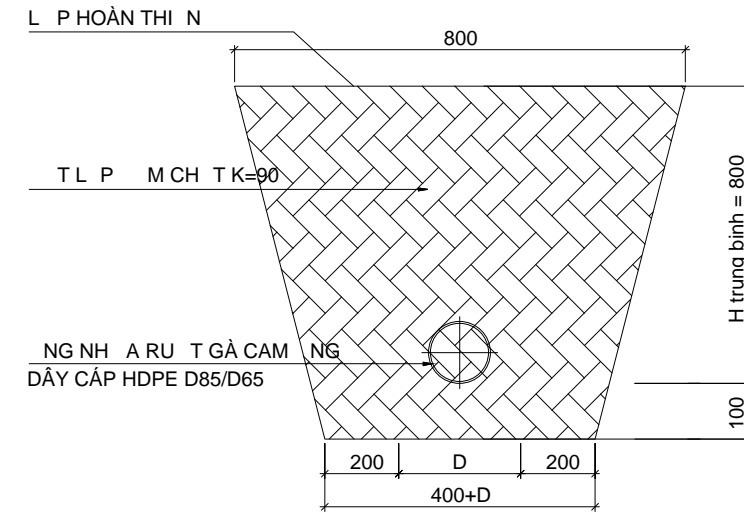
M T C T I N HÌNH M NG T NG NH A
