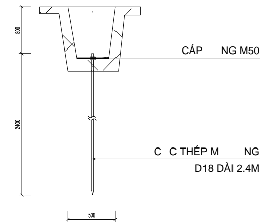
M T C T NGANG CHÔN C C TI P A
