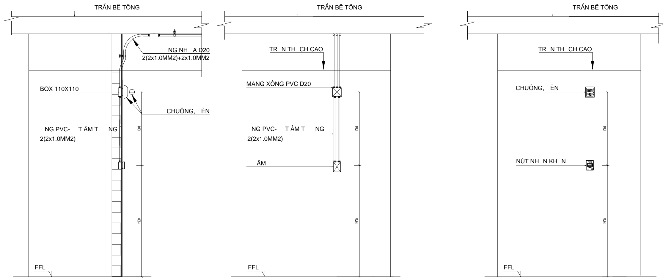
CHI TIẾT LẮP ĐẶT CHUÔNG ĐÈN NÚT ẮN
