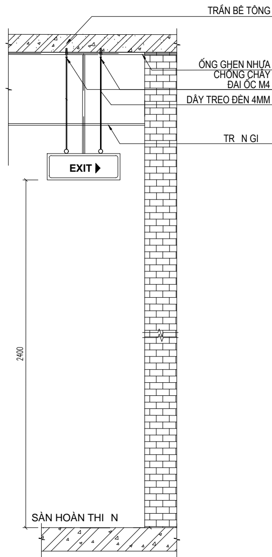
CHI TIẾT LẮP ĐẶT ĐÈN CHỈ LỐI THOÁT NẠN EXIT KHU VỰC CÓ TRẦN GIẢ
