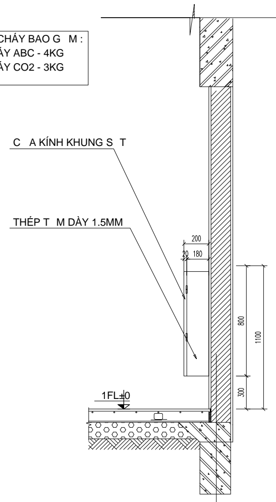
CHI TI T L P I N HÌNH T T NG BÌNH CH A CHÁY
