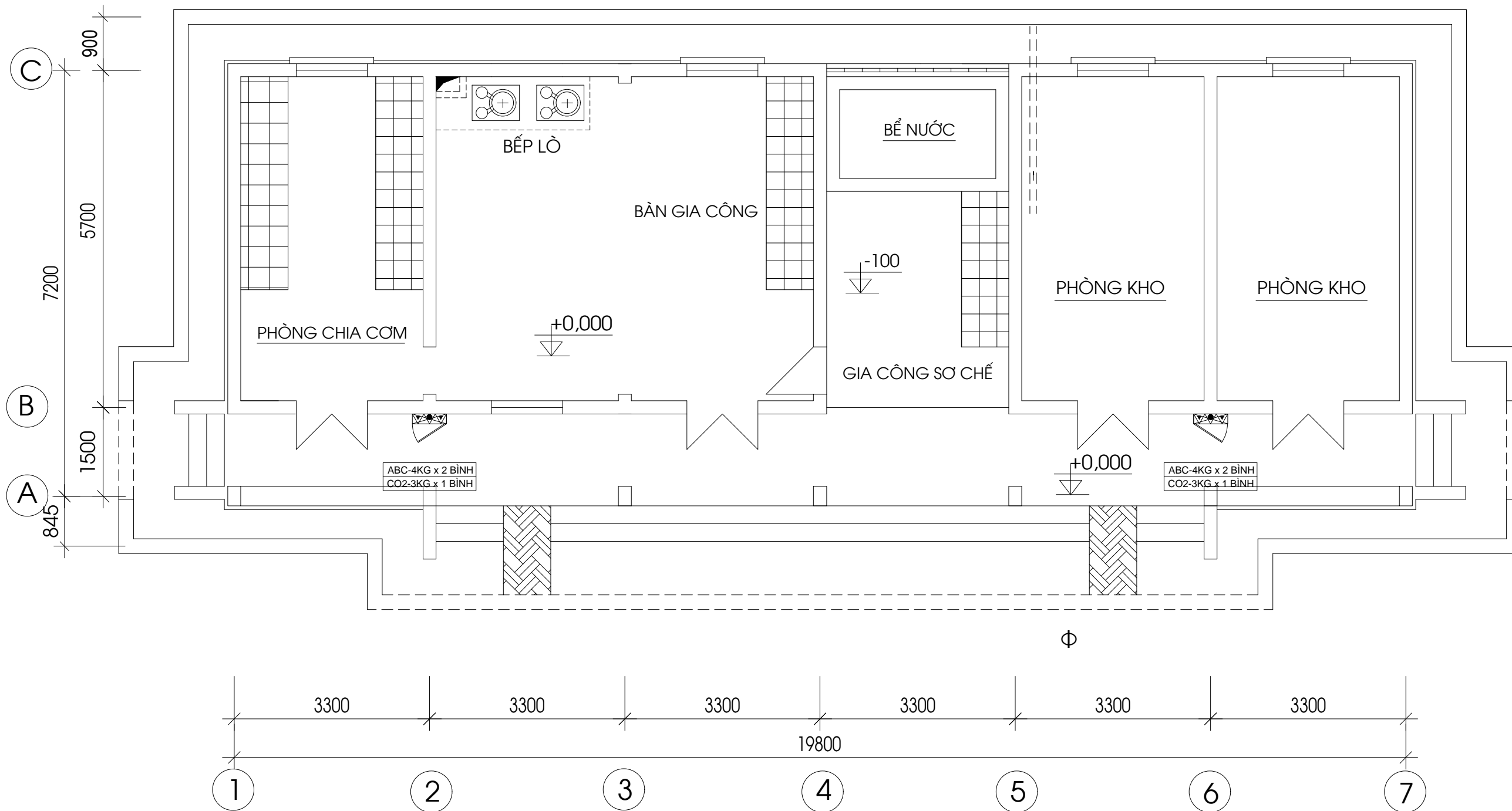
M T B NG CH A CHÁY T NG 1
