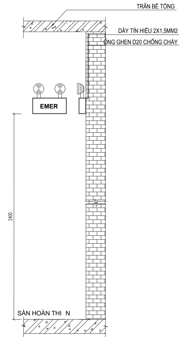
CHI TIẾT LẮP ĐẶT ĐÈN CHIẾU SÁNG SỰ CỐ KHU VỰC KHÔNG CÓ TRẦN GIẢ
