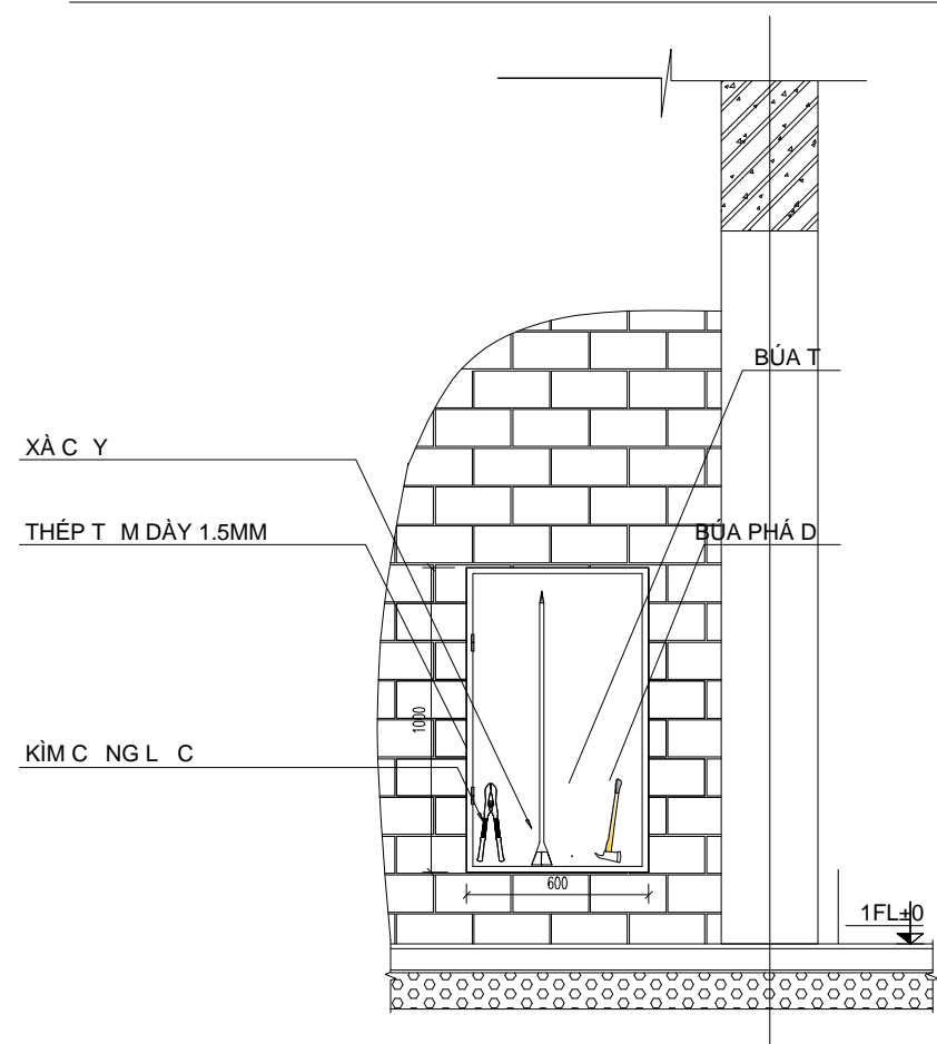
CHI TI TL P I N HÌNH TT CH A CHÁY VÁCH T NG
