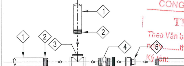
CHI TIẾT LẮP TÊ, KÉP, CÔN THU
