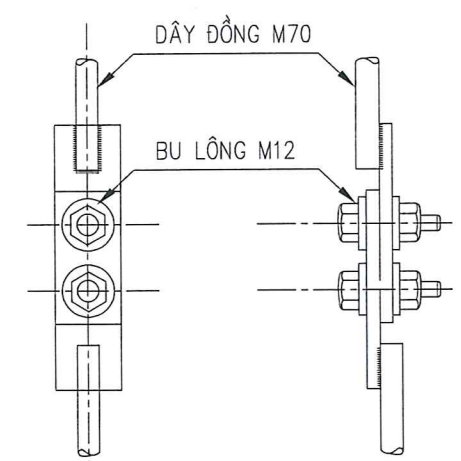
MỐI NỐI KIỂM TRA
