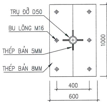
CHÂN ĐỂ TRỤ THU SÉT
