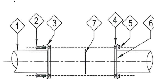
CHI TIẾT NỐI ỐNG BẰNG MẶT BÍCH
