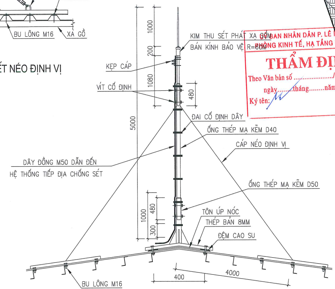
CHI TIẾT KIM THU SÉT
