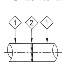
CHI TIẾT HÀN NỐI ỐNG VỚI ỐNG
