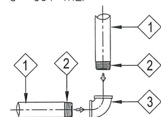
CHI TIẾT LẮP CÚT
