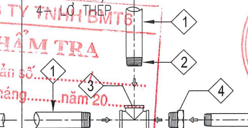
CHI TIẾT LẮP LỖ THÉP GIẬT CẤP
