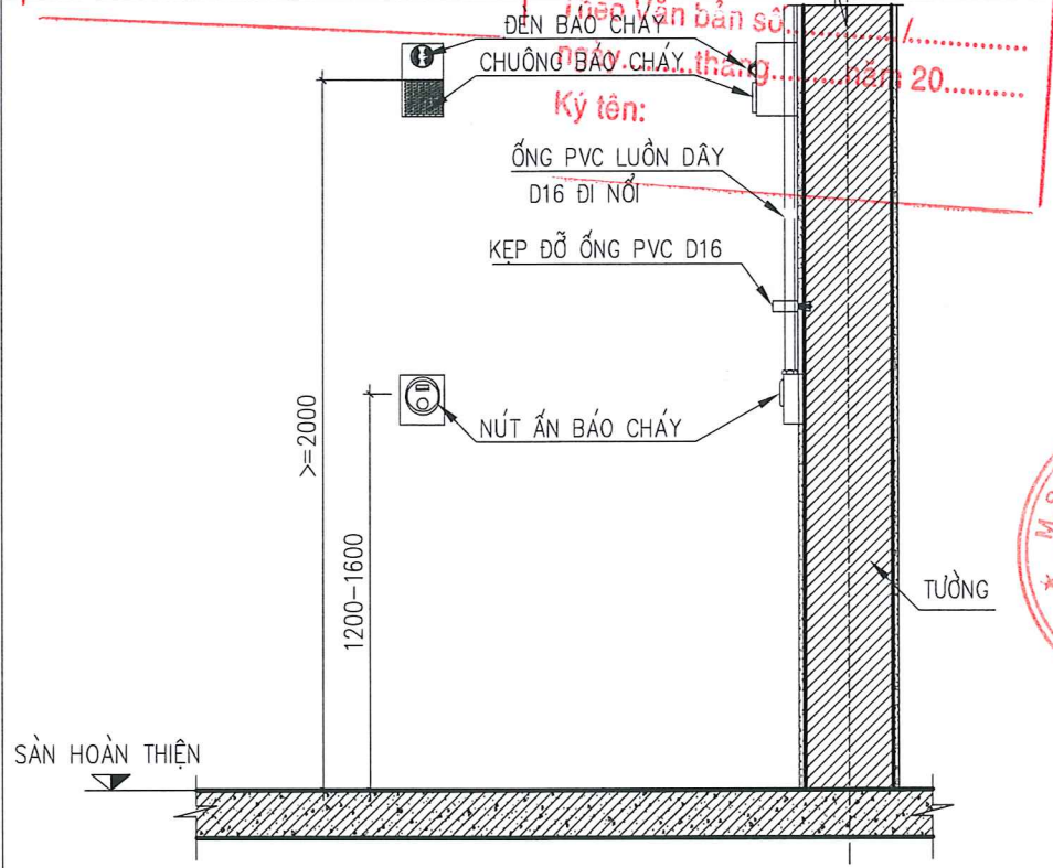
CHI TIẾT LẮP ĐẶT TỔ HỢP CHUÔNG ĐÈN, NÚT ẤN BÁO CHÁY
