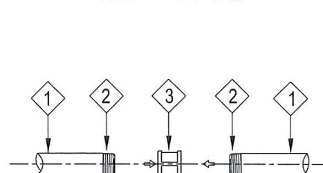
CHI TIẾT LẮP MĂNG XÔNG NỐI ỐNG
