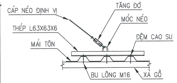
CHI TIẾT NÉO ĐINH VỊ
