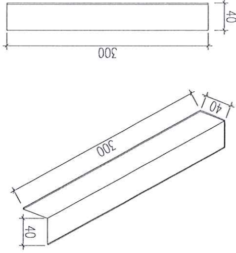
CẦU TẠO 02 THANH SỐ 03
