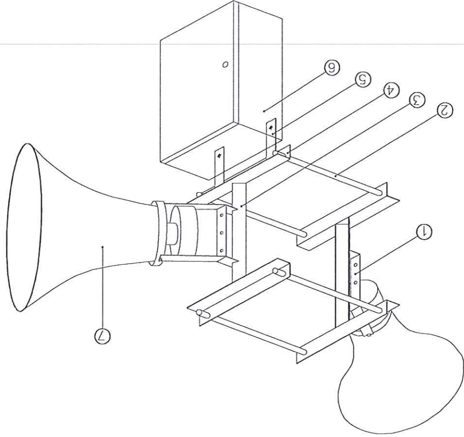
BỘ KHUNG TREO LOA VÀ THIẾT BỊ THU PHÁT KỸ THUẬT SỐ
