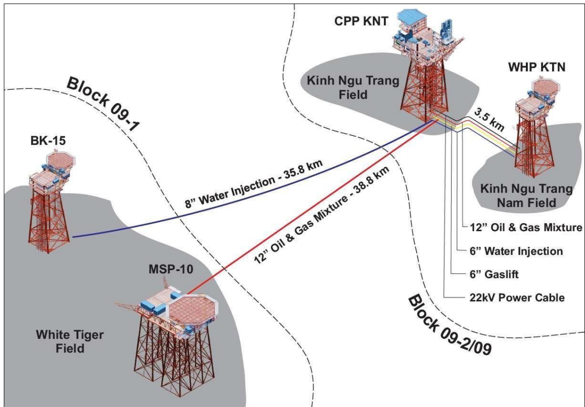
Hình 1: Vị trí giàn CPP KNT và WHP KTN thuộc mỏ Kinh Ngư Trắng – Kinh Ngư Trắng Nam, Lô 09-2/09
