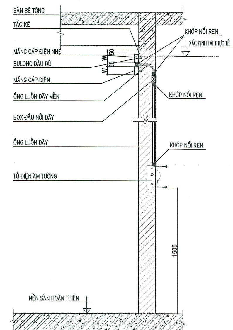
CHI TIẾT ĐẦU NỐI TỪ MĂNG CÁP VỀ TỦ PHÒNG (ĐIỂN HÌNH)
