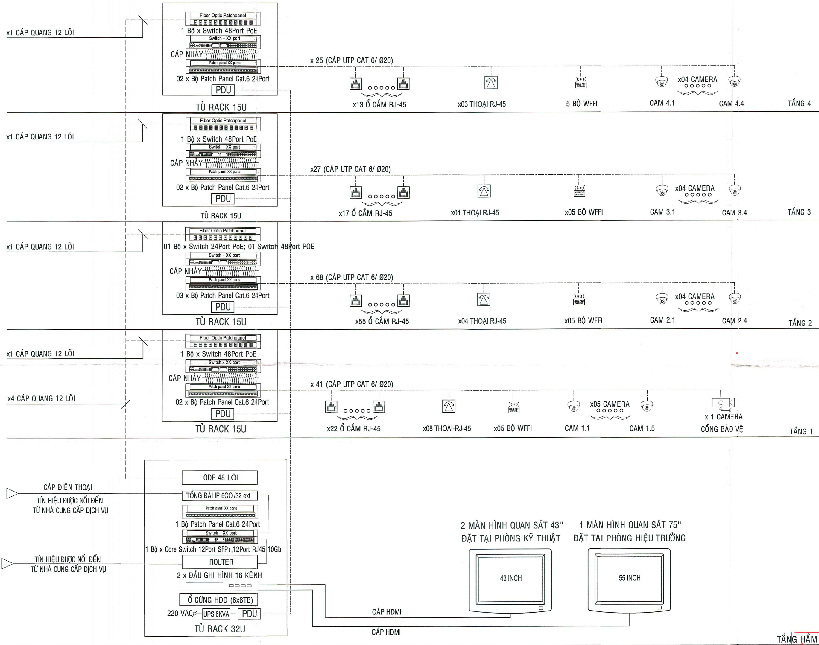
SƠ ĐỒ NGUYÊN LÝ HỆ THỐNG ĐIỆN THOẠI, MẠNG INTERNET, CAMERA, WIFI
