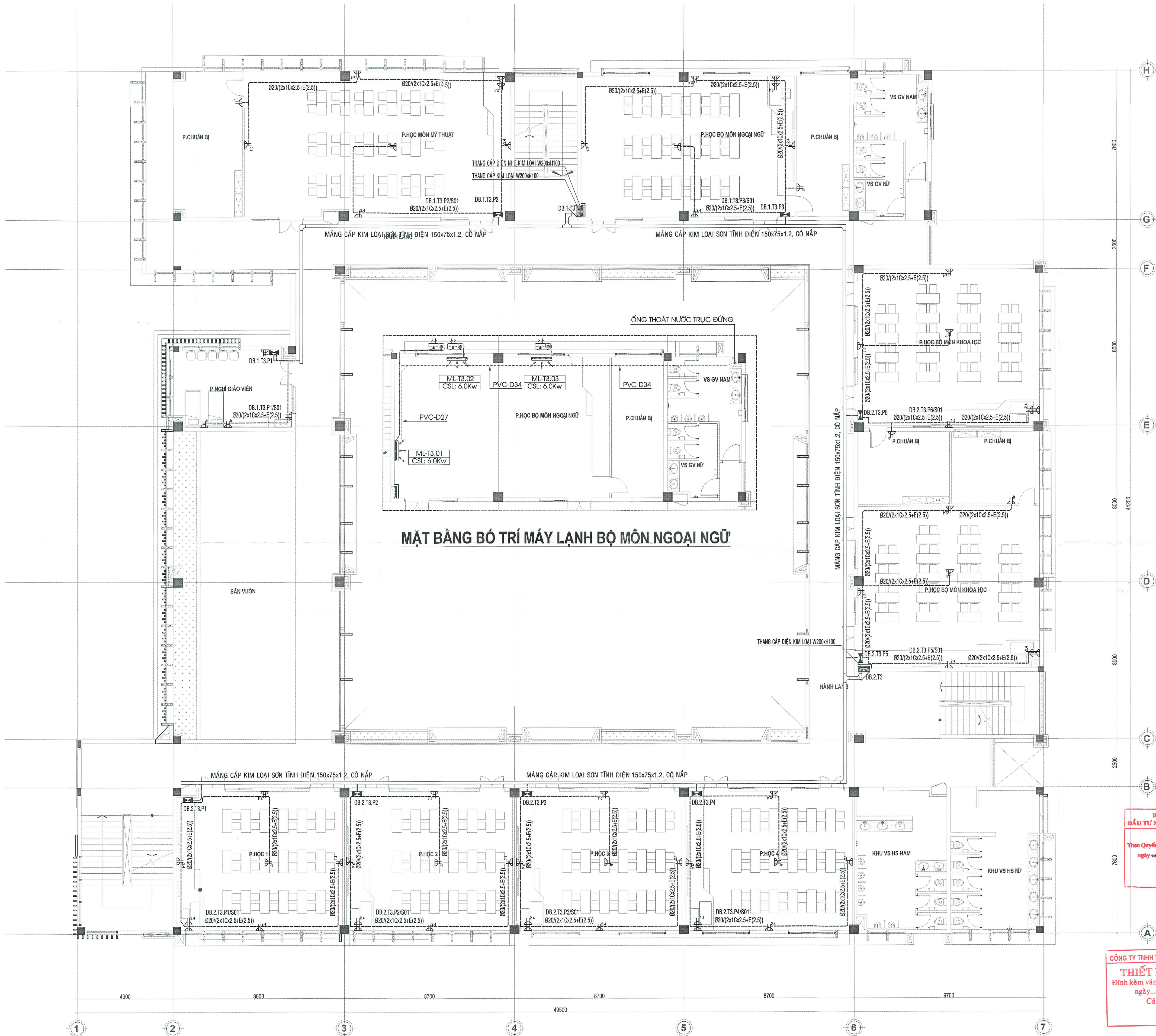
MẶT BẰNG ĐIỆN ĐỘNG LỰC TẦNG 3
