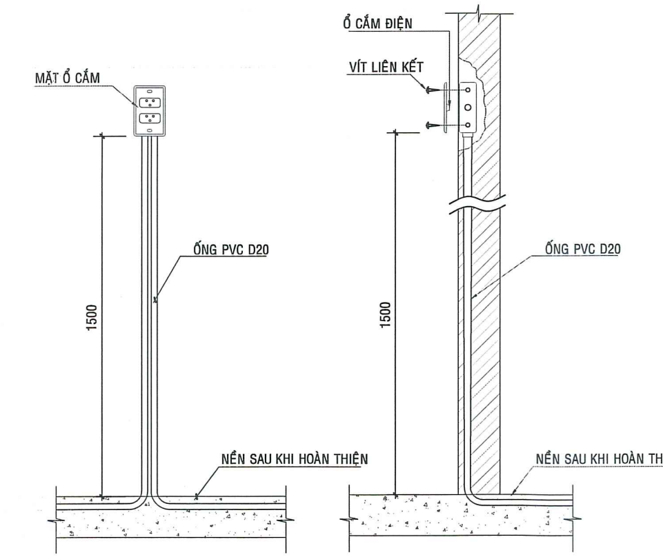
CHI TIẾT LẮP ĐẶT Ố CẮM ĐIỆN
