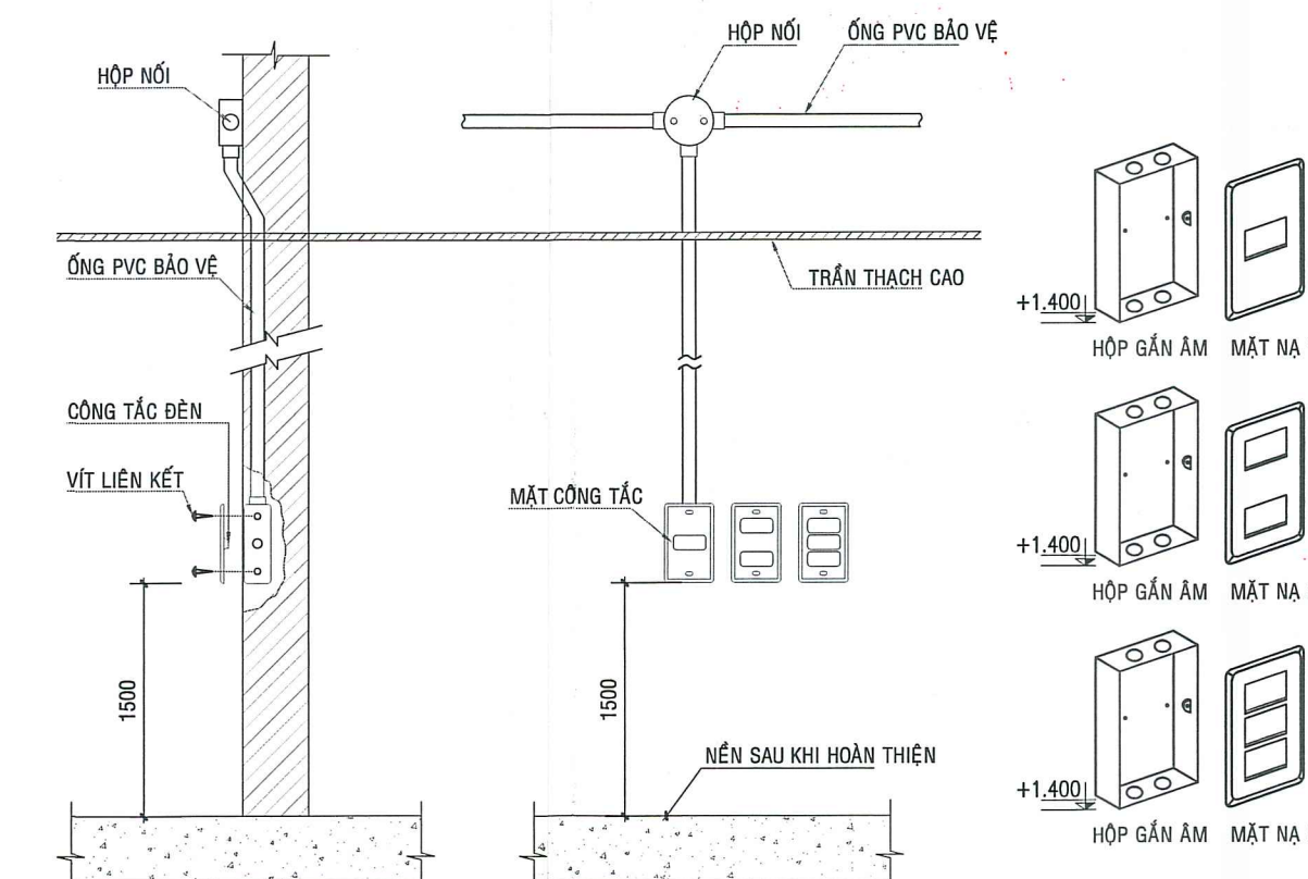
CHI TIẾT LẮP ĐẶT CÔNG TẮC
