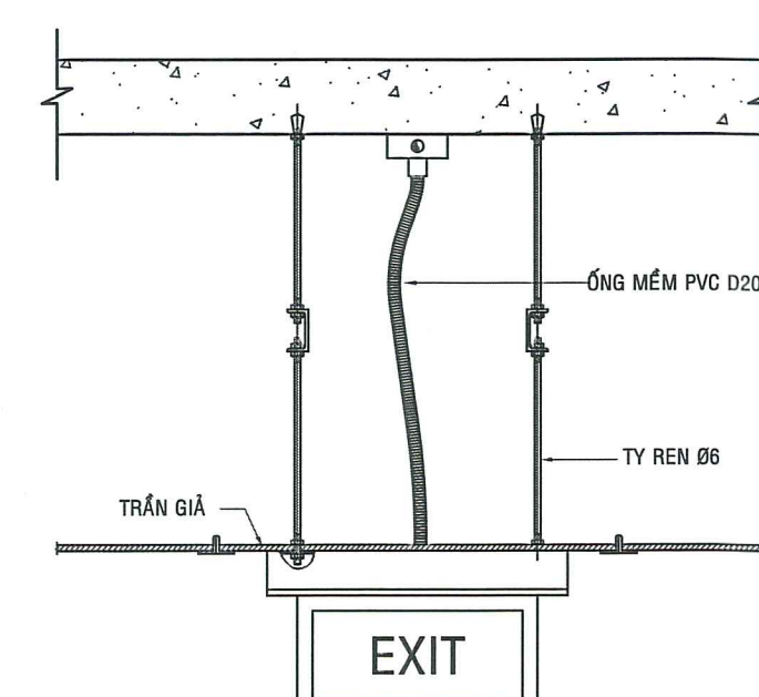
CT LẮP ĐÉN EXIT - ĐÉN CHIẾU SÁNG KHẨN
