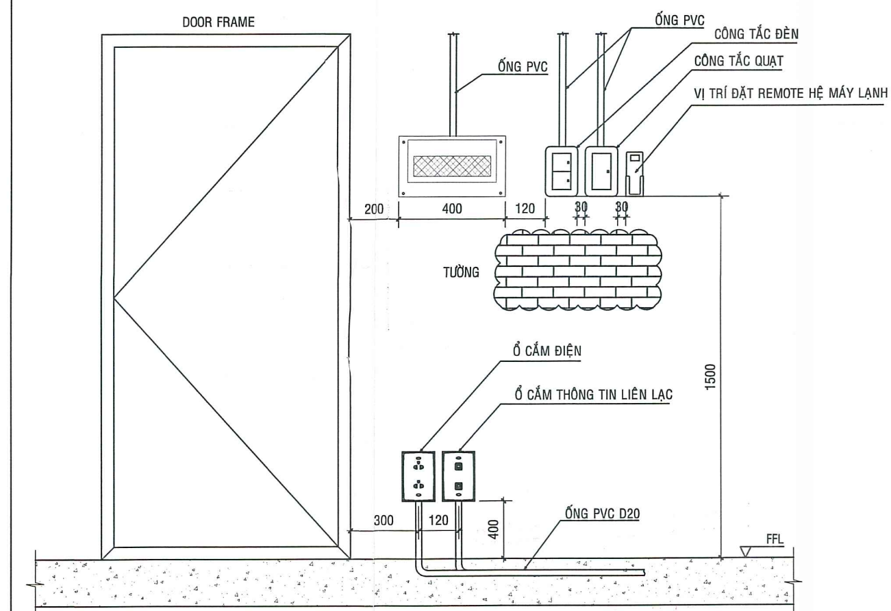
CHI TIẾT LẮP ĐẶT TỦ ĐIỆN, CÔNG TẮC, Ố CẮM TRONG PHÒNG ĐIỆN HÌNH
