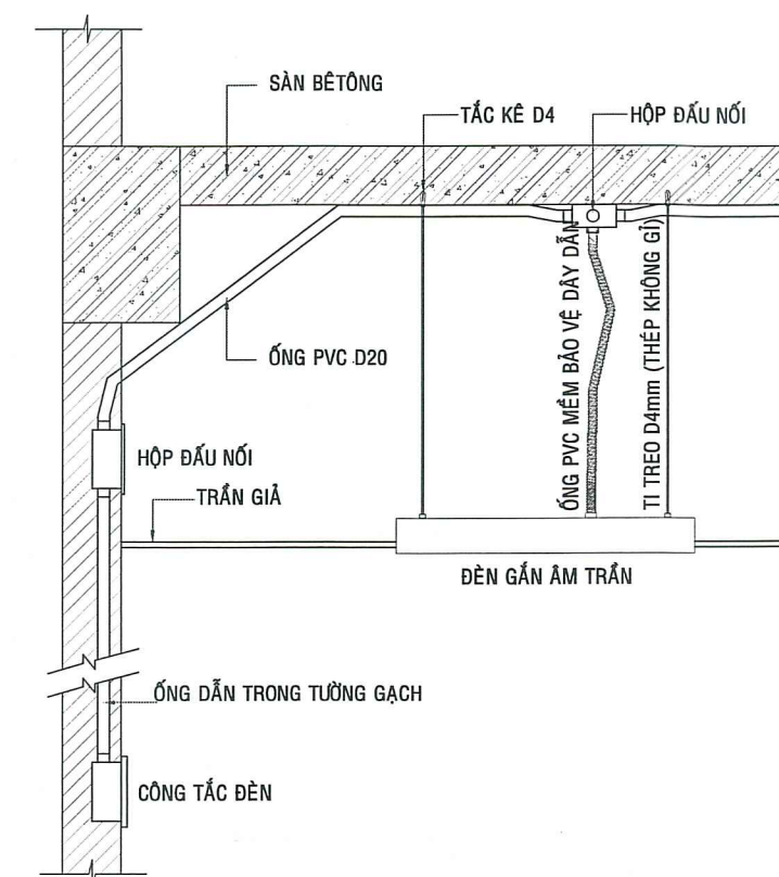
CHI TIẾT LẮP ĐÉN 2x18W ẨM TRẦN
