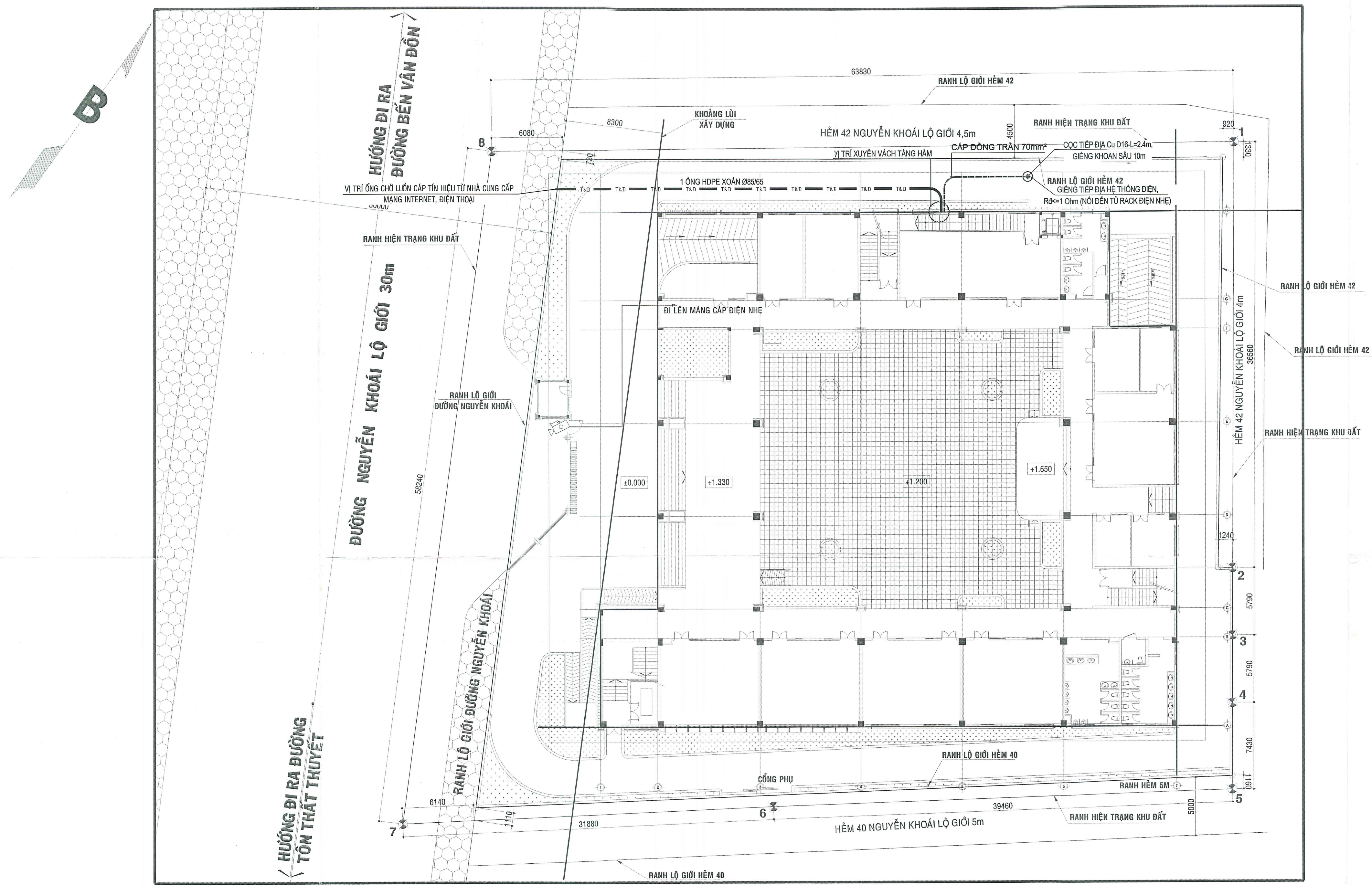
MẶT BẰNG ĐIỆN NHỆ TỔNG THỂ
