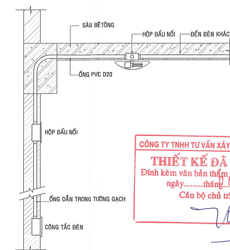
CHI TIẾT LẮP ĐÉN ỐP TRẦN
