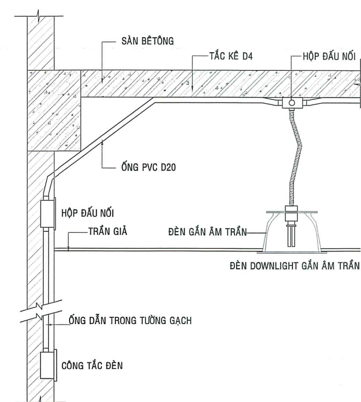
CHI TIẾT ĐÉN DOWLIGHT ẨM TRẦN
