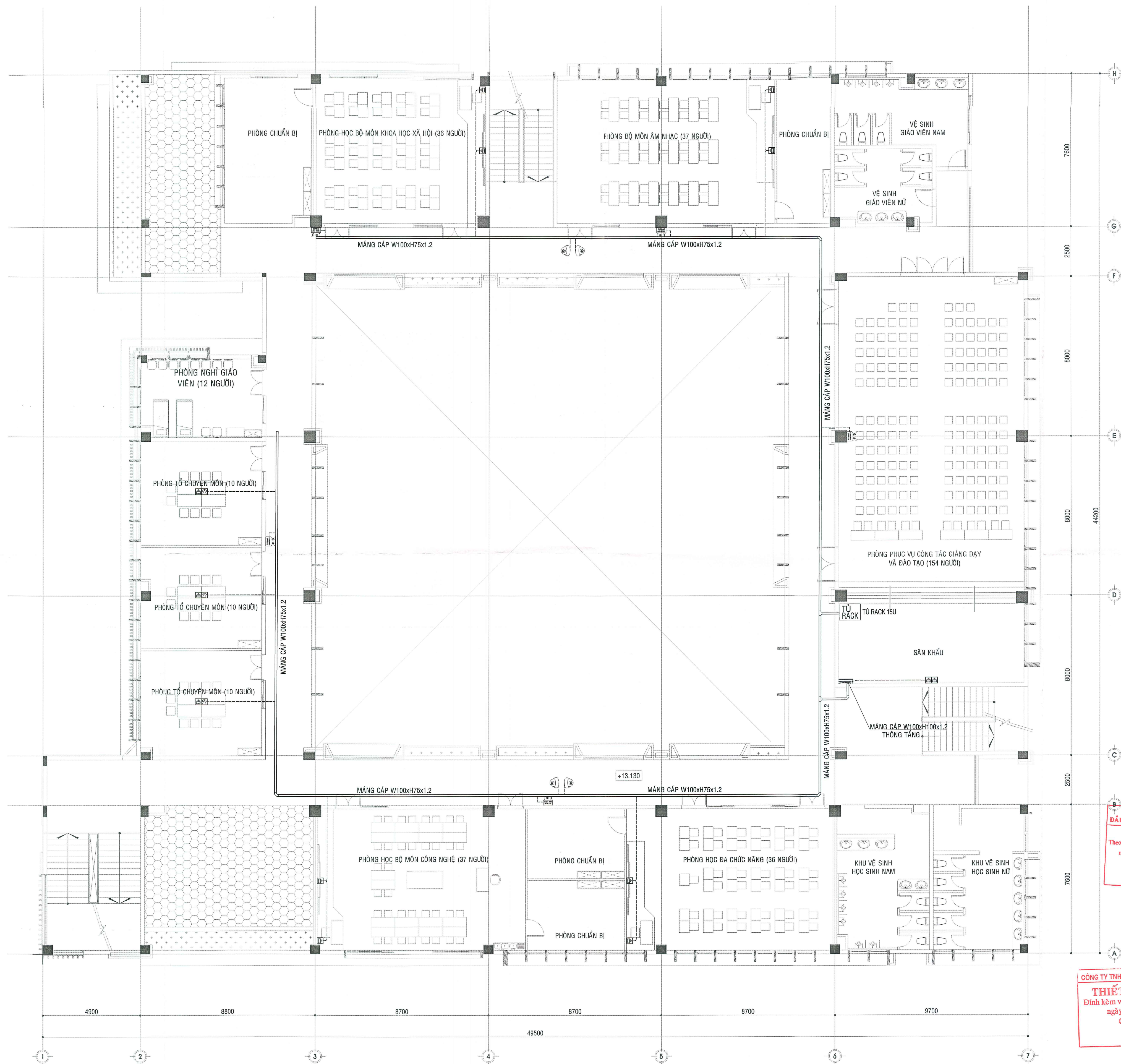
MẶT BẰNG ĐIỆN NHỆ TẦNG 4
