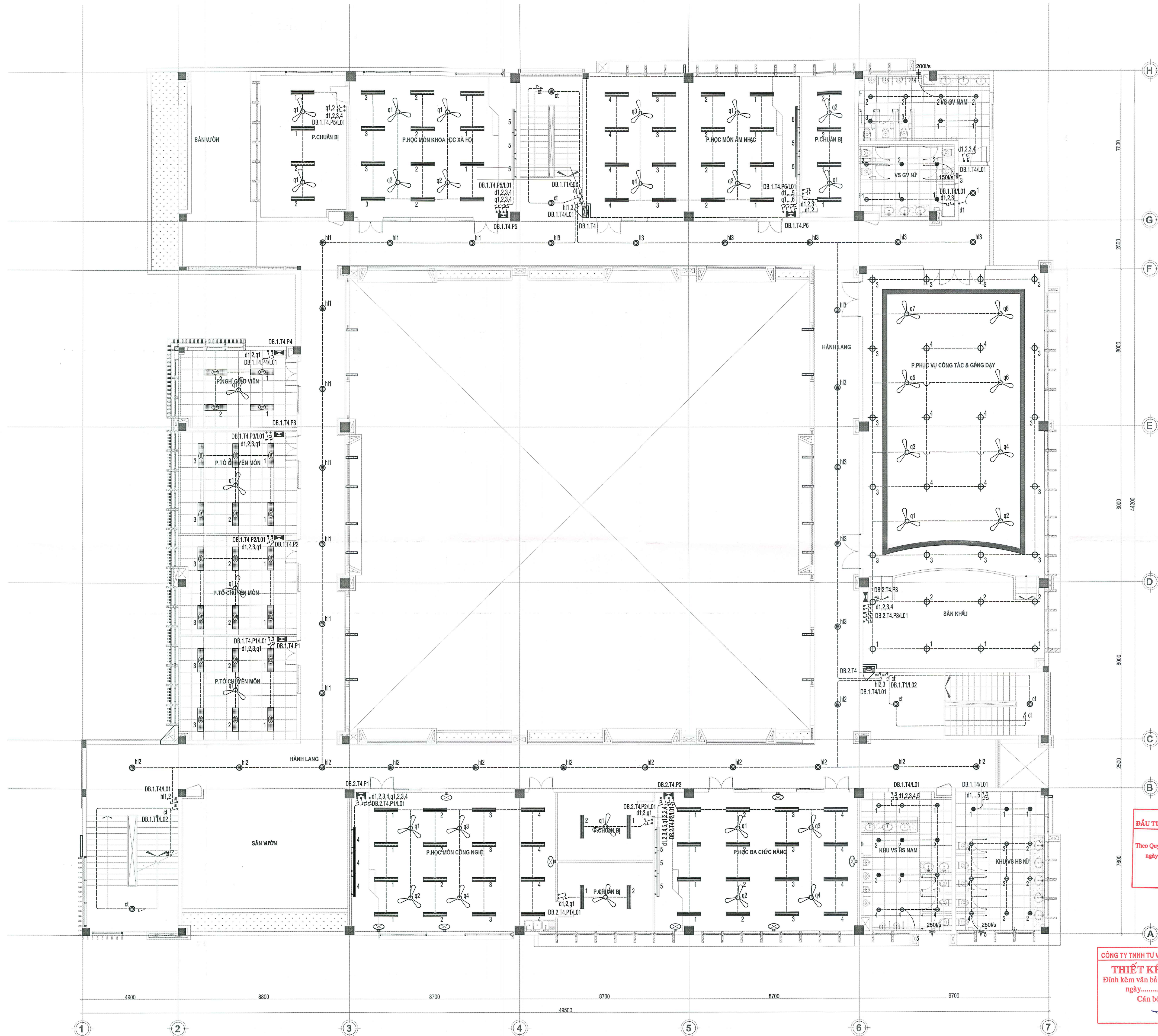
MẶT BẰNG ĐIỆN CHIẾU SÁNG TẦNG 4
