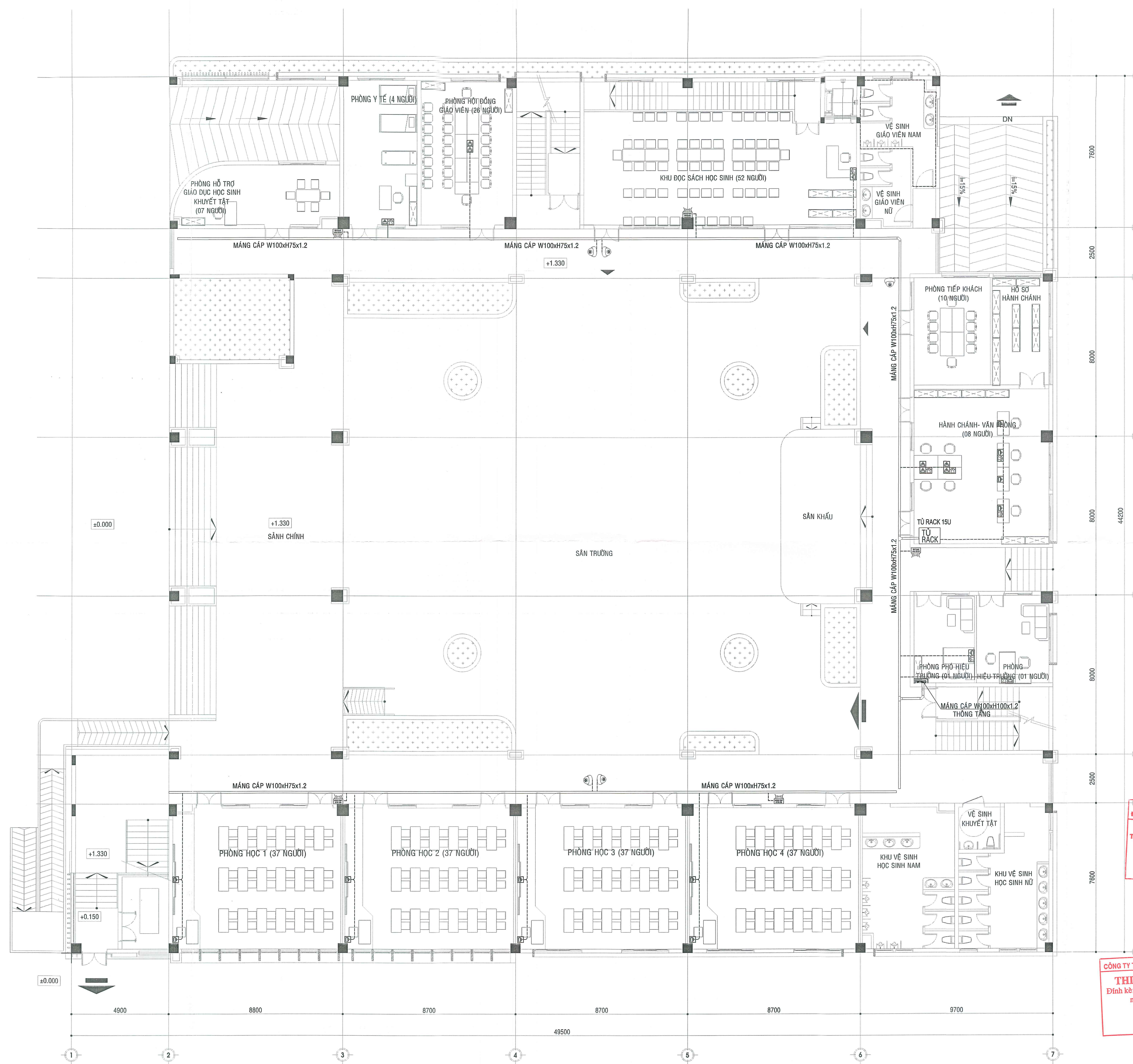
MẶT BẰNG ĐIỆN NHỆ TẦNG 1
