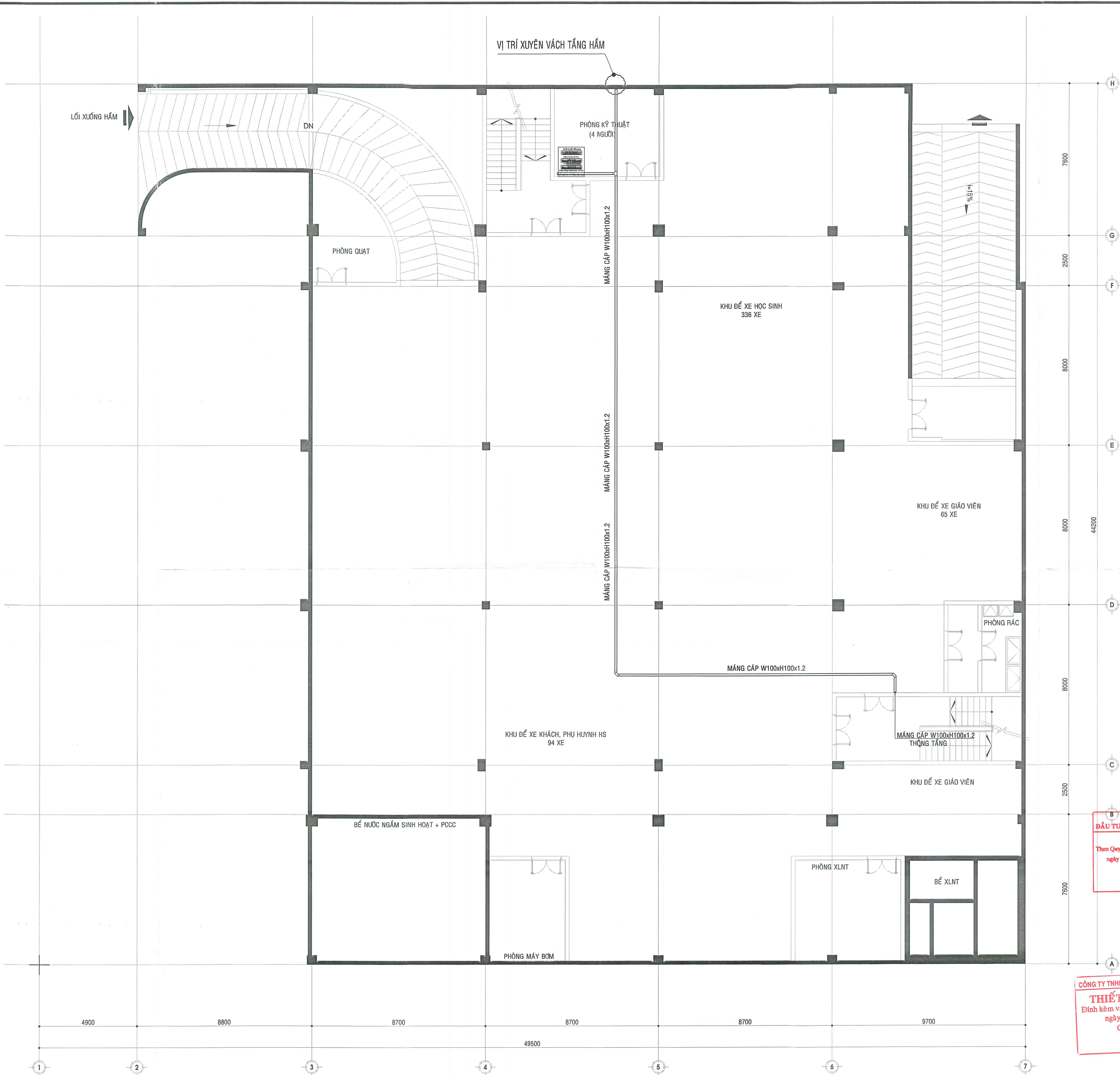
MẶT BẰNG ĐIỆN NHỆ TẦNG HẦM
