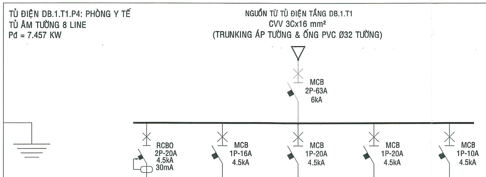
SƠ ĐỒ NGUYÊN LÝ TỦ ĐIỆN DB.1.T1.P1
