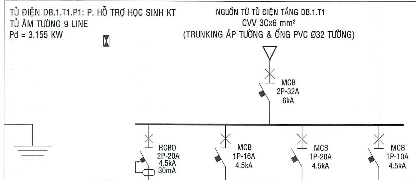
SƠ ĐỒ NGUYÊN LÝ TỦ ĐIỆN DB.H
