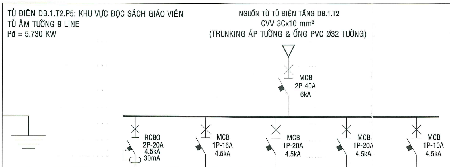
SƠ ĐỒ NGUYÊN LÝ TỦ ĐIỆN DB.1.T2.P2
