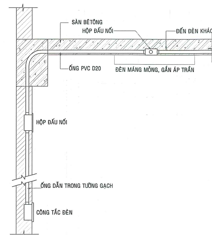
CHI TIẾT ĐÉN 1x36W, 2x36W LẮP NỐI
