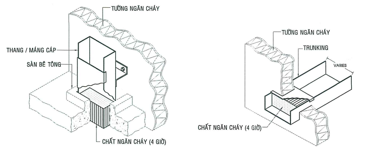
CT. LẮP ĐẶT THANG / MĂNG CÁP THÔNG SÀN
