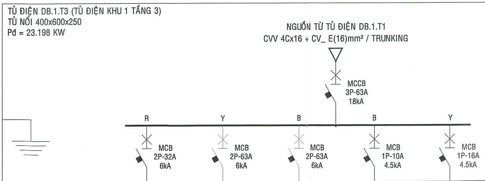
SƠ ĐỒ NGUYÊN LÝ TỦ ĐIỆN DB.1.T2.P4
