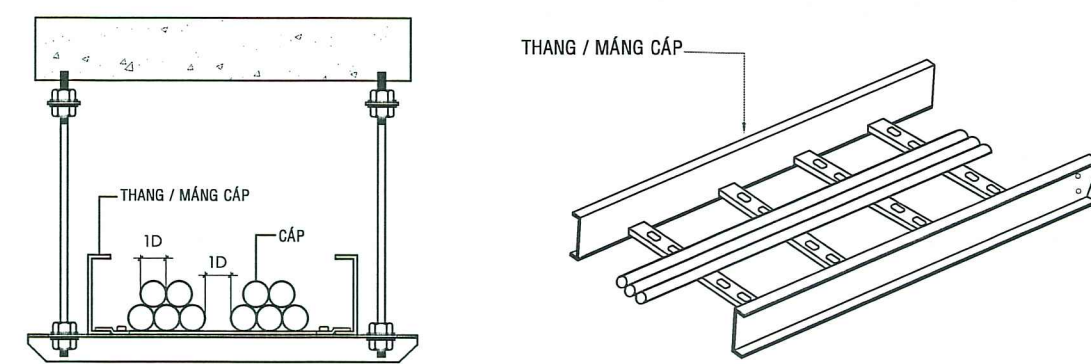
CHI TIẾT ĐẶT CÁP TRONG THANG / MĂNG CÁP (ĐIỂN HÌNH)
