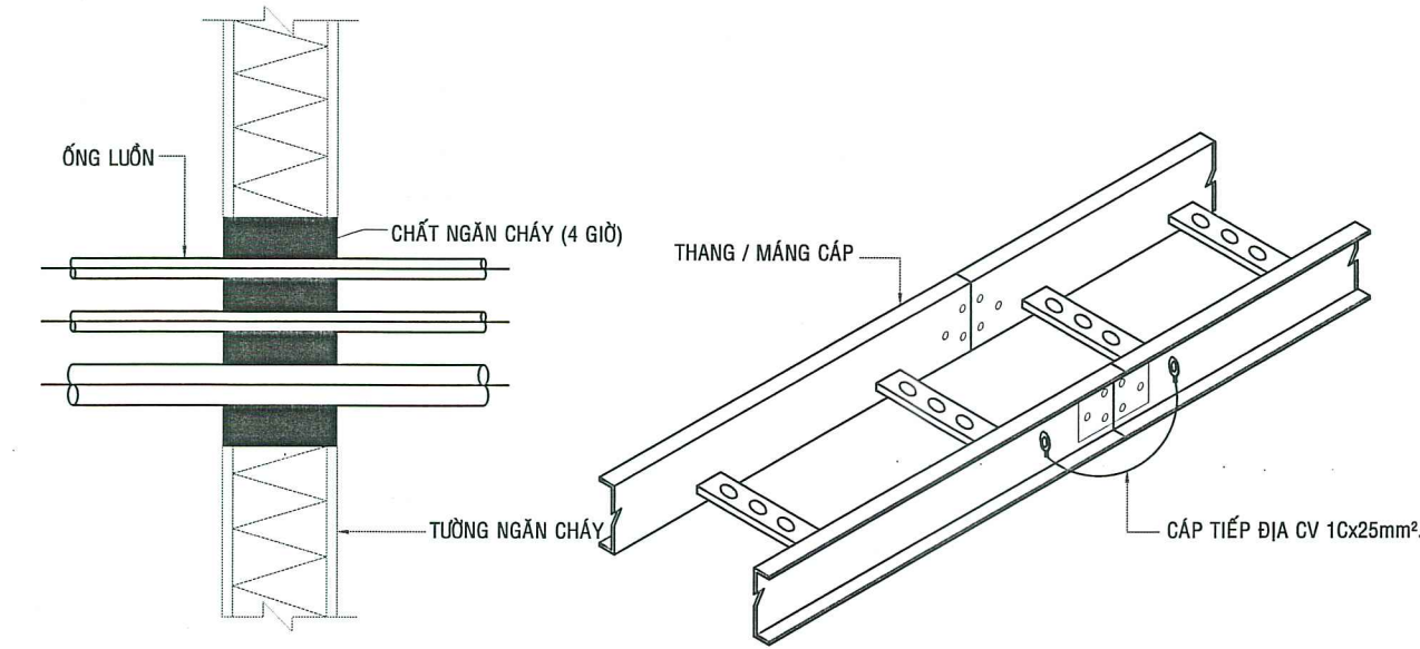
CT. LẮP ĐẶT CHỐNG CHÁY LAN ỐNG XUYÊN TƯỜNG
