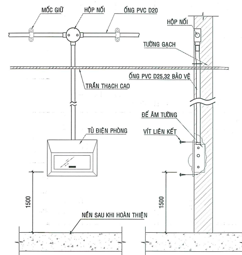
CHI TIẾT LẮP TỦ ĐIỆN PHÒNG ẨM TƯỜNG
