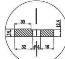
CHI TIẾT E
