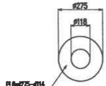
CHI TIẾT VÀNH TĂNG CƯỜNG SỐ LƯỢNG : 01
