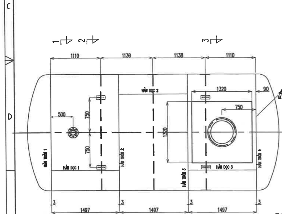
BỒN CHỨA 24,5M3 (O.D2500)
