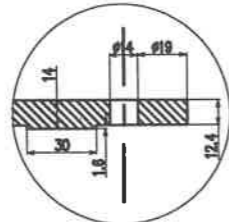
CHI TIẾT D
