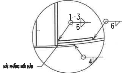
CHI TIẾT C
