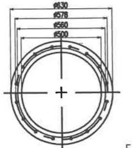
MẶT BÍCH TRÊN SỐ LƯỢNG : 01
