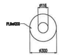
VÒNG TĂNG CỨNG SỐ LƯỢNG : 01
