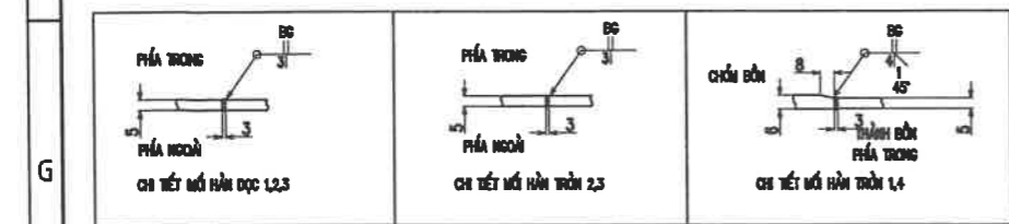
BỒN CHỨA 24,5M3 (O.D2500)
