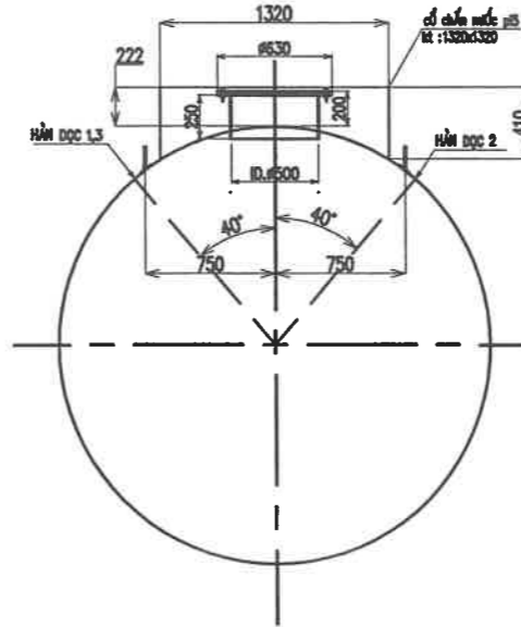
MẶT CẮT 3-3
