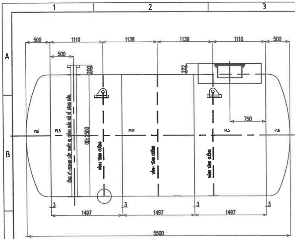
BỒN CHỨA 24,5M3 (O.D2500)
