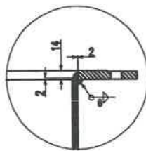
CHI TIẾT A
