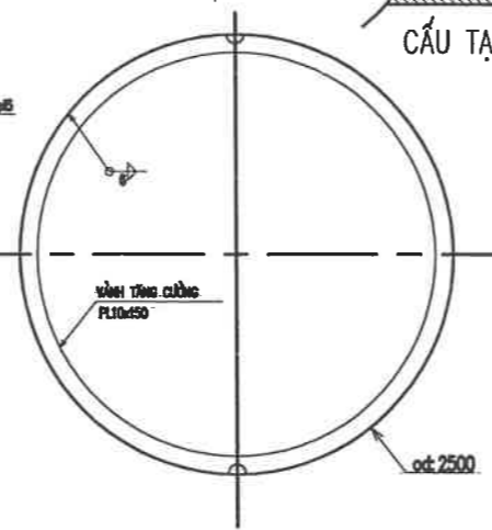
MẶT CẮT 2-2
