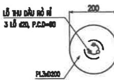
CHI TIẾT NẮP LỖ THU DẦU SỐ LƯỢNG : 01
