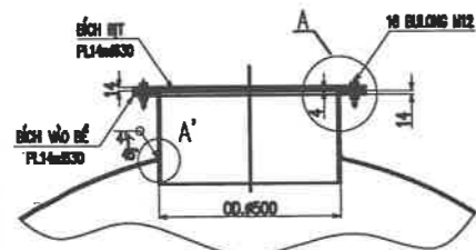
CHI TIẾT CỬA BỂ
