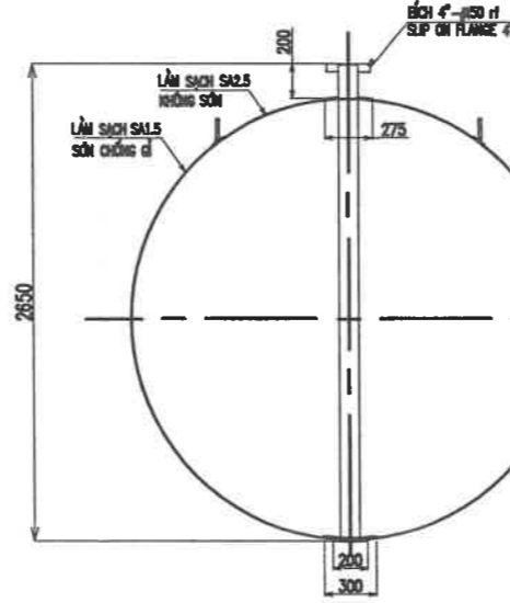
MẶT CẮT 1-1
