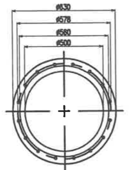
MẶT BÍCH TRÊN SỐ LƯỢNG : 01
