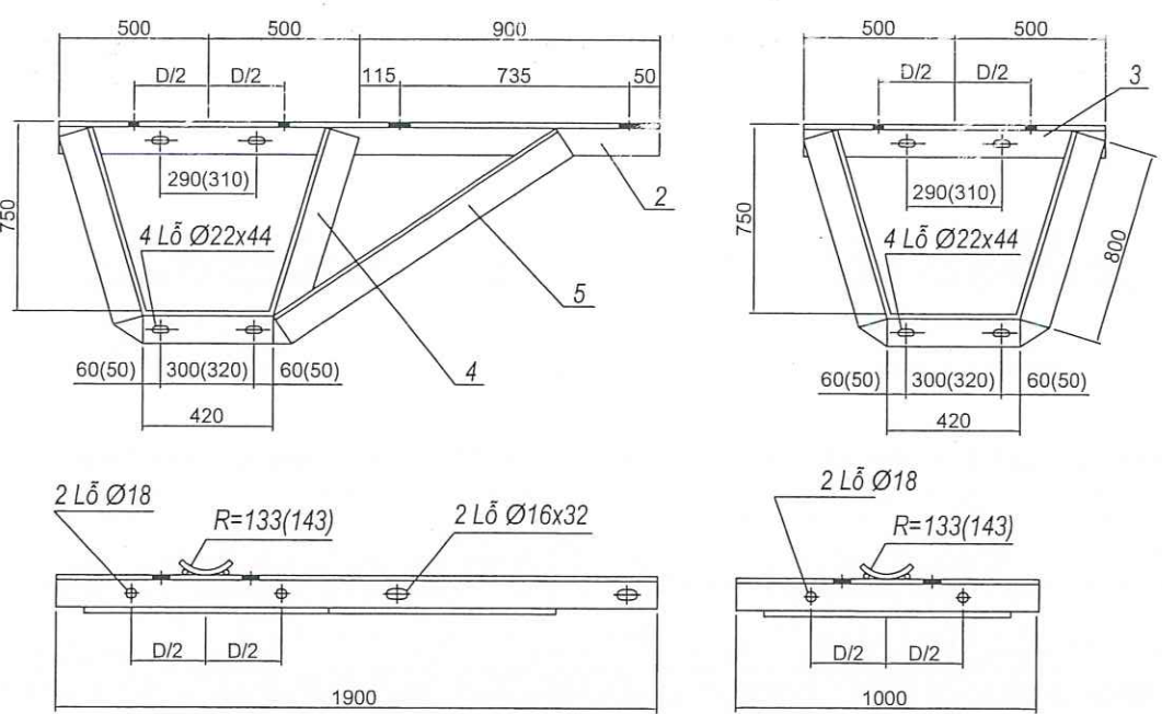
CÔNG SON ĐỖ MBA
