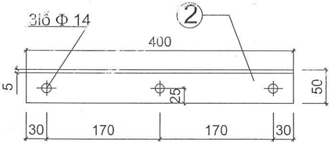
Thanh bắt cáp
