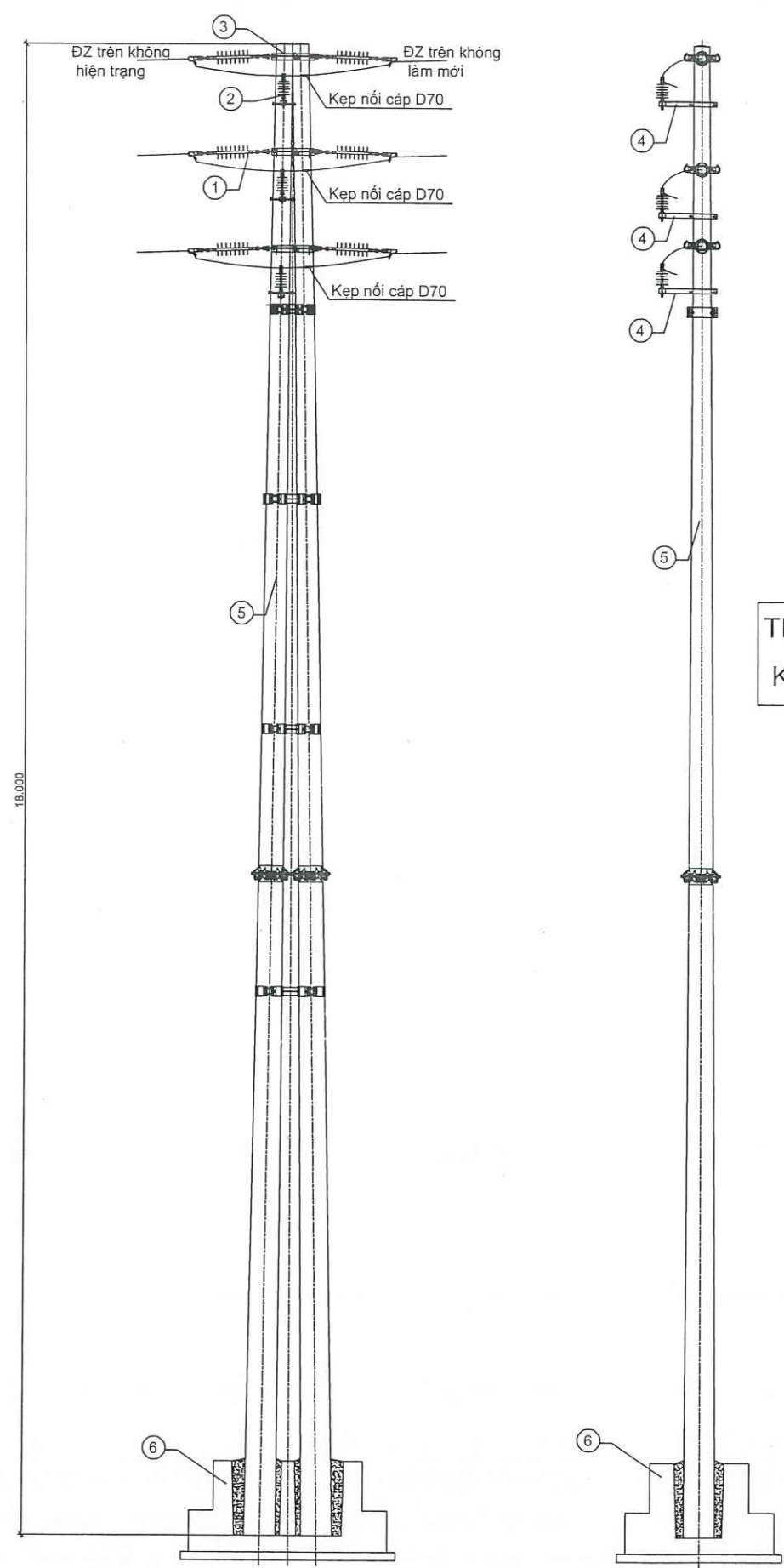
CỘT ĐẦU NỐI HIỆN TRẠNG DZ373E18.2
