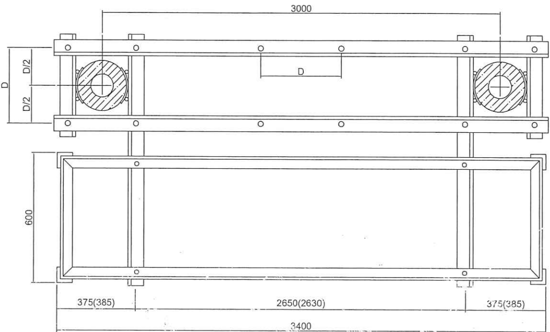
MẶT BẰNG CÔNG SON VÀ GHẾ THAO TÁC
