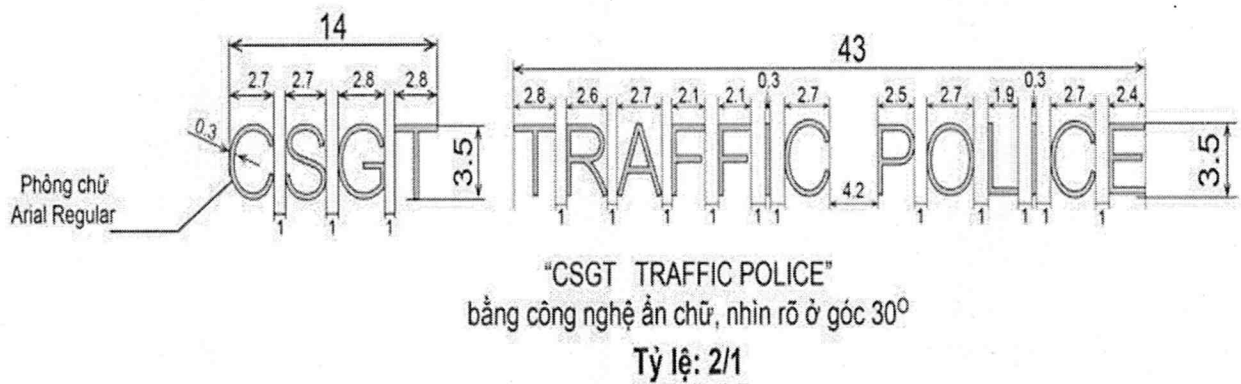
Hình 2: Quy cách cụm ký tự "CSGT" và "TRAFFIC POLICE"
