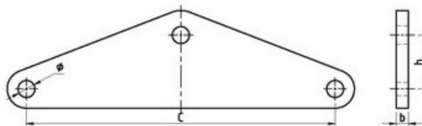
d) Vòng treo đầu tròn – YokE platE
