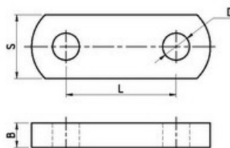
c) Khánh mắc chuỗi cách điện kép – YokE platE
