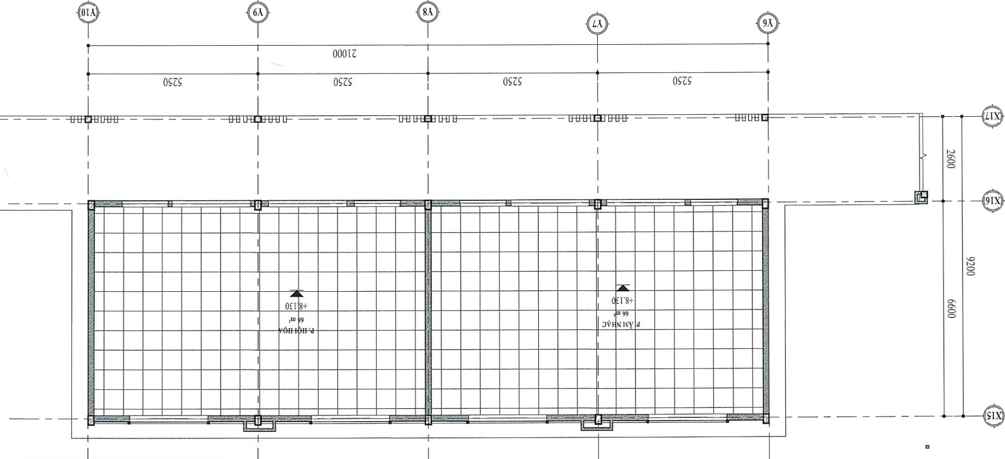
MẶT BẰNG TRẦN TẦNG 2 - KHỐI B 1 : 100
