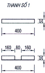
CHI TIẾT THÉP GÓC TL:1/10
