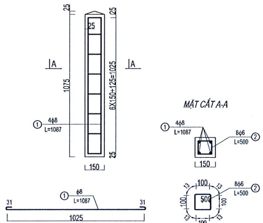
CHI TIẾT CỐT THÉP CỌC TIÊU _ TL:1/20
