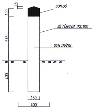
CHI TIẾT CỌC TIÊU _ TL:1/20
