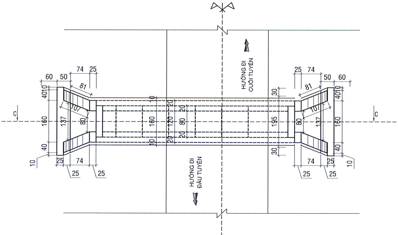
MẶT BẰNG CỐNG, TL 1/100
