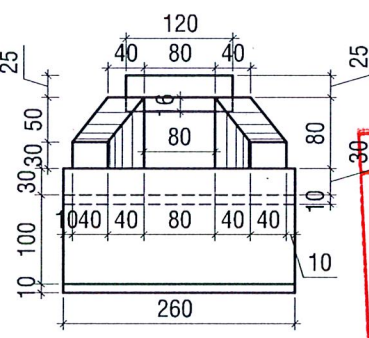
CHÍNH DIỆN THƯỢNG HẠ LƯU CỐNG TỶ LỆ: 1/100
