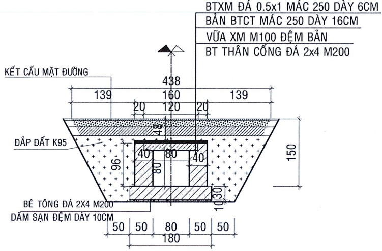
MẶT CẮT NGANG TIM CỐNG TỶ LỆ: 1/100
