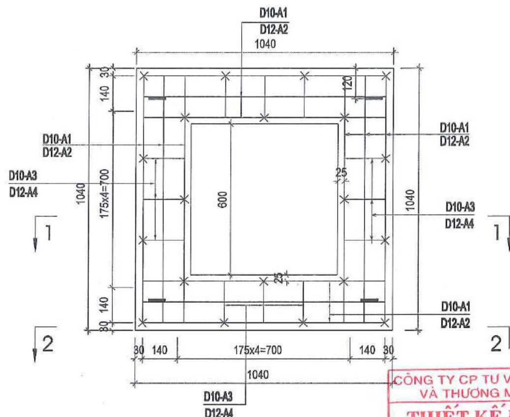
MẶT CẮT 1 - 1
