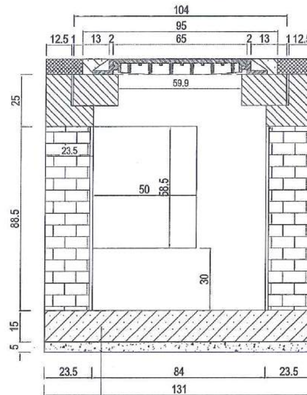
MẶT CẮT II - II
