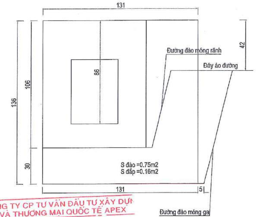
MẶT CẮT ĐÀO ĐẮP GA
