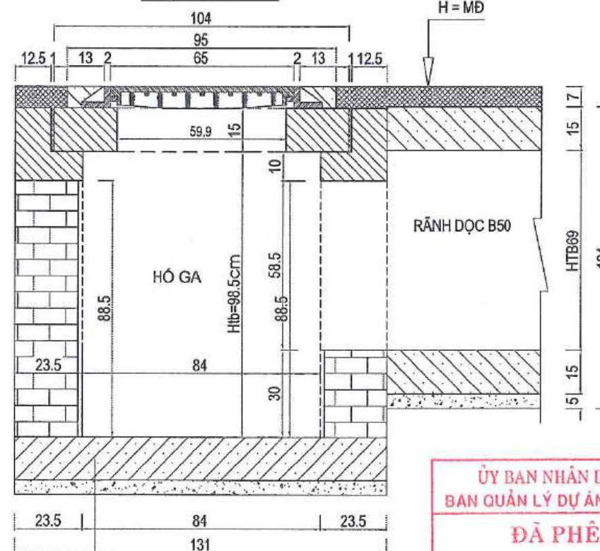
MẶT CẮT I - I
