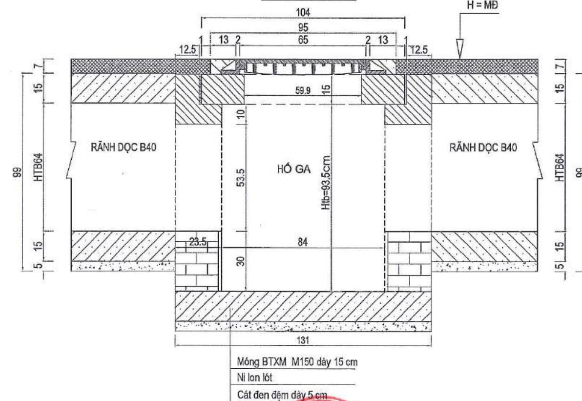
MẶT CẮT I - I
