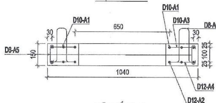
MẶT CẮT 2-2
