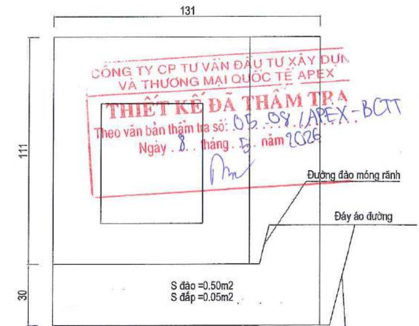
MẶT CẮT ĐÀO ĐẮP GA
