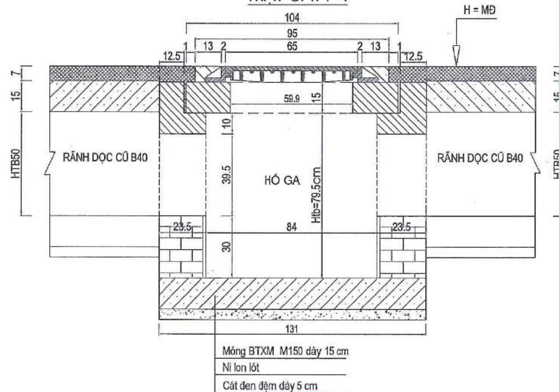
MẶT CẮT I - I
