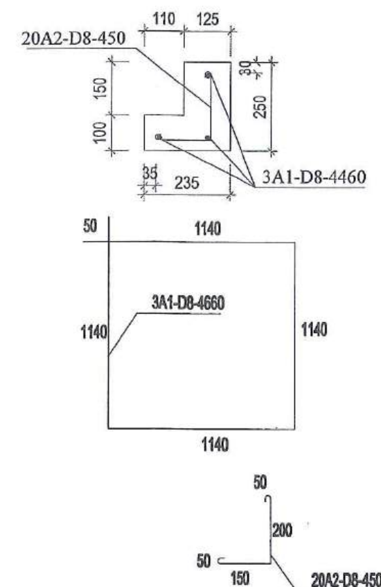
BẢNG KHỐI LƯỢNG CHO 1 TẤM NẮP HỐ GA (MÉP ĐƯỜNG) BÊ TÔNG CHỊU LỰC KT (1.04X1.04X0.15)M, TƯỜNG MŨ BTCT 01 HỐ GA
