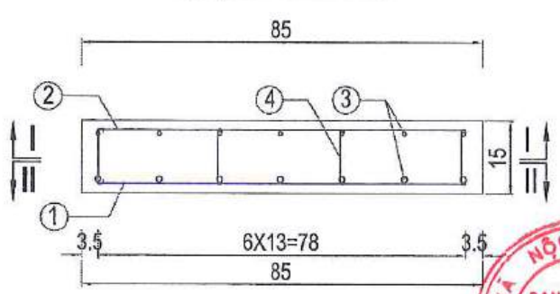
MẶT CẮT III - III
