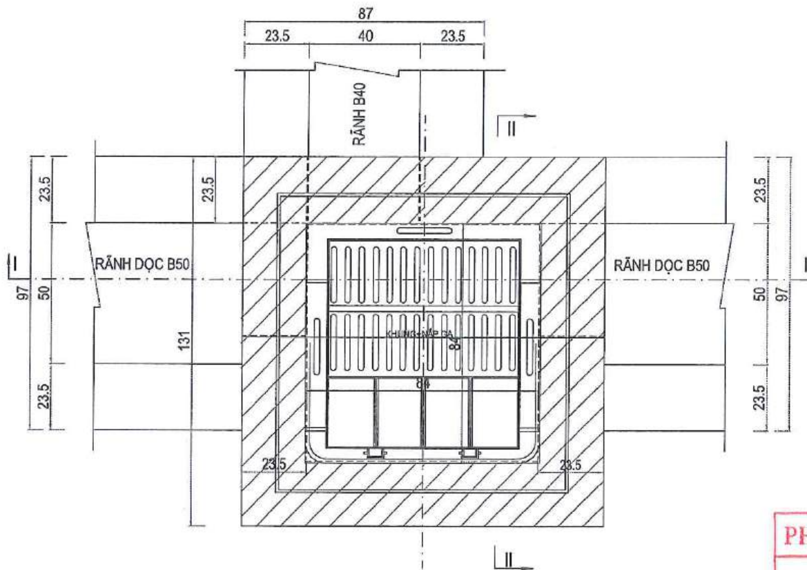
MẶT BẰNG HỐ GA
