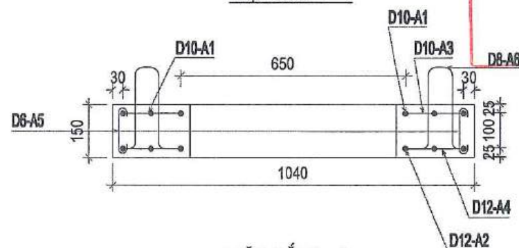
MẶT CẮT 2 - 2
