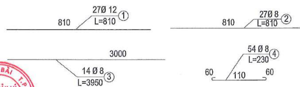
CHI TIẾT THÉP
