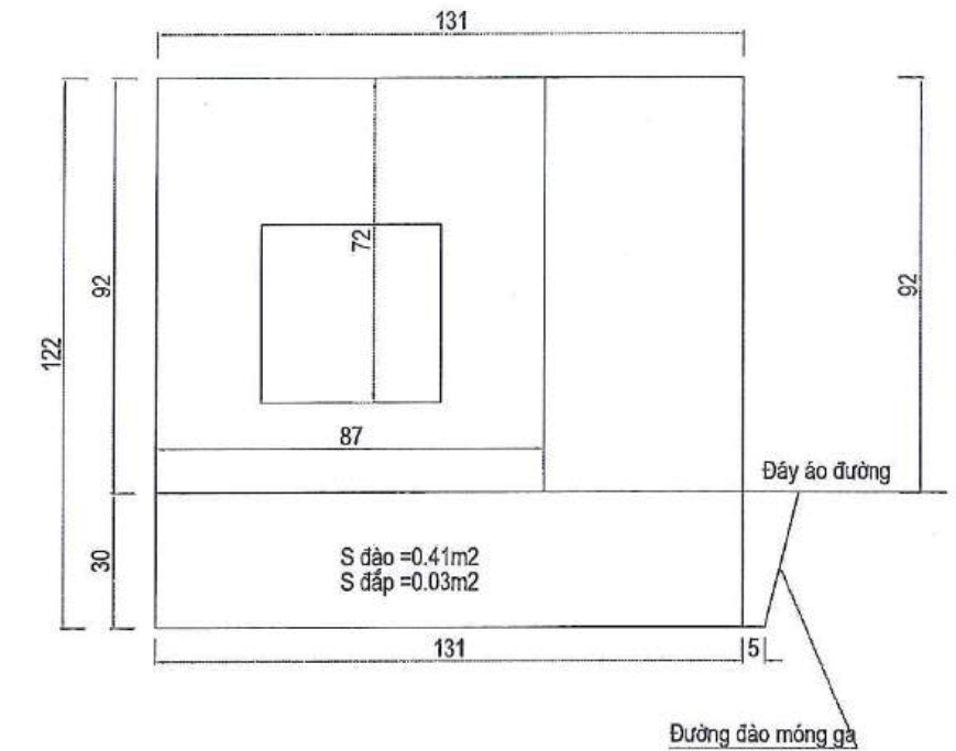
MẶT CẮT ĐÀO ĐẮP GA
