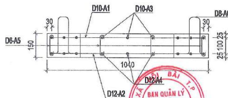
MẶT CẮT 2-2
