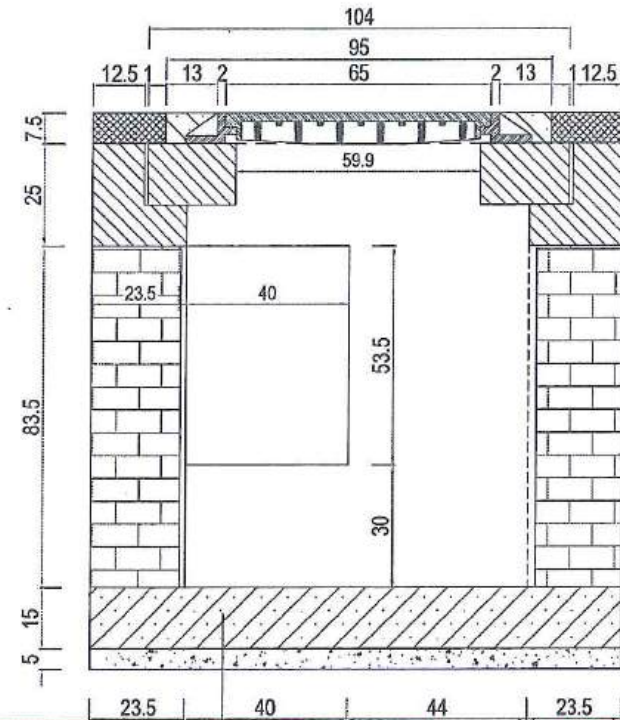
MẶT CẮT II - II
