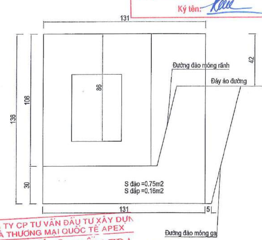
MẶT CẮT ĐÀO ĐẬP GA
