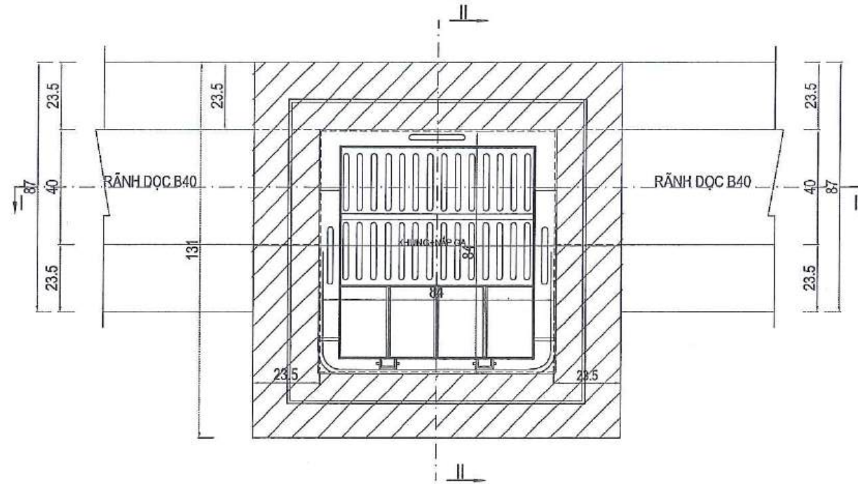
MẶT BẰNG HỐ GA
