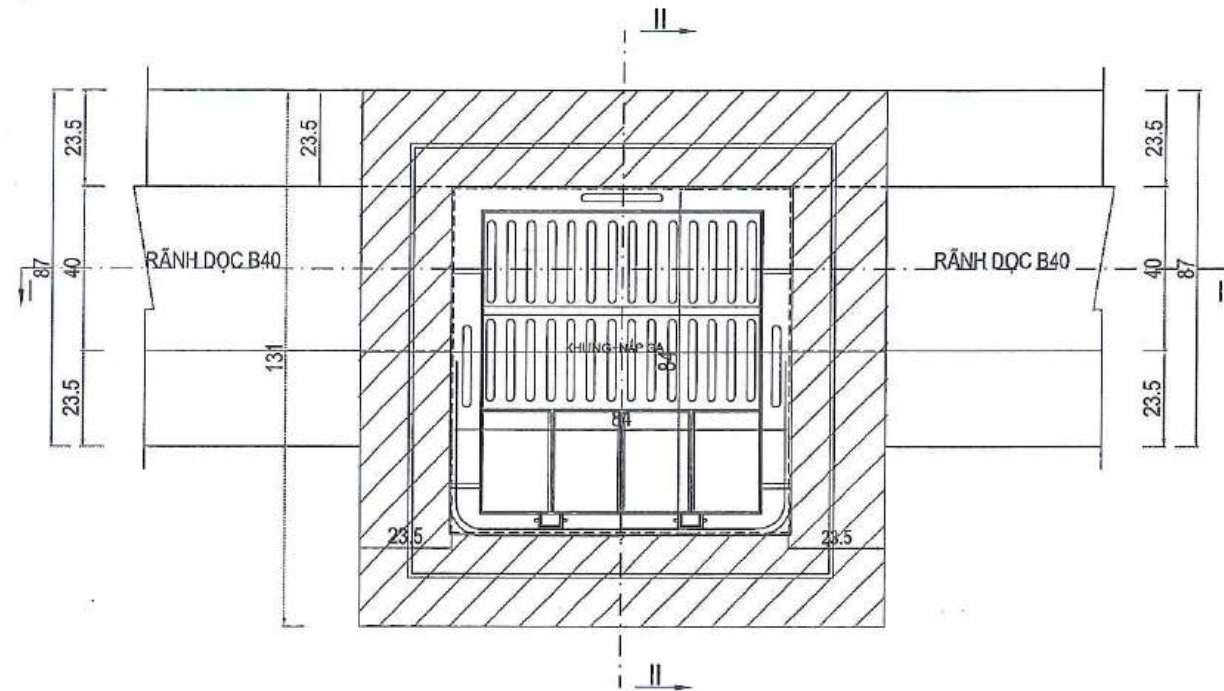
MẶT BẰNG HỔ GA
