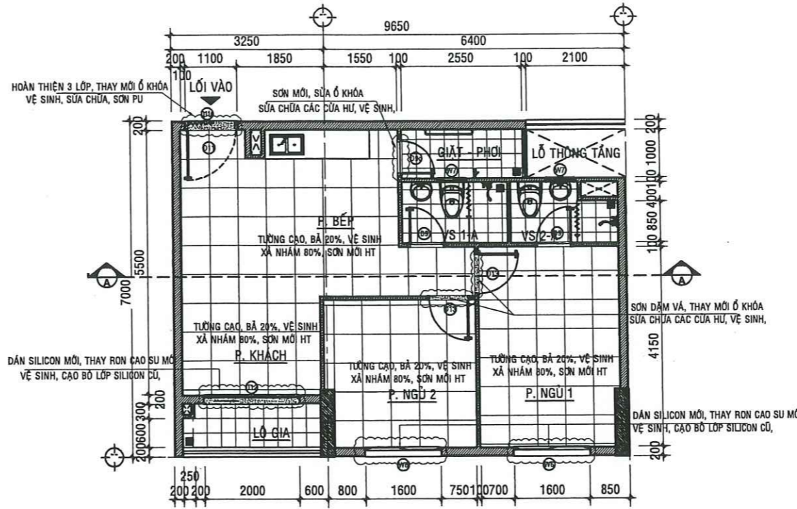
MẶT BẰNG SỬA CHỮA CĂN HỘ A - 09.01 - TL:1/50
