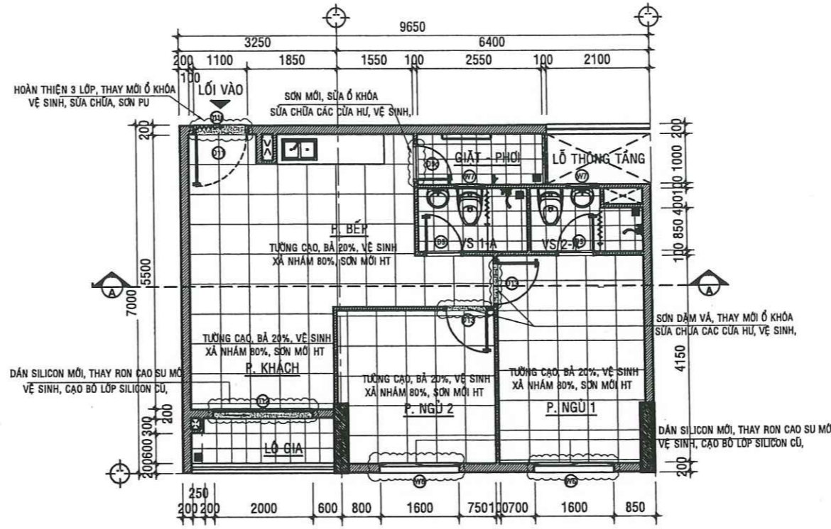
MẶT BẰNG SỬA CHỮA CĂN HỘ A - 10.01 - TL:1/50
