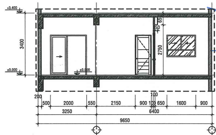
MẶT CẮT B-B - TL:1/50
