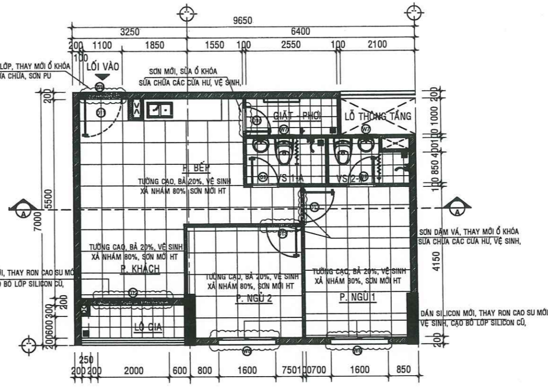
MẶT BẰNG SỬA CHỮA CĂN HỘ A - 12.08 - TL:1/50
