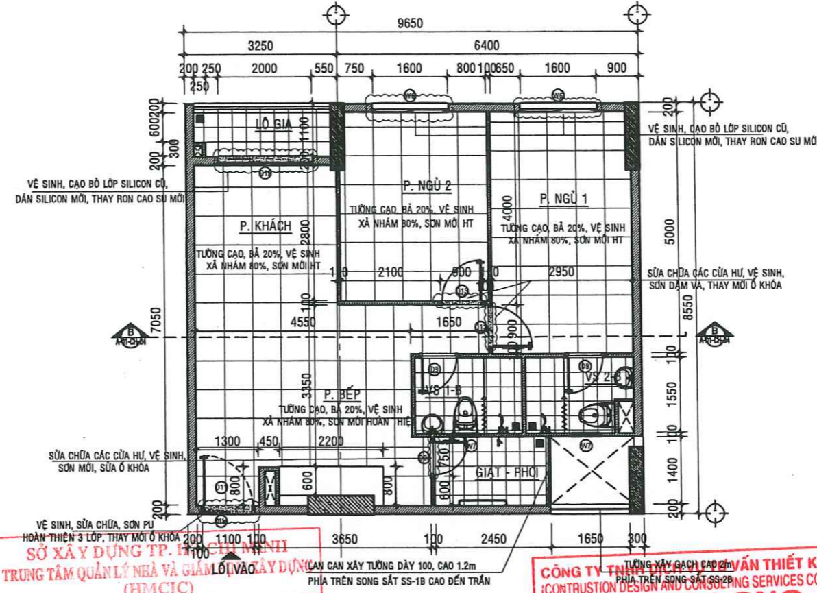
MẶT BẰNG SỬA CHỮA CĂN HỘ A - 12.06 - TL:1/50
