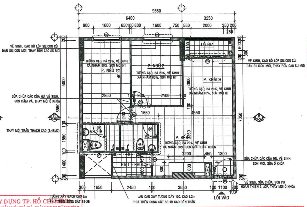
MẶT BẰNG SỬA CHỮA CĂN HỘ A -04.03 - TL:1/50
