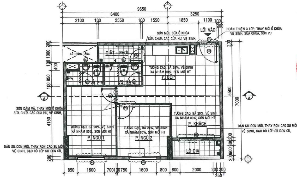
MẶT BẰNG SỬA CHỮA CĂN HỘ A - 11.02 - TL:1/50
