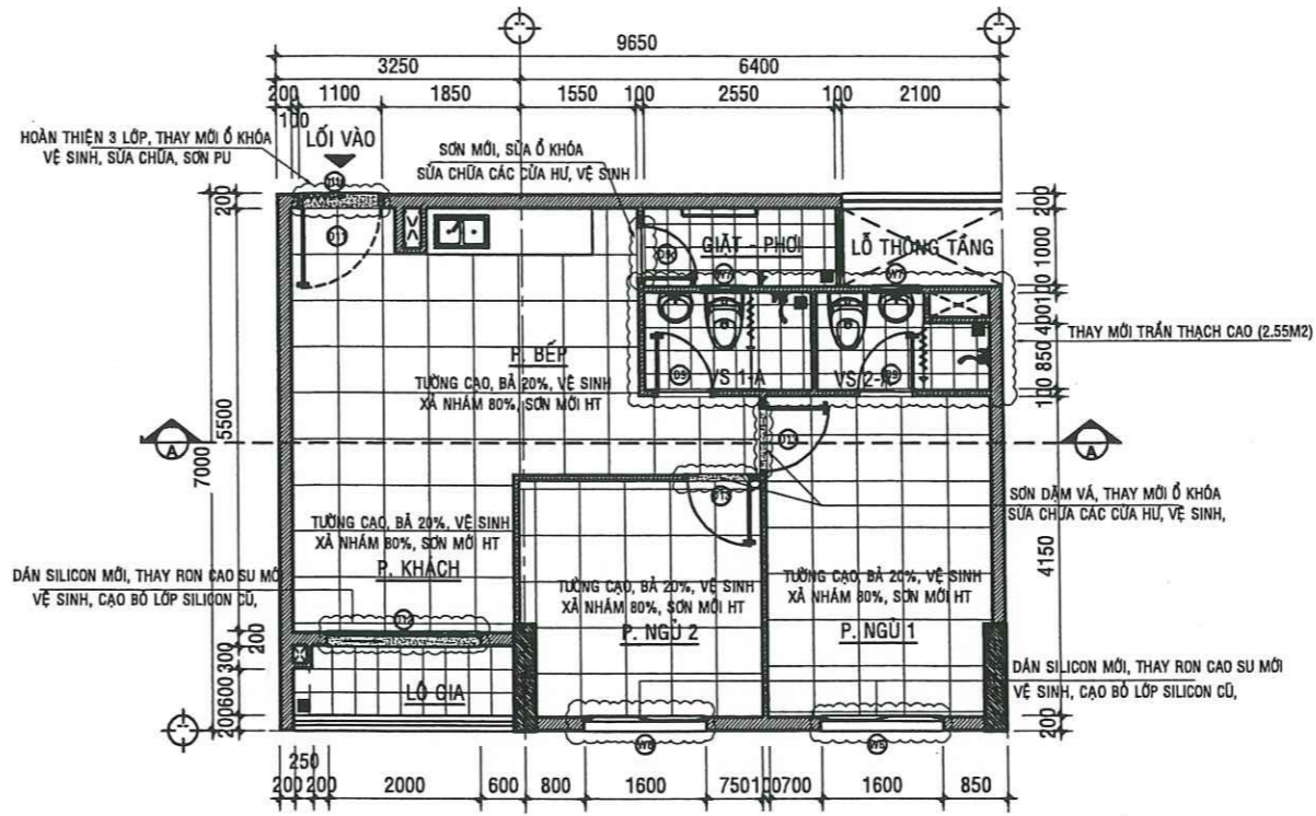
MẶT BẰNG SỬA CHỮA CĂN HỘ A -04.08 - TL:1/50
