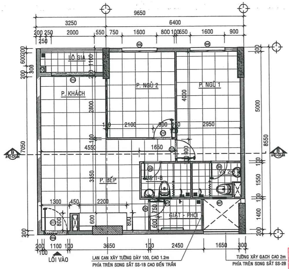
MẶT BẰNG HIỆN TRẠNG CĂN HỘ A - 13.04 - TL:1/50
