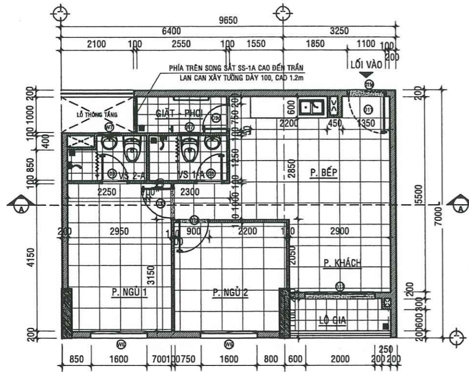
MẶT BẰNG HIỆN TRẠNG CĂN HỘ A -04.02 - TL:1/50
