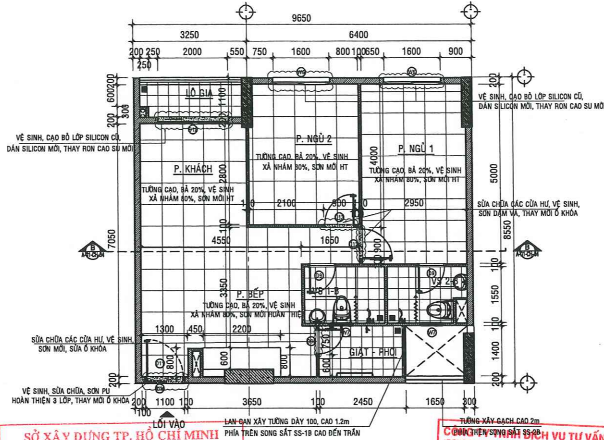
MẶT BẰNG SỬA CHỮA CĂN HỘ A - 06.06 - TL:1/50
