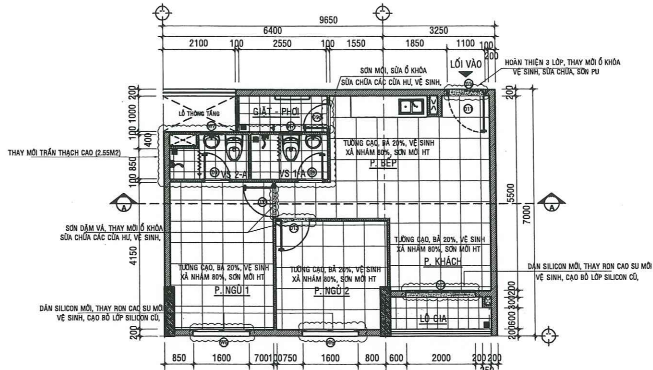
MẶT BẰNG SỬA CHỮA CĂN HỘ A -04.02 - TL:1/50
