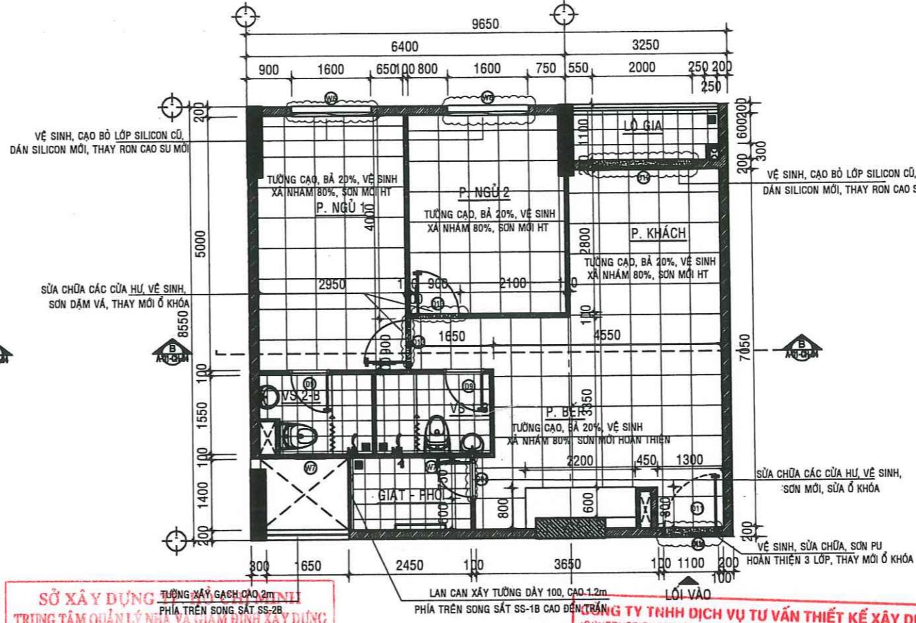
MẶT BẰNG SỬA CHỮA CĂN HỘ A - 12.05 - TL:1/50
