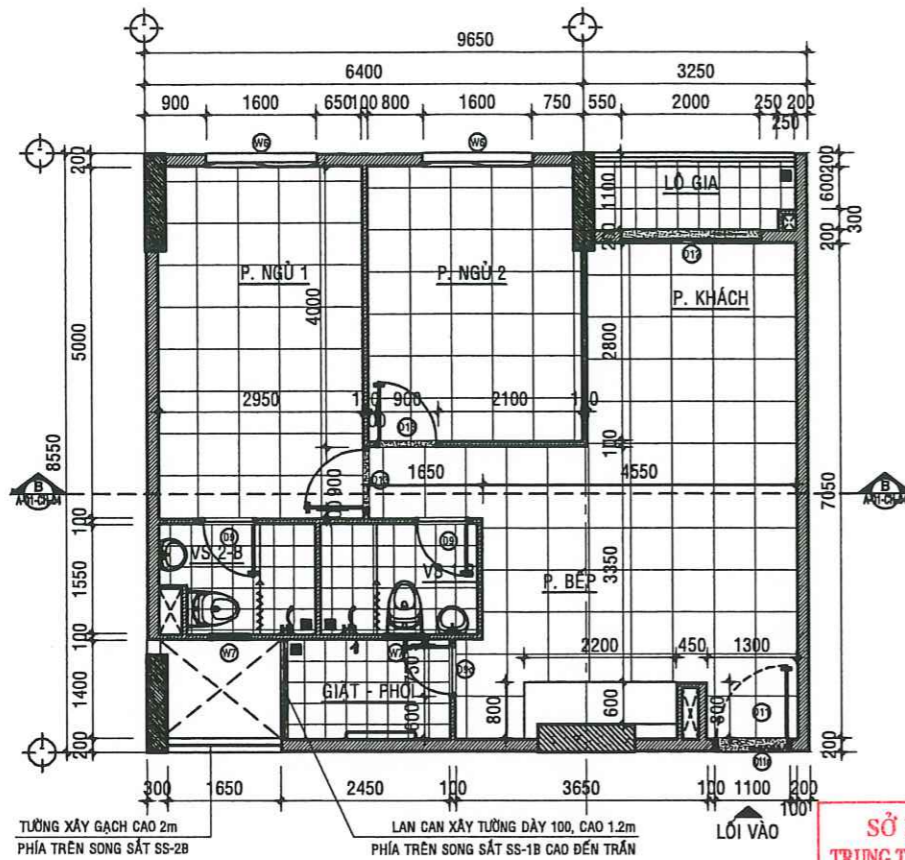
MẶT BẰNG HIỆN TRẠNG CĂN HỘ A - 05.05 - TL:1/50
