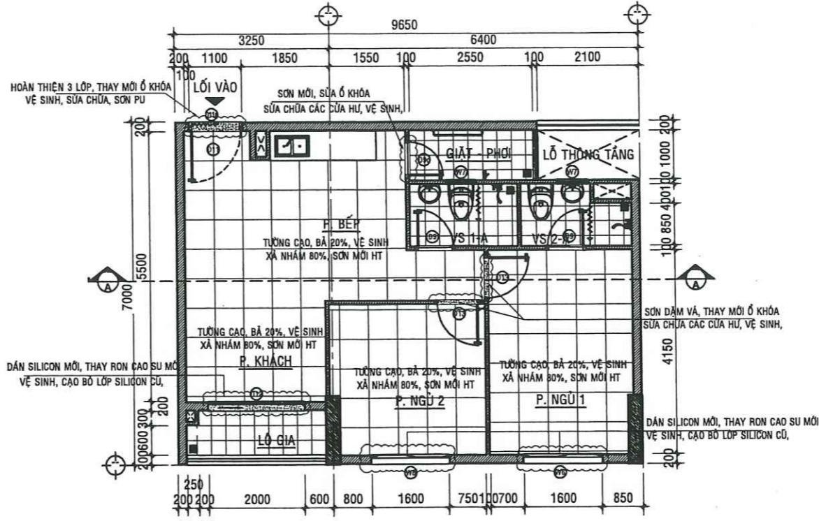
MẶT BẰNG SỬA CHỮA CĂN HỘ A - 11.01 - TL:1/50
