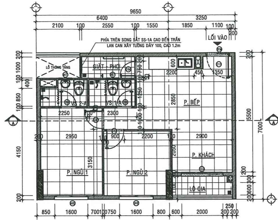
MẶT BẰNG HIỆN TRẠNG CĂN HỘ A - 09.02 - TL:1/50
