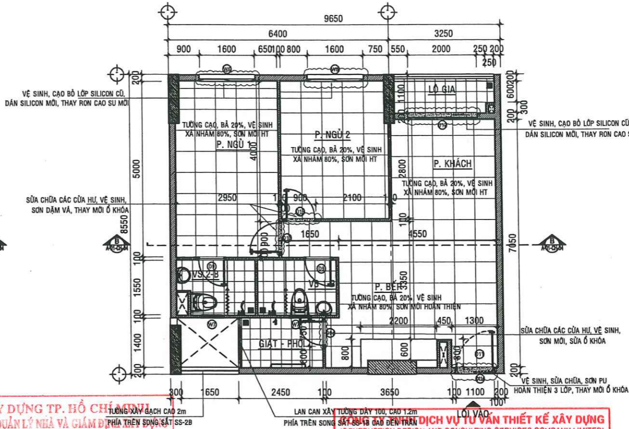
MẶT BẰNG SỬA CHỮA CĂN HỘ A - 10.03 - TL:1/50
