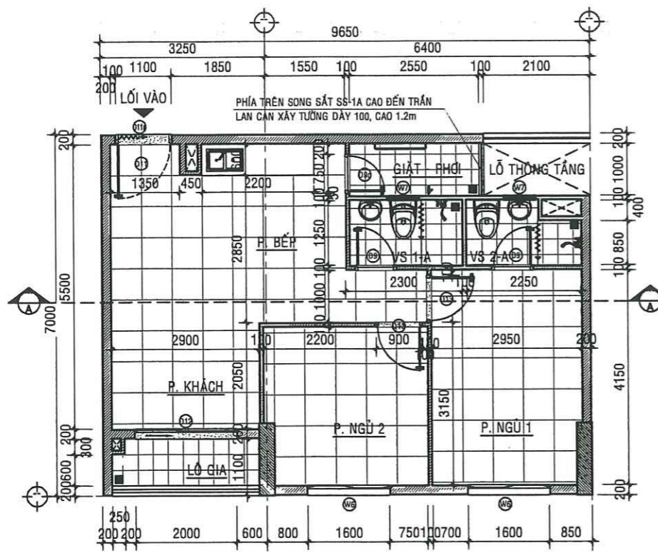
MẶT BẰNG HIỆN TRẠNG CĂN HỘ A - 14.01 - TL:1/50
