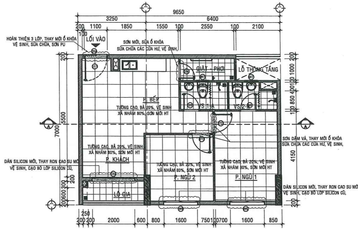
MẶT BẰNG SỬA CHỮA CĂN HỘ A - 05.01 - TL:1/50
