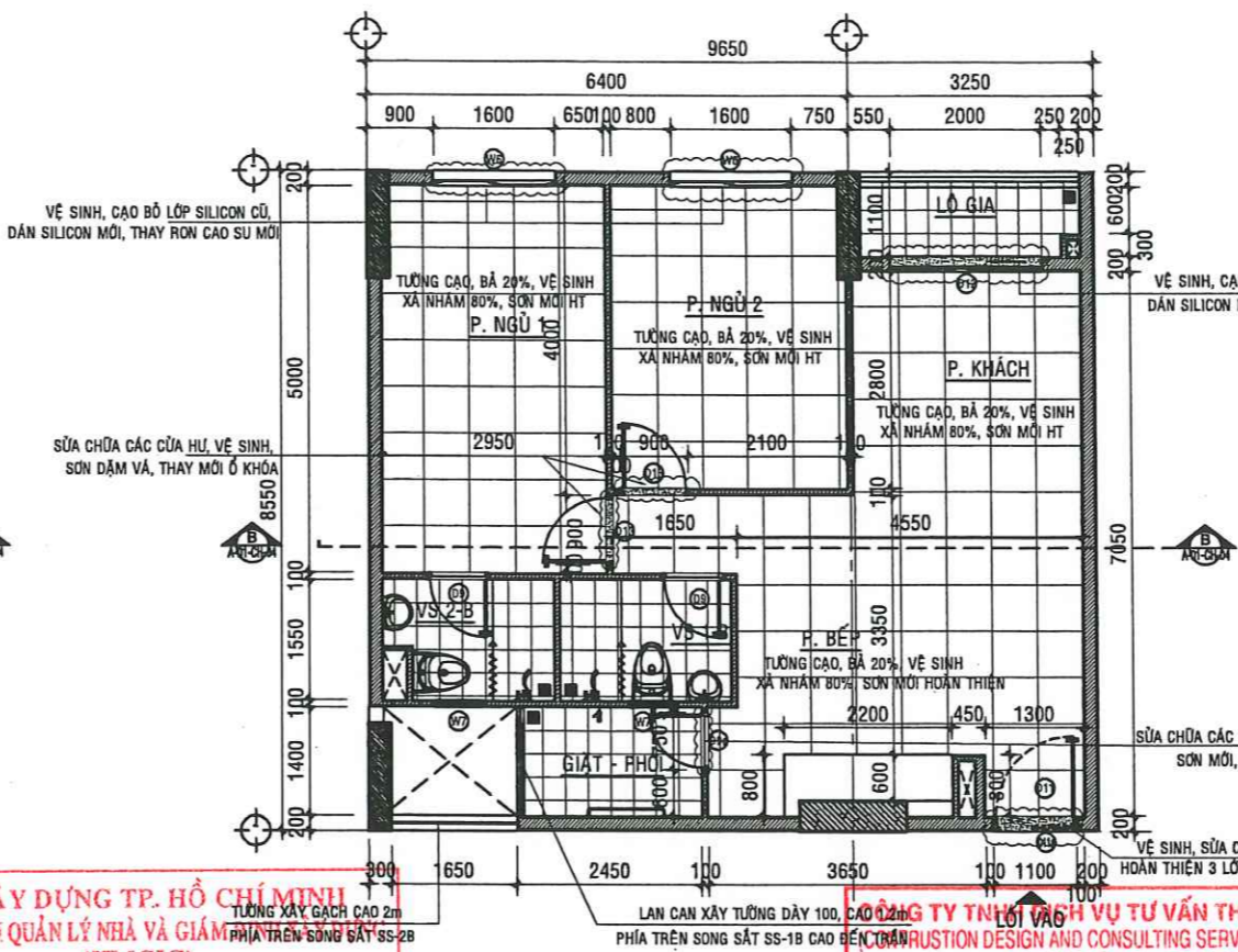
MẶT BẰNG SỬA CHỮA CĂN HỘ A -03.05 - TL:1/50
