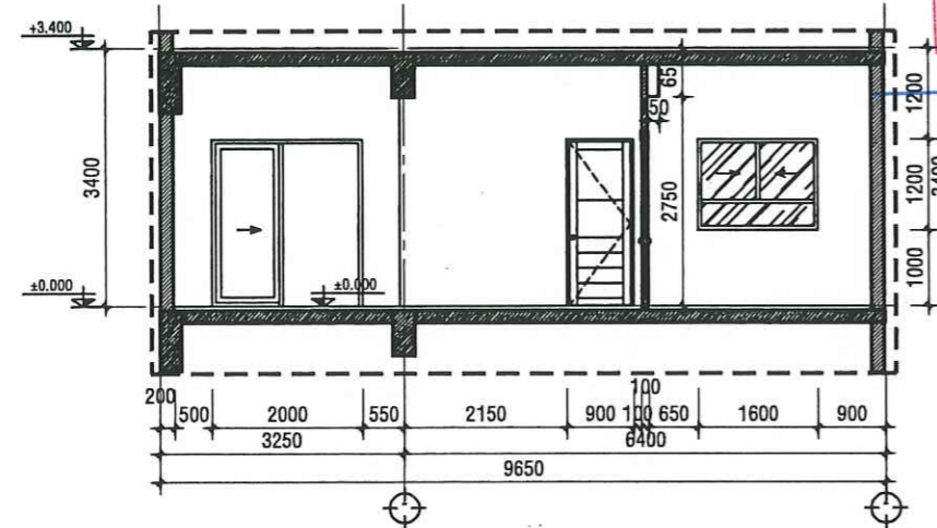
MẶT CẮT B-B - TL:1/50
