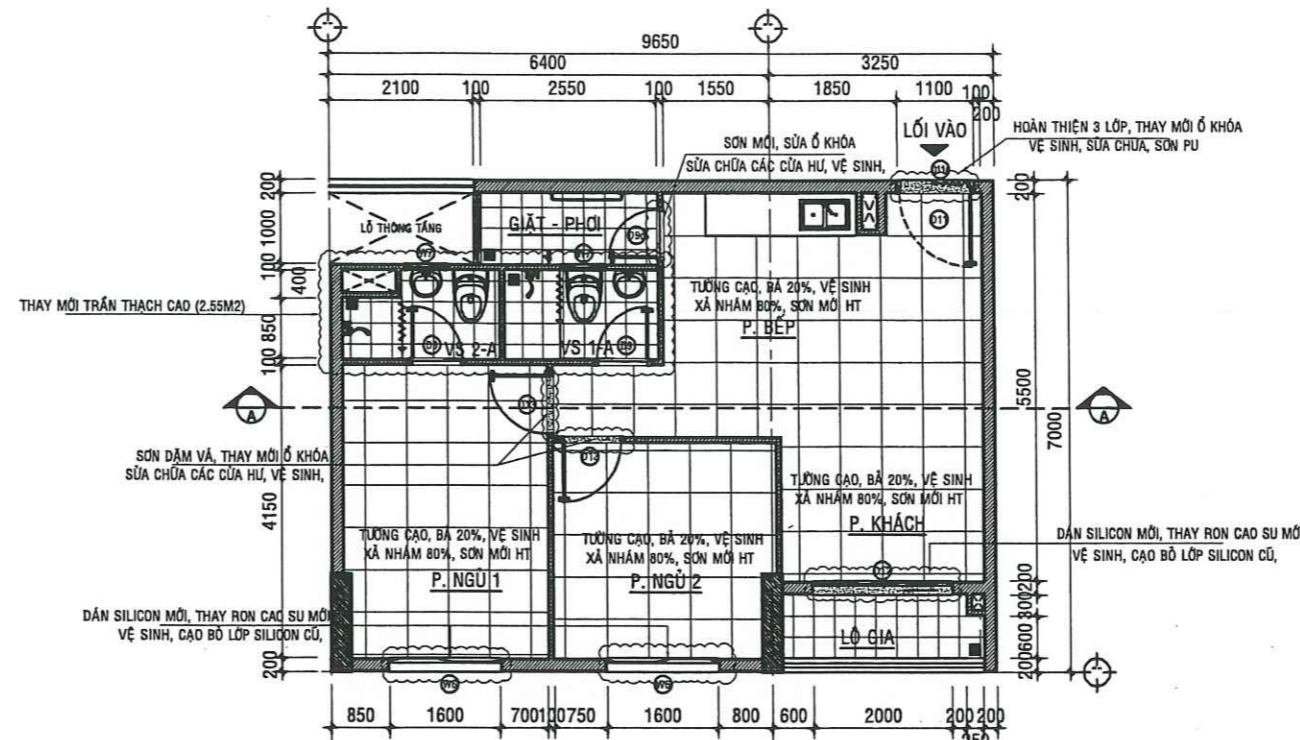
MẶT BẰNG SỬA CHỮA CĂN HỘ A -02.02 - TL:1/50
