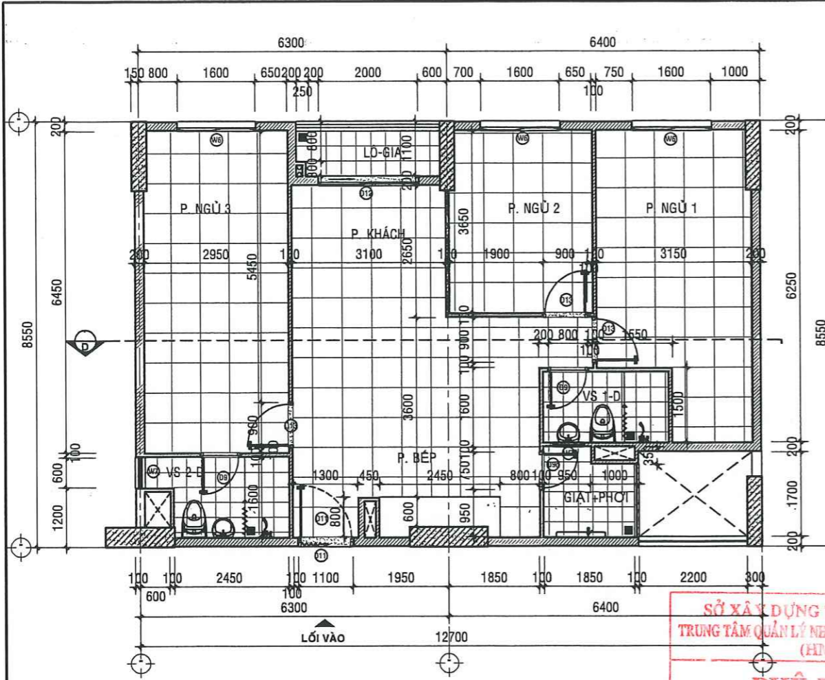
MẶT BẰNG HIỆN TRẠNG CĂN HỘ A - 15.03 - TL: 1/50
