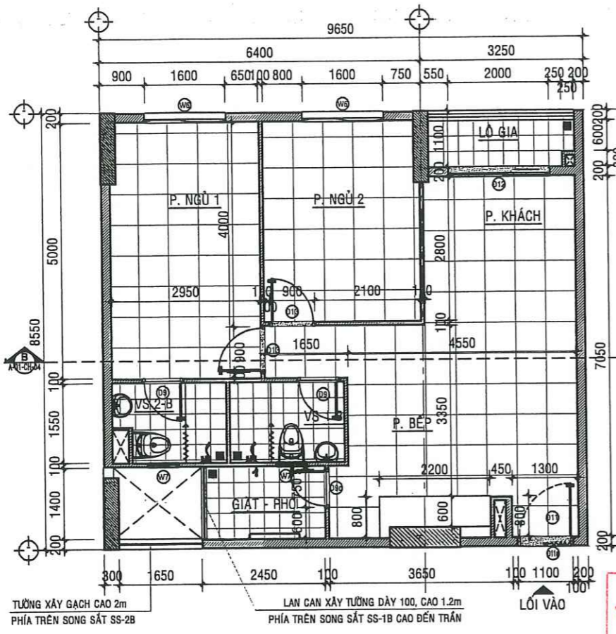
MẶT BẰNG HIỆN TRẠNG CĂN HỘ A - 14.05 - TL:1/50
