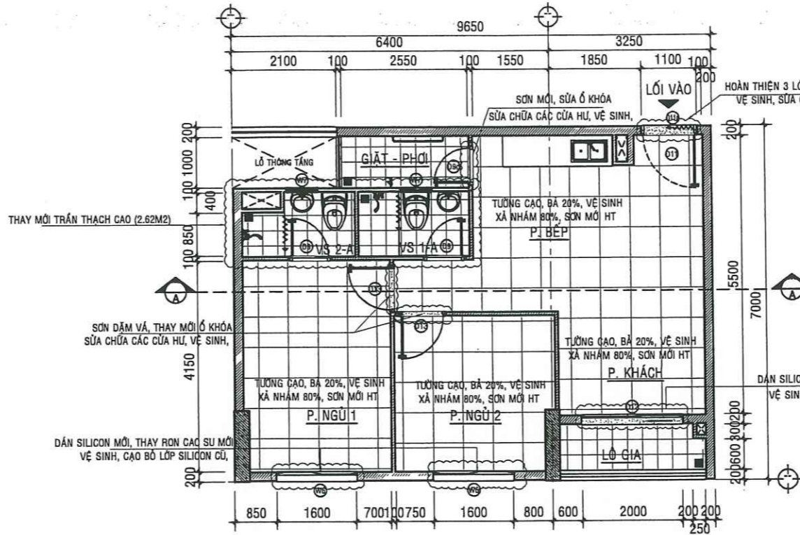
MẶT BẰNG SỬA CHỮA CĂN HỘ A - 14.02 - TL:1/50
