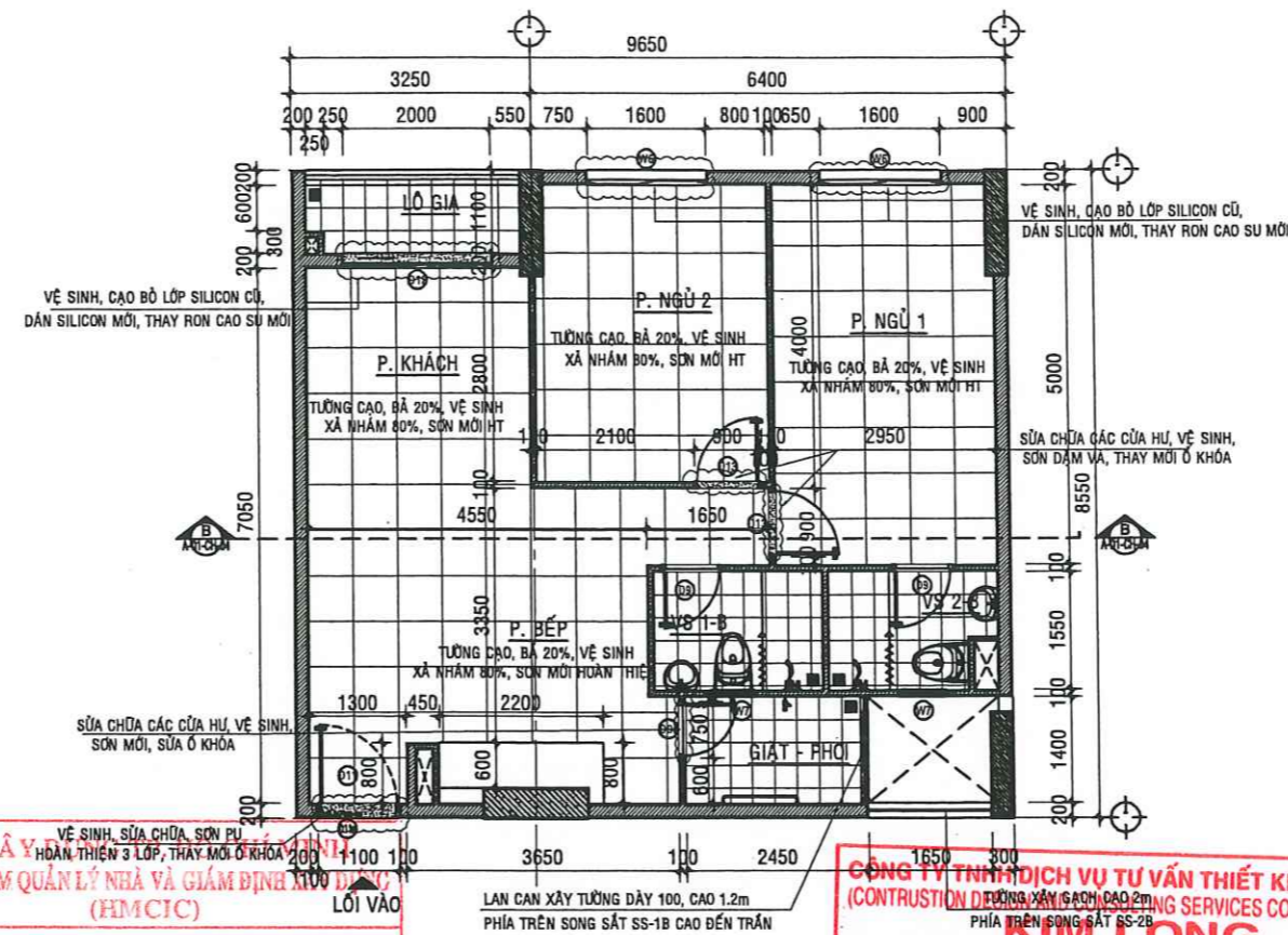
MẶT BẰNG SỬA CHỮA CĂN HỘ A - 09.06 - TL:1/50
