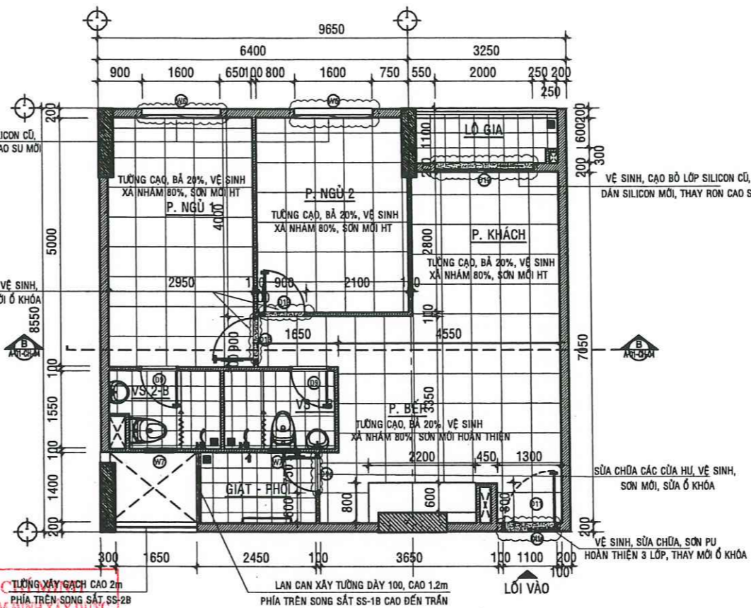
MẶT BẰNG SỬA CHỮA CĂN HỘ A - 07.03 - TL:1/50
