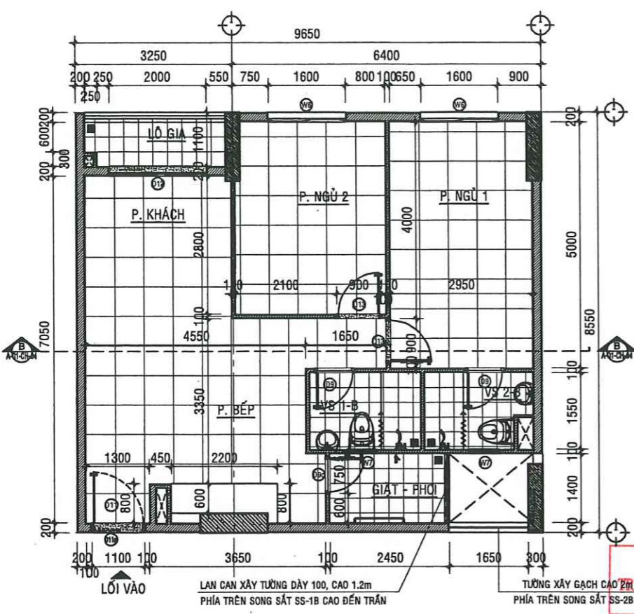
MẶT BẰNG HIỆN TRẠNG CĂN HỘ A -03.06 - TL:1/50
