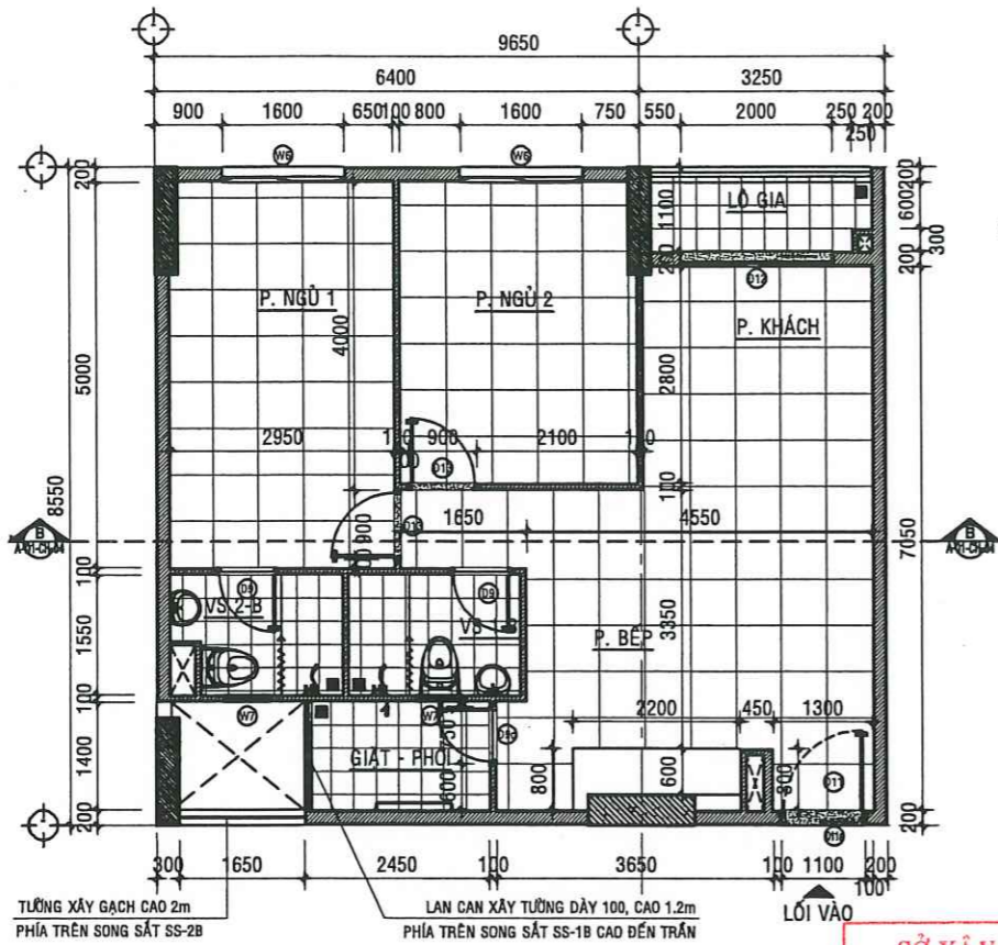
MẶT BẰNG HIỆN TRẠNG CĂN HỘ A - 07.05 - TL:1/50
