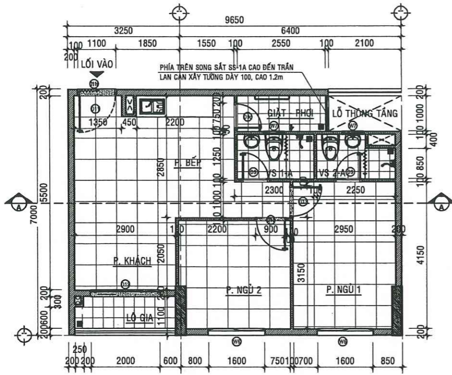
MẶT BẰNG HIỆN TRẠNG CĂN HỘ A - 05.01 - TL:1/50
