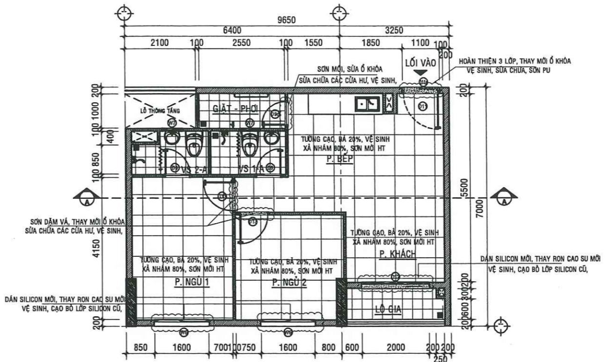
MẶT BẰNG SỬA CHỮA CĂN HỘ A - 07.02 - TL:1/50
