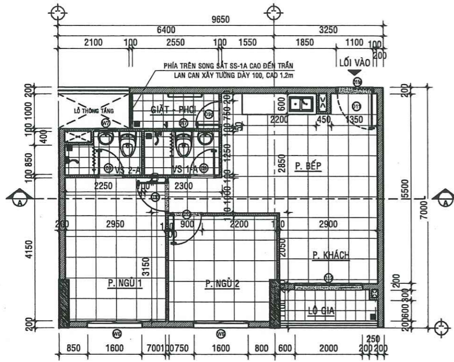
MẶT BẰNG HIỆN TRẠNG CĂN HỘ A -02.09 - TL:1/50
