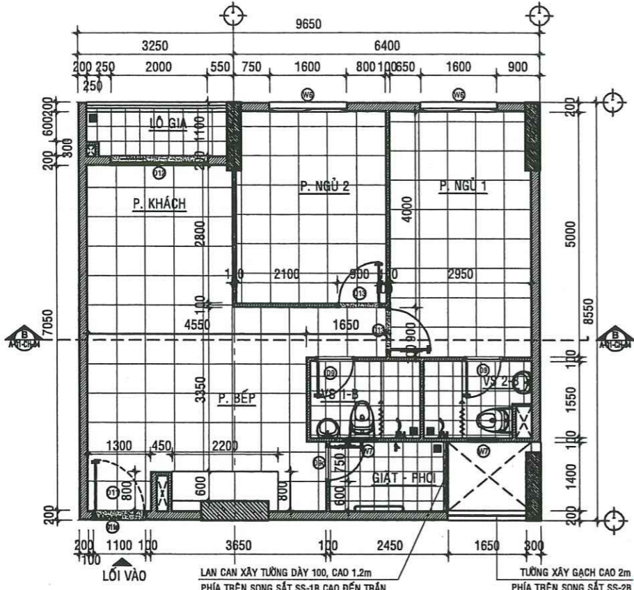
MẶT BẰNG HIỆN TRẠNG CĂN HỘ A -02.04 - TL:1/50
