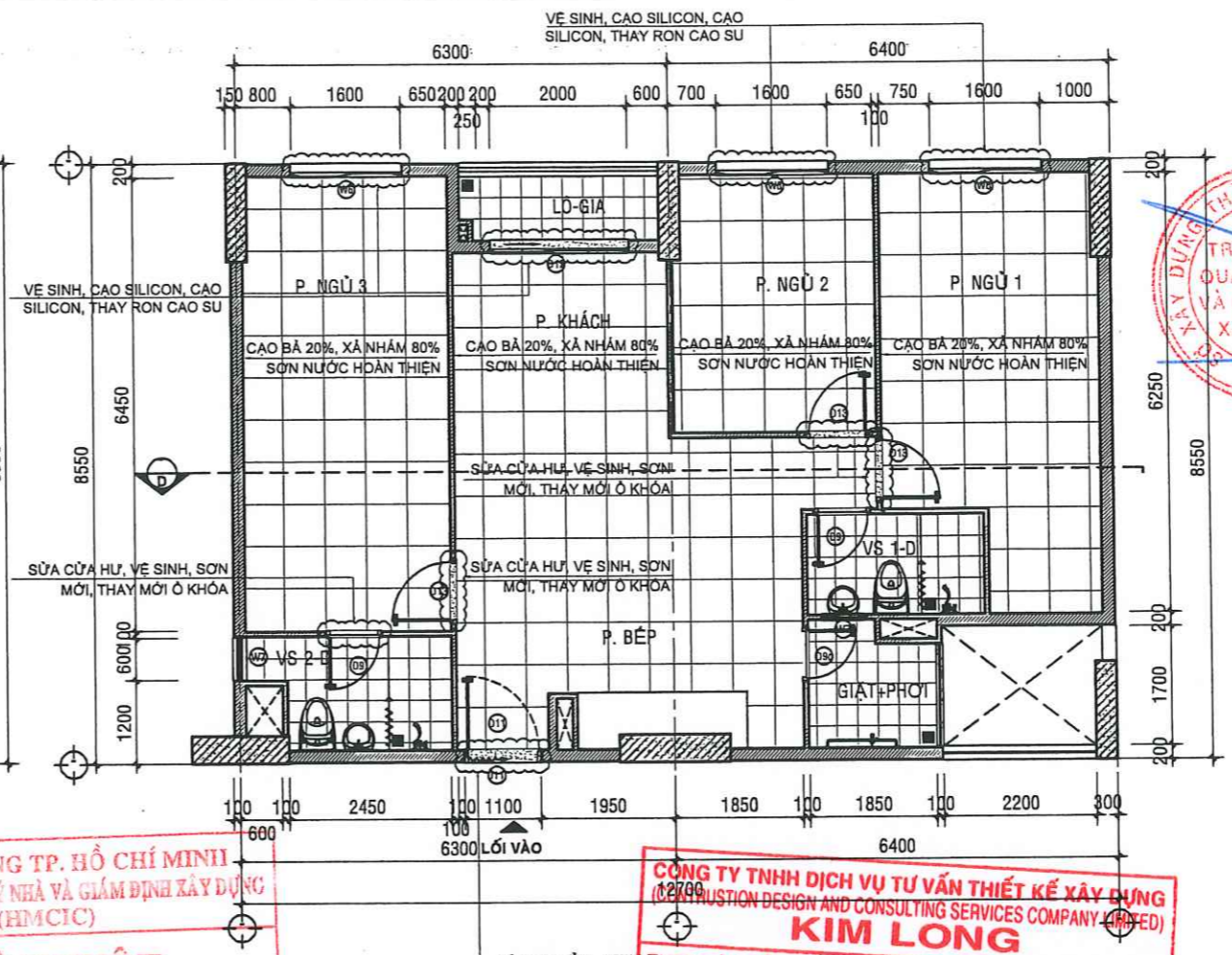
MẶT BẰNG SỬA CHỮA CĂN HỘ A - 13.07 - TL: 1/50
