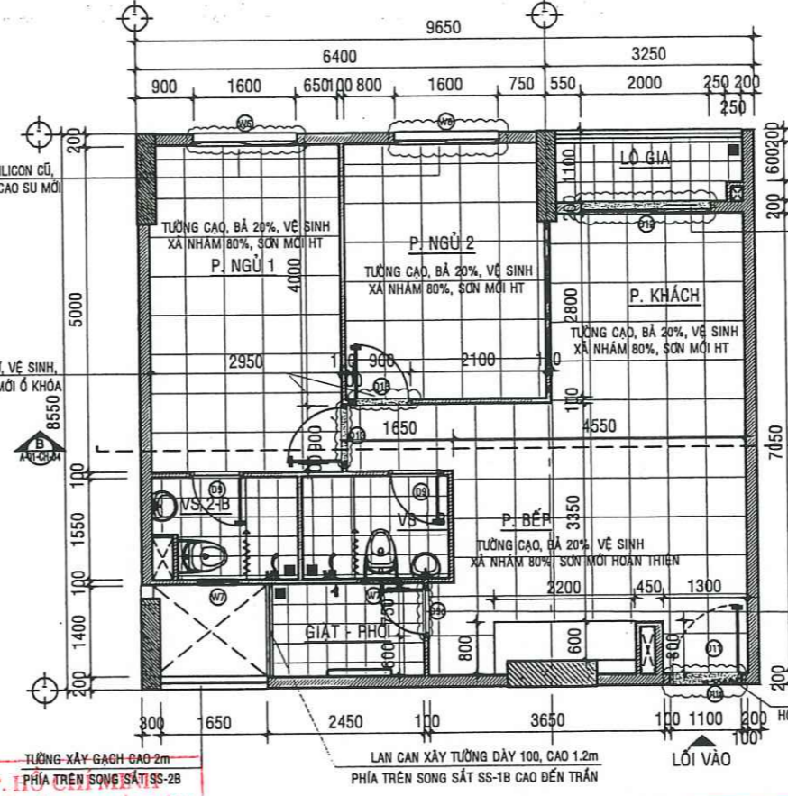
MẶT BẰNG SỬA CHỮA CĂN HỘ A - 13.03 - TL:1/50
