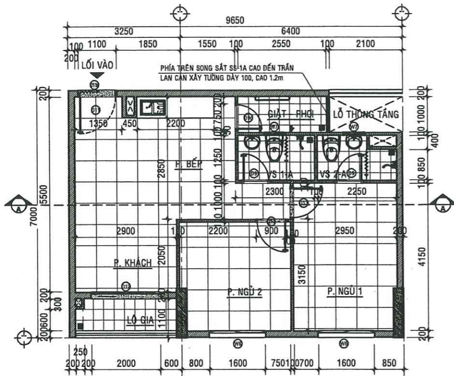
MẶT BẰNG HIỆN TRẠNG CĂN HỘ A - 07.01 - TL:1/50
