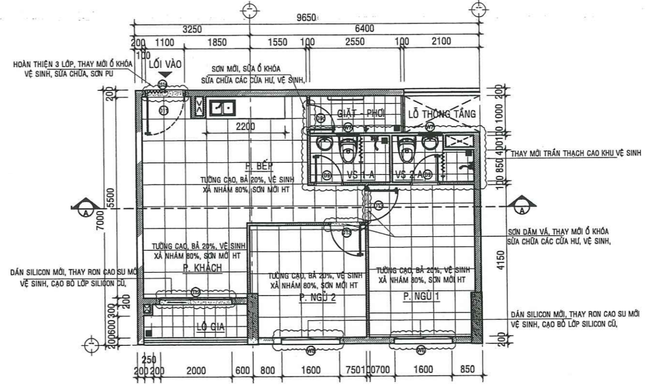
MẶT BẰNG SỬA CHỮA CĂN HỘ A - 15.04 - TL:1/50
