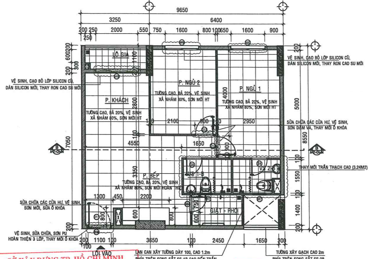
MẶT BẰNG SỬA CHỮA CĂN HỘ A -02.04 - TL:1/50
