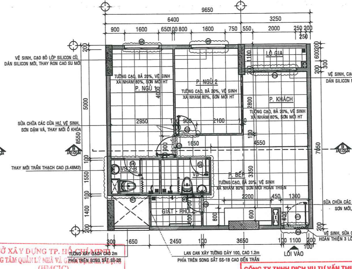
MẶT BẰNG SỬA CHỮA CĂN HỘ A - 14.05 - TL:1/50
