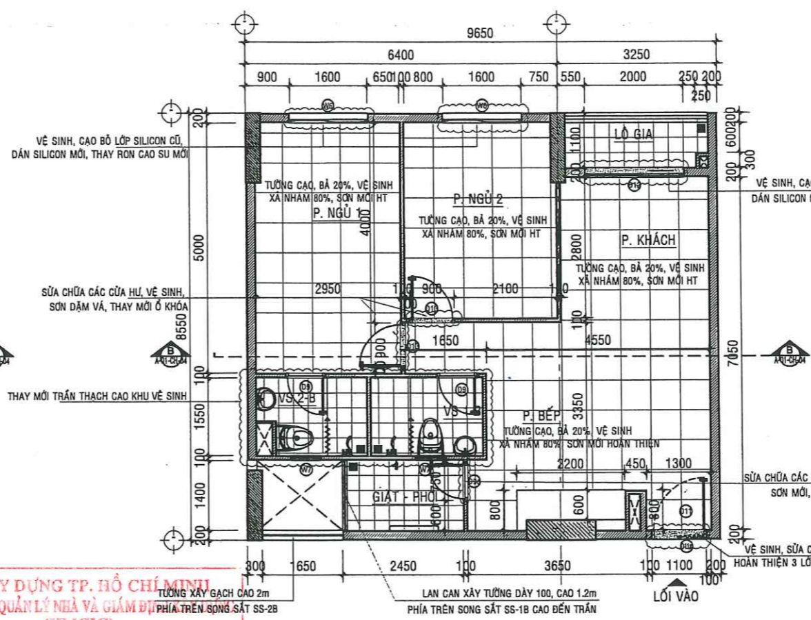
MẶT BẰNG SỬA CHỮA CĂN HỘ A - 15.01 - TL:1/50
