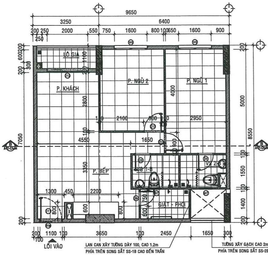
MẶT BẰNG HIỆN TRẠNG CĂN HỘ A - 06.06 - TL:1/50
