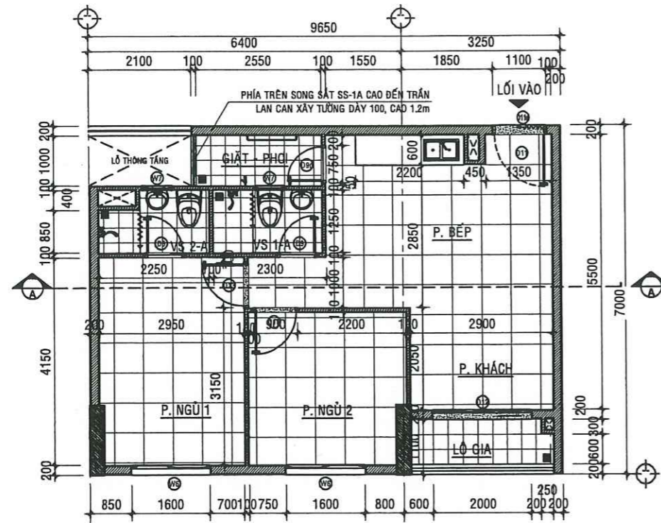
MẶT BẰNG HIỆN TRẠNG CĂN HỘ A - 10.02 - TL:1/50
