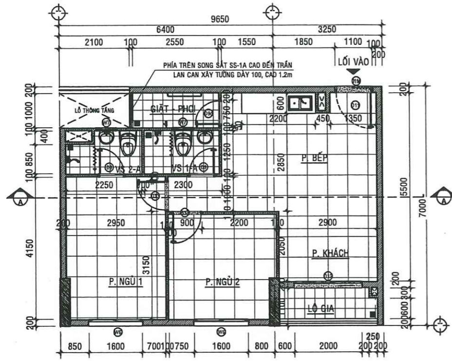
MẶT BẰNG HIỆN TRẠNG CĂN HỘ A - 11.09 - TL:1/50
