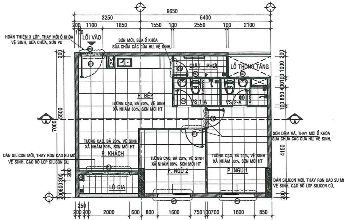
MẶT BẰNG SỬA CHỮA CĂN HỘ A -03.08 - TL:1/50
