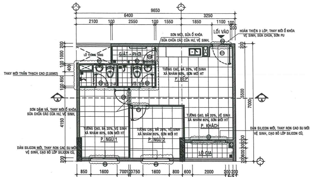
MẶT BẰNG SỬA CHỮA CĂN HỘ A -01.05 - TL:1/50
