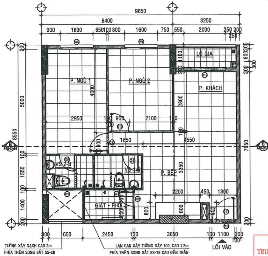
MẶT BẰNG HIỆN TRẠNG CĂN HỘ A - 11.05 - TL:1/50
