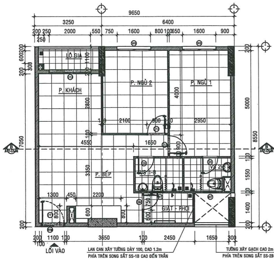
MẶT BẰNG HIỆN TRẠNG CĂN HỘ A - 07.04 - TL:1/50
