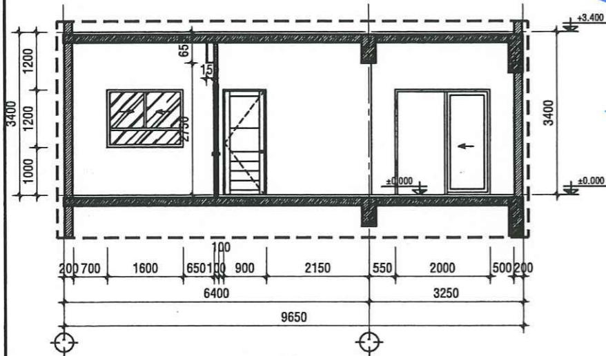
MẶT CẮT B-B - TL:1/50
