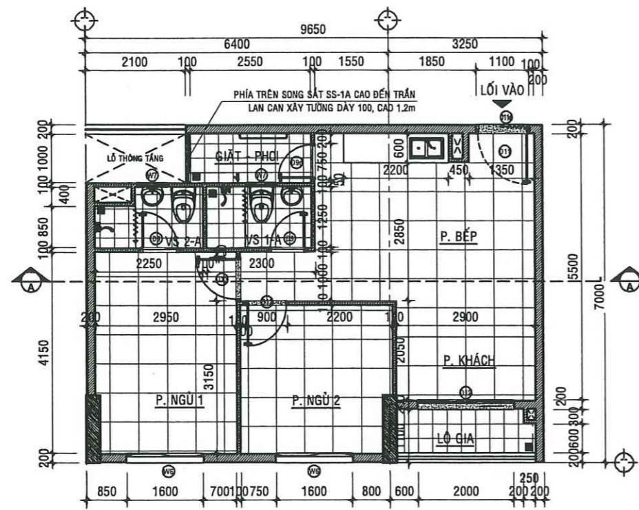
MẶT BẰNG HIỆN TRẠNG CĂN HỘ A -04.09 - TL:1/50
