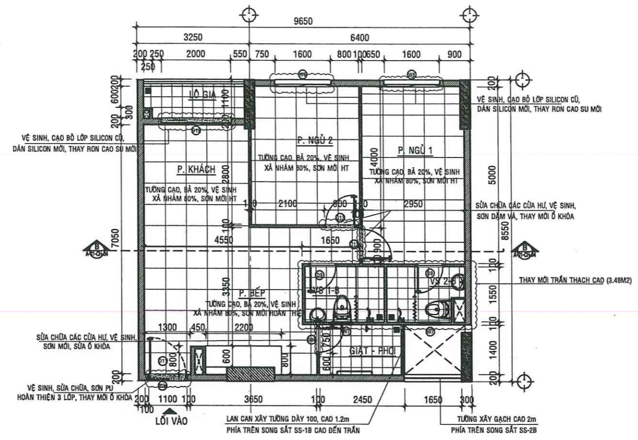
MẶT BẰNG SỬA CHỮA CĂN HỘ A -01.02 - TL:1/50
