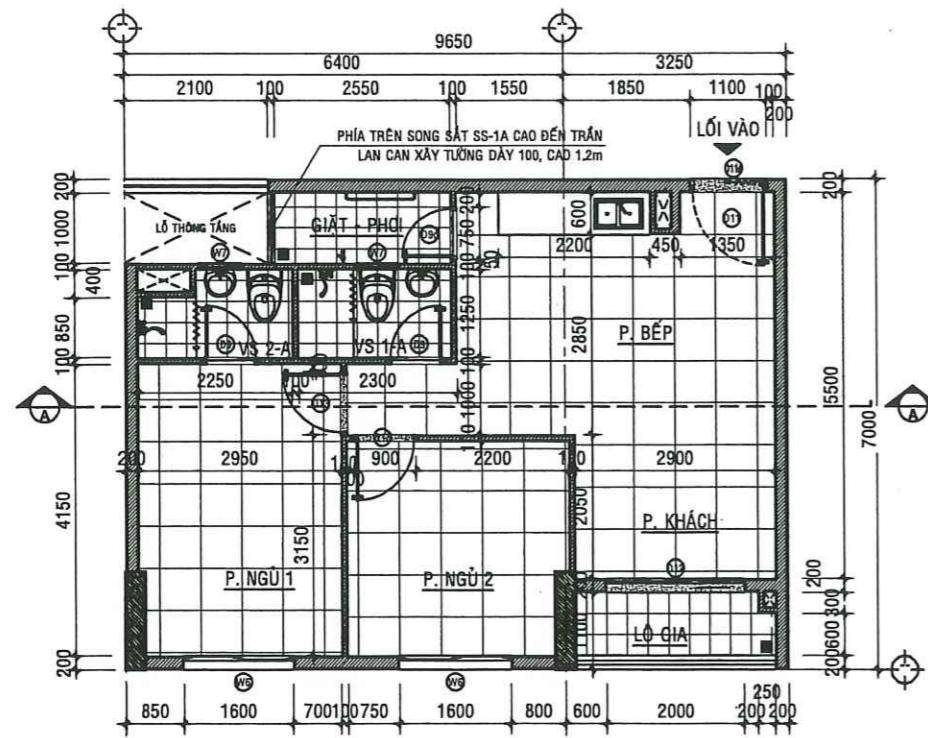
MẶT BẰNG HIỆN TRẠNG CĂN HỘ A - 07.09 - TL:1/50
