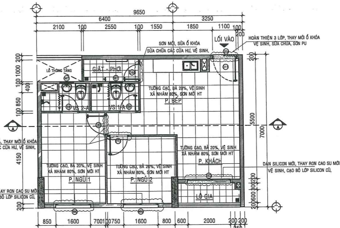
MẶT BẰNG SỬA CHỮA CĂN HỘ A - 13.09 - TL:1/50
