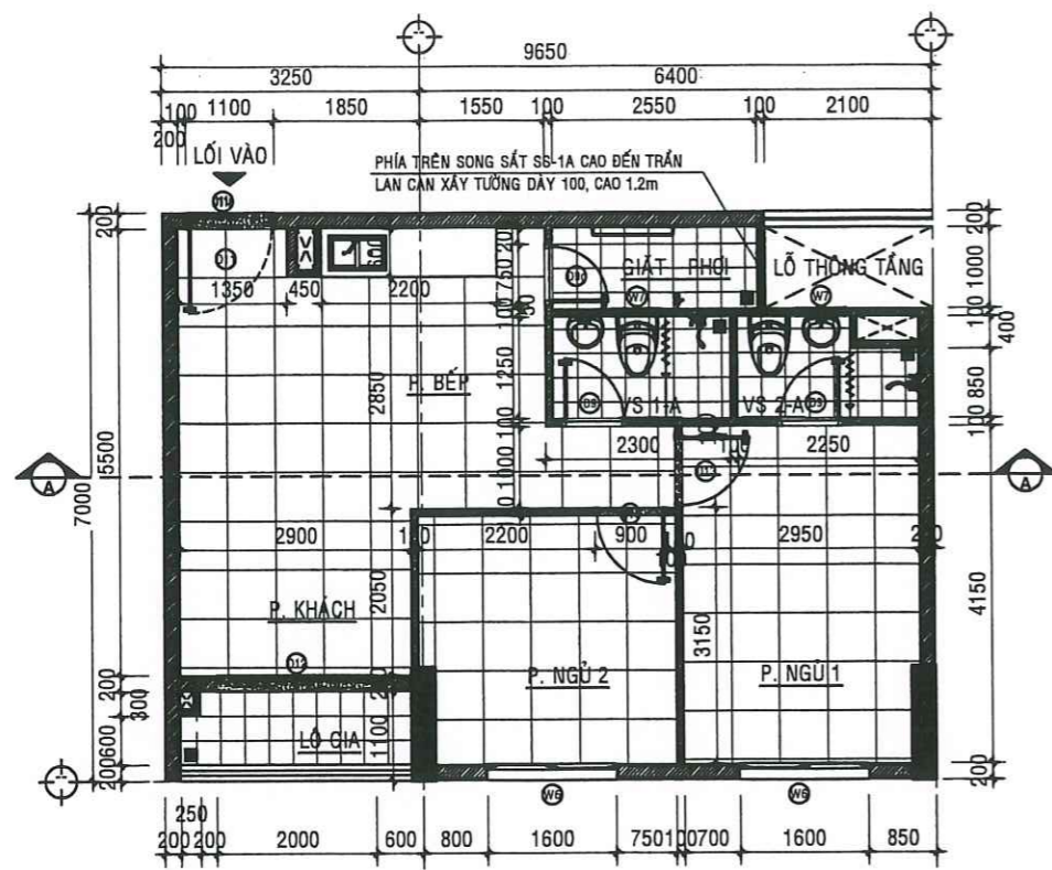
MẶT BẰNG HIỆN TRẠNG CĂN HỘ A - 12.08 - TL:1/50
