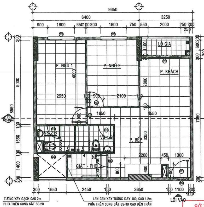
MẶT BẰNG HIỆN TRẠNG CĂN HỘ A -01.01 - TL:1/50
