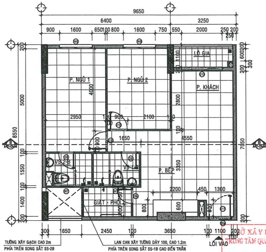
MẶT BẰNG HIỆN TRẠNG CĂN HỘ A - 09.05 - TL:1/50
