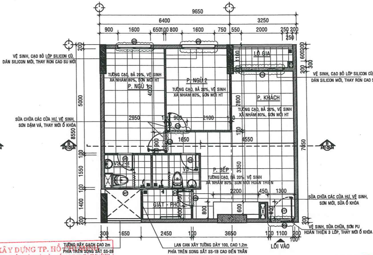
MẶT BẰNG SỬA CHỮA CĂN HỘ A - 12.03 - TL:1/50
