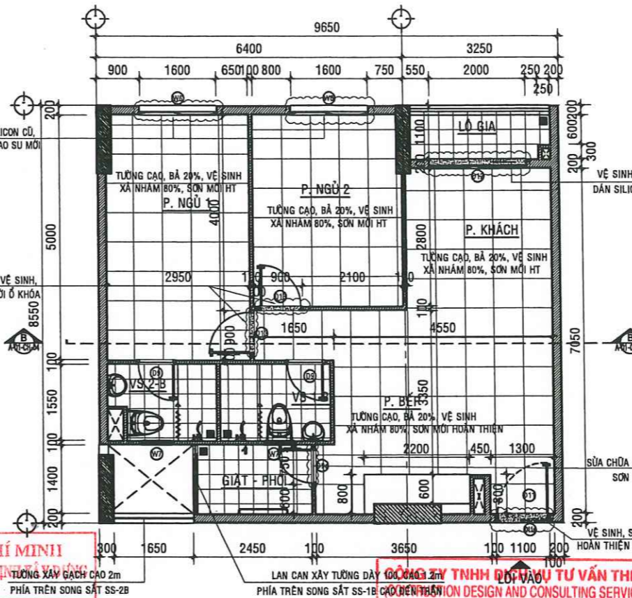
MẶT BẰNG SỬA CHỮA CĂN HỘ A - 09.05 - TL:1/50
