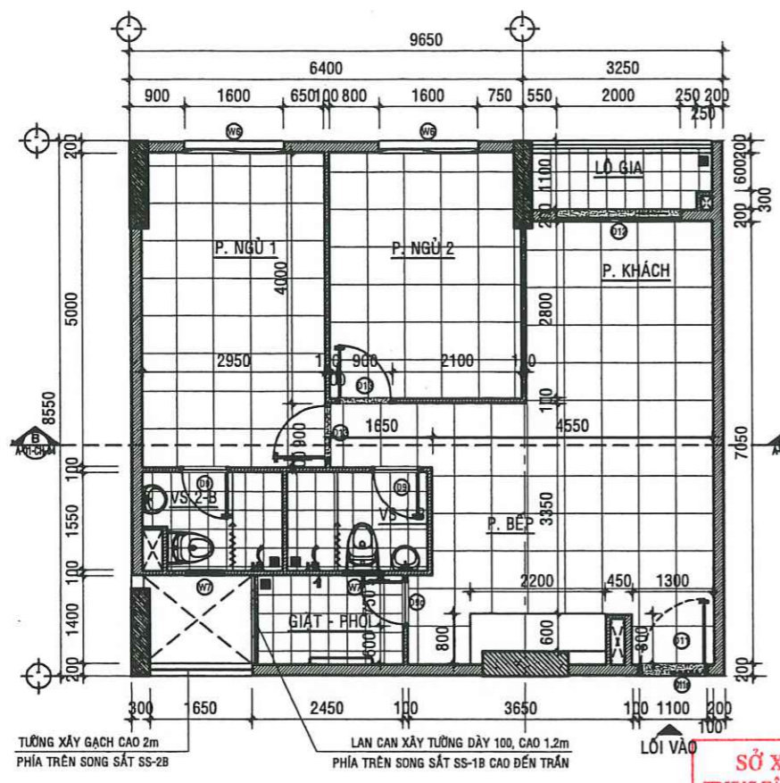
MẶT BẰNG HIỆN TRẠNG CĂN HỘ A -04.03 - TL:1/50
