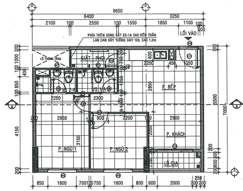
MẶT BẰNG HIỆN TRẠNG CĂN HỘ A - 07.02 - TL:1/50
