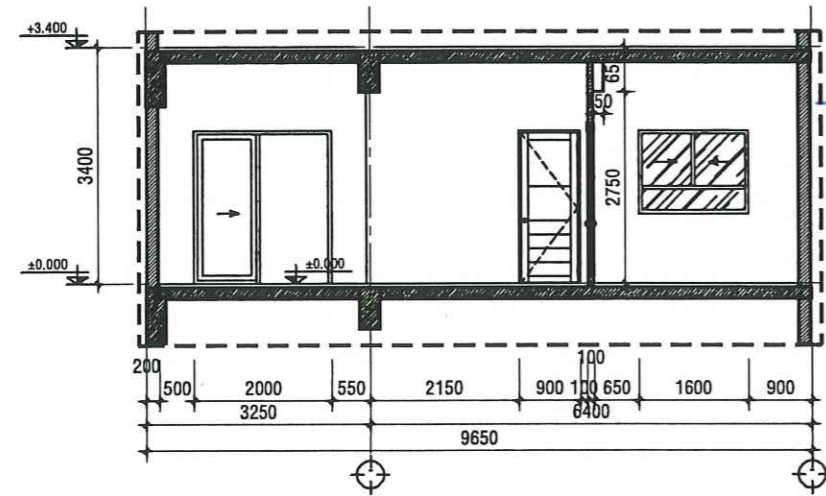
MẶT CẮT B-B - TL:1/50
