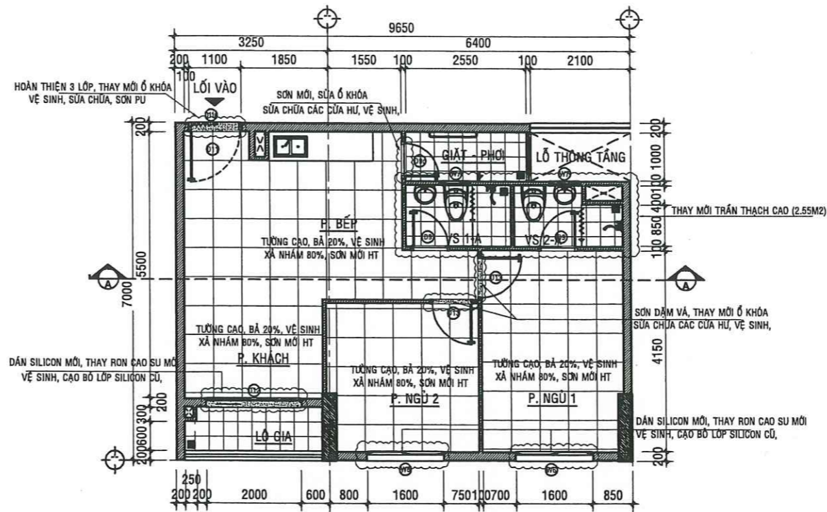
MẶT BẰNG SỬA CHỮA CĂN HỘ A -02.08 - TL:1/50
