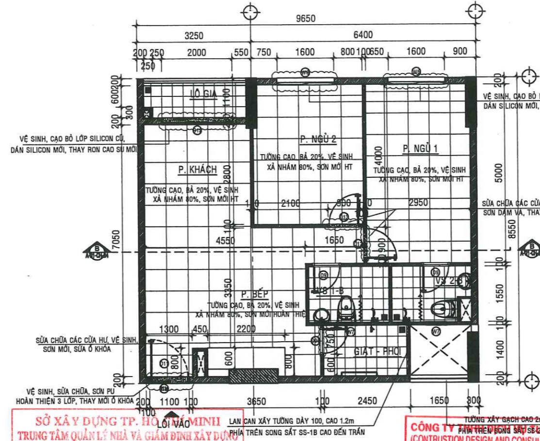
MẶT BẰNG SỬA CHỮA CĂN HỘ A - 11.06 - TL:1/50
