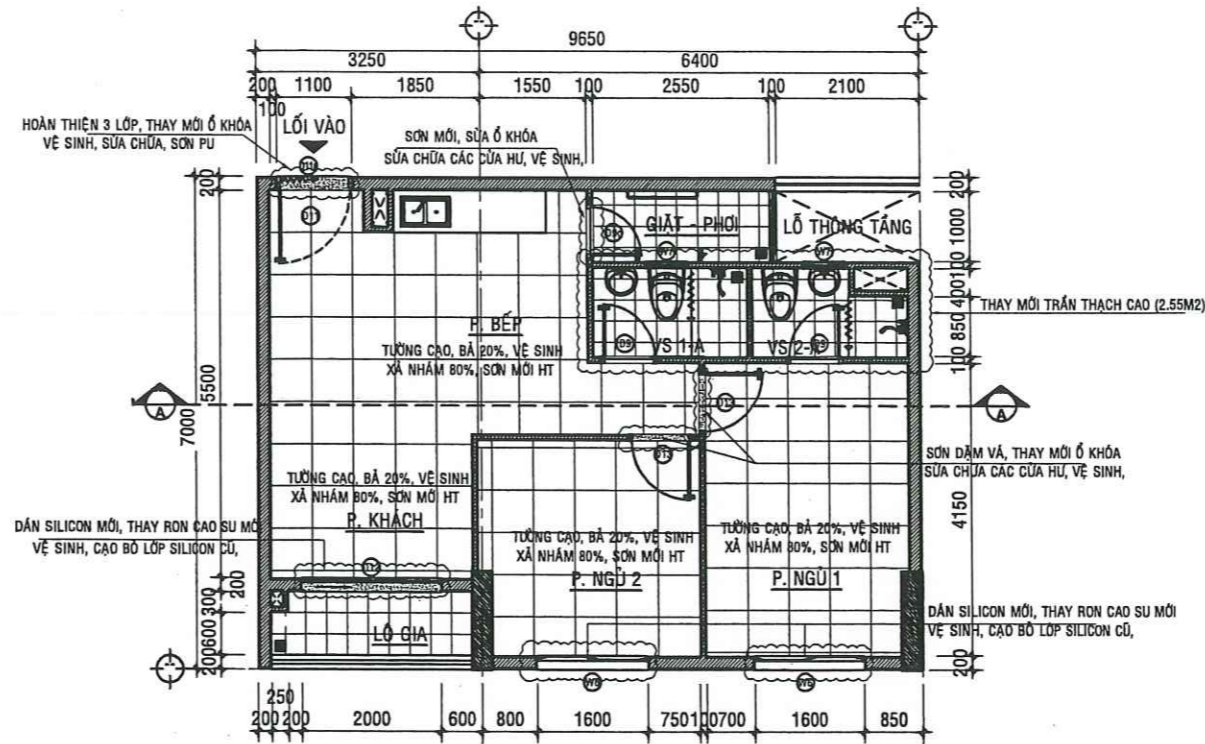
MẶT BẰNG SỬA CHỮA CĂN HỘ LOẠI A -02.01 - TL:1/50
