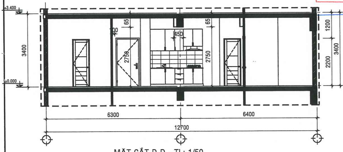
MẶT CẮT D-D - TL: 1/50
