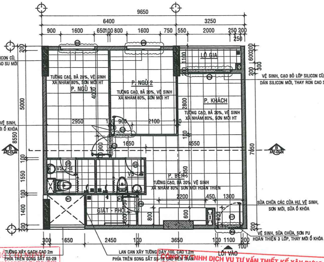
MẶT BẰNG SỬA CHỮA CĂN HỘ A - 09.03 - TL:1/50
