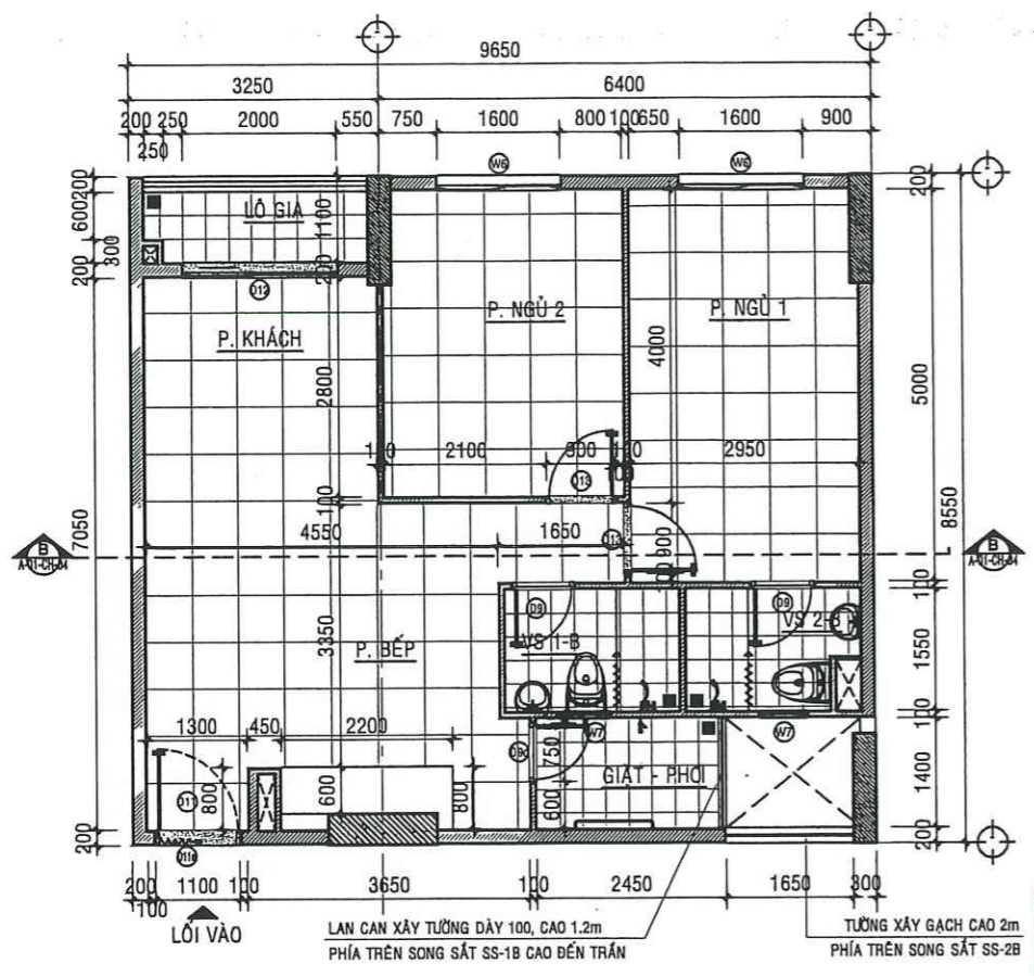
MẶT BẰNG HIỆN TRẠNG CĂN HỘ A - 13.06 - TL:1/50
