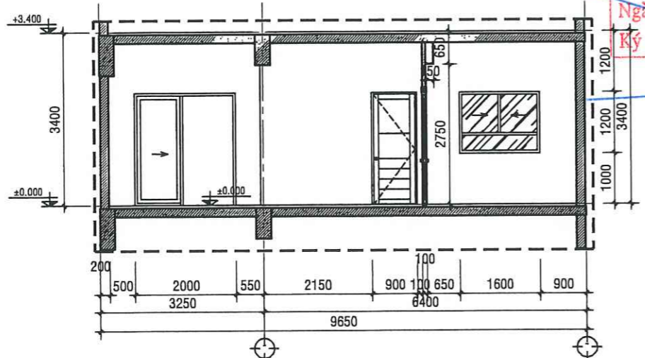
MẶT CẮT B-B - TL:1/50
