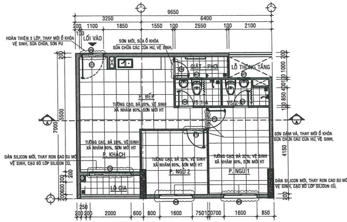
MẶT BẰNG SỬA CHỮA CĂN HỘ A - 10.08 - TL:1/50
