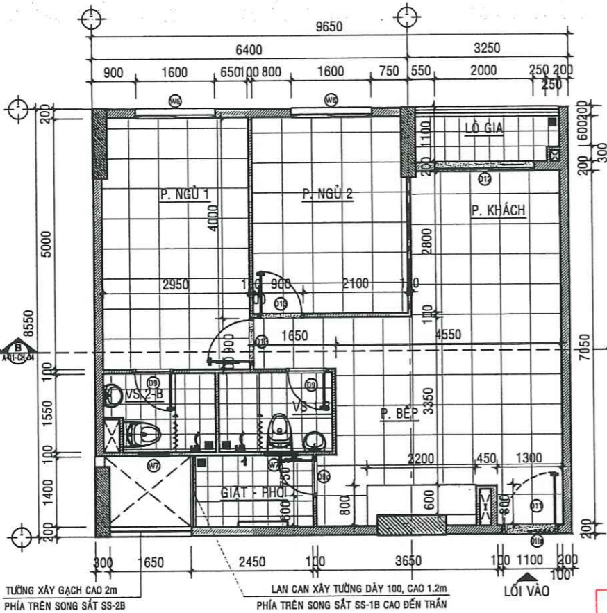
MẶT BẰNG HIỆN TRẠNG CĂN HỘ A - 13.03 - TL:1/50
