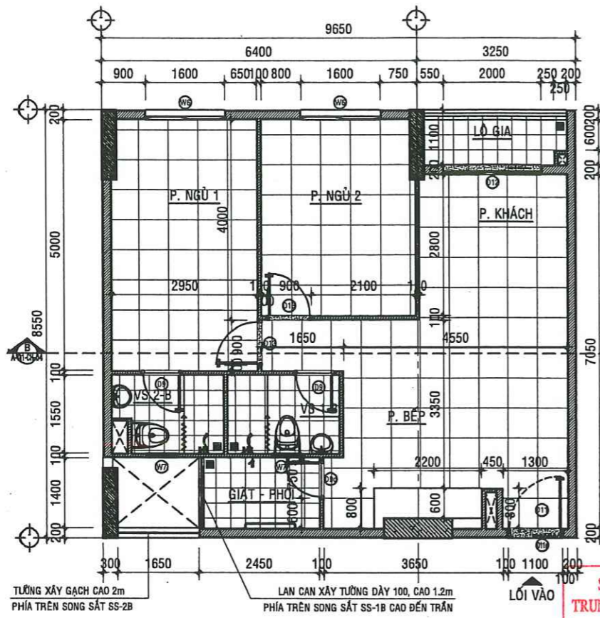
MẶT BẰNG HIỆN TRẠNG CĂN HỘ A -03.05 - TL:1/50
