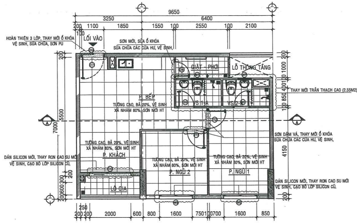
MẶT BẰNG SỬA CHỮA CĂN HỘ A - 14.01 - TL:1/50
