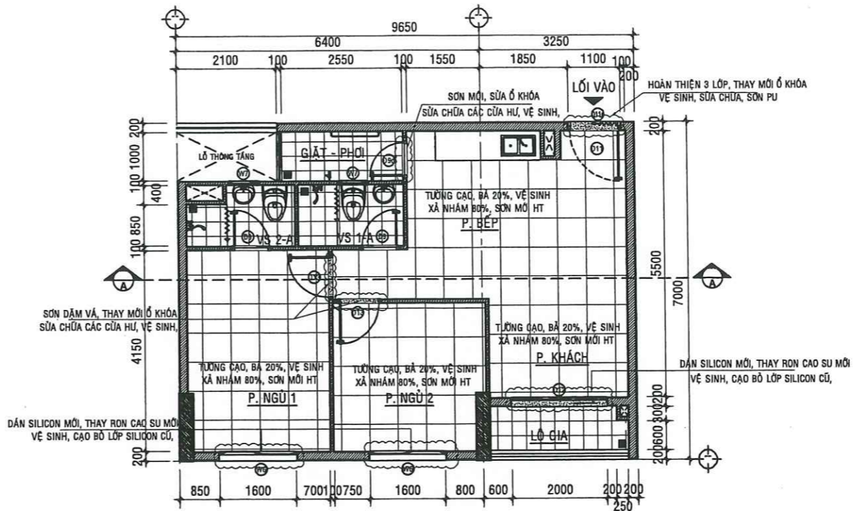
MẶT BẰNG SỬA CHỮA CĂN HỘ A - 09.09 - TL:1/50
