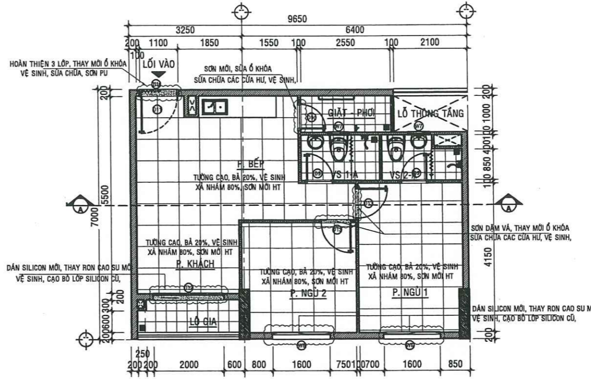
MẶT BẰNG SỬA CHỮA CĂN HỘ A - 08.08 - TL:1/50
