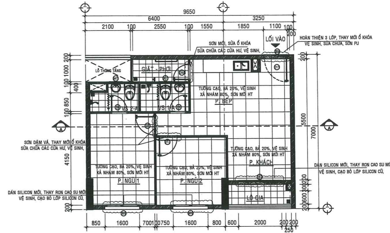
MẶT BẰNG SỬA CHỮA CĂN HỘ A - 12.09 - TL:1/50
