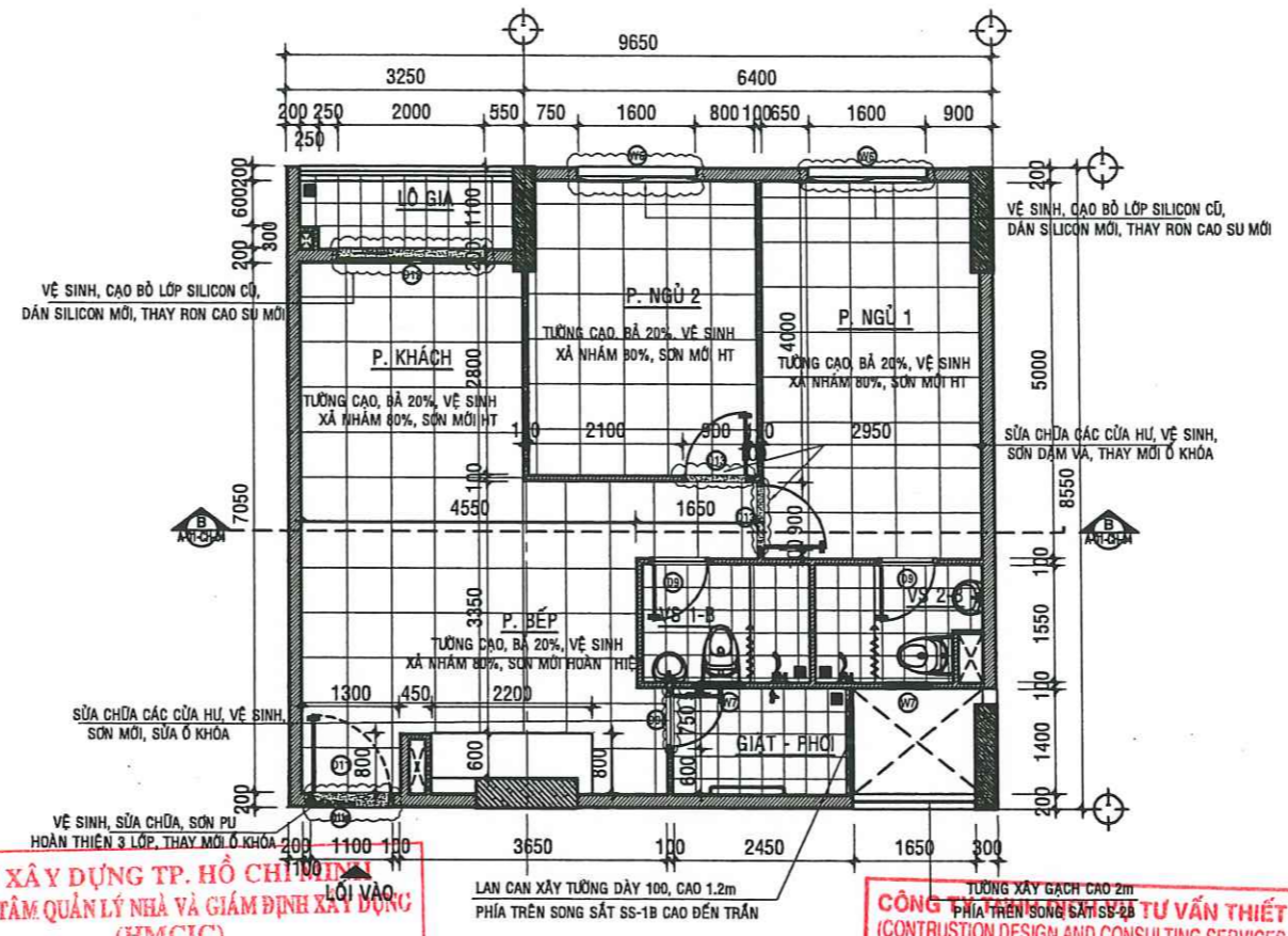
MẶT BẰNG SỬA CHỮA CĂN HỘ A -03.04 - TL:1/50
