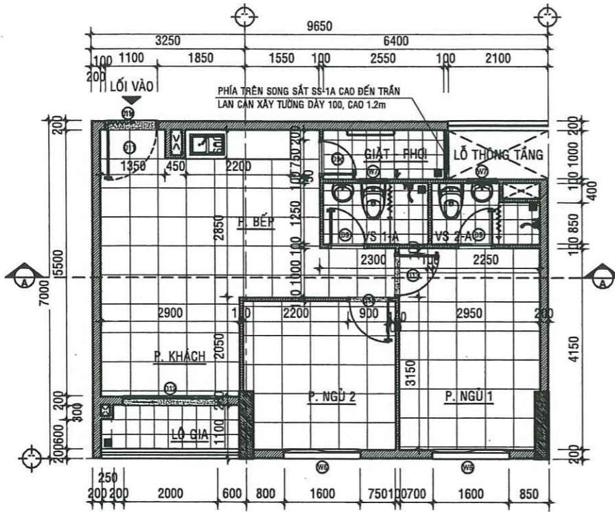
MẶT BẰNG HIỆN TRẠNG CĂN HỘ A -02.08 - TL:1/50
