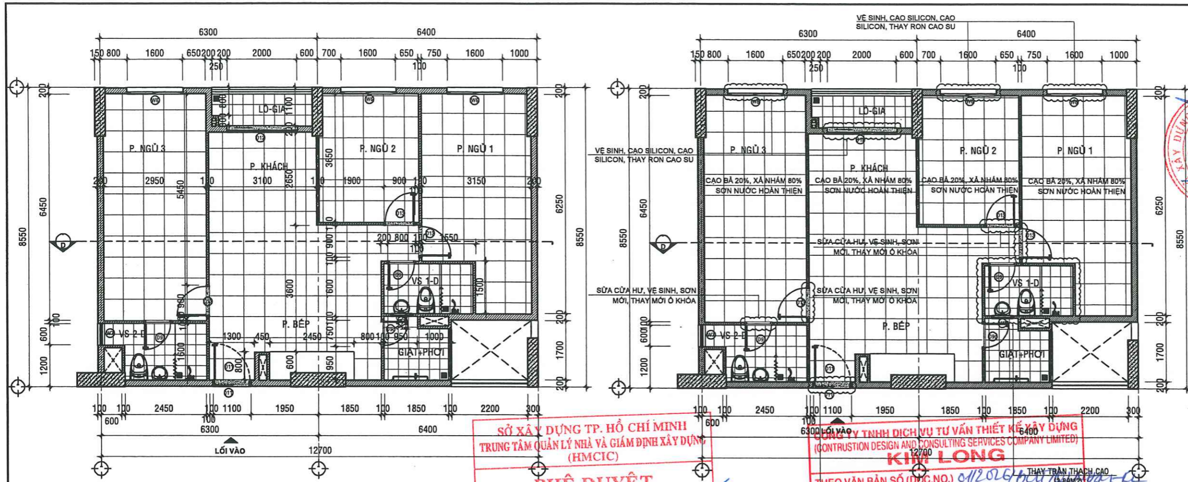
MẶT BẰNG HIỆN TRẠNG CĂN HỘ A -02.07 - TL: 1/50
