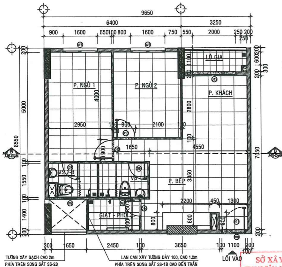
MẶT BẰNG HIỆN TRẠNG CĂN HỘ A - 08.03 - TL:1/50
