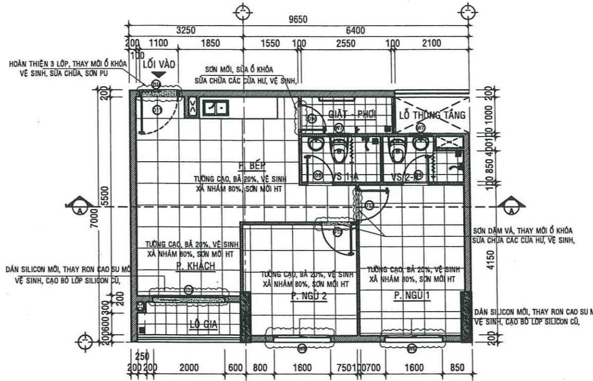
MẶT BẰNG SỬA CHỮA CĂN HỘ A - 07.08 - TL:1/50
