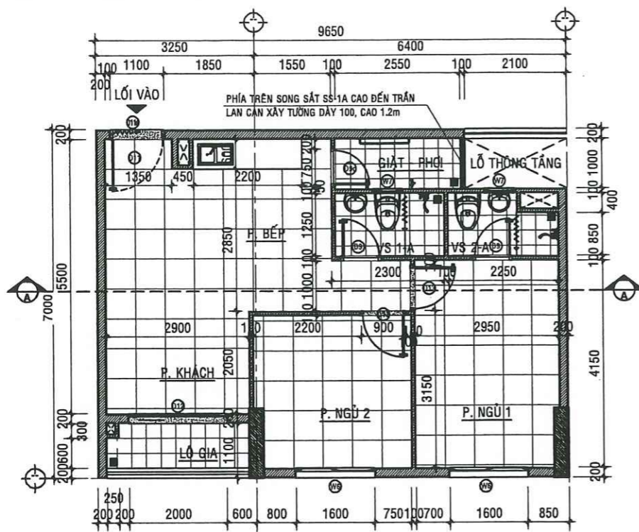
MẶT BẰNG HIỆN TRẠNG CĂN HỘ A - 10.08 - TL:1/50
