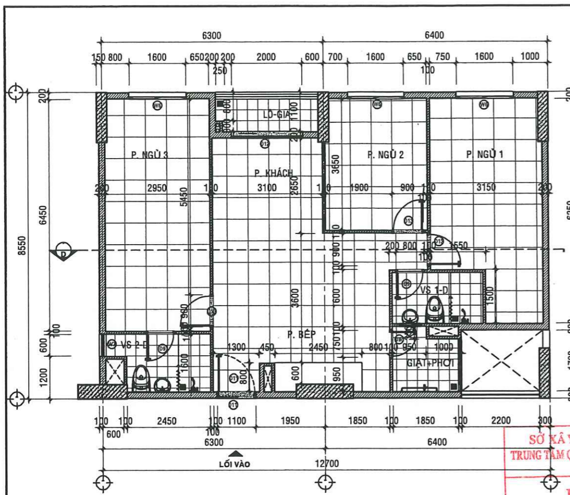
MẶT BẰNG HIỆN TRẠNG CĂN HỘ A - 08.07 - TL: 1/50
