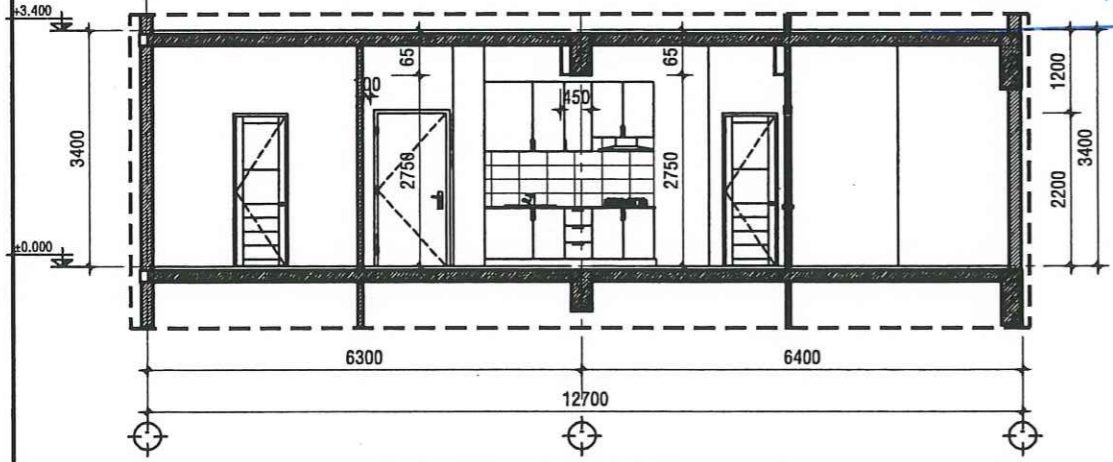
MẶT CẮT D-D - TL: 1/50
