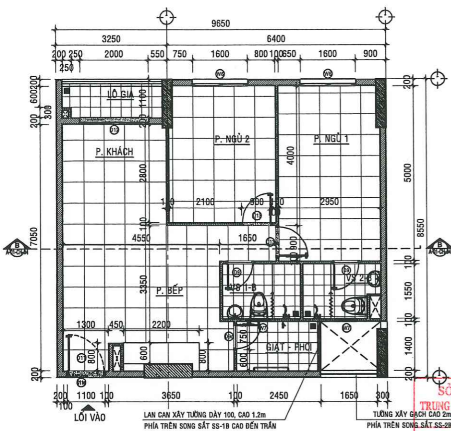
MẶT BẰNG HIỆN TRẠNG CĂN HỘ A - 09.06 - TL:1/50
