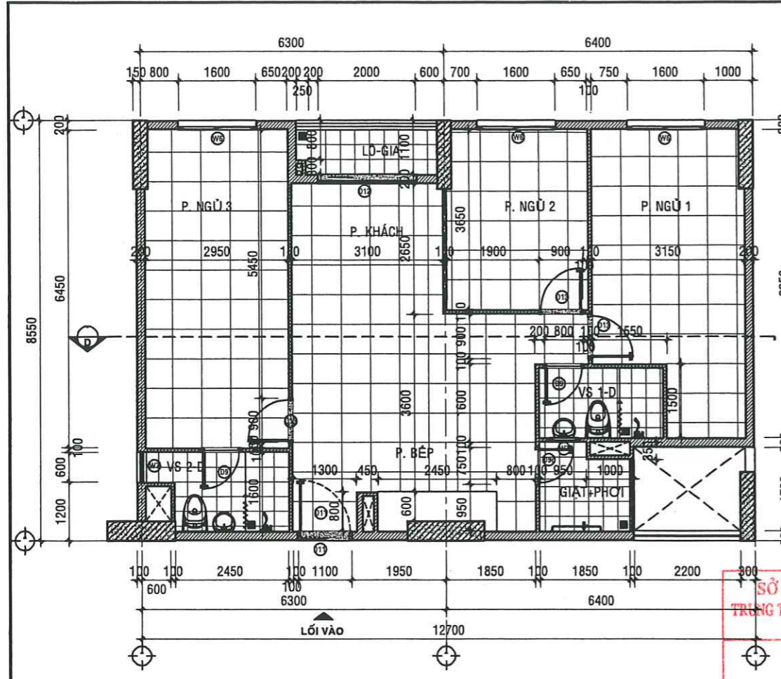
MẶT BẰNG HIỆN TRẠNG CĂN HỘ A - 10.07 - TL: 1/50
