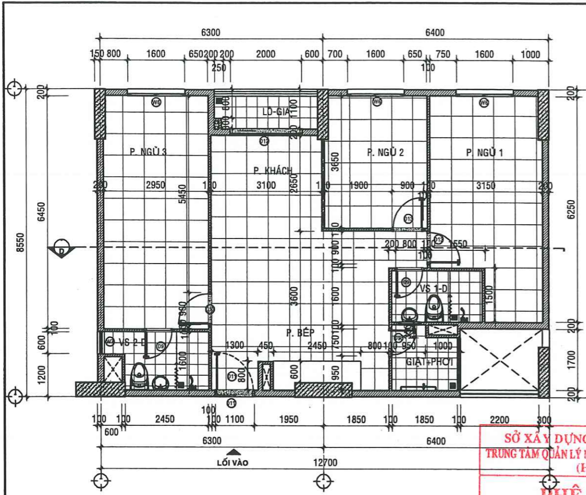
MẶT BẰNG HIỆN TRẠNG CĂN HỘ A -01.03 - TL: 1/50
