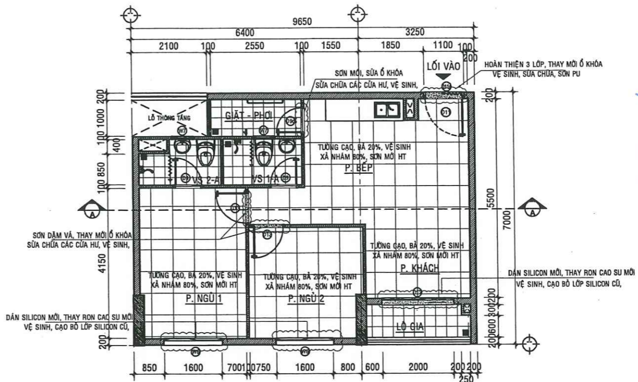
MẶT BẰNG SỬA CHỮA CĂN HỘ A - 12.02 - TL:1/50
