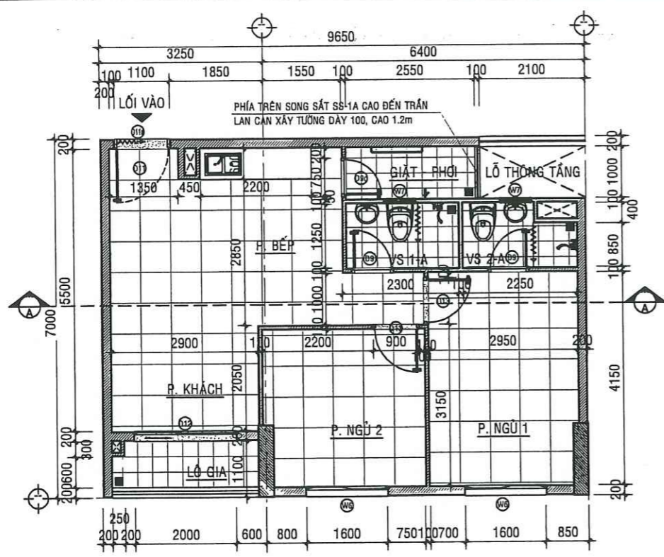
MẶT BẰNG HIỆN TRẠNG CĂN HỘ A - 14.08 - TL:1/50
