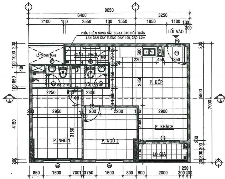
MẶT BẰNG HIỆN TRẠNG CĂN HỘ A -01.05 - TL:1/50
