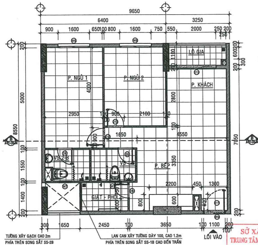
MẶT BẰNG HIỆN TRẠNG CĂN HỘ A - 10.05 - TL:1/50
