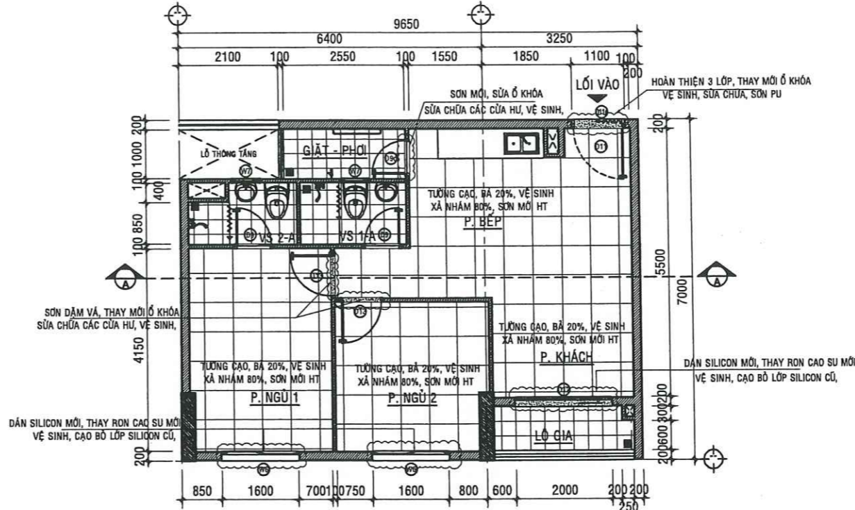
MẶT BẰNG SỬA CHỮA CĂN HỘ A - 10.02 - TL:1/50
