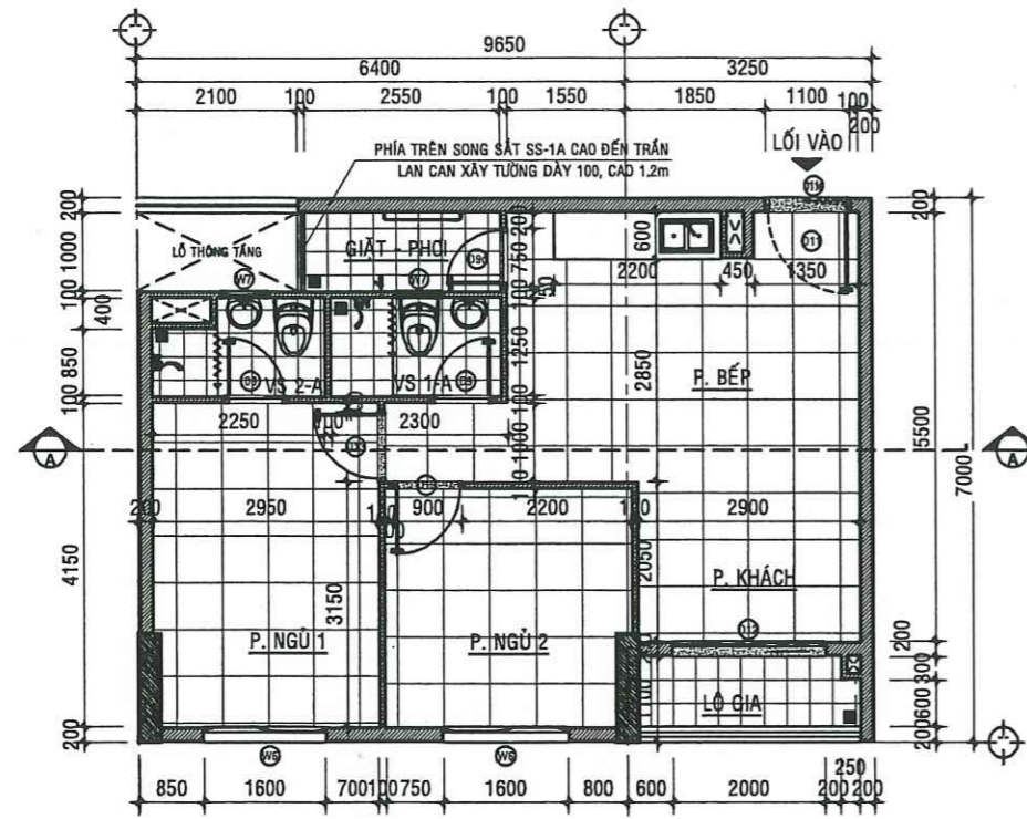
MẶT BẰNG HIỆN TRẠNG CĂN HỘ A -02.02 - TL:1/50
