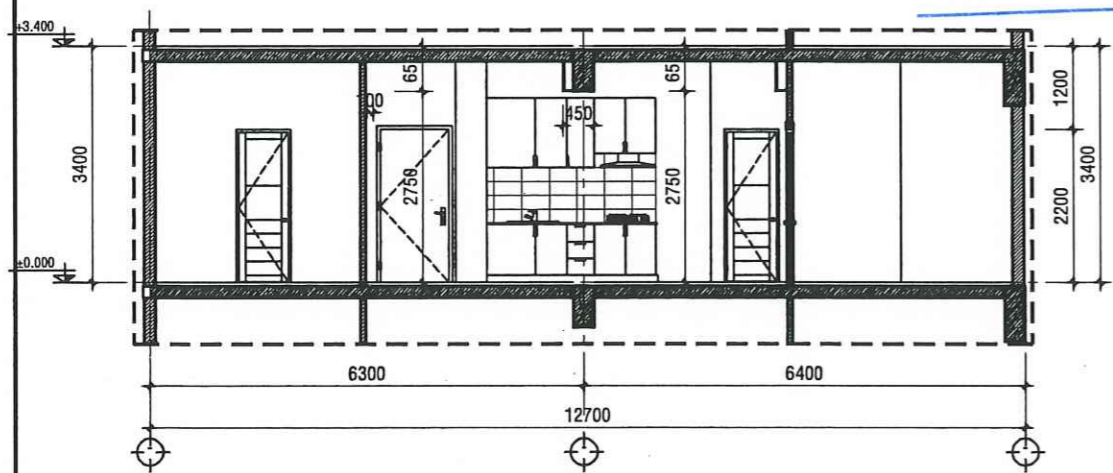
MẶT CẮT D-D - TL: 1/50
