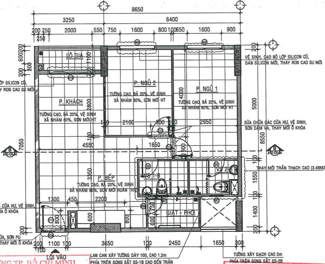
MẶT BẰNG SỬA CHỮA CĂN HỘ A - 14.04 - TL:1/50
