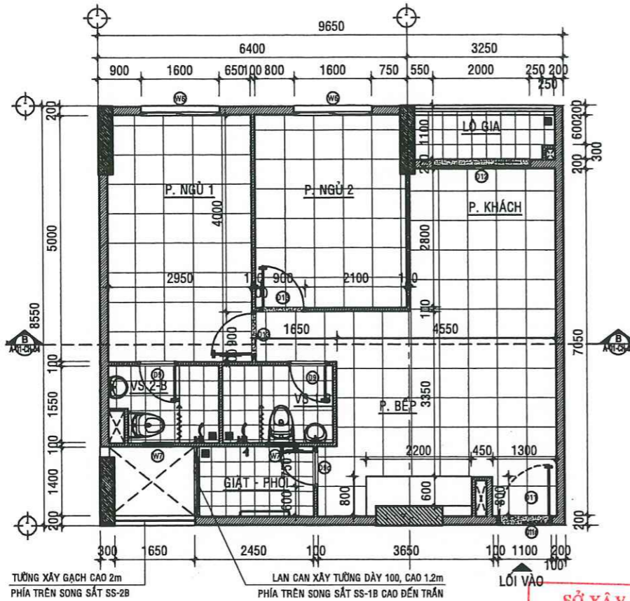
MẶT BẰNG HIỆN TRẠNG CĂN HỘ A -04.05 - TL:1/50
