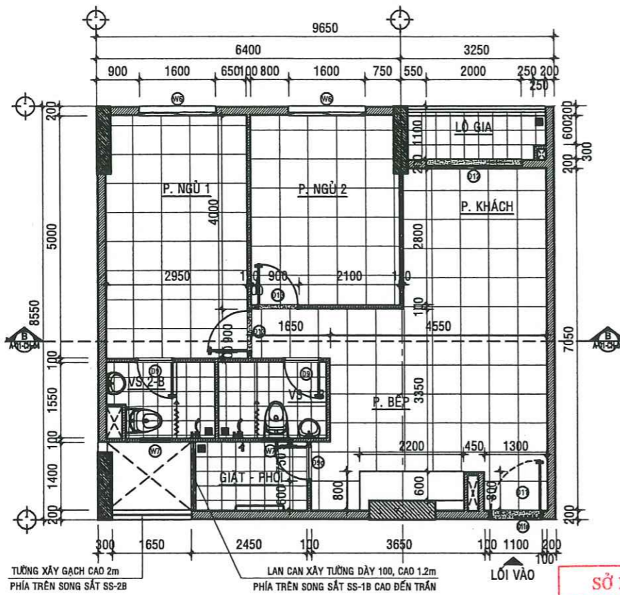
MẶT BẰNG HIỆN TRẠNG CĂN HỘ A - 06.03 - TL:1/50
