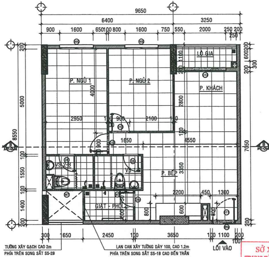
MẶT BẰNG HIỆN TRẠNG CĂN HỘ A - 06.05 - TL:1/50
