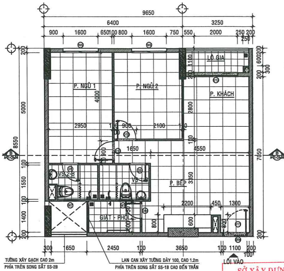
MẶT BẰNG HIỆN TRẠNG CĂN HỘ A -03.03 - TL:1/50
