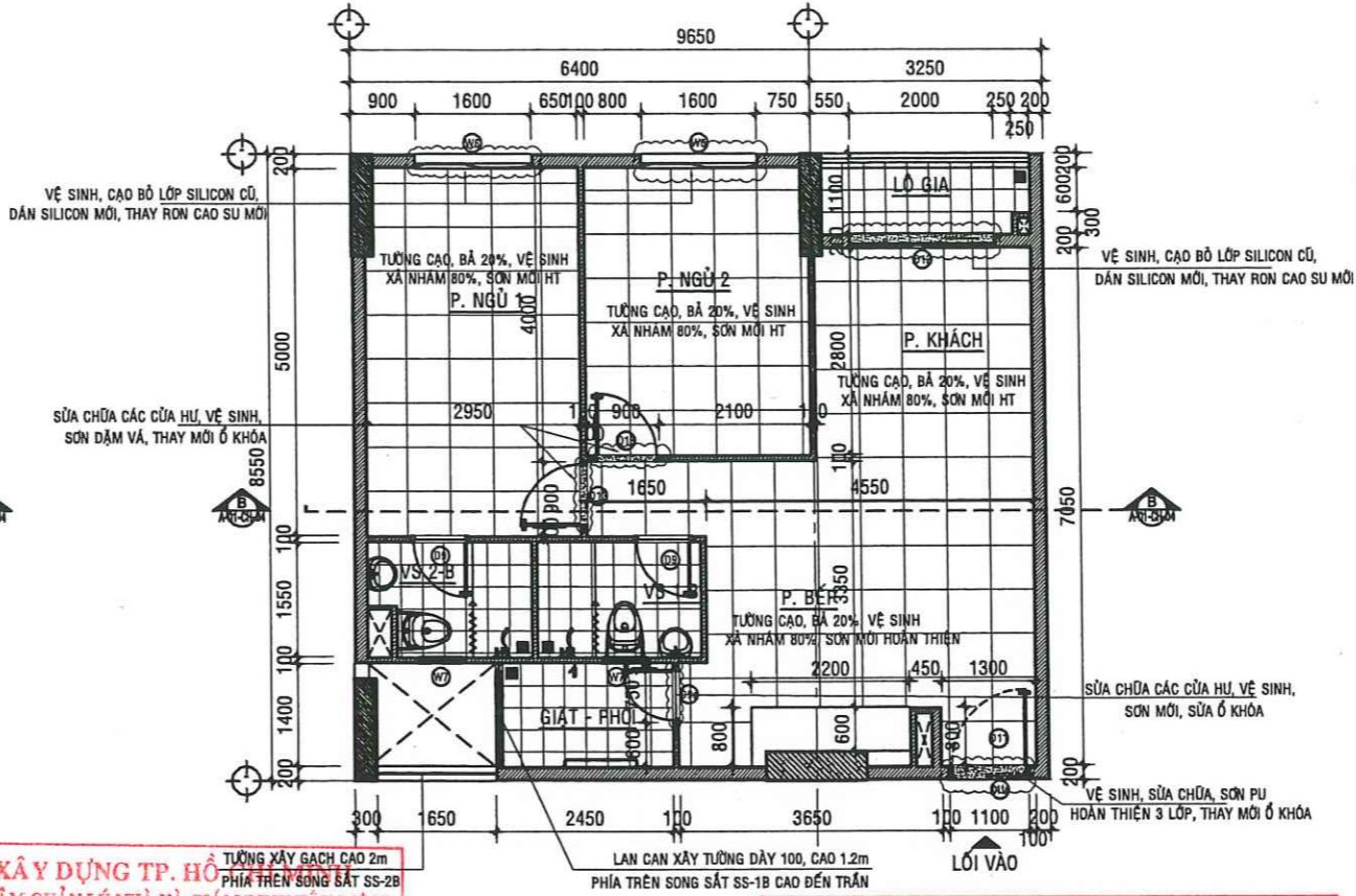
MẶT BẰNG SỬA CHỮA CĂN HỘ A - 06.05 - TL:1/50
