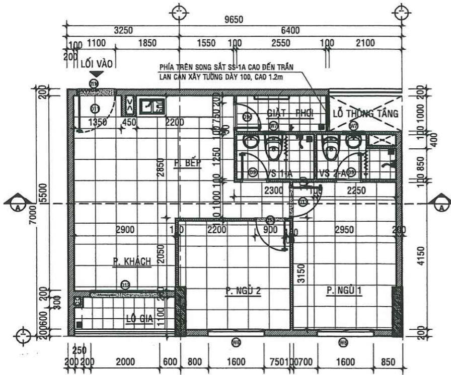
MẶT BẰNG HIỆN TRẠNG CĂN HỘ A -03.01 - TL:1/50
