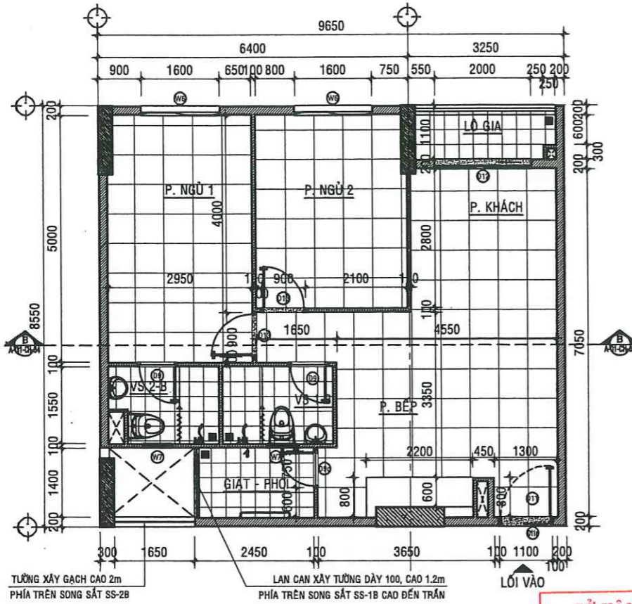
MẶT BẰNG HIỆN TRẠNG CĂN HỘ A - 05.03 - TL:1/50
