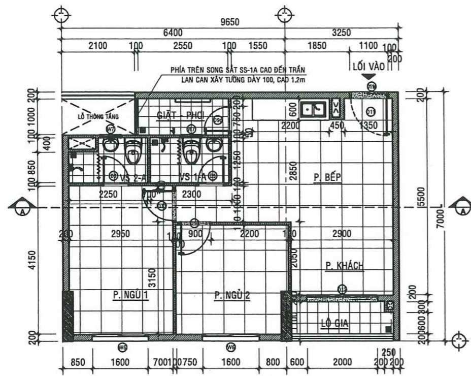
MẶT BẰNG HIỆN TRẠNG CĂN HỘ A - 08.09 - TL:1/50
