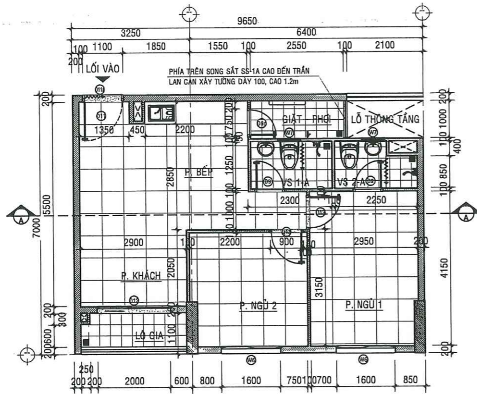
MẶT BẰNG HIỆN TRẠNG CĂN HỘ A - 15.04 - TL:1/50
