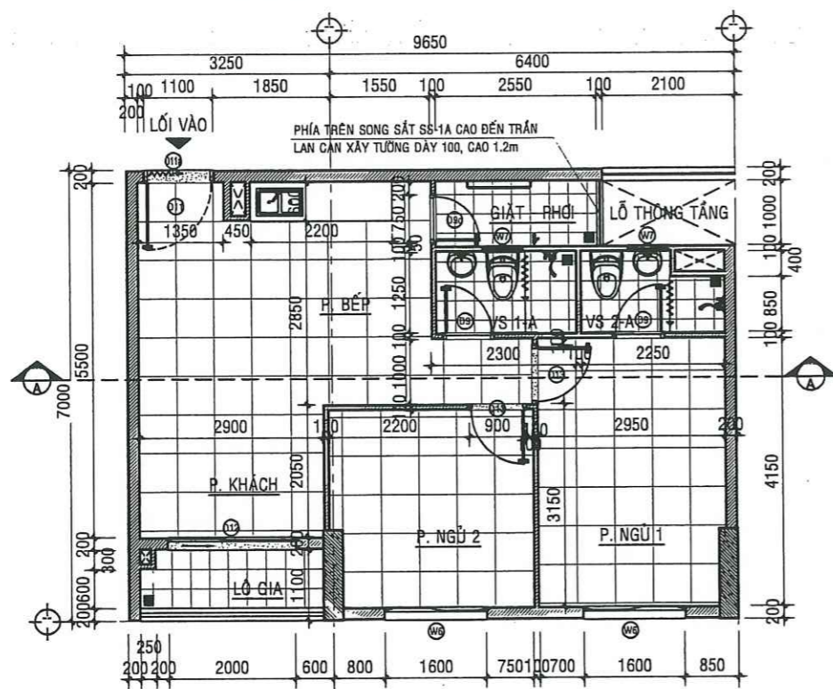
MẶT BẰNG HIỆN TRẠNG CĂN HỘ A - 13.08 - TL:1/50
