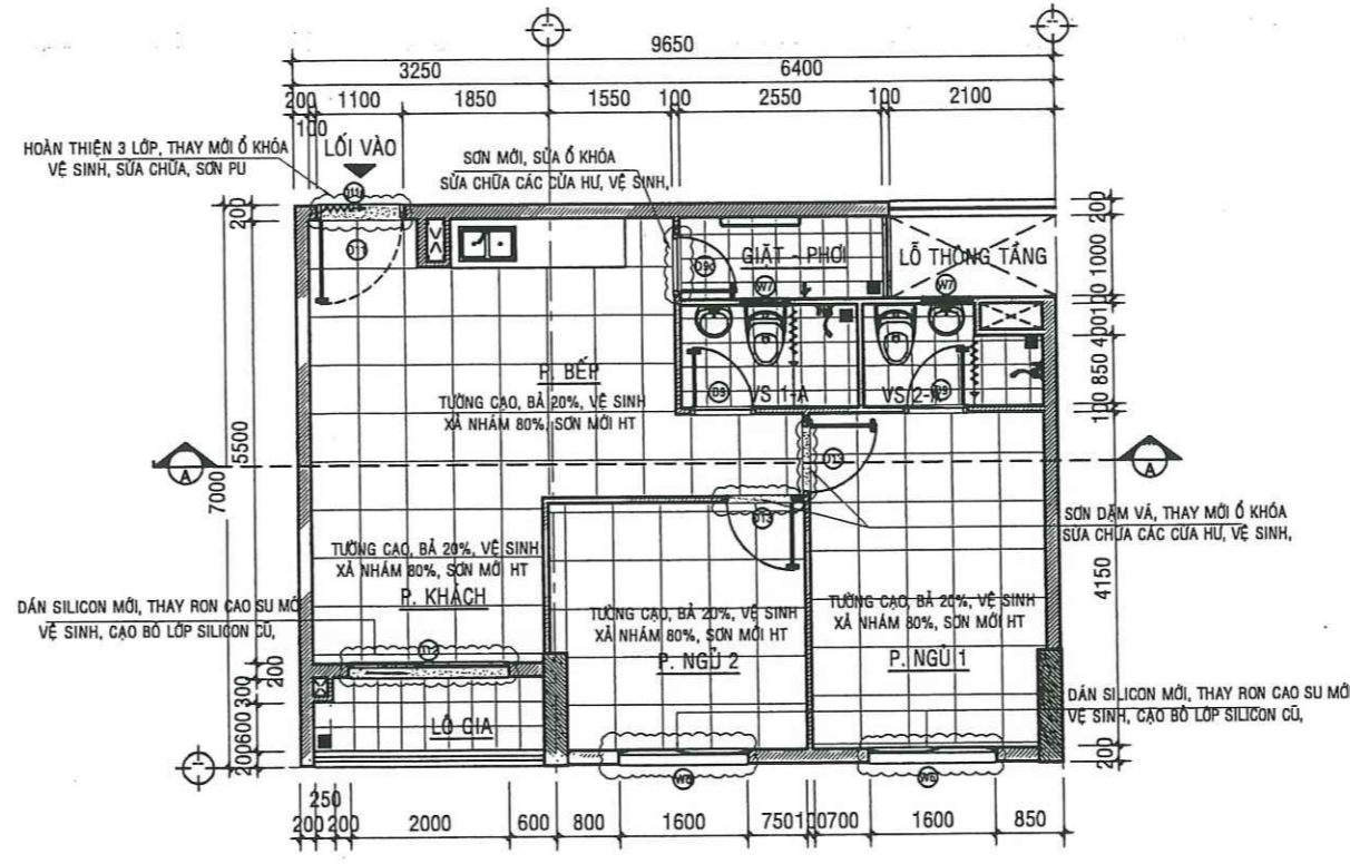
MẶT BẰNG SỬA CHỮA CĂN HỘ A - 13.01 - TL:1/50
