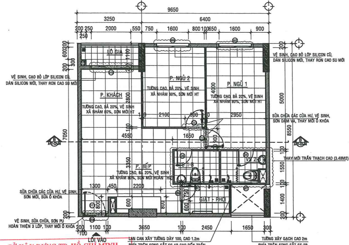
MẶT BẰNG SỬA CHỮA CĂN HỘ A -02.06 - TL:1/50
