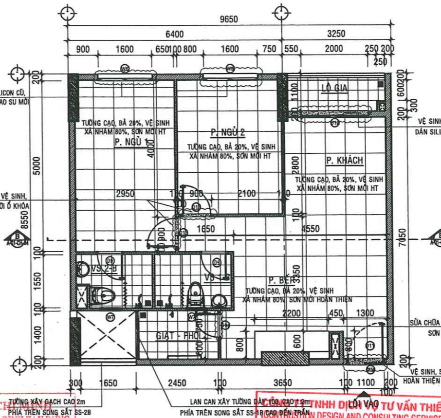
MẶT BẰNG SỬA CHỮA CĂN HỘ A - 08.03 - TL:1/50
