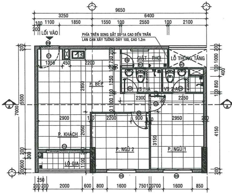
MẶT BẰNG HIỆN TRẠNG CĂN HỘ A -04.08 - TL:1/50
