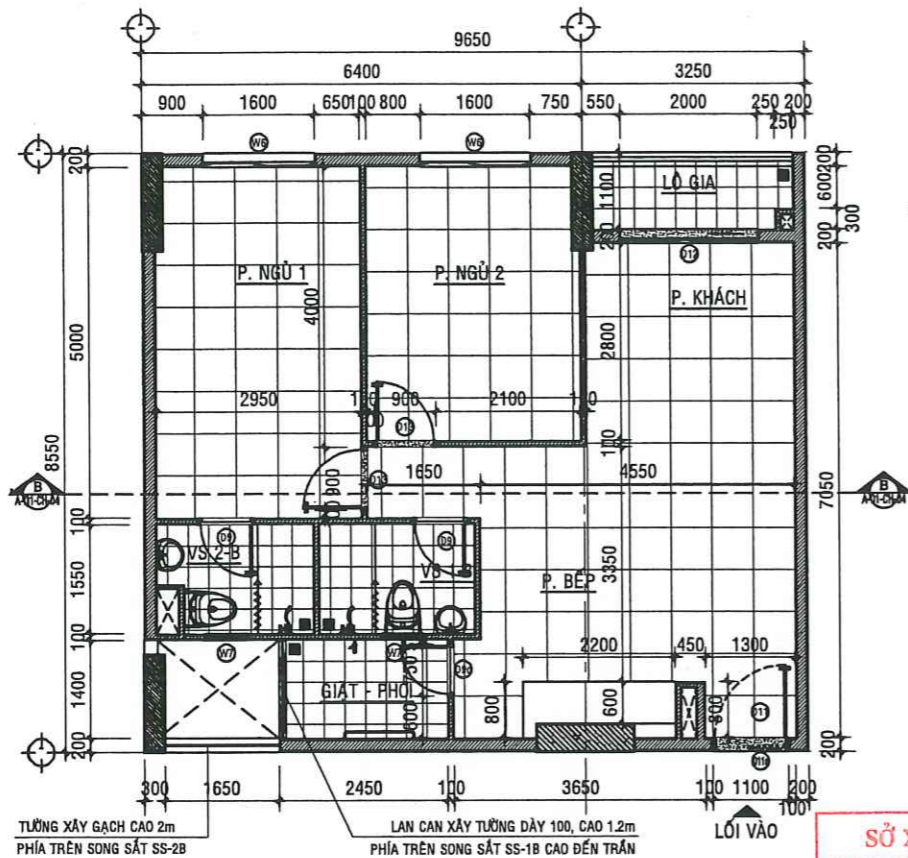
MẶT BẰNG HIỆN TRẠNG CĂN HỘ A - 09.03 - TL:1/50
