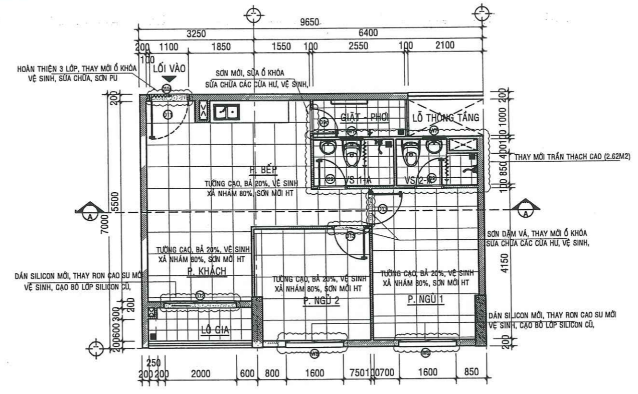
MẶT BẰNG SỬA CHỮA CĂN HỘ A - 14.08 - TL:1/50
