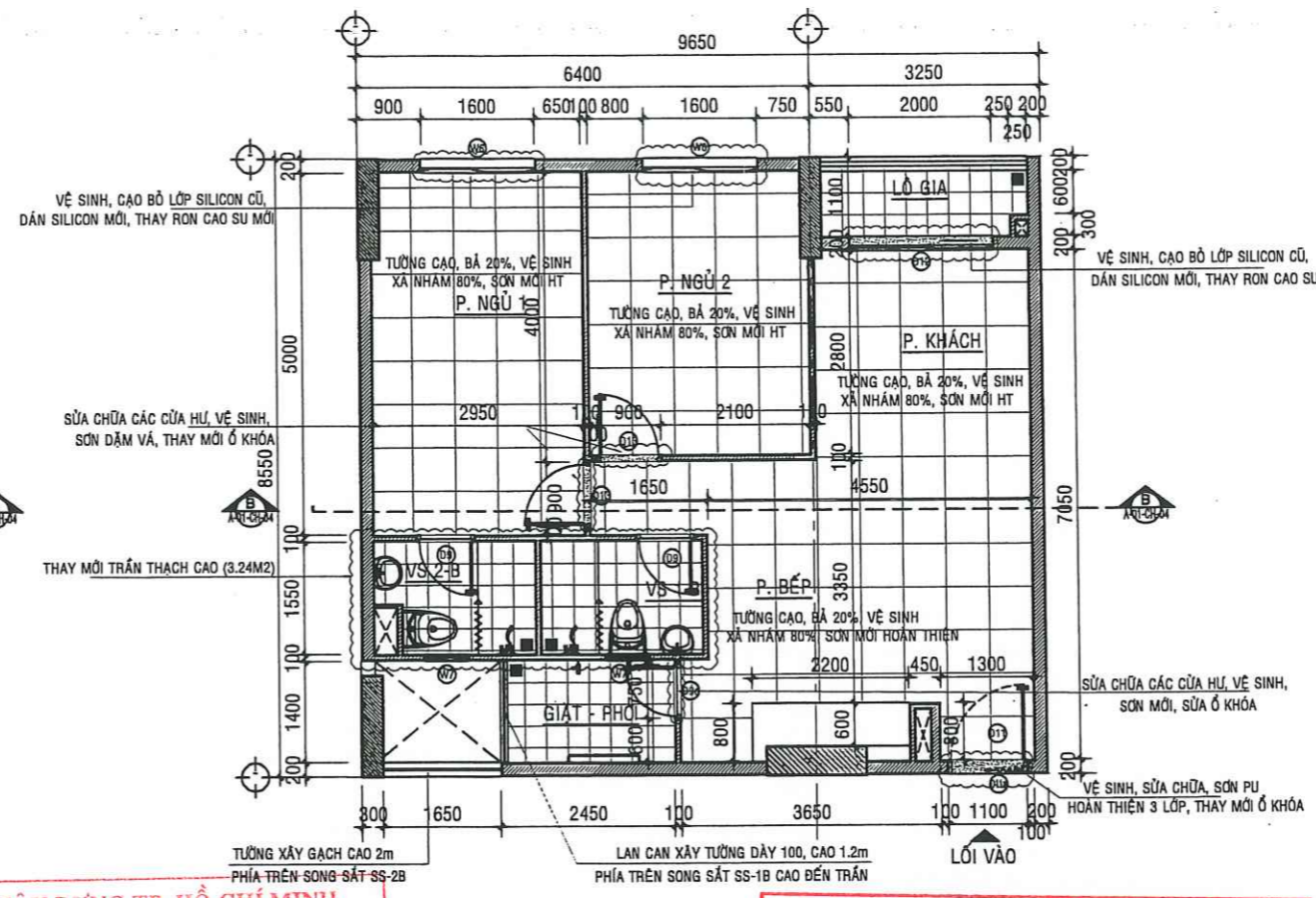
MẶT BẰNG SỬA CHỮA CĂN HỘ A - 14.03 - TL:1/50
