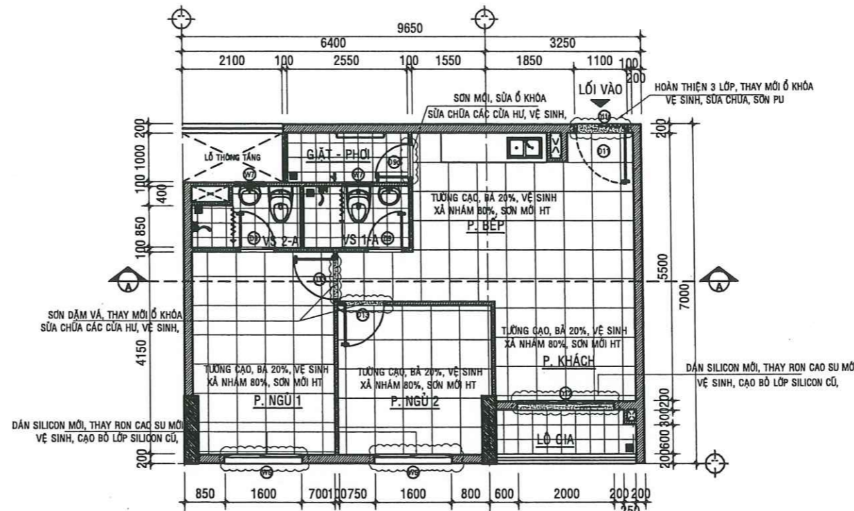
MẶT BẰNG SỬA CHỮA CĂN HỘ A - 07.09 - TL:1/50
