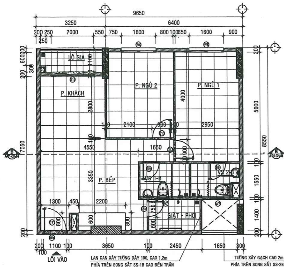
MẶT BẰNG HIỆN TRẠNG CĂN HỘ A - 05.06 - TL:1/50
