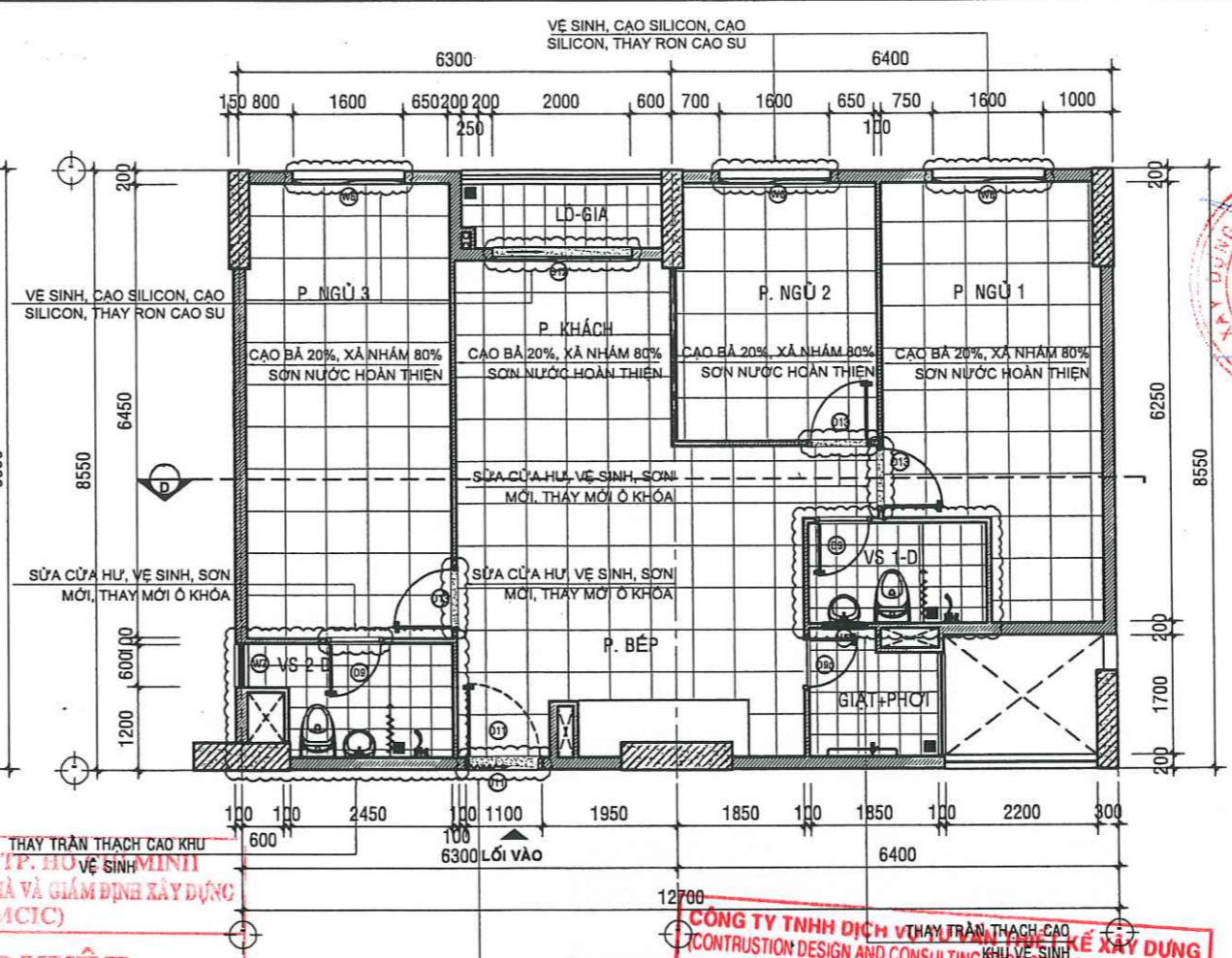
MẶT BẰNG SỬA CHỮA CĂN HỘ A - 15.03 - TL: 1/50
