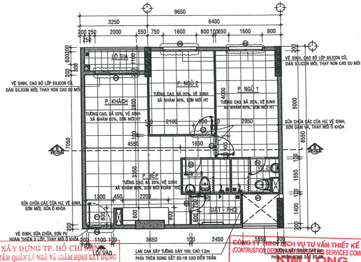
MẶT BẰNG SỬA CHỮA CĂN HỘ A - 08.06 - TL:1/50
