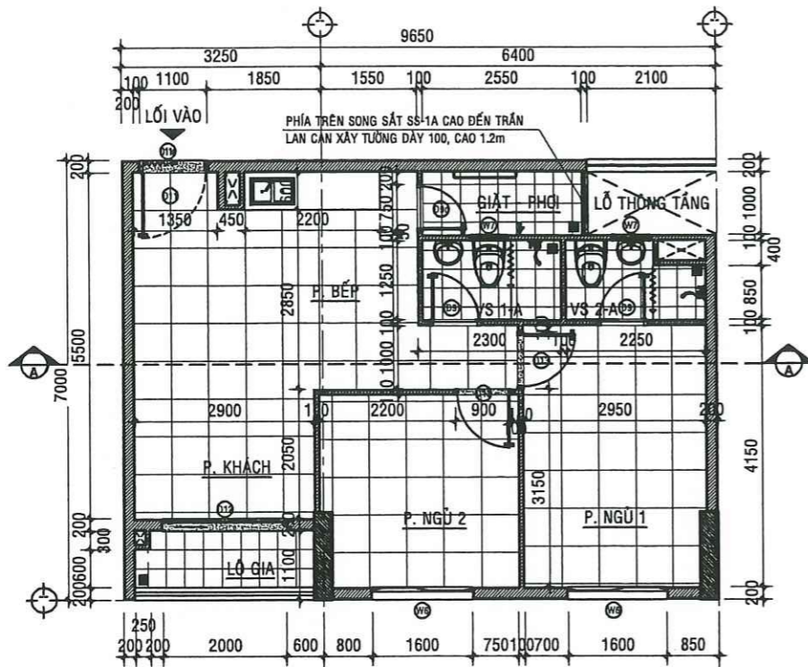
MẶT BẰNG HIỆN TRẠNG CĂN HỘ A - 08.01 - TL:1/50
