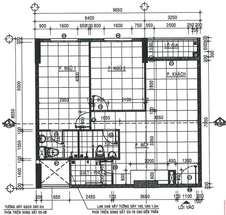
MẶT BẰNG HIỆN TRẠNG CĂN HỘ A - 12.05 - TL:1/50
