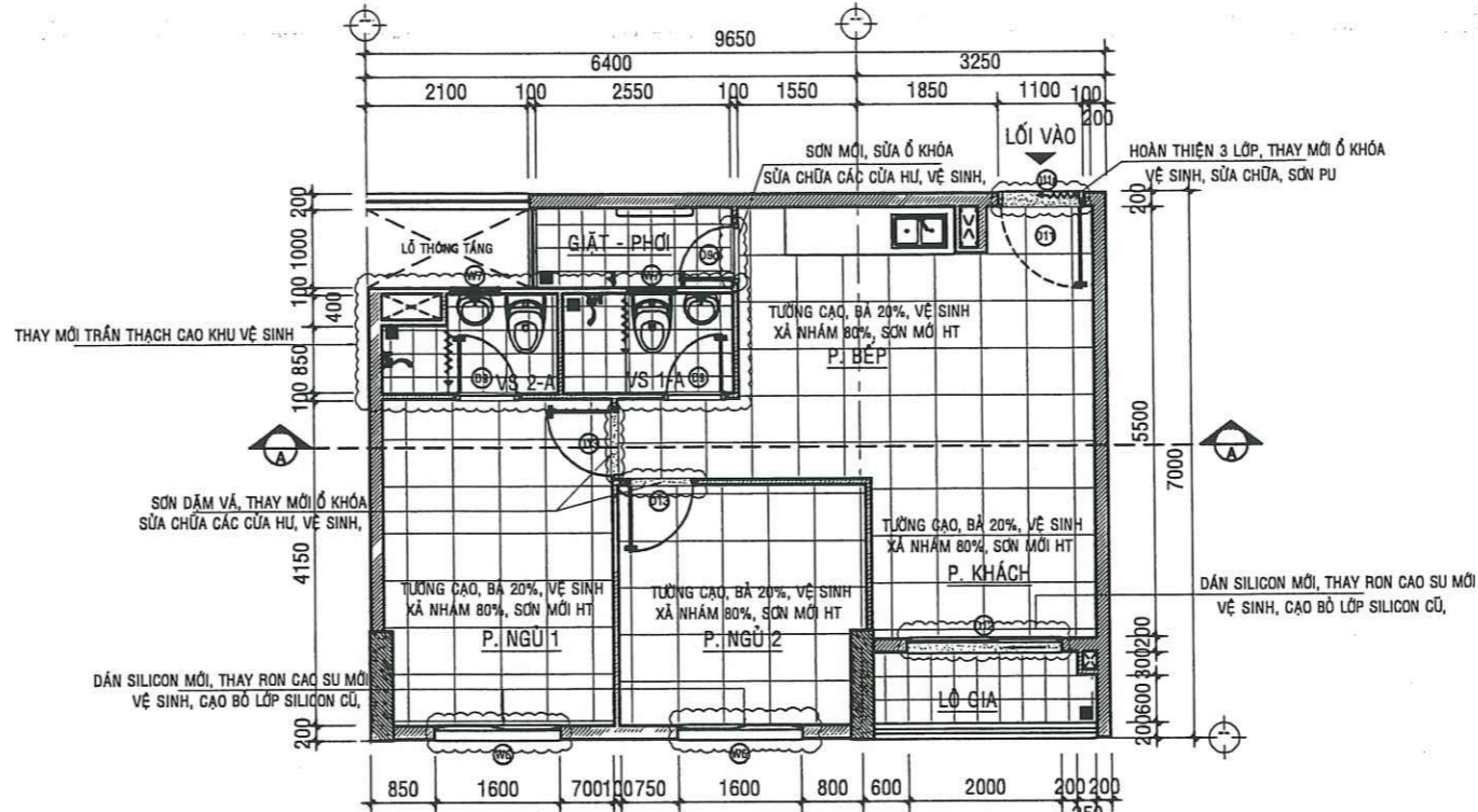
MẶT BẰNG SỬA CHỮA CĂN HỘ A - 15.05 - TL:1/50
