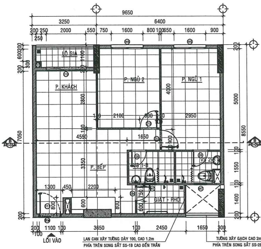
MẶT BẰNG HIỆN TRẠNG CĂN HỘ A - 12.04 - TL:1/50
