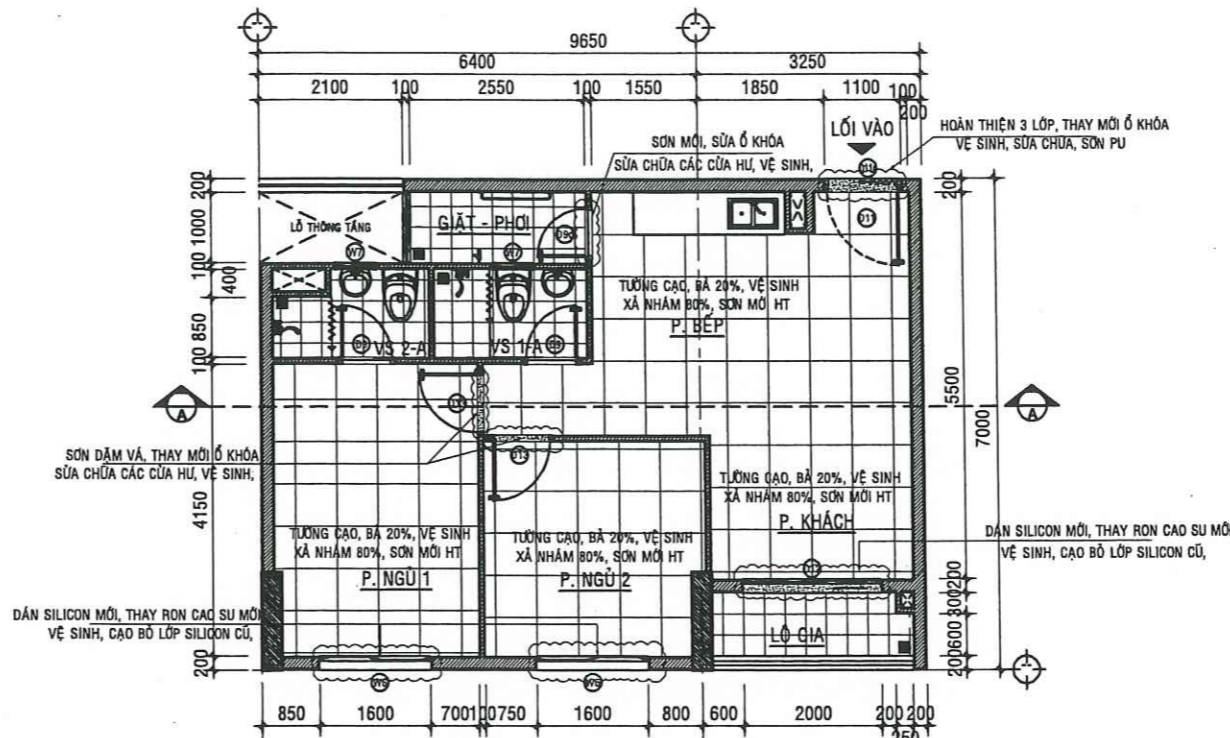
MẶT BẰNG SỬA CHỮA CĂN HỘ A -03.09 - TL:1/50
