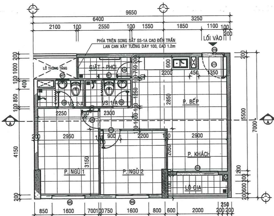
MẶT BẰNG HIỆN TRẠNG CĂN HỘ A - 14.09 - TL:1/50
