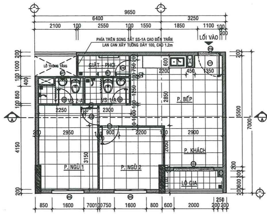
MẶT BẰNG HIỆN TRẠNG CĂN HỘ A - 05.02 - TL:1/50
