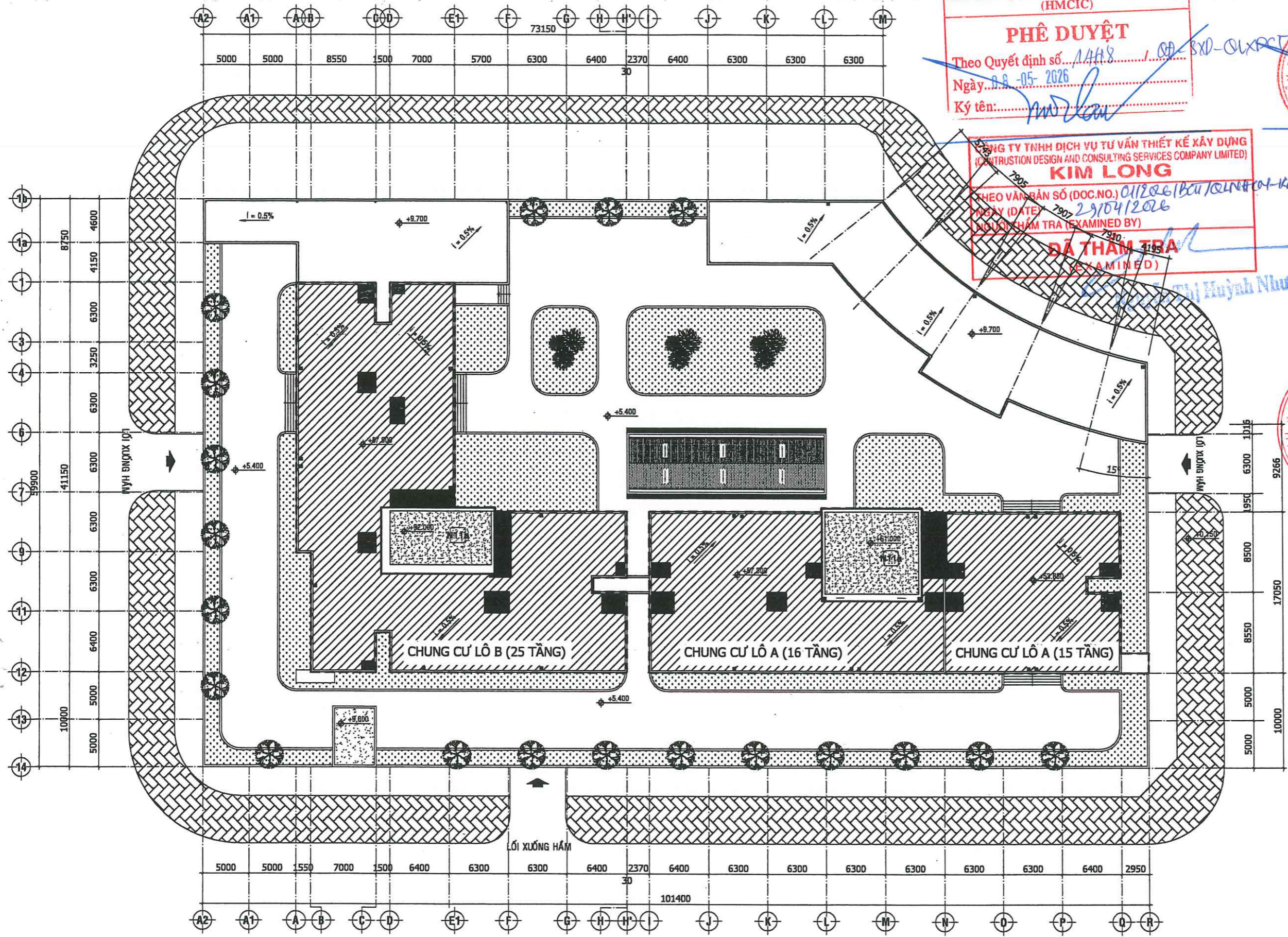
MẶT BẰNG TỔNG THỂ TẦNG MÁI - TL: 1/400
