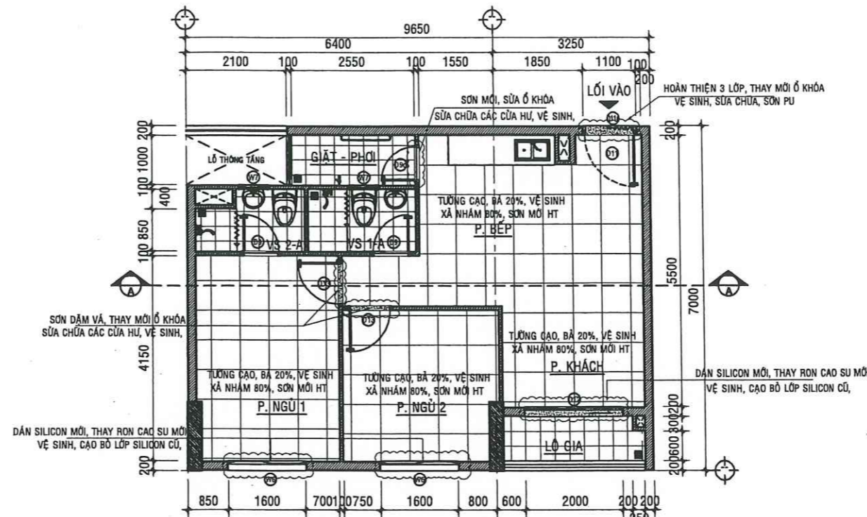
MẶT BẰNG SỬA CHỮA CĂN HỘ A - 06.02 - TL:1/50
