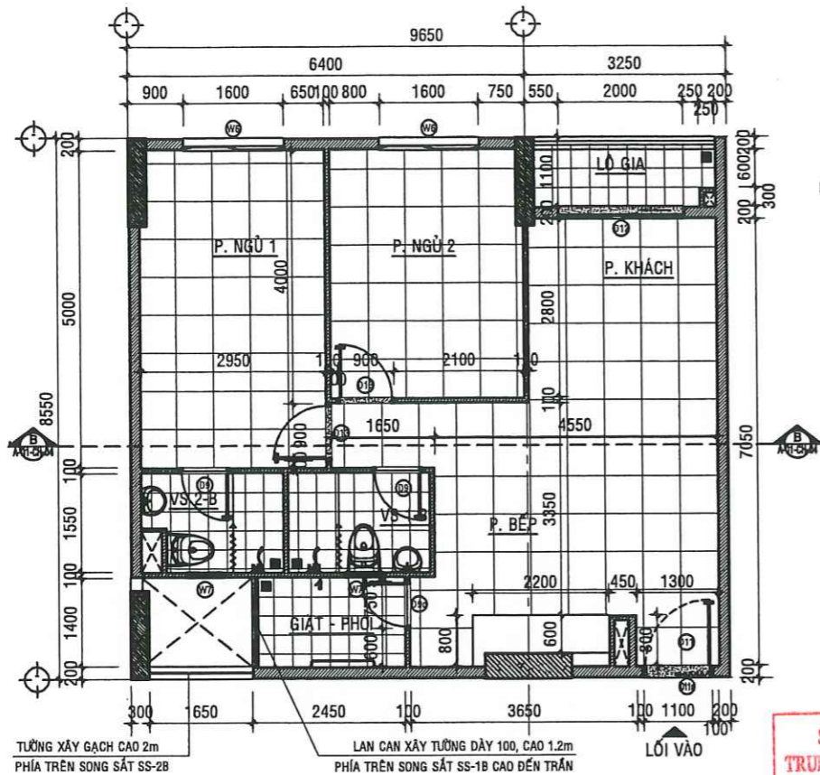
MẶT BẰNG HIỆN TRẠNG CĂN HỘ A - 11.03 - TL:1/50
