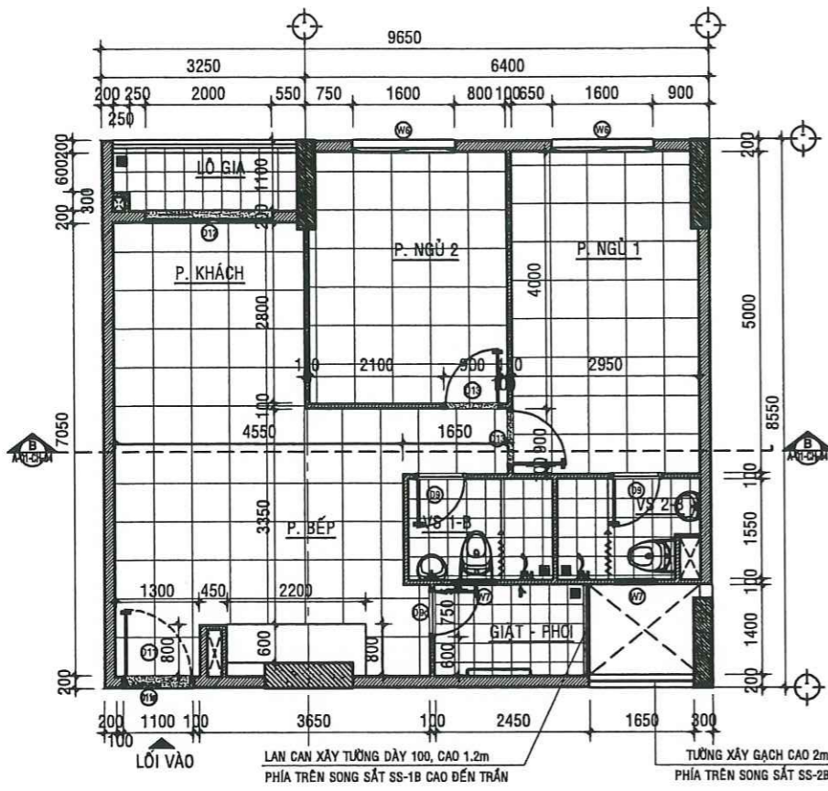
MẶT BẰNG HIỆN TRẠNG CĂN HỘ A - 12.06 - TL:1/50
