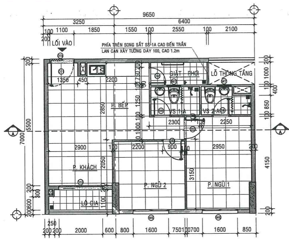
MẶT BẰNG HIỆN TRẠNG CĂN HỘ A - 13.01 - TL:1/50
