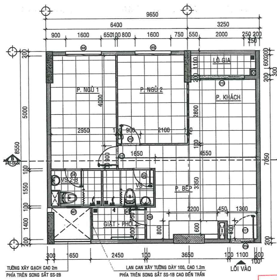
MẶT BẰNG HIỆN TRẠNG CĂN HỘ A - 14.03 - TL:1/50
