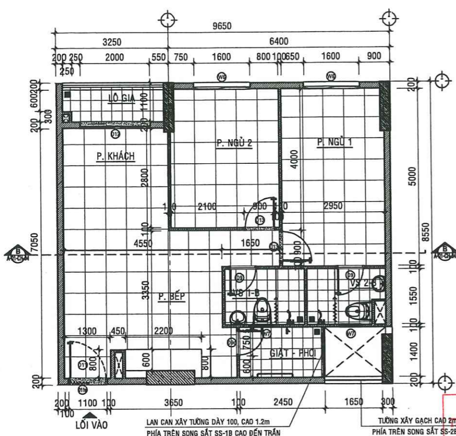
MẶT BẰNG HIỆN TRẠNG CĂN HỘ A - 10.04 - TL:1/50
