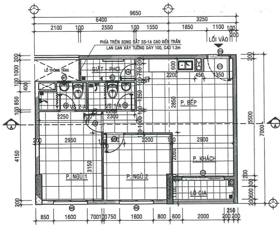
MẶT BẰNG HIỆN TRẠNG CĂN HỘ A - 14.02 - TL:1/50
