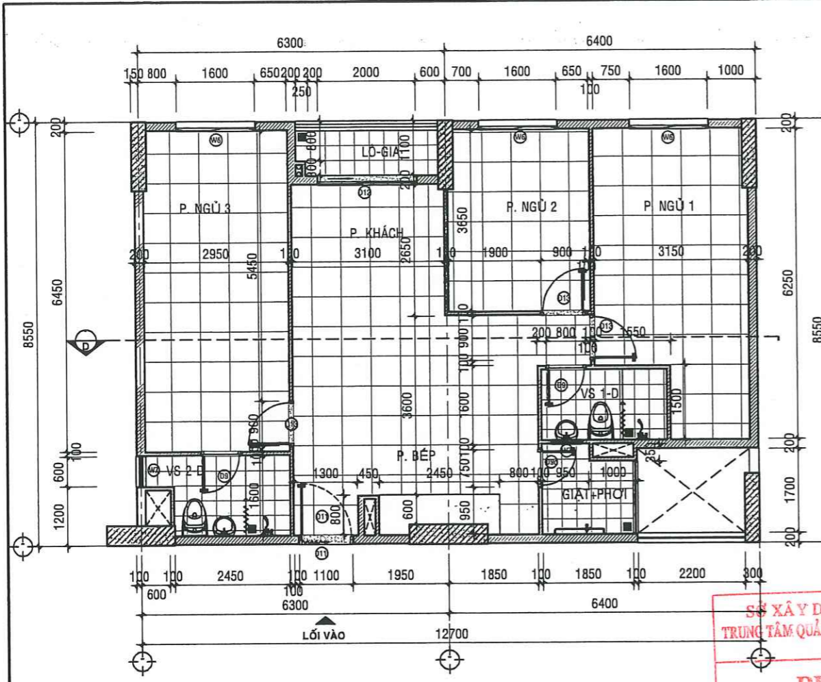
MẶT BẰNG HIỆN TRẠNG CĂN HỘ A - 14.07 - TL: 1/50
