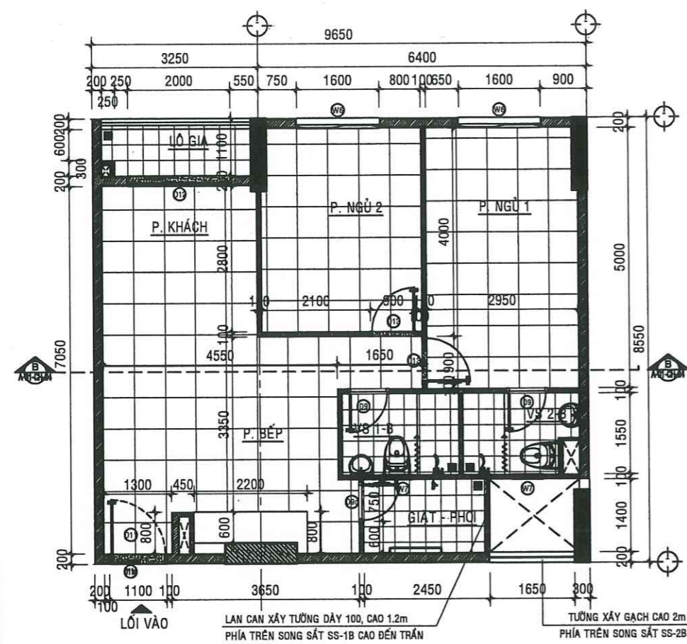
MẶT BẰNG HIỆN TRẠNG CĂN HỘ A - 11.06 - TL:1/50
