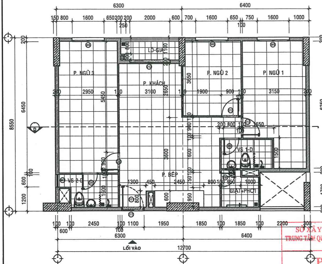
MẶT BẰNG HIỆN TRẠNG CĂN HỘ A - 06.07 - TL: 1/50
