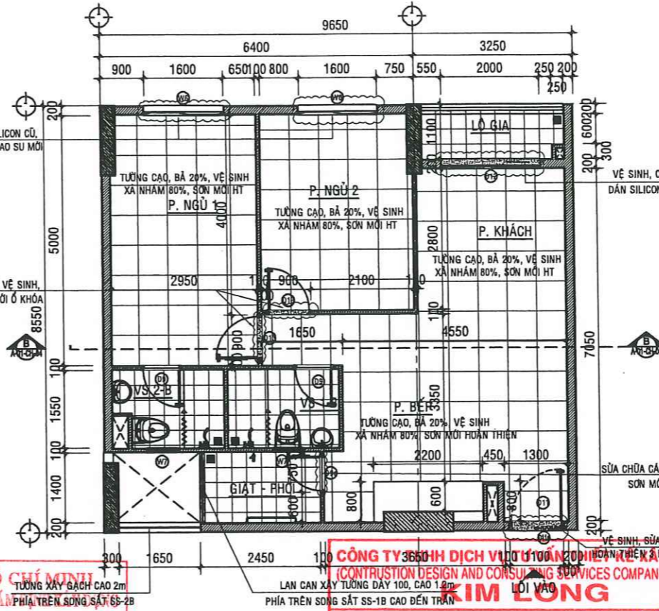
MẶT BẰNG SỬA CHỮA CĂN HỘ A - 10.05 - TL:1/50
