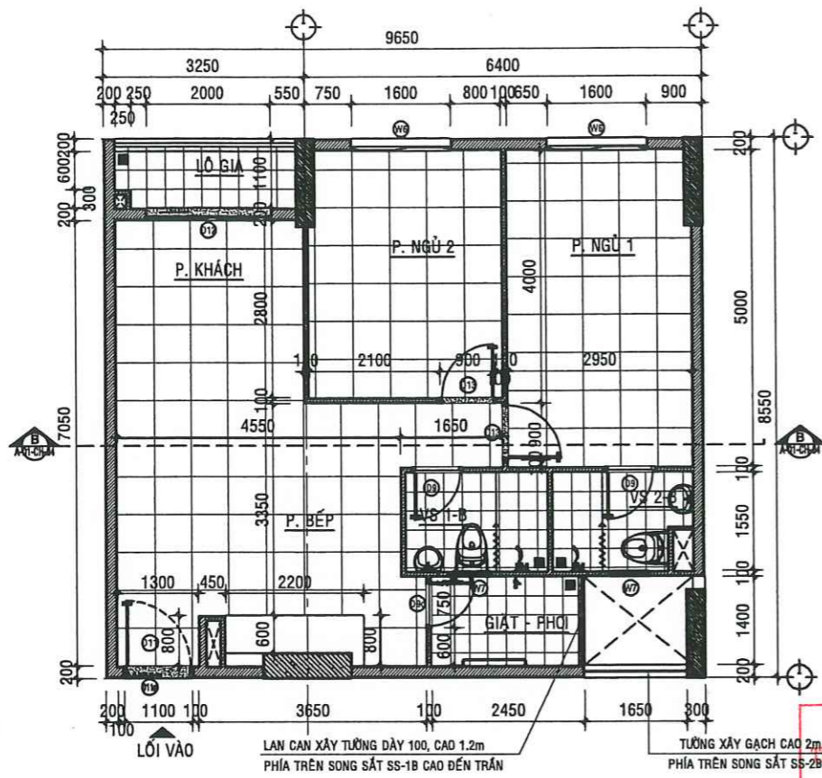
MẶT BẰNG HIỆN TRẠNG CĂN HỘ A - 08.04 - TL:1/50
