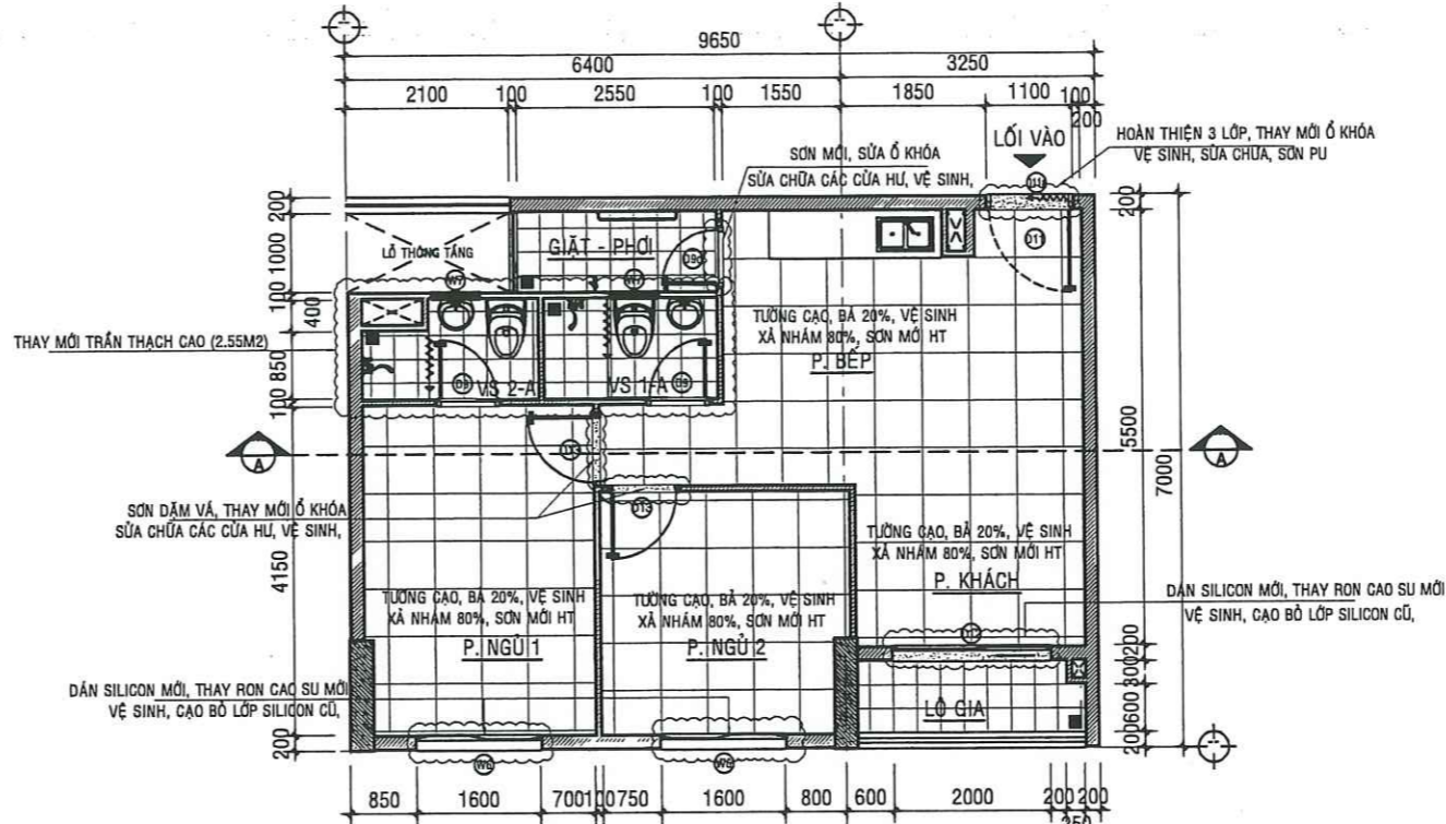
MẶT BẰNG SỬA CHỮA CĂN HỘ A - 14.09 - TL:1/50
