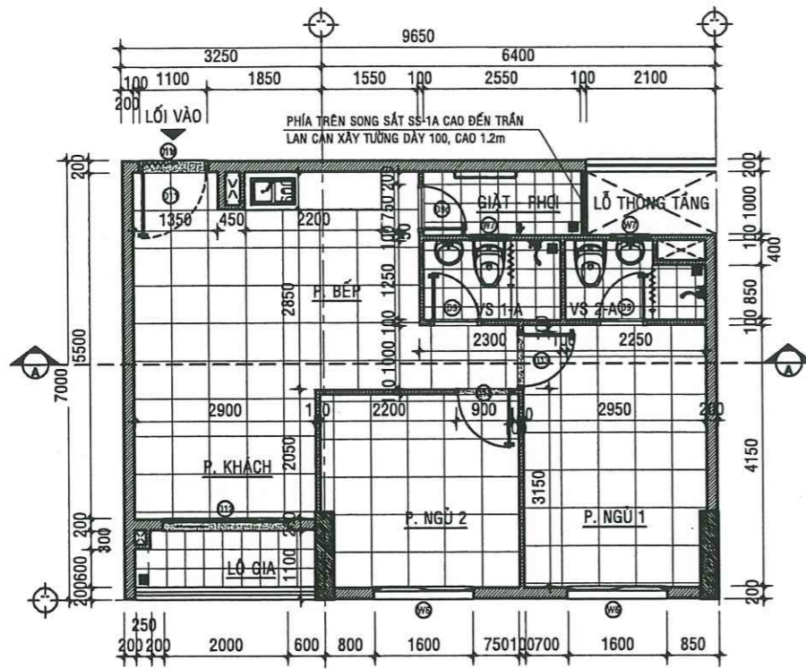
MẶT BẰNG HIỆN TRẠNG CĂN HỘ A - 06.08 - TL:1/50
