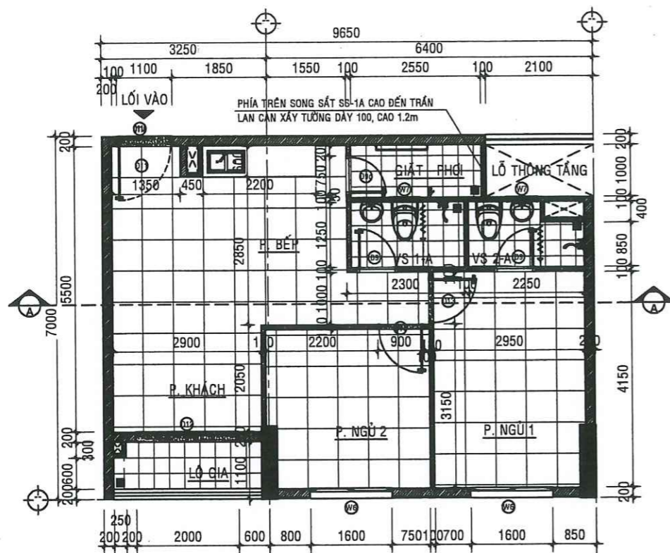
MẶT BẰNG HIỆN TRẠNG CĂN HỘ A - 12.01 - TL:1/50
