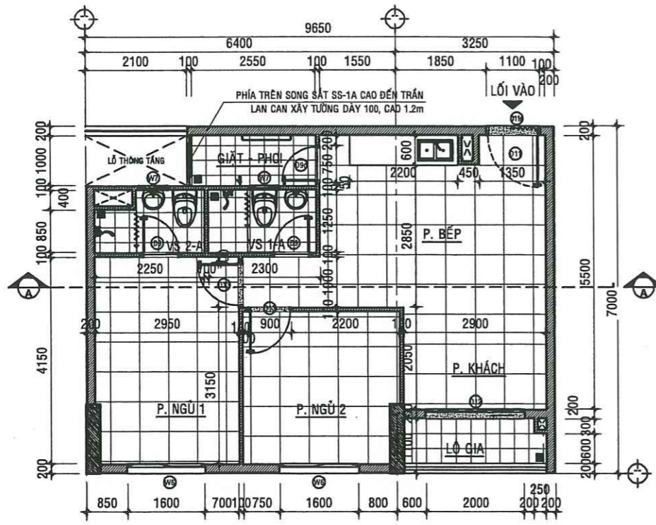
MẶT BẰNG HIỆN TRẠNG CĂN HỘ A -03.02 - TL:1/50
