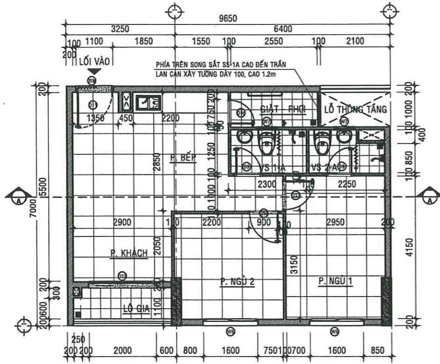
MẶT BẰNG HIỆN TRẠNG CĂN HỘ A -04.01 - TL:1/50
