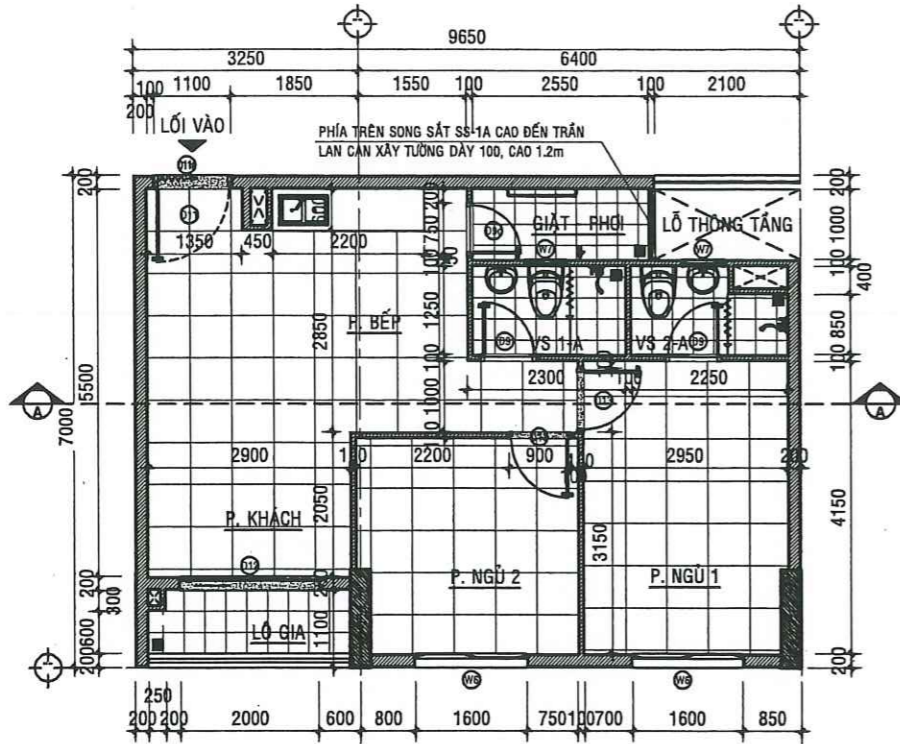
MẶT BẰNG HIỆN TRẠNG CĂN HỘ A -02.01 - TL:1/50
