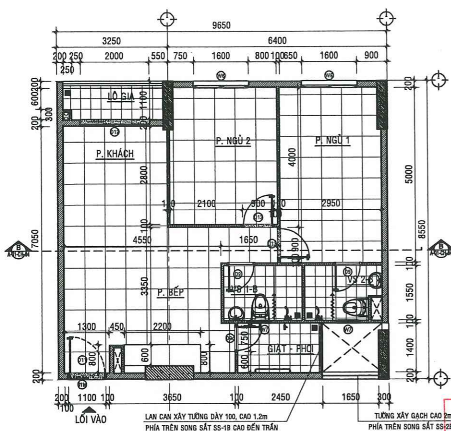
MẶT BẰNG HIỆN TRẠNG CĂN HỘ A - 09.04 - TL:1/50
