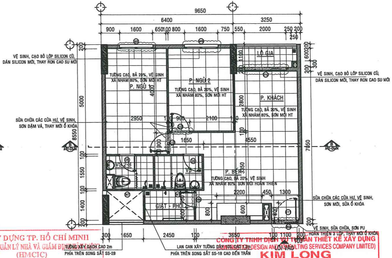
MẶT BẰNG SỬA CHỮA CĂN HỘ A - 08.05 - TL:1/50
