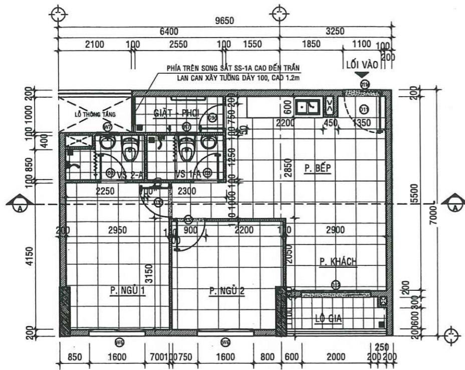
MẶT BẰNG HIỆN TRẠNG CĂN HỘ A -03.09 - TL:1/50
