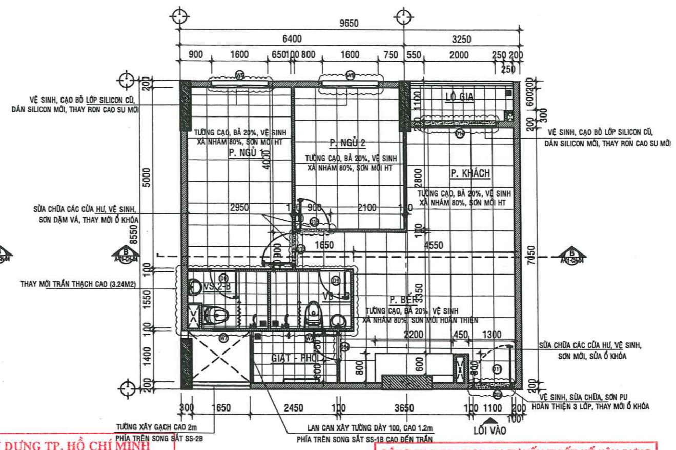
MẶT BẰNG SỬA CHỮA CĂN HỘ A -02.05 - TL:1/50
