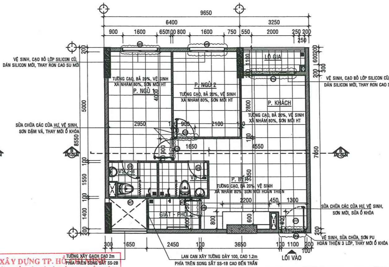
MẶT BẰNG SỬA CHỮA CĂN HỘ A - 06.03 - TL:1/50
