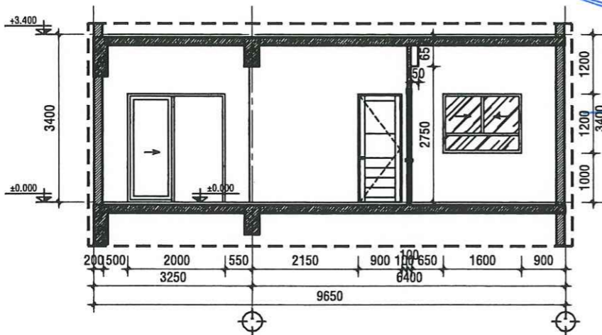
MẶT CẮT B-B - TL:1/50
