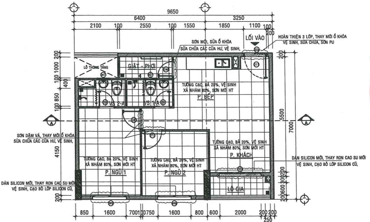
MẶT BẰNG SỬA CHỮA CĂN HỘ A - 10.09 - TL:1/50
