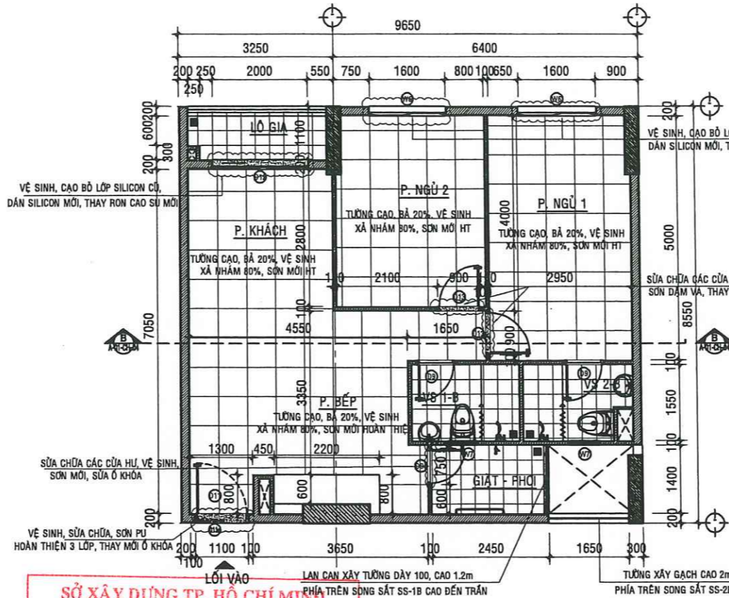
MẶT BẰNG SỬA CHỮA CĂN HỘ A - 05.06 - TL:1/50
