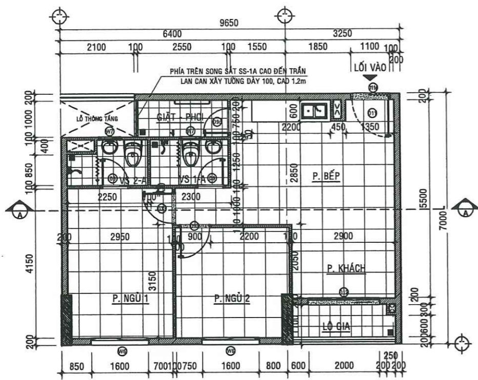
MẶT BẰNG HIỆN TRẠNG CĂN HỘ A - 09.09 - TL:1/50
