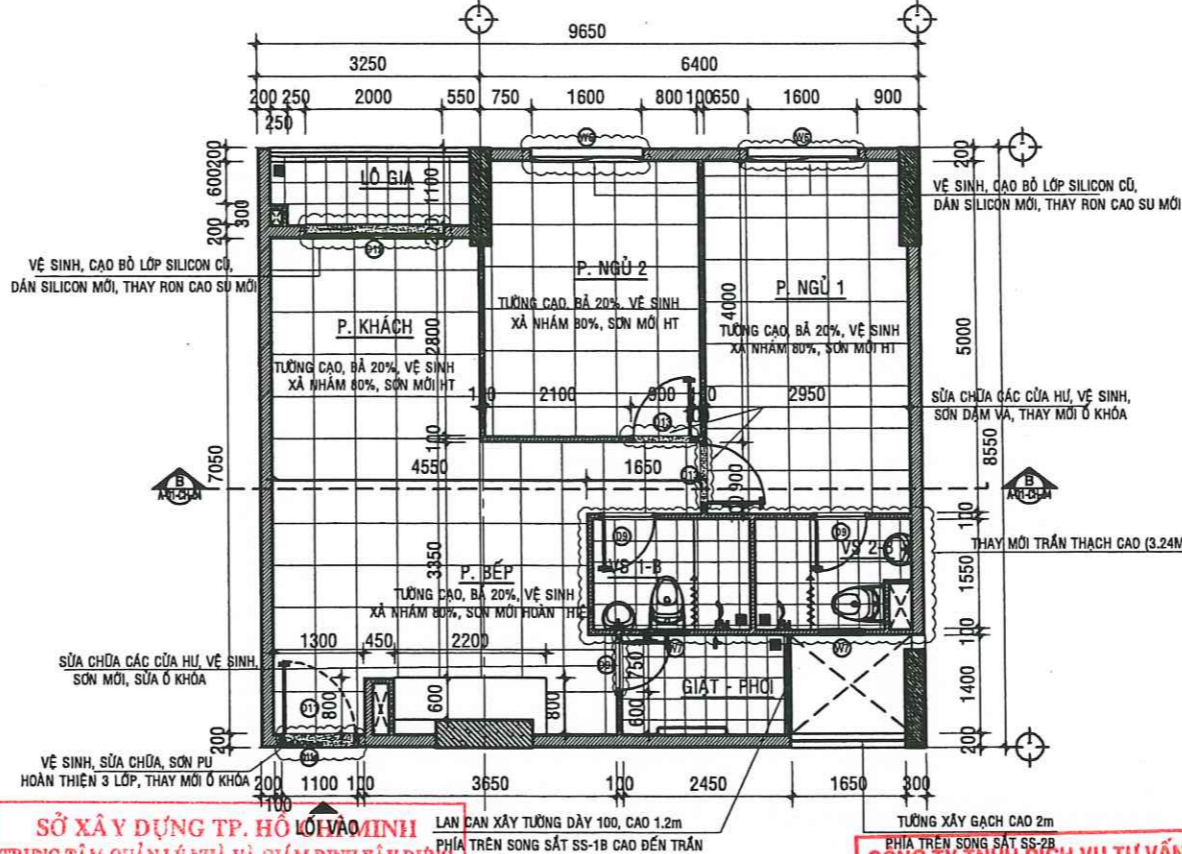
MẶT BẰNG SỬA CHỮA CĂN HỘ A -04.06 - TL:1/50
