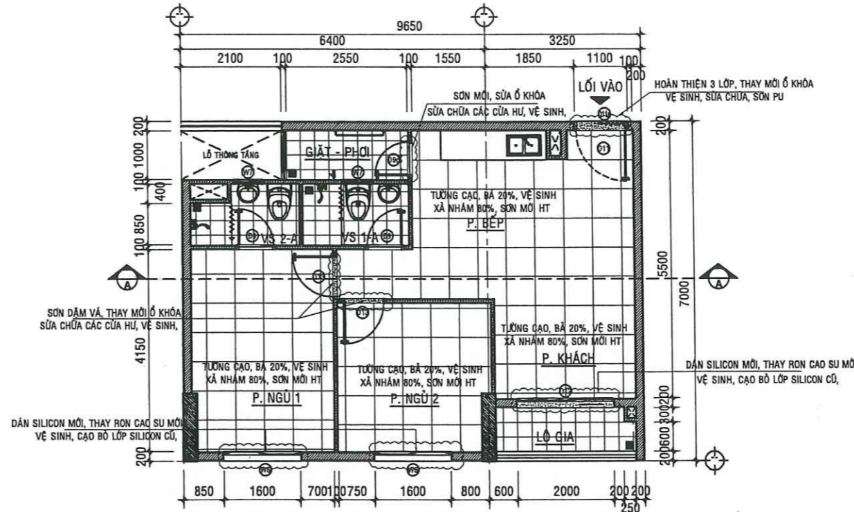
MẶT BẰNG SỬA CHỮA CĂN HỘ A - 11.09 - TL:1/50
