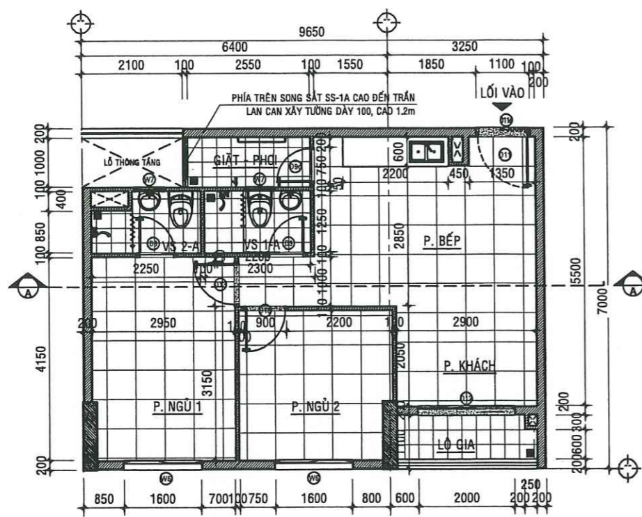
MẶT BẰNG HIỆN TRẠNG CĂN HỘ A - 12.02 - TL:1/50
