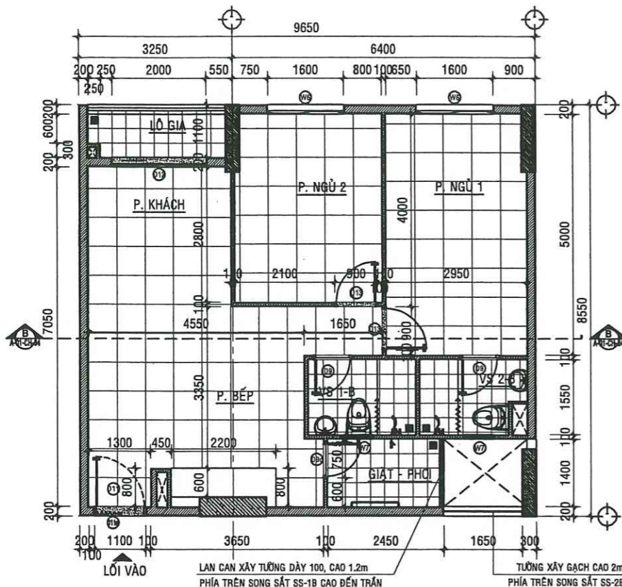
MẶT BẰNG HIỆN TRẠNG CĂN HỘ A -04.04 - TL:1/50
