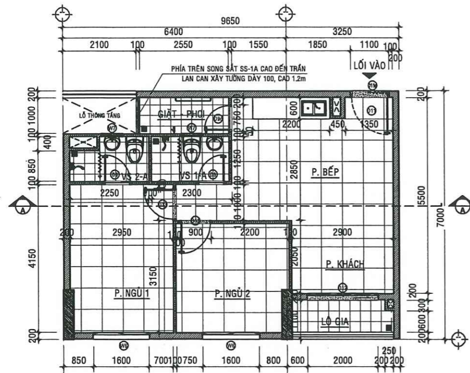
MẶT BẰNG HIỆN TRẠNG CĂN HỘ A - 06.02 - TL:1/50
