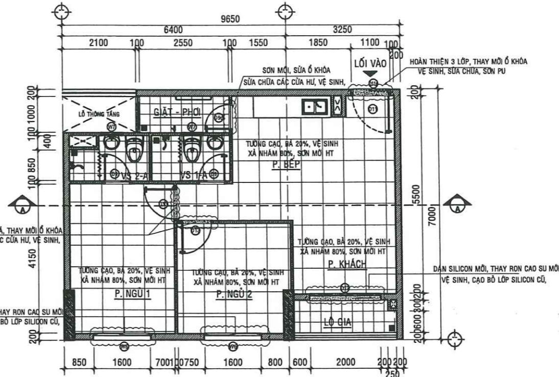
MẶT BẰNG SỬA CHỮA CĂN HỘ A - 05.09 - TL:1/50
