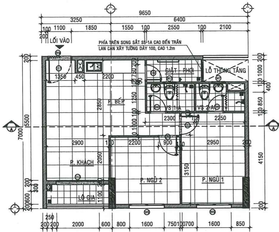
MẶT BẰNG HIỆN TRẠNG CĂN HỘ A - 10.01 - TL:1/50
