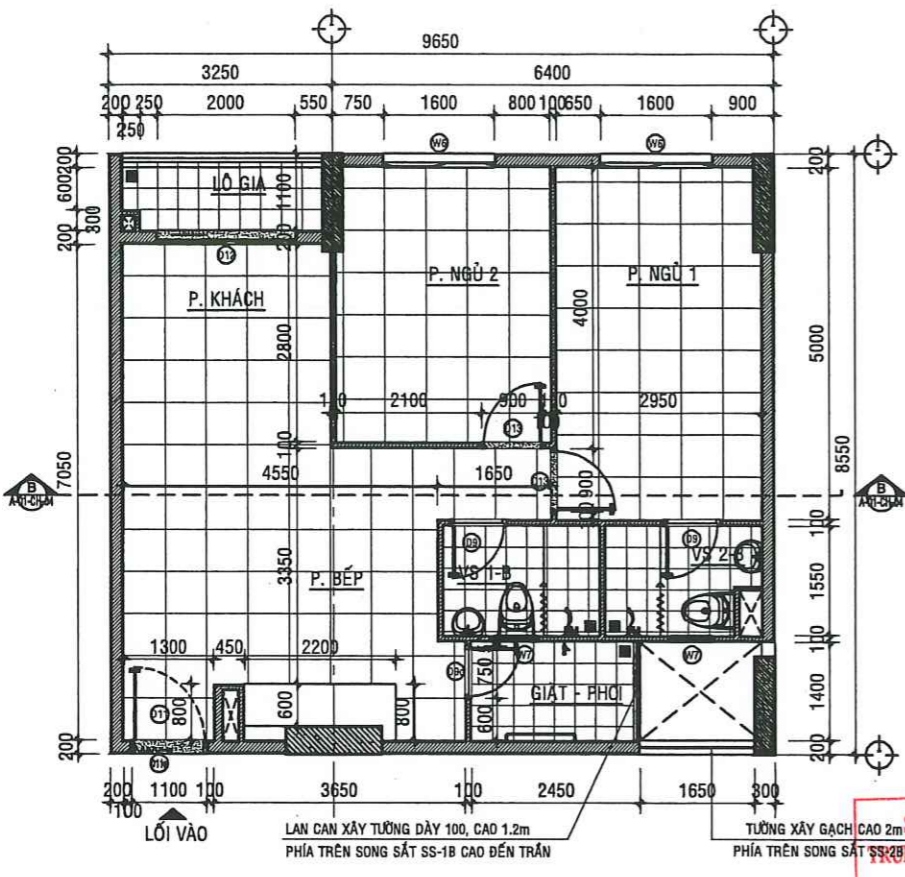
MẶT BẰNG HIỆN TRẠNG CĂN HỘ A -03.04 - TL:1/50
