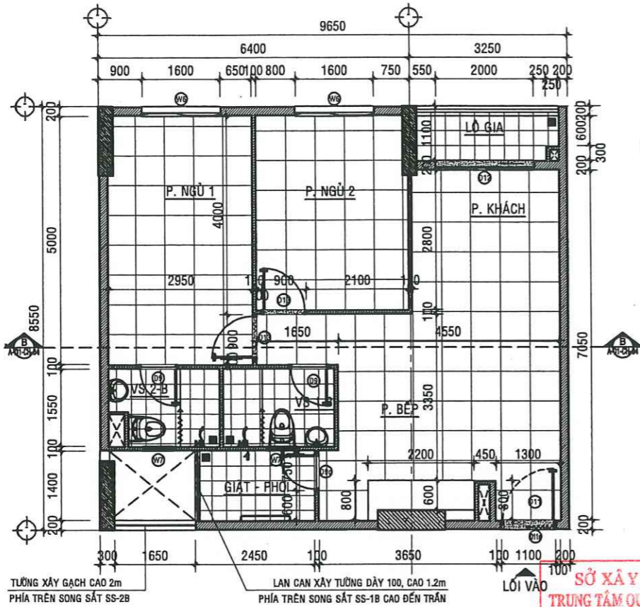
MẶT BẰNG HIỆN TRẠNG CĂN HỘ A - 10.03 - TL:1/50
