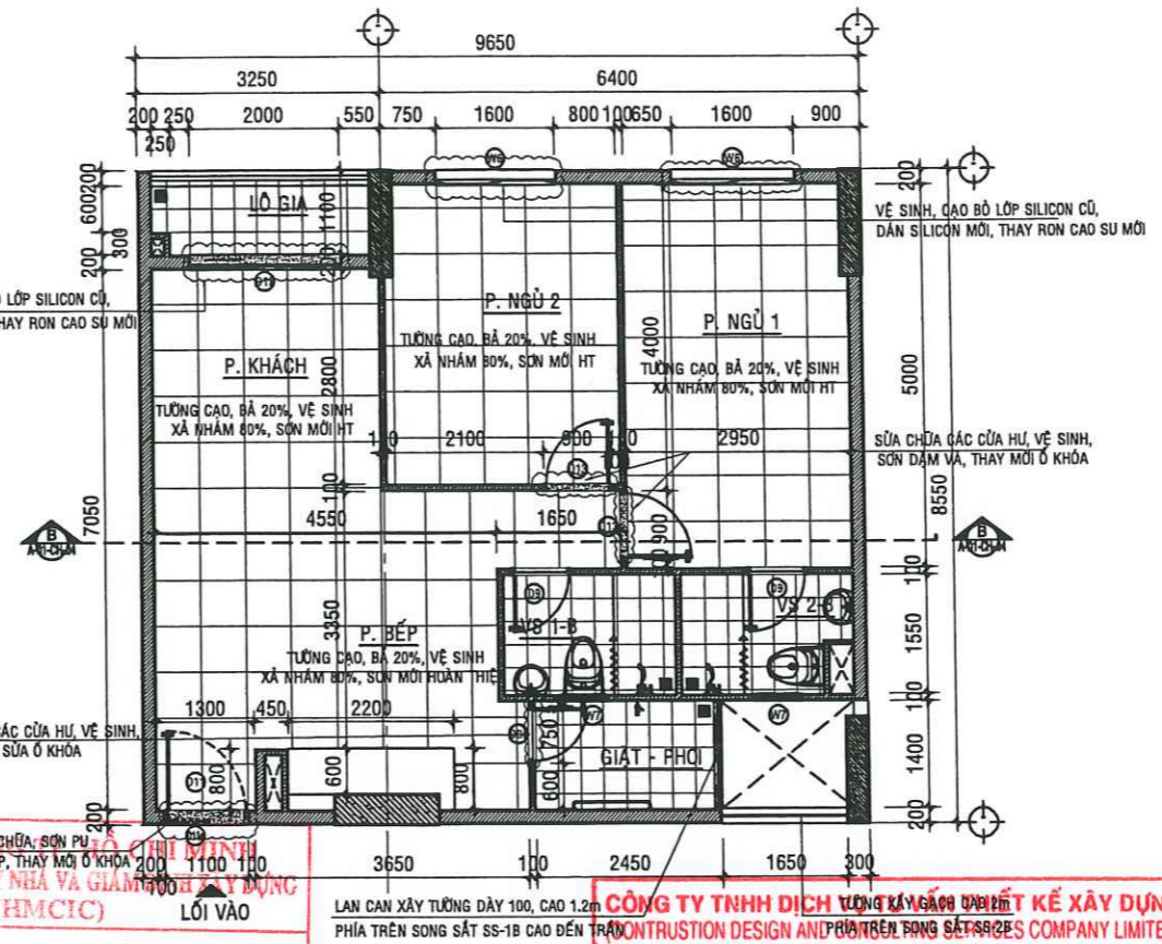
MẶT BẰNG SỬA CHỮA CĂN HỘ A - 10.06 - TL:1/50
