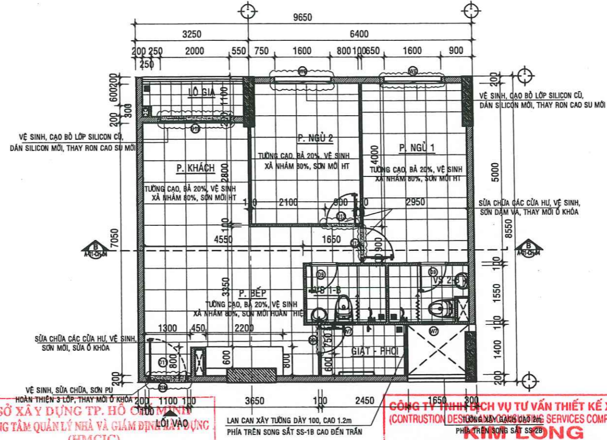
MẶT BẰNG SỬA CHỮA CĂN HỘ A - 08.04 - TL:1/50
