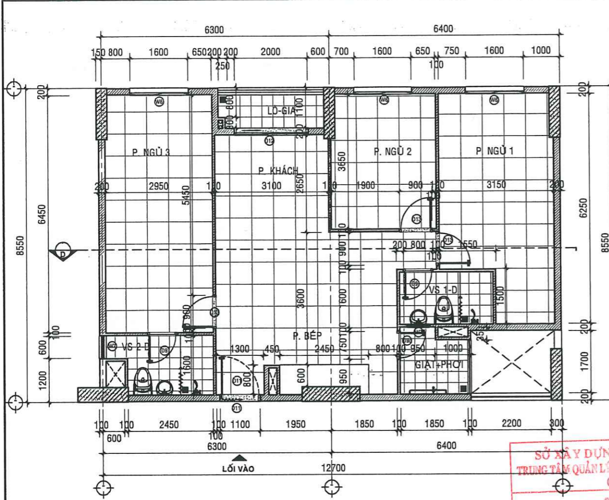
MẶT BẰNG HIỆN TRẠNG CĂN HỘ A - 13.07 - TL: 1/50
