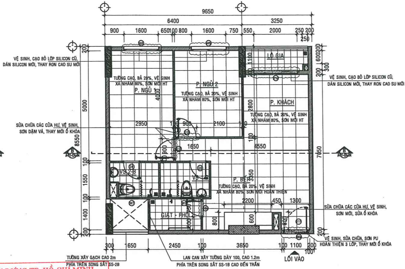
MẶT BẰNG SỬA CHỮA CĂN HỘ A - 05.03 - TL:1/50
