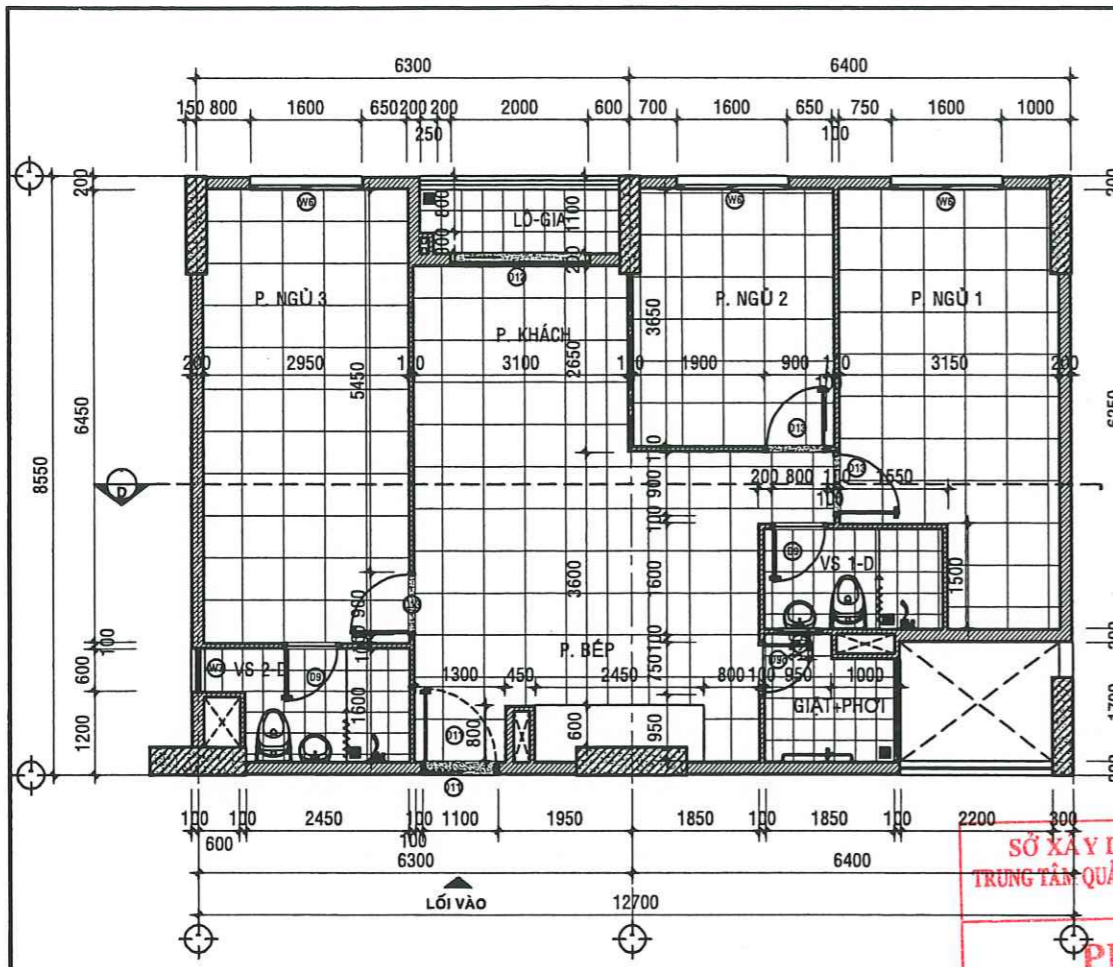
MẶT BẰNG HIỆN TRẠNG CĂN HỘ A -04.07 - TL: 1/50
