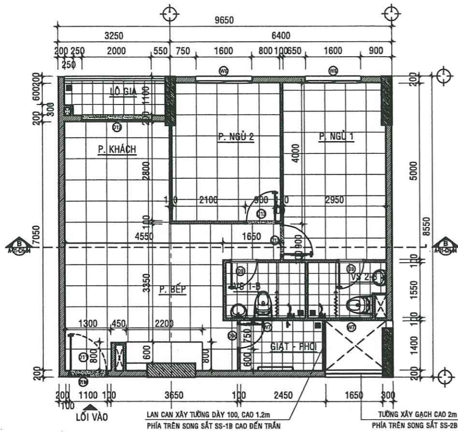
MẶT BẰNG HIỆN TRẠNG CĂN HỘ A - 07.06 - TL:1/50
