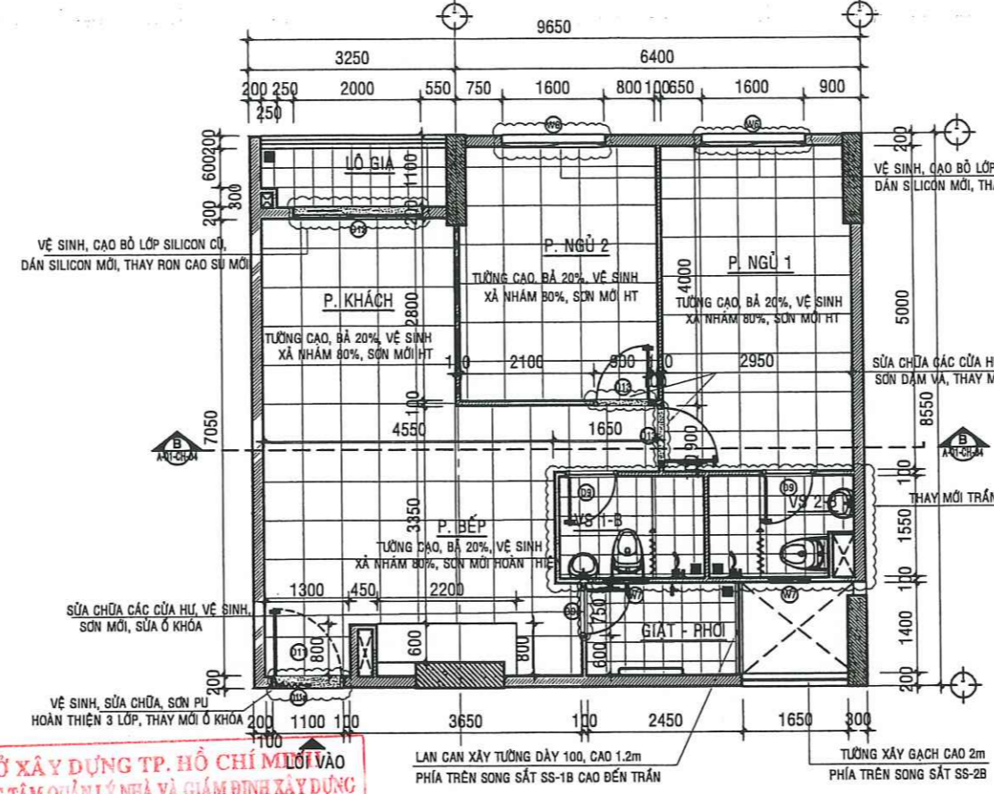
MẶT BẰNG SỬA CHỮA CĂN HỘ A - 14.06 - TL:1/50
