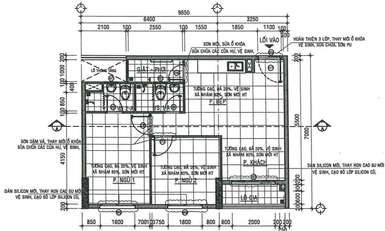
MẶT BẰNG SỬA CHỮA CĂN HỘ A -03.02 - TL:1/50
