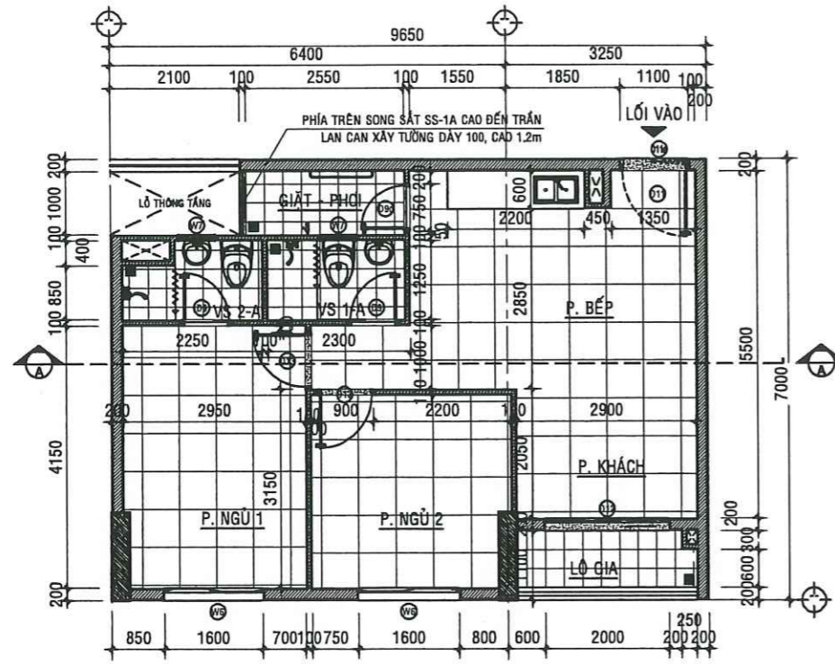
MẶT BẰNG HIỆN TRẠNG CĂN HỘ A - 05.09 - TL:1/50
