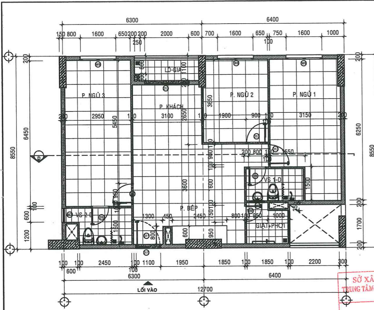
MẶT BẰNG HIỆN TRẠNG CĂN HỘ A - 12.07 - TL: 1/50
