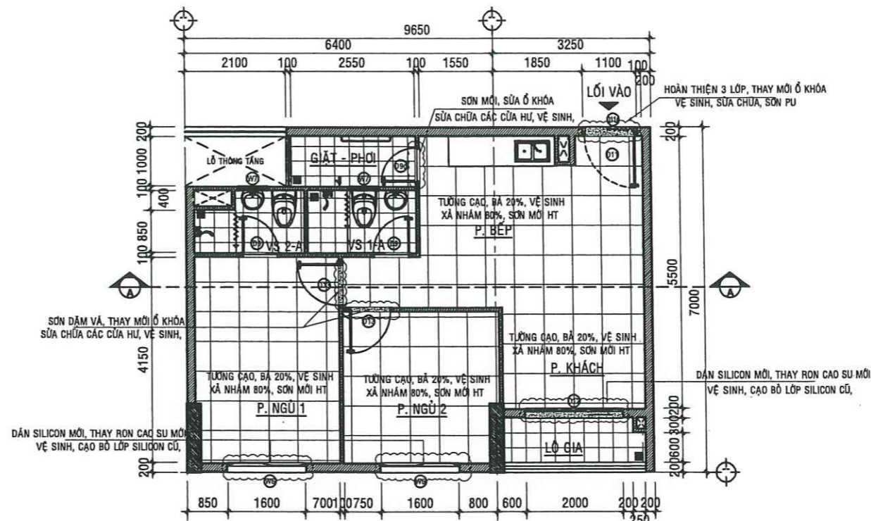
MẶT BẰNG SỬA CHỮA CĂN HỘ A - 08.09 - TL:1/50
