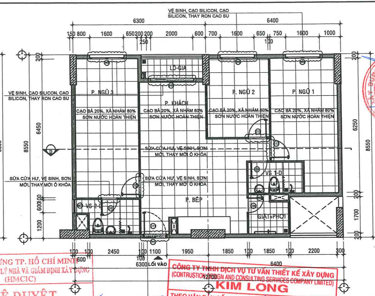
MẶT BẰNG SỬA CHỮA CĂN HỘ A - 08.07 - TL: 1/50
