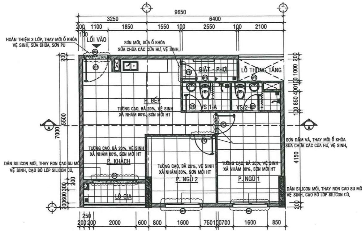
MẶT BẰNG SỬA CHỮA CĂN HỘ A - 05.08 - TL:1/50
