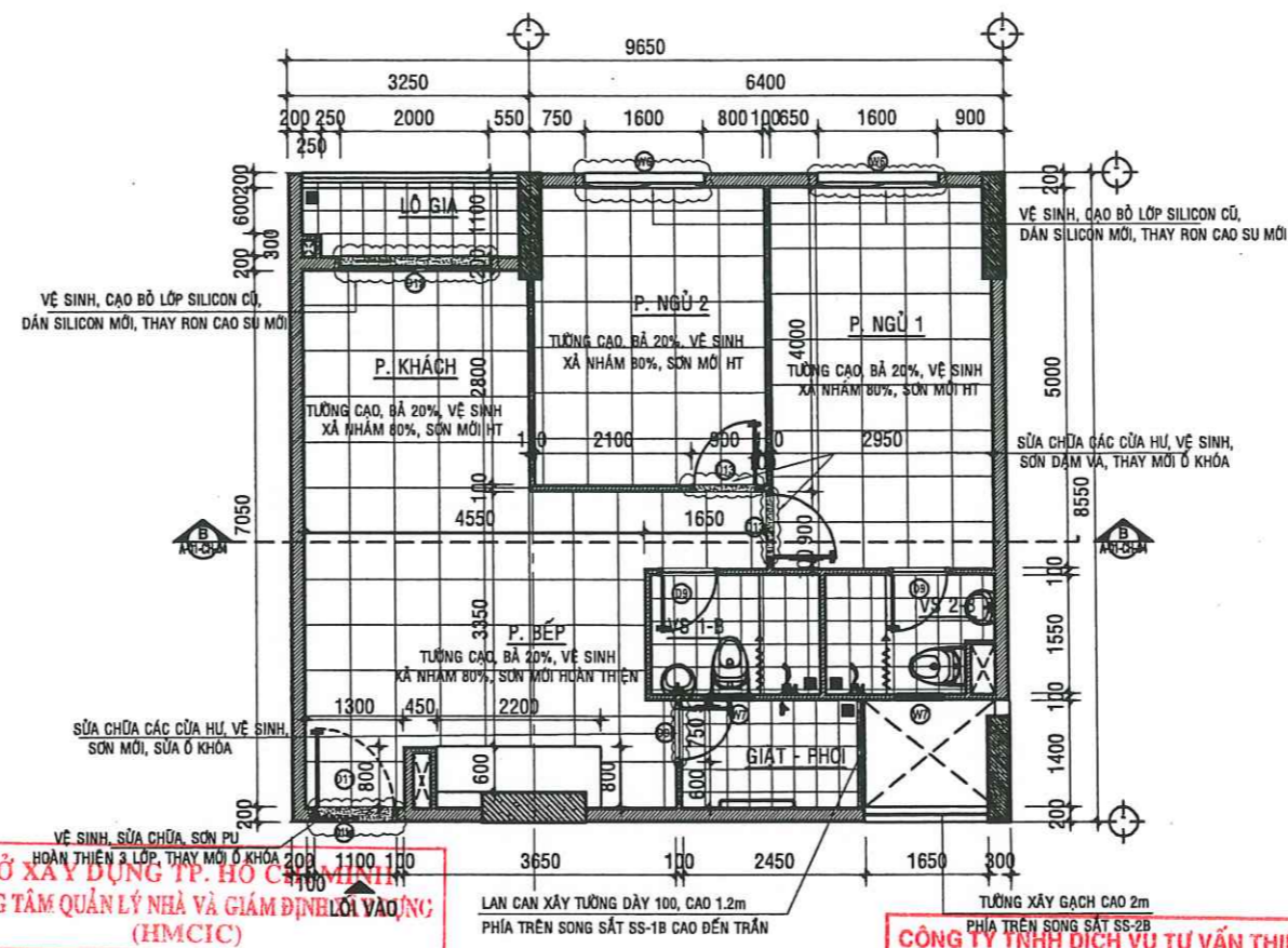
MẶT BẰNG SỬA CHỮA CĂN HỘ A -03.06 - TL:1/50
