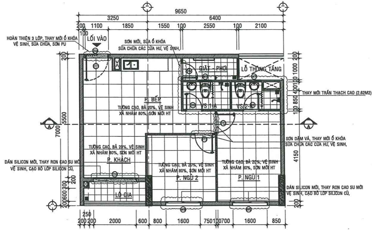
MẶT BẰNG SỬA CHỮA CĂN HỘ A -04.01 - TL:1/50
