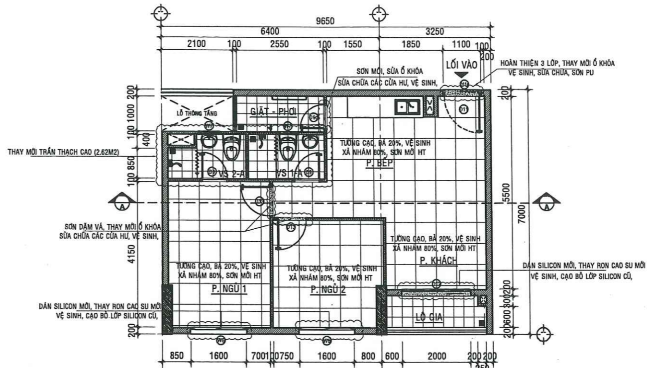
MẶT BẰNG SỬA CHỮA CĂN HỘ A -02.09 - TL:1/50
