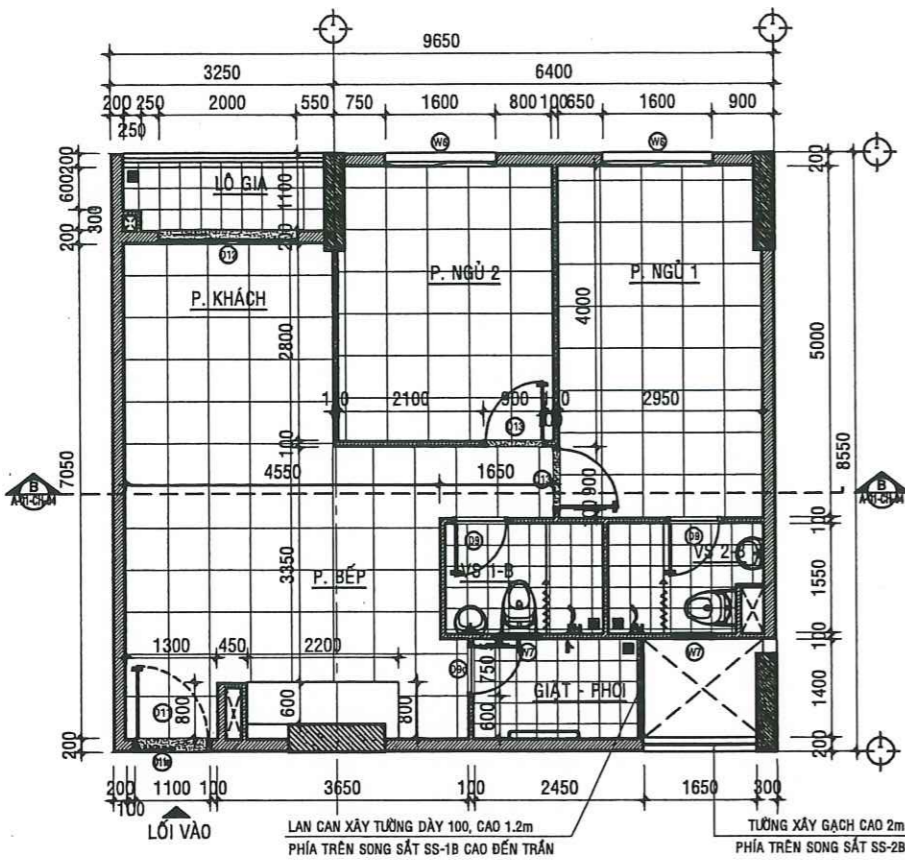
MẶT BẰNG HIỆN TRẠNG CĂN HỘ A - 06.04 - TL:1/50
