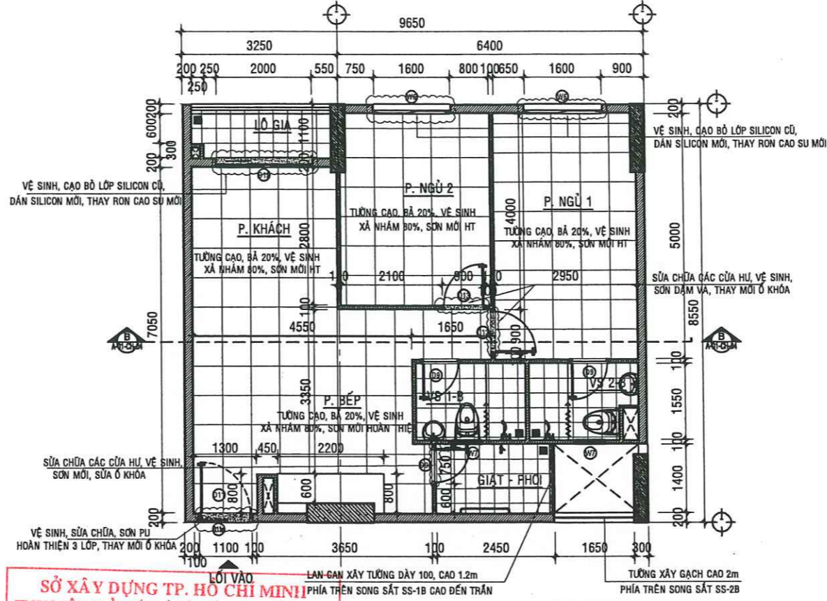
MẶT BẰNG SỬA CHỮA CĂN HỘ A - 05.04 - TL:1/50
