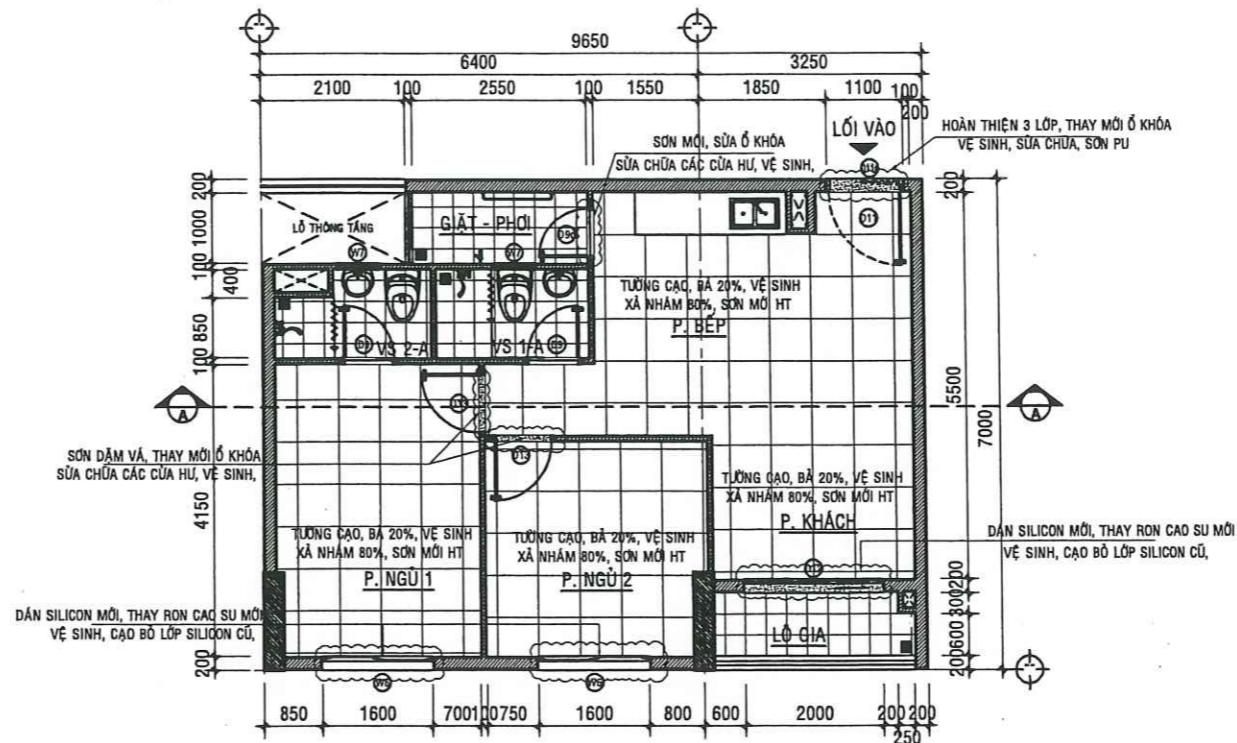
MẶT BẰNG SỬA CHỮA CĂN HỘ A - 05.02 - TL:1/50
