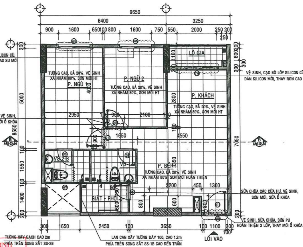
MẶT BẰNG SỬA CHỮA CĂN HỘ A -03.03 - TL:1/50
