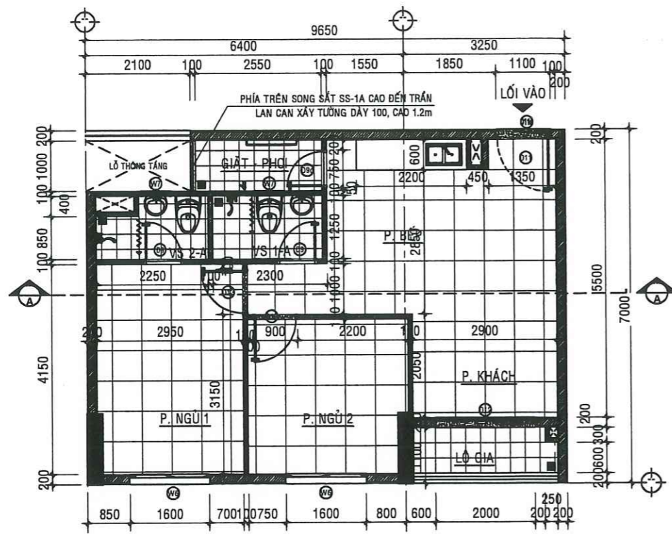
MẶT BẰNG HIỆN TRẠNG CĂN HỘ A - 12.09 - TL:1/50
