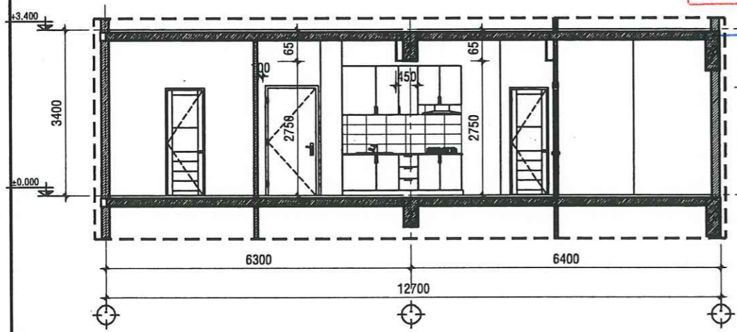
MẶT CẮT D-D - TL: 1/50
