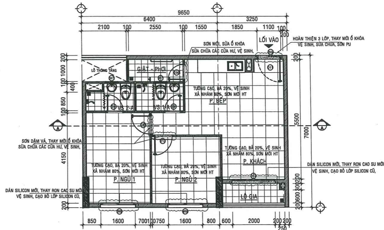
MẶT BẰNG SỬA CHỮA CĂN HỘ A - 08.02 - TL:1/50
