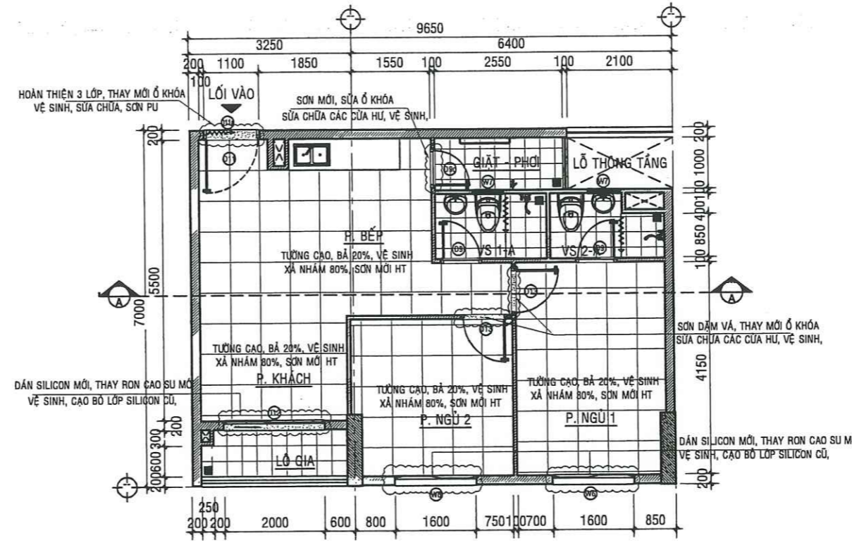
MẶT BẰNG SỬA CHỮA CĂN HỘ A - 13.08 - TL:1/50
