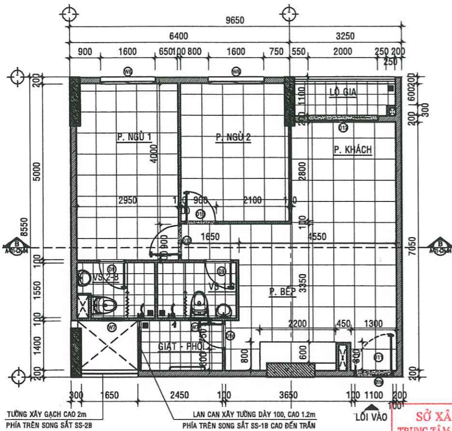
MẶT BẰNG HIỆN TRẠNG CĂN HỘ A - 07.03 - TL:1/50
