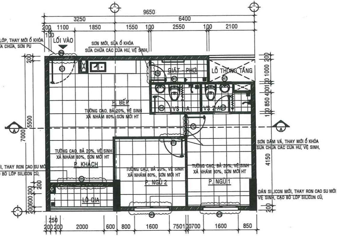
MẶT BẰNG SỬA CHỮA CĂN HỘ A - 12.01 - TL:1/50
