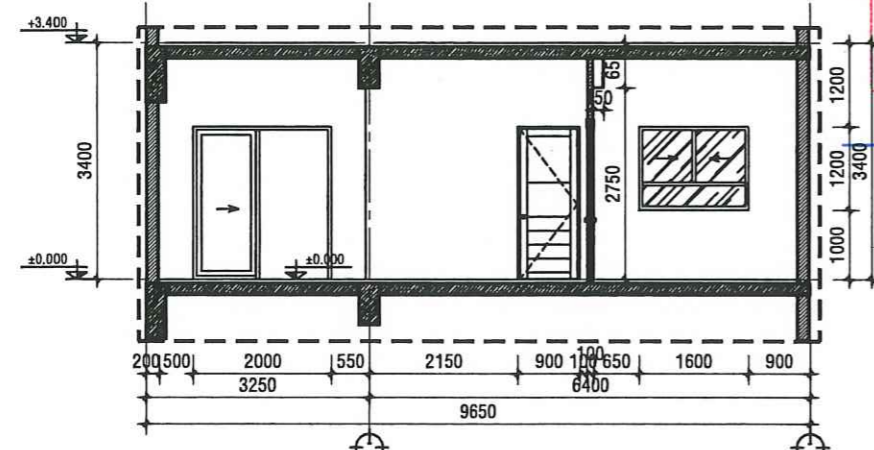
MẶT CẮT B-B - TL:1/50
