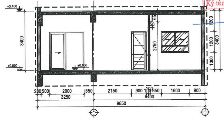
MẶT CẮT B-B - TL:1/50
