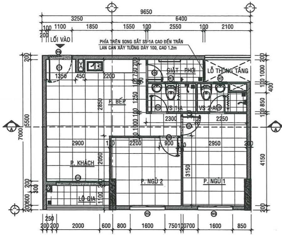
MẶT BẰNG HIỆN TRẠNG CĂN HỘ A -01.04 - TL:1/50
