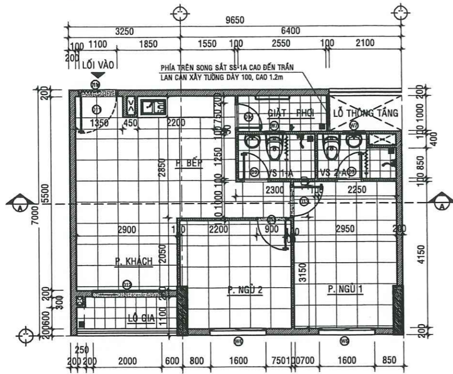
MẶT BẰNG HIỆN TRẠNG CĂN HỘ A - 11.01 - TL:1/50
