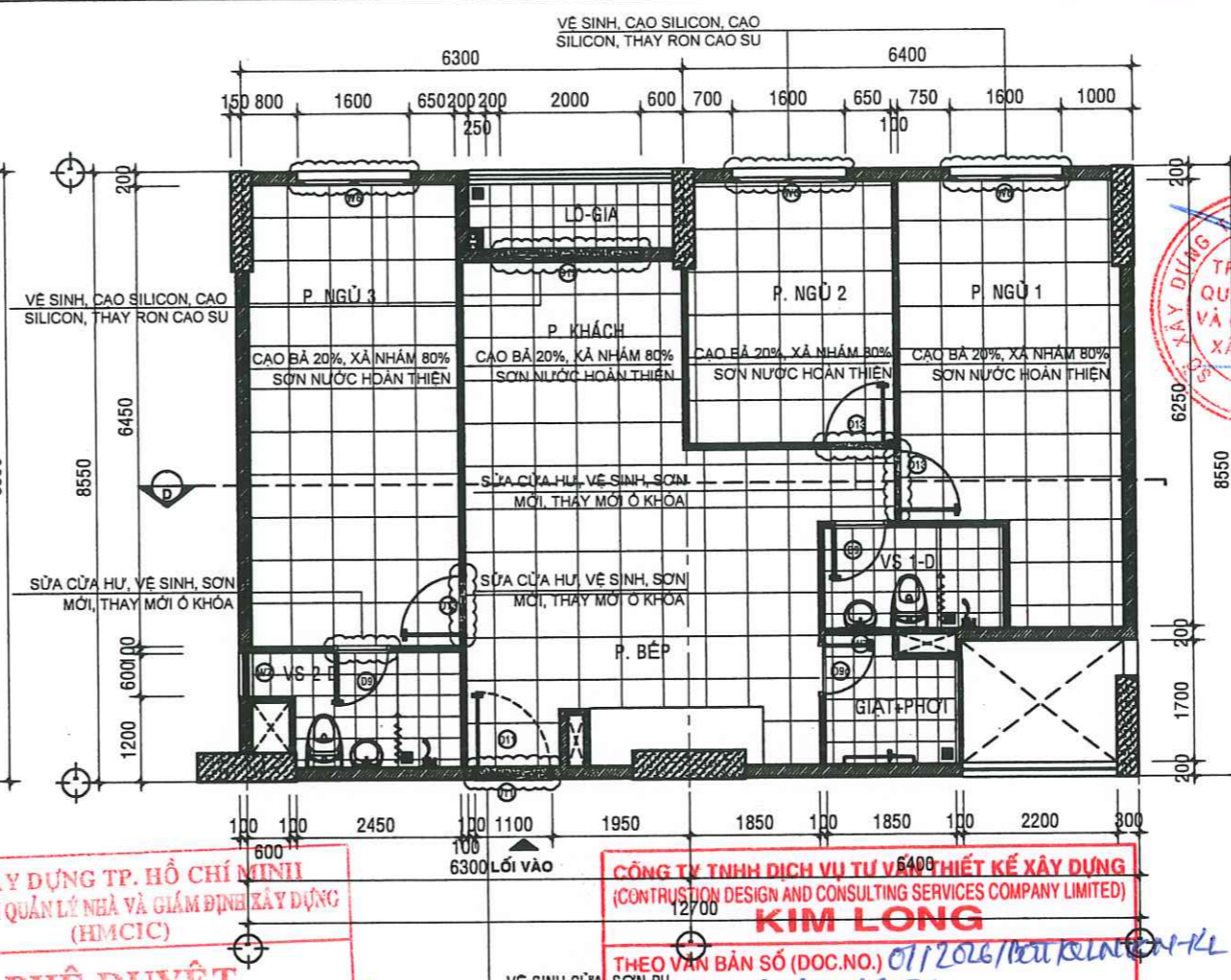
MẶT BẰNG SỬA CHỮA CĂN HỘ A - 12.07 - TL: 1/50
