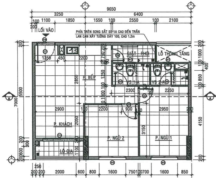
MẶT BẰNG HIỆN TRẠNG CĂN HỘ A -03.08 - TL:1/50
