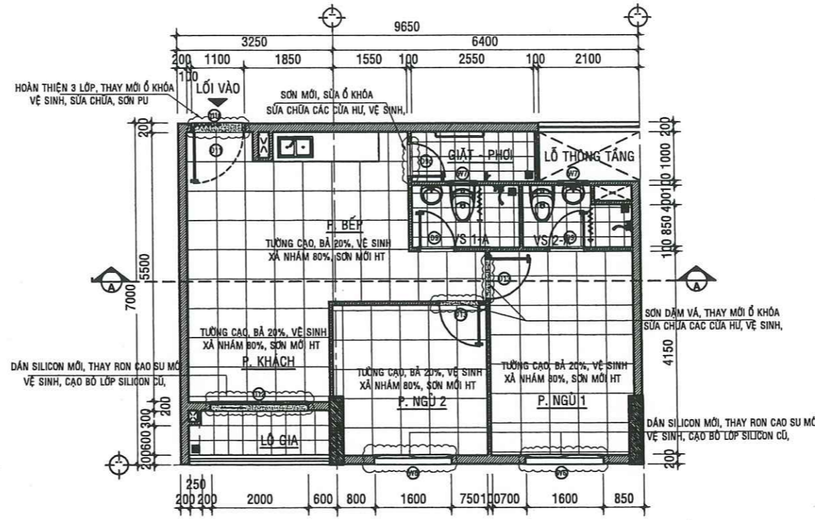
MẶT BẰNG SỬA CHỮA CĂN HỘ A - 06.08 - TL:1/50
