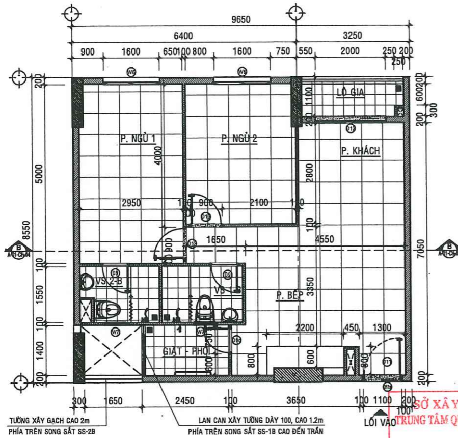
MẶT BẰNG HIỆN TRẠNG CĂN HỘ A - 08.05 - TL:1/50
