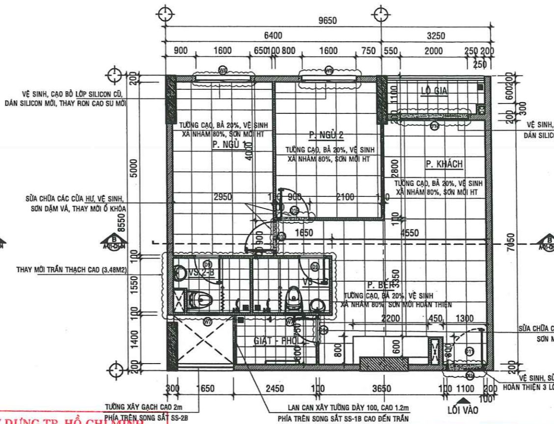
MẶT BẰNG SỬA CHỮA CĂN HỘ A -01.01 - TL:1/50
