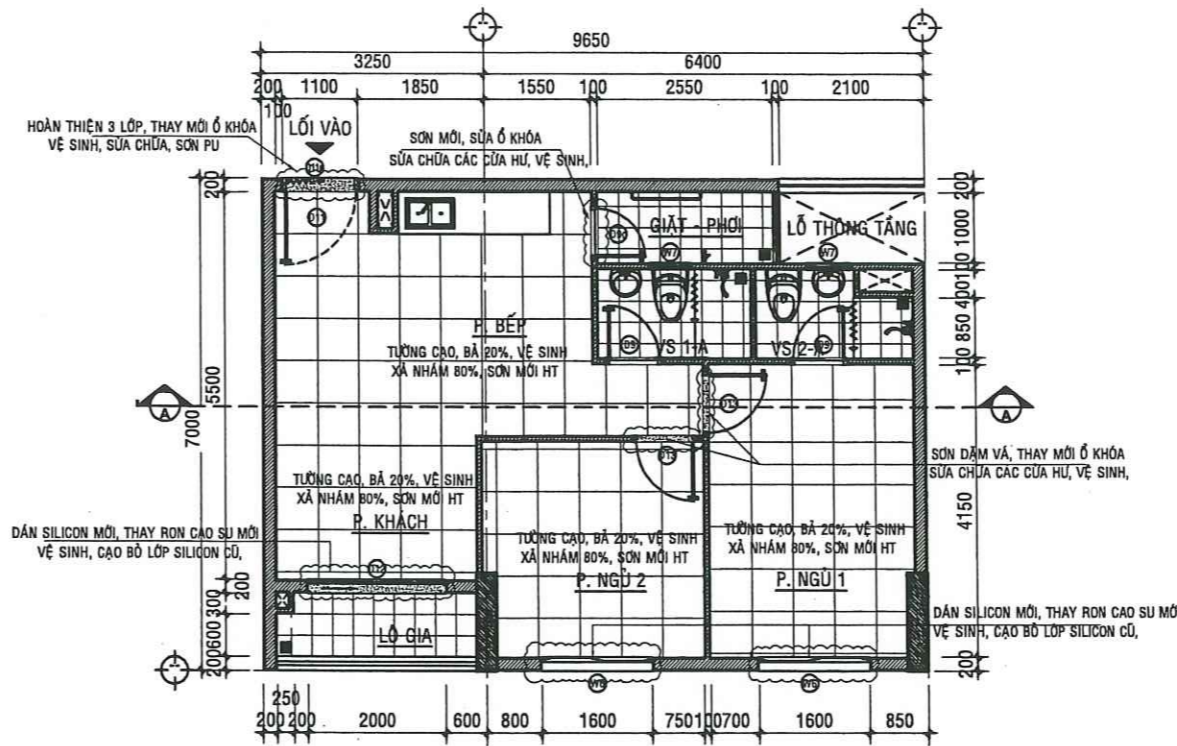
MẶT BẰNG SỬA CHỮA CĂN HỘ A -03.01 - TL:1/50
