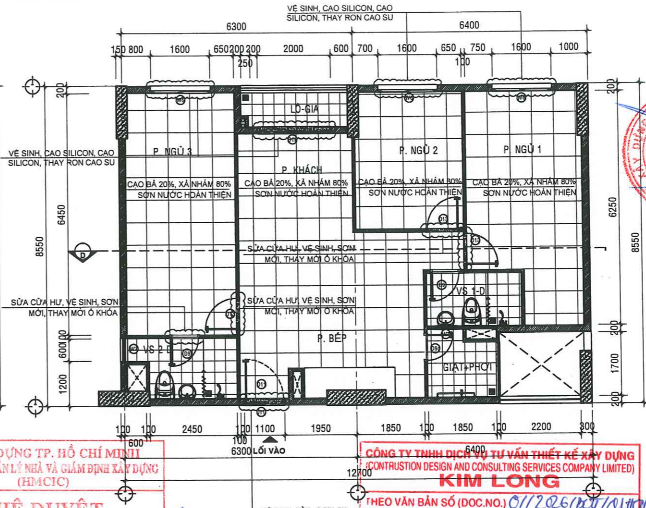
MẶT BẰNG SỬA CHỮA CĂN HỘ A - 11.07 - TL: 1/50
