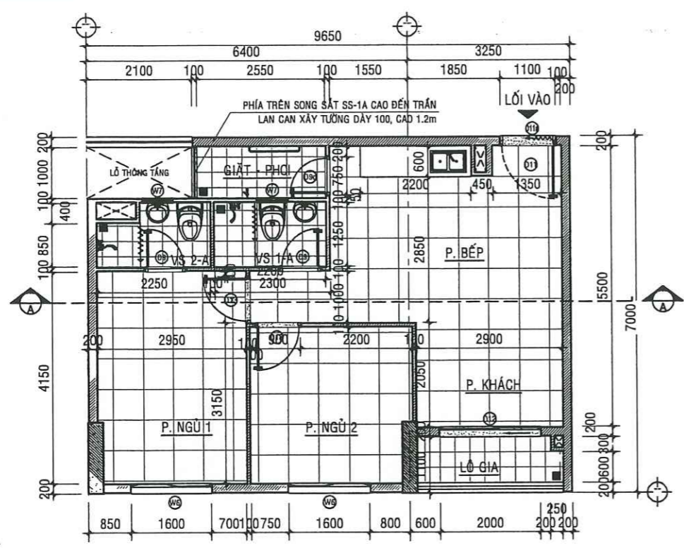
MẶT BẰNG HIỆN TRẠNG CĂN HỘ A - 13.02 - TL:1/50
