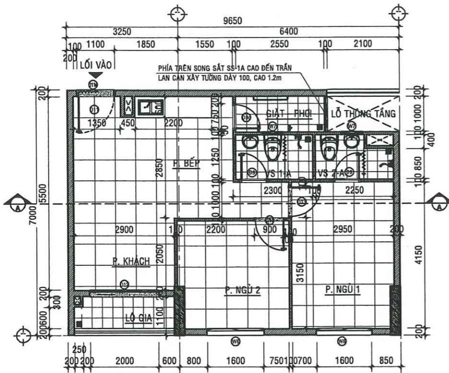
MẶT BẰNG HIỆN TRẠNG CĂN HỘ A - 05.08 - TL:1/50
