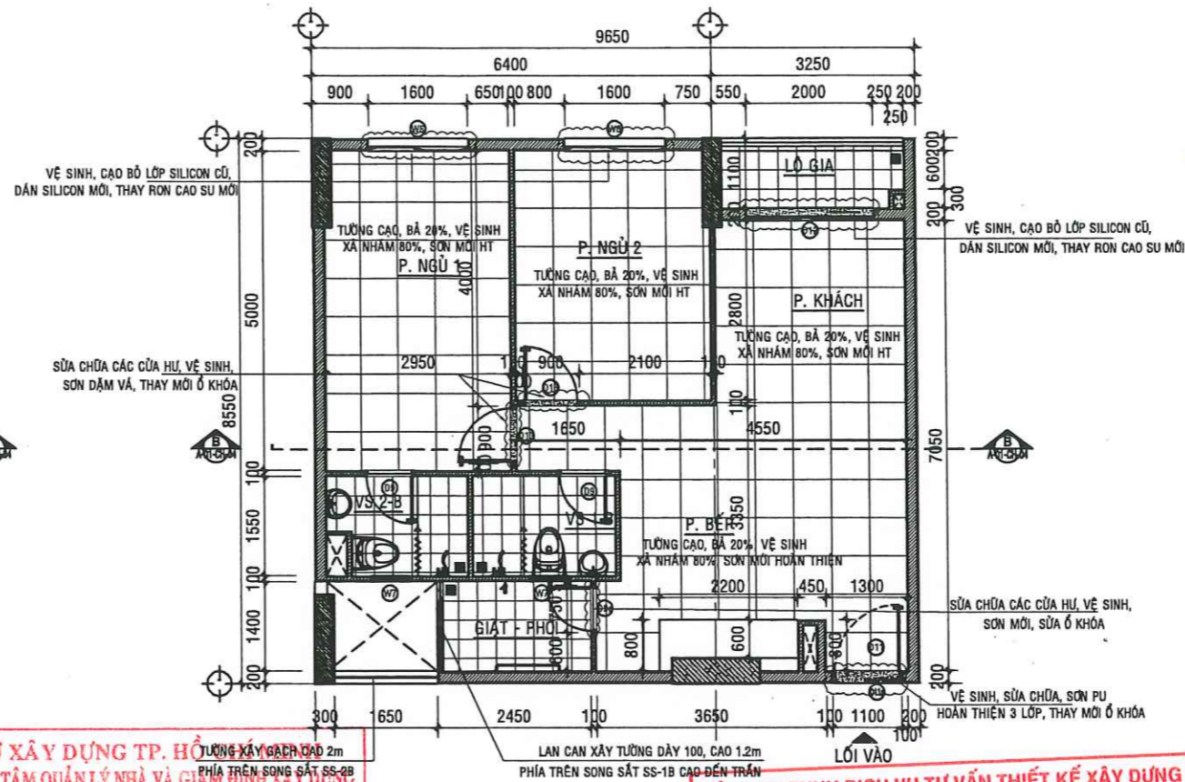
MẶT BẰNG SỬA CHỮA CĂN HỘ A - 05.05 - TL:1/50
