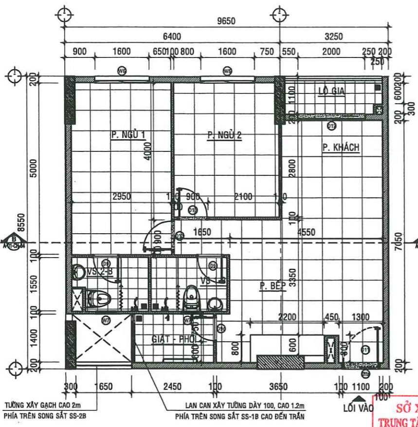
MẶT BẰNG HIỆN TRẠNG CĂN HỘ A -02.03 - TL:1/50
