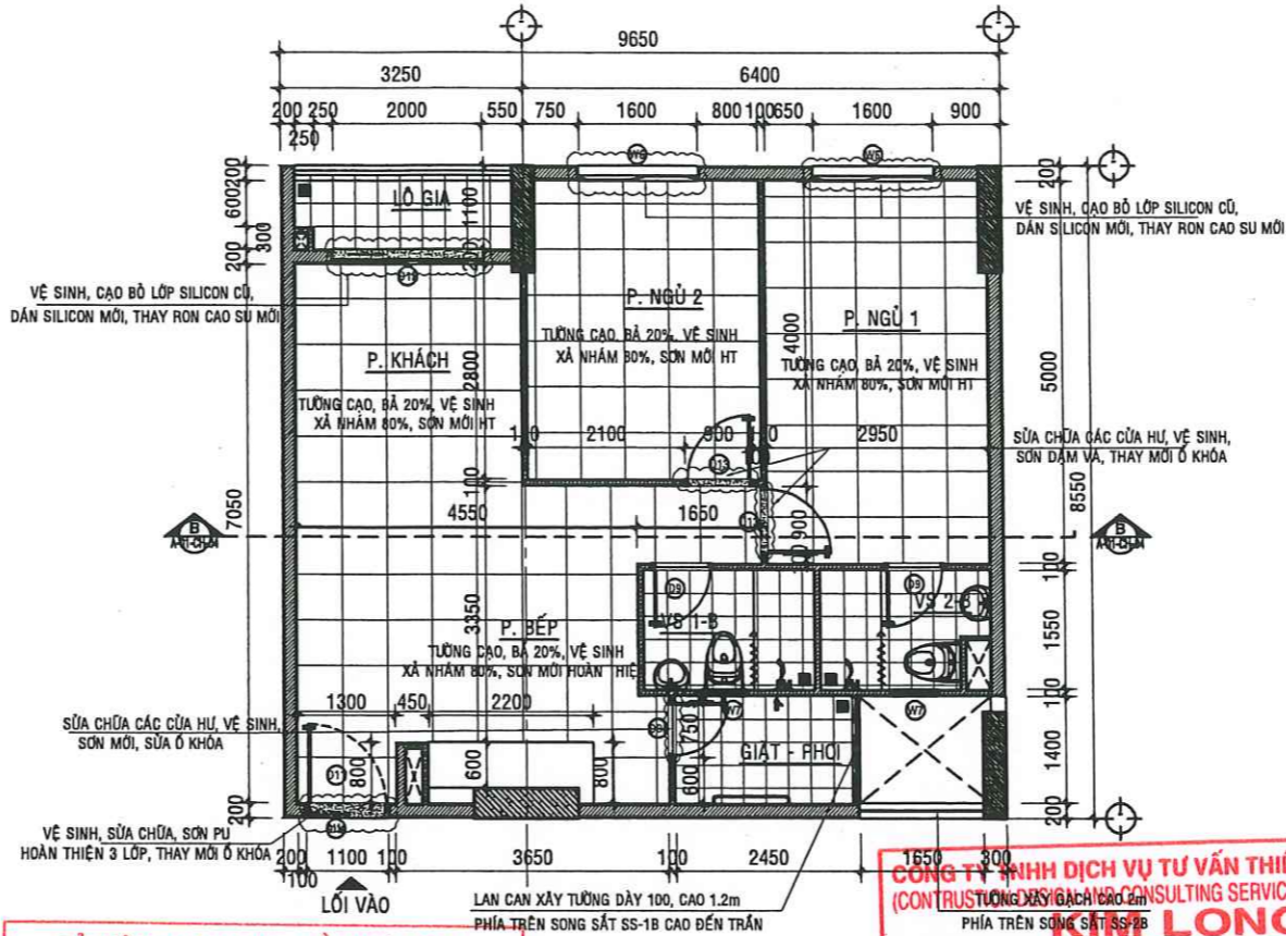
MẶT BẰNG SỬA CHỮA CĂN HỘ A - 07.06 - TL:1/50
