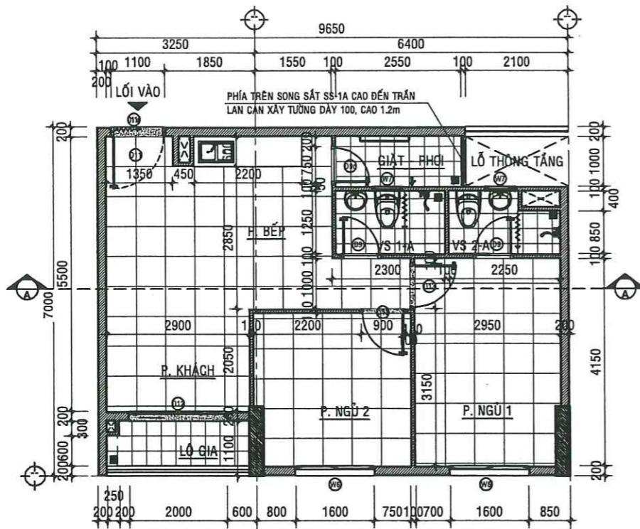
MẶT BẰNG HIỆN TRẠNG CĂN HỘ A - 09.08 - TL:1/50
