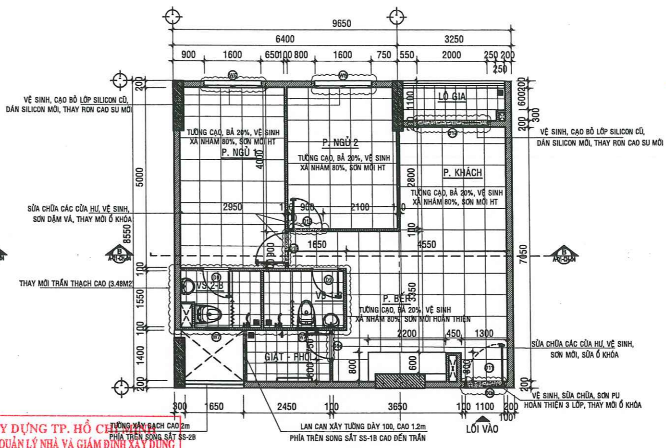
MẶT BẰNG SỬA CHỮA CĂN HỘ A -02.03 - TL:1/50
