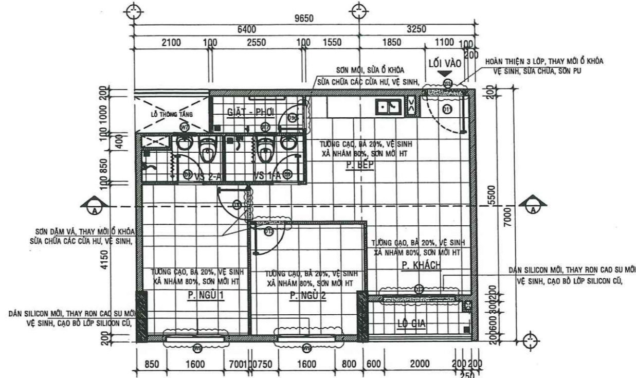
MẶT BẰNG SỬA CHỮA CĂN HỘ A - 09.02 - TL:1/50
