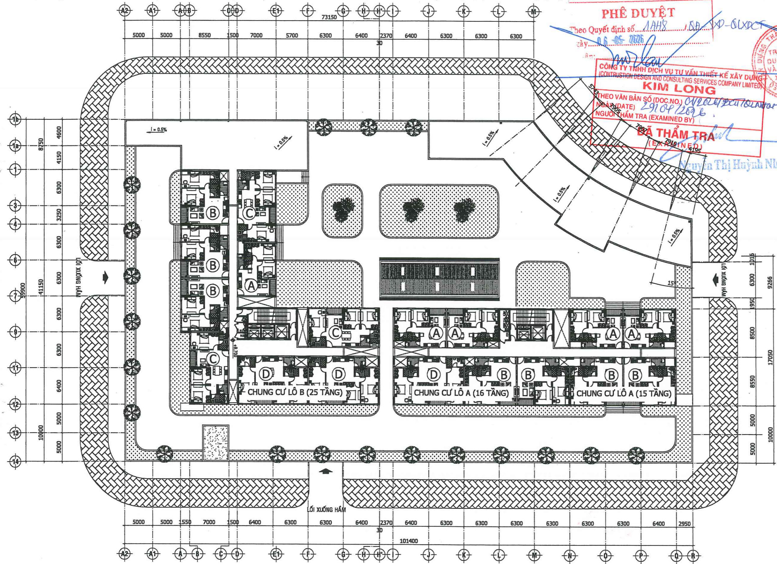
MẶT BẰNG TỔNG THỂ CĂN HỘ ĐIỂN HÌNH - TL: 1/400
