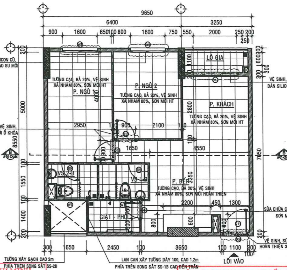
MẶT BẰNG SỬA CHỮA CĂN HỘ A - 07.05 - TL:1/50
