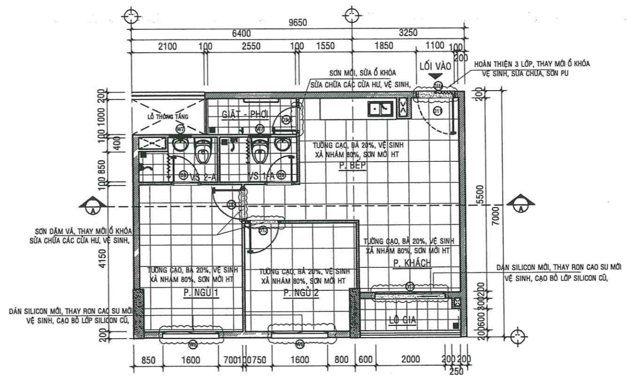
MẶT BẰNG SỬA CHỮA CĂN HỘ A - 13.02 - TL:1/50
