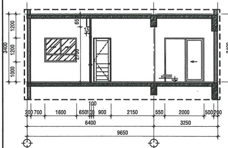
MẶT CẮT B-B - TL:1/50
