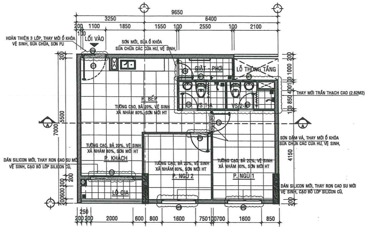
MẶT BẰNG SỬA CHỮA CĂN HỘ A -01.04 - TL:1/50
