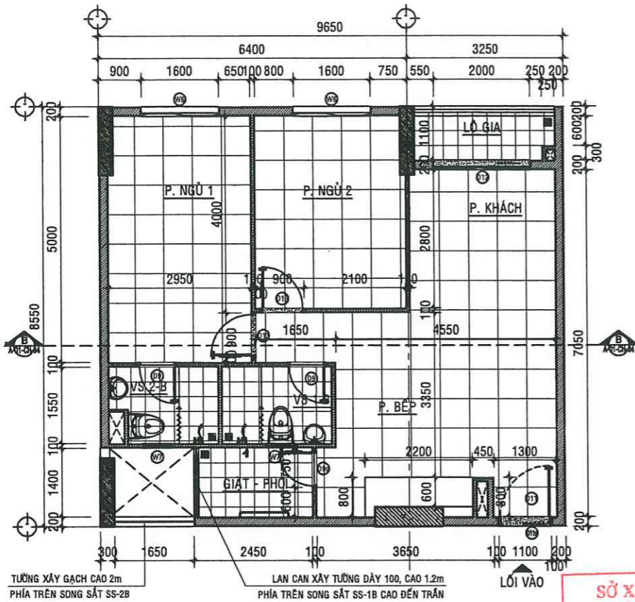
MẶT BẰNG HIỆN TRẠNG CĂN HỘ A - 12.03 - TL:1/50
