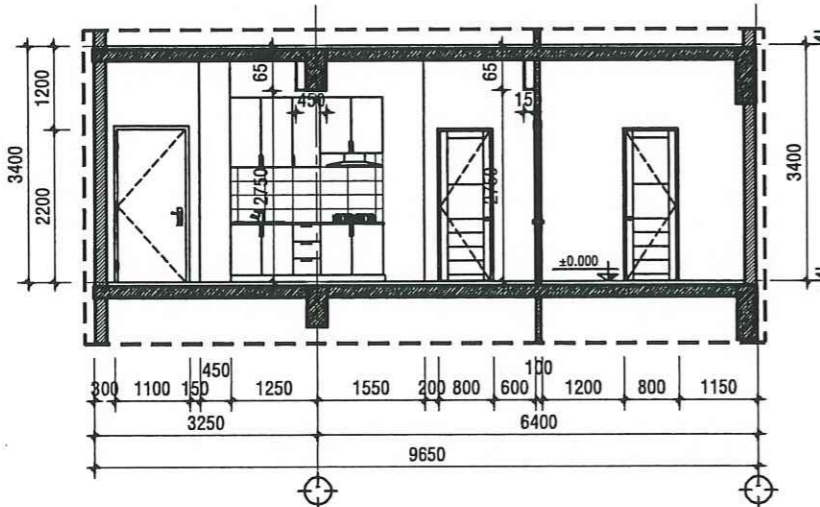
MẶT CẮT A-A - TL:1/50
