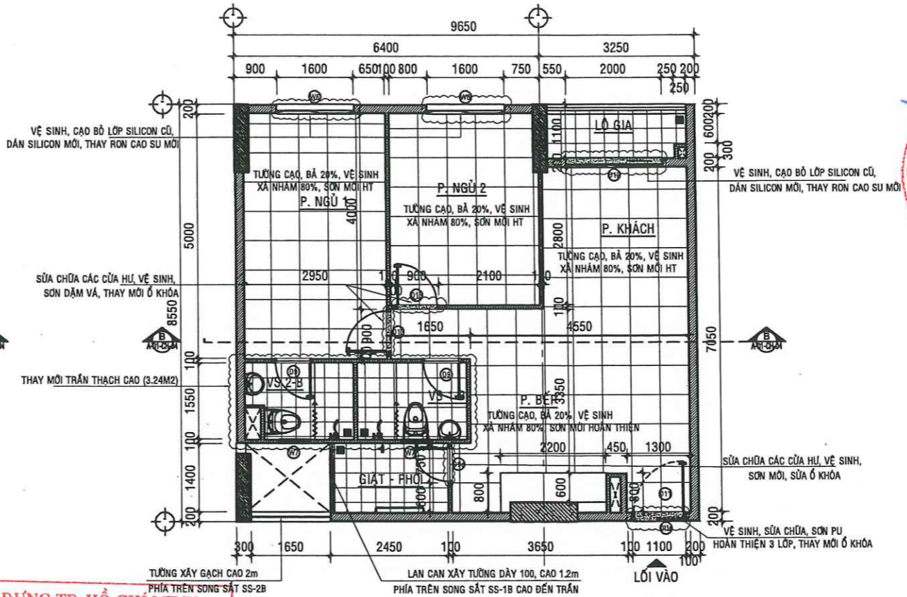
MẶT BẰNG SỬA CHỮA CĂN HỘ A -04.05 - TL:1/50
