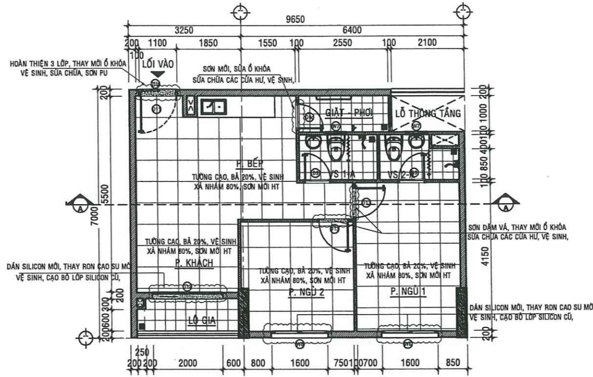
MẶT BẰNG SỬA CHỮA CĂN HỘ A - 08.01 - TL:1/50
