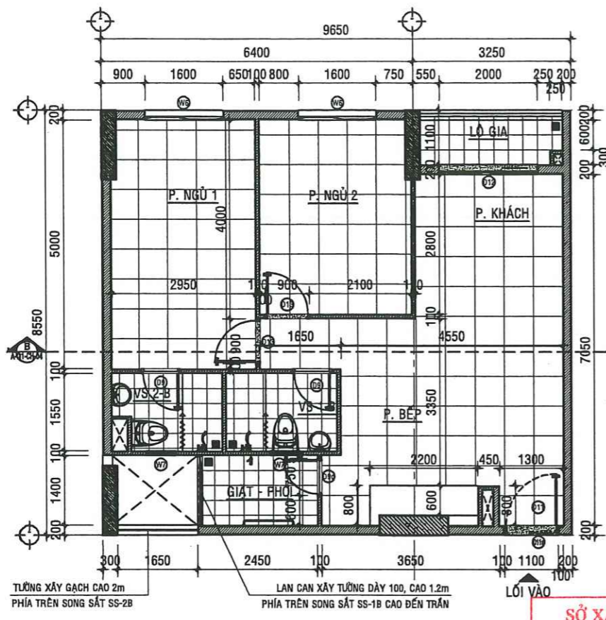
MẶT BẰNG HIỆN TRẠNG CĂN HỘ A -02.05 - TL:1/50
