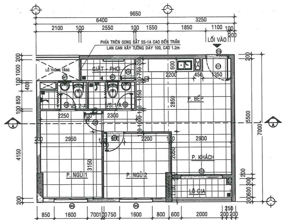
MẶT BẰNG HIỆN TRẠNG CĂN HỘ A - 13.09 - TL:1/50
