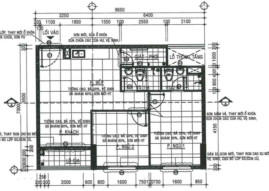
MẶT BẰNG SỬA CHỮA CĂN HỘ A - 11.08 - TL:1/50
