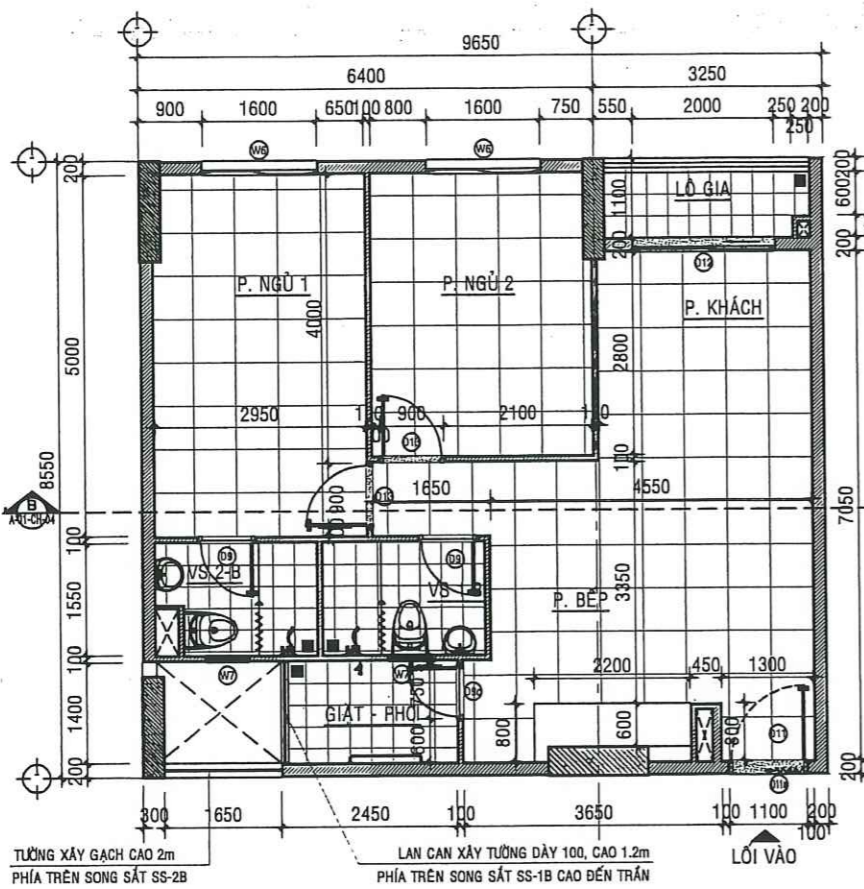
MẶT BẰNG HIỆN TRẠNG CĂN HỘ A - 13.05 - TL:1/50
