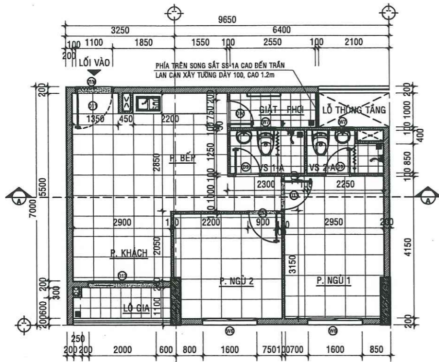
MẶT BẰNG HIỆN TRẠNG CĂN HỘ A - 06.01 - TL:1/50
