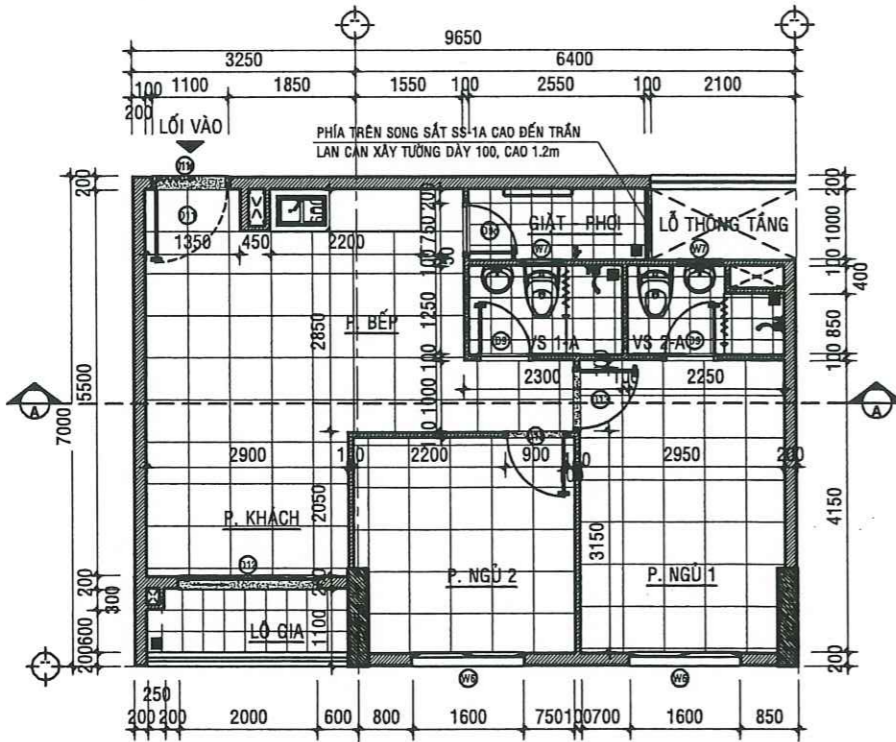
MẶT BẰNG HIỆN TRẠNG CĂN HỘ A - 07.08 - TL:1/50
