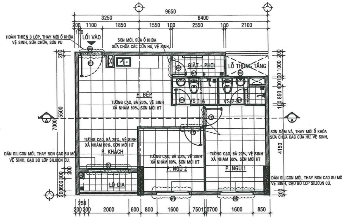
MẶT BẰNG SỬA CHỮA CĂN HỘ A - 09.08 - TL:1/50
