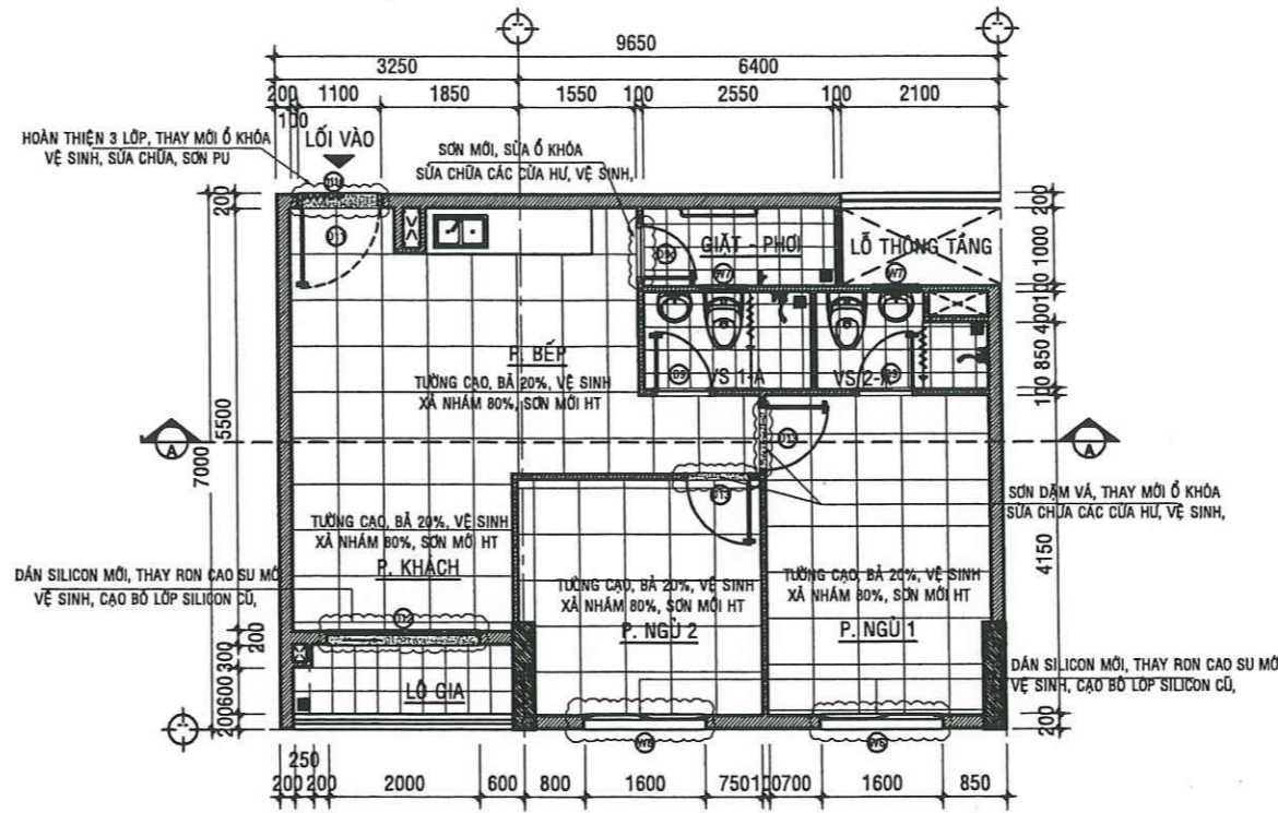
MẶT BẰNG SỬA CHỮA CĂN HỘ A - 07.01 - TL:1/50
