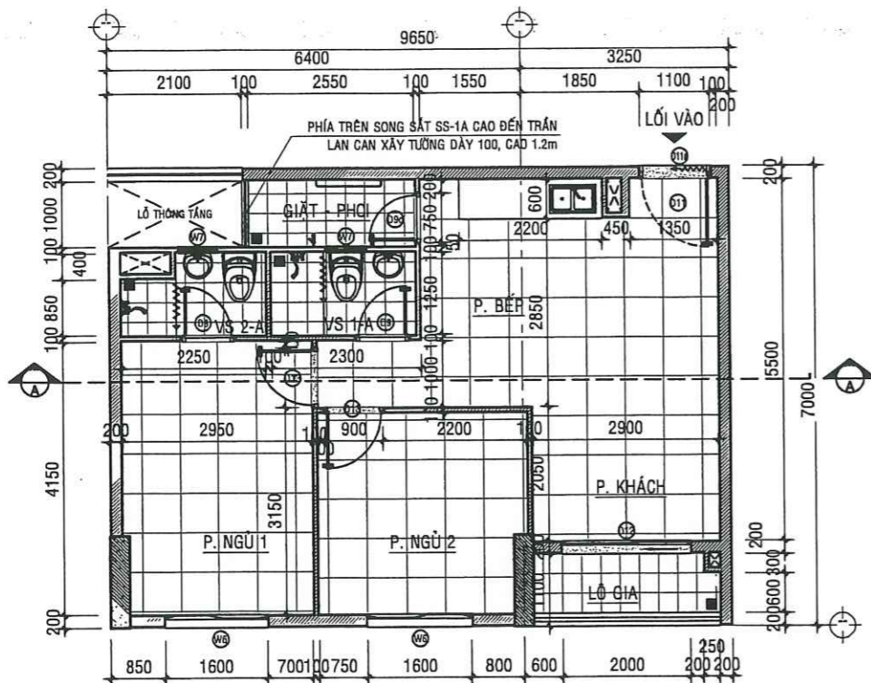
MẶT BẰNG HIỆN TRẠNG CĂN HỘ A - 15.05 - TL:1/50
