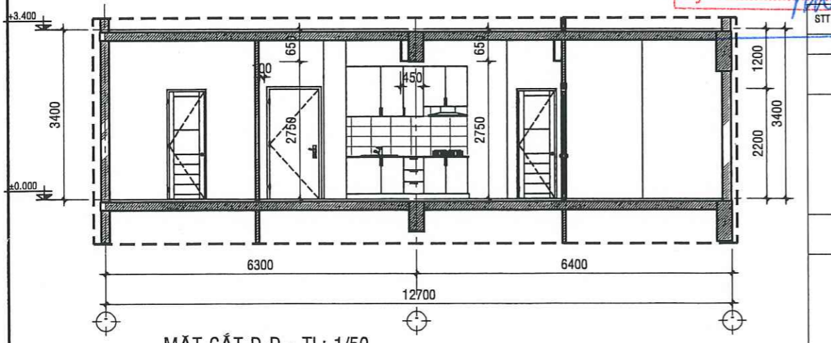
MẶT CẮT D-D - TL: 1/50
