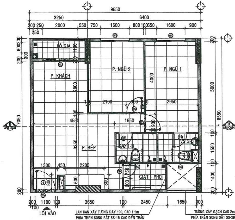
MẶT BẰNG HIỆN TRẠNG CĂN HỘ A -04.06 - TL:1/50
