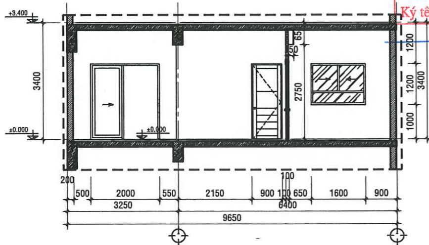
MẶT CẮT B-B - TL:1/50
