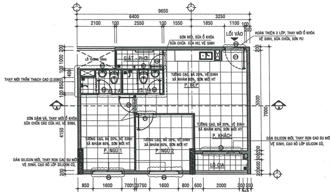
MẶT BẰNG SỬA CHỮA CĂN HỘ A -04.09 - TL:1/50
