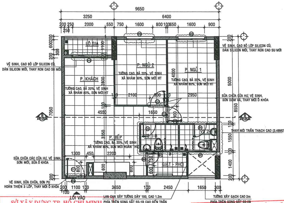
MẶT BẰNG SỬA CHỮA CĂN HỘ A -04.04 - TL:1/50
