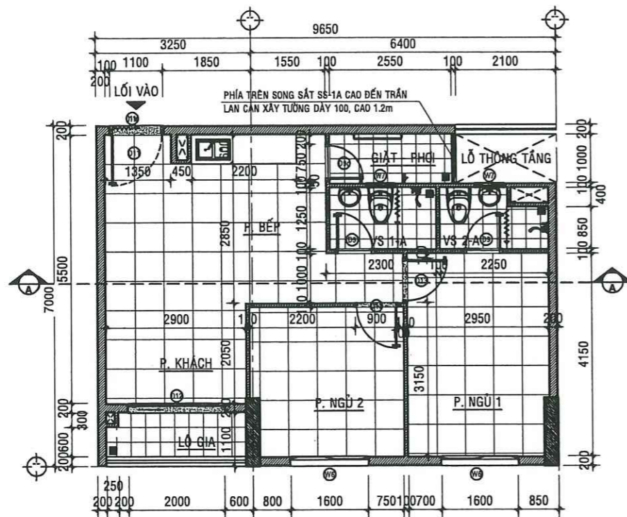
MẶT BẰNG HIỆN TRẠNG CĂN HỘ A - 09.01 - TL:1/50
