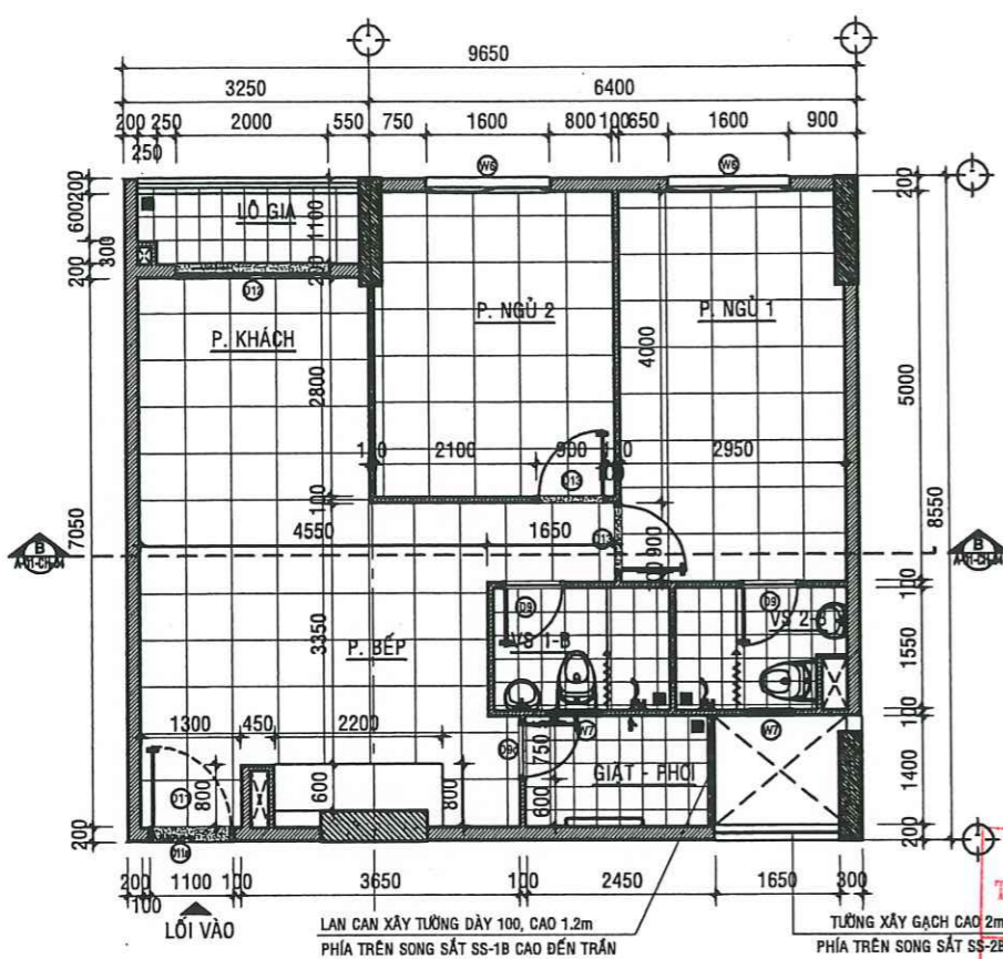
MẶT BẰNG HIỆN TRẠNG CĂN HỘ A - 10.06 - TL:1/50
