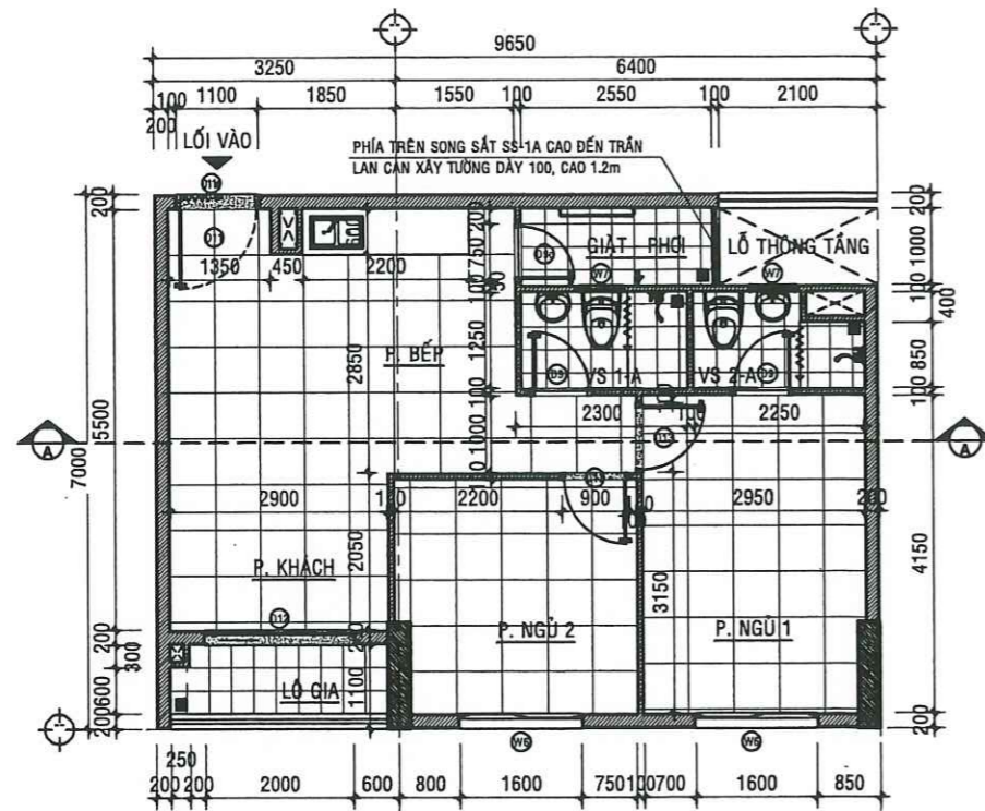
MẶT BẰNG HIỆN TRẠNG CĂN HỘ A - 08.08 - TL:1/50
