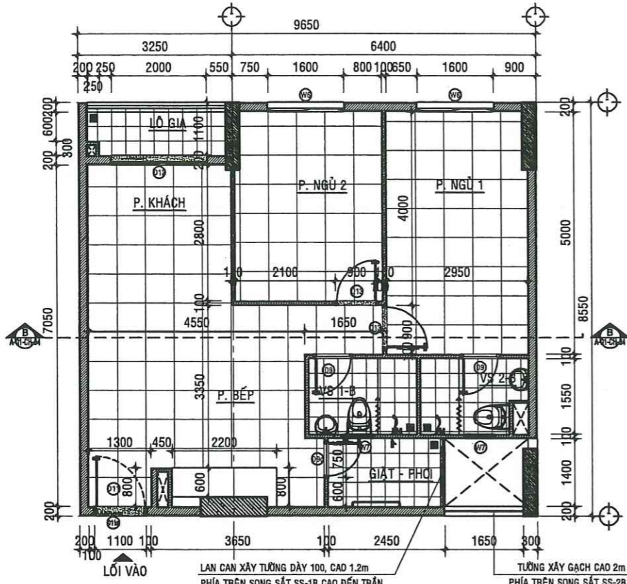
MẶT BẰNG HIỆN TRẠNG CĂN HỘ A -02.06 - TL:1/50
