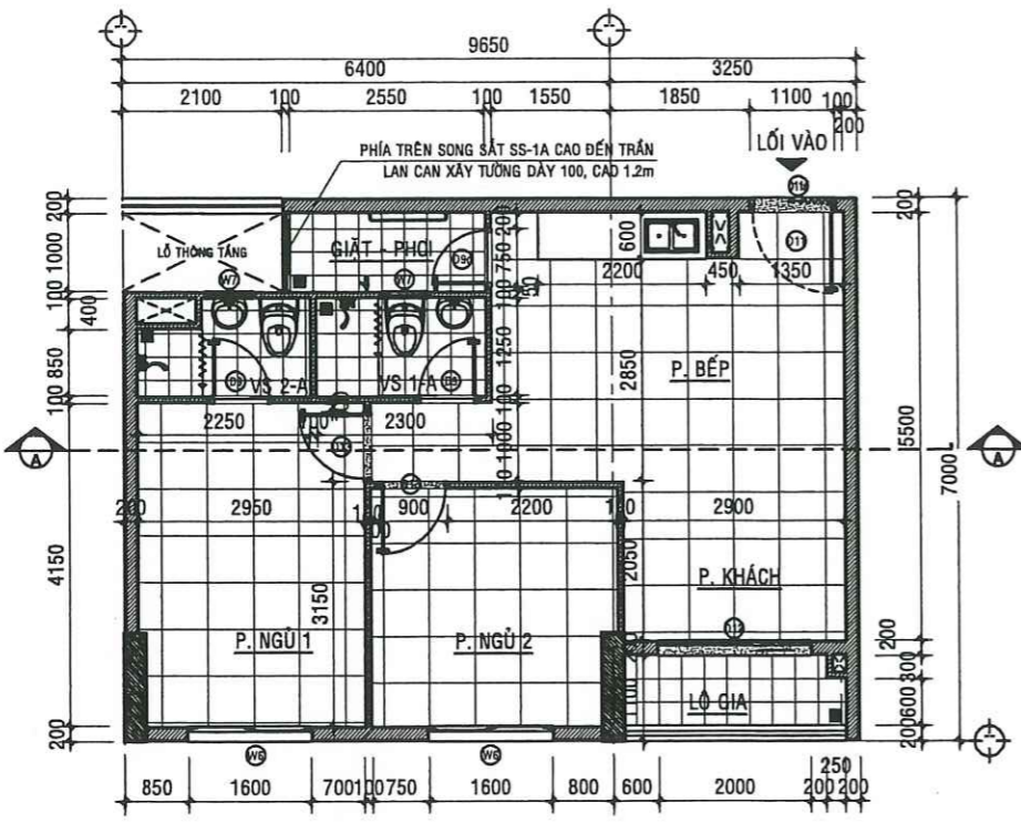
MẶT BẰNG HIỆN TRẠNG CĂN HỘ A - 10.09 - TL:1/50
