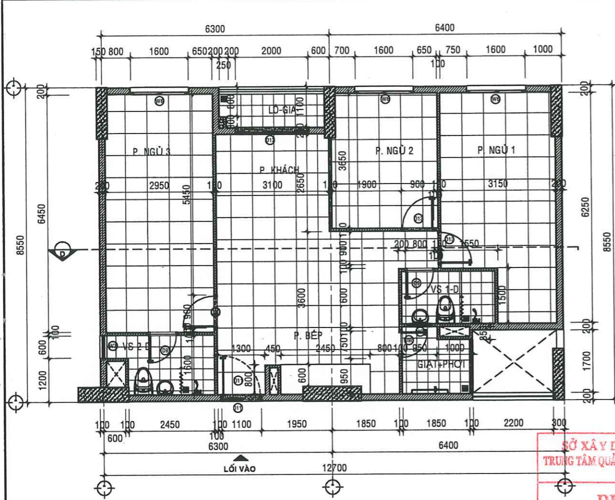
MẶT BẰNG HIỆN TRẠNG CĂN HỘ A - 11.07 - TL: 1/50
