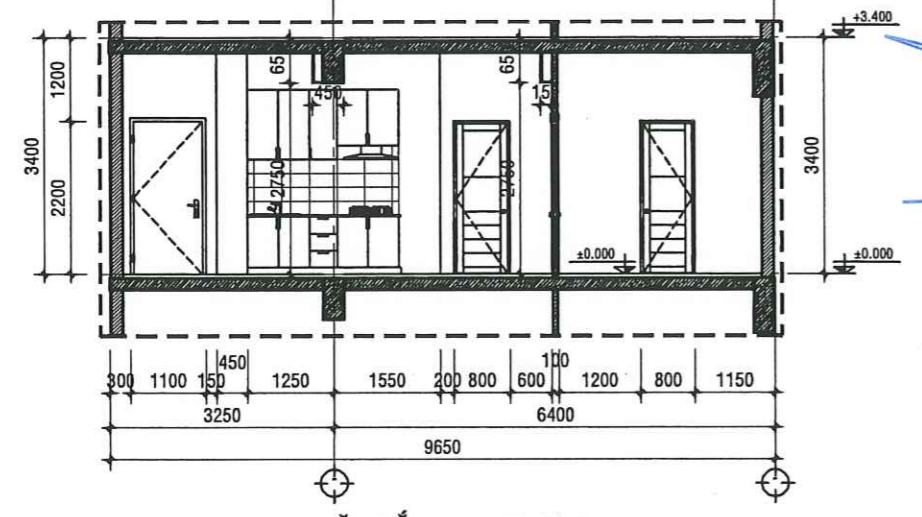
MẶT CẮT A-A - TL:1/50
