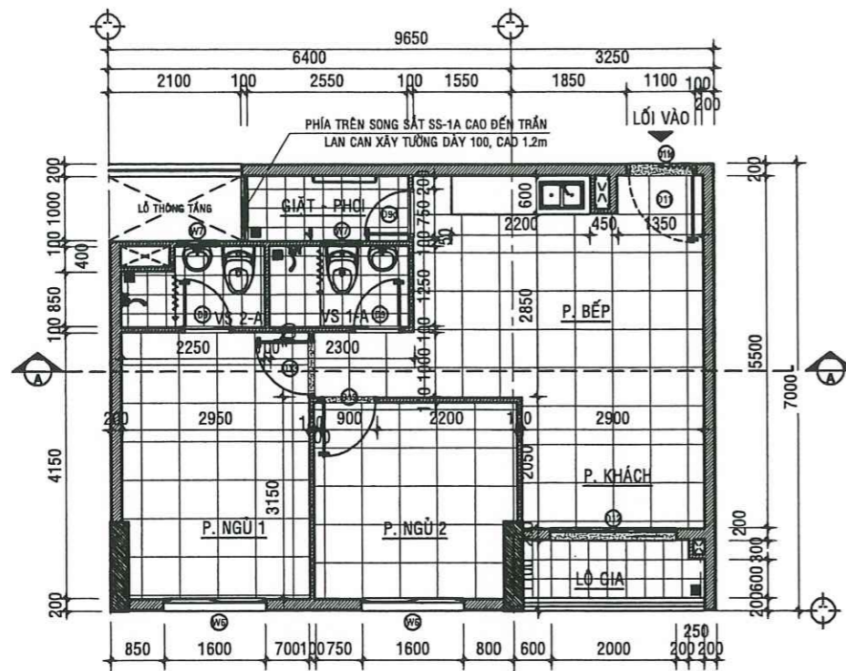
MẶT BẰNG HIỆN TRẠNG CĂN HỘ A - 06.09 - TL:1/50
