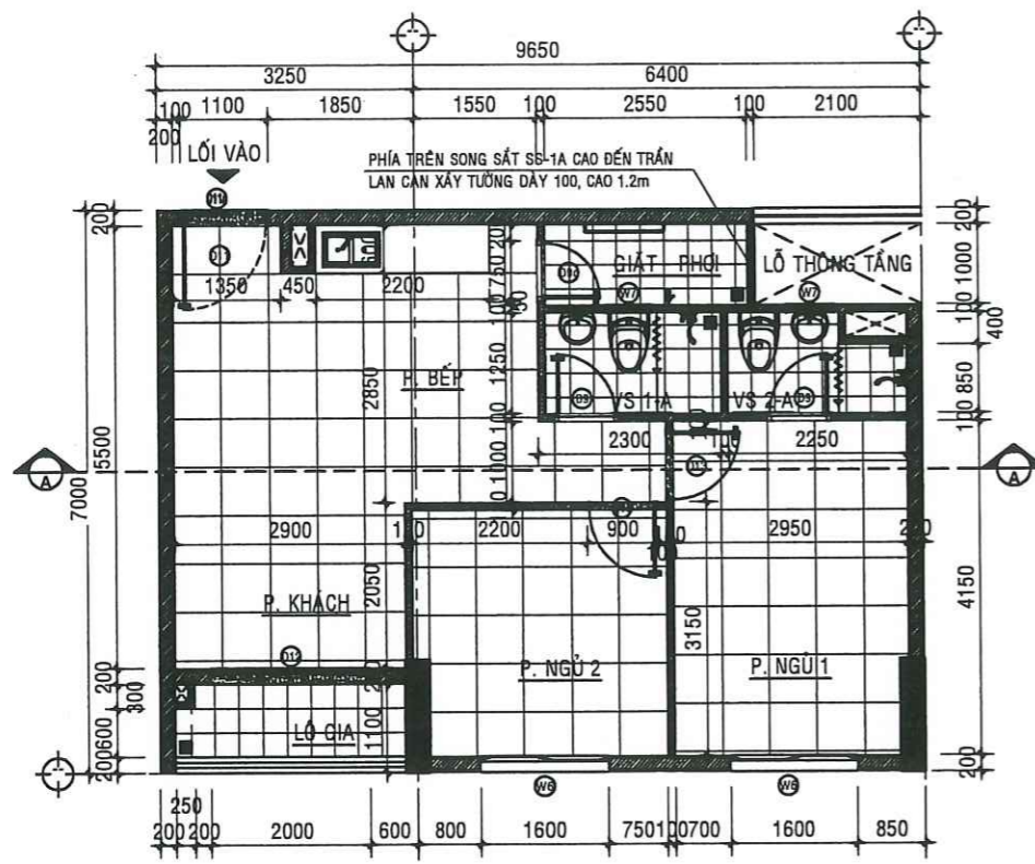
MẶT BẰNG HIỆN TRẠNG CĂN HỘ A - 11.08 - TL:1/50
