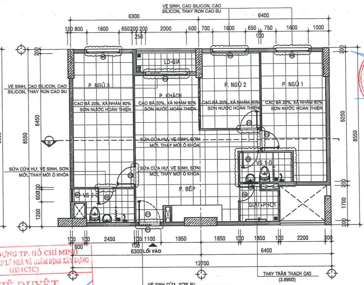
MẶT BẰNG SỬA CHỮA CĂN HỘ A - 14.07 - TL: 1/50
