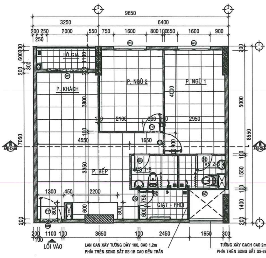
MẶT BẰNG HIỆN TRẠNG CĂN HỘ A -01.02 - TL:1/50
