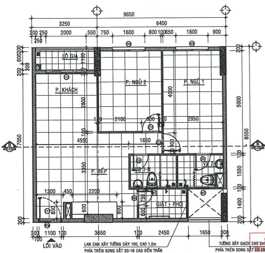
MẶT BẰNG HIỆN TRẠNG CĂN HỘ A - 08.06 - TL:1/50
