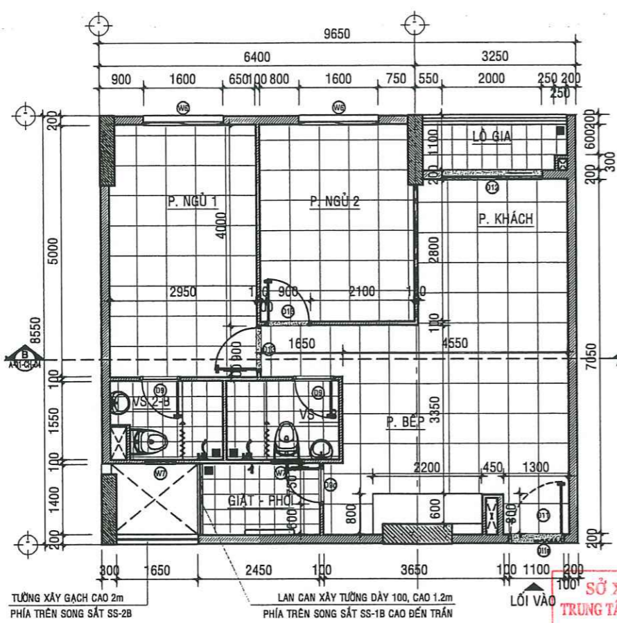
MẶT BẰNG HIỆN TRẠNG CĂN HỘ A - 15.01 - TL:1/50
