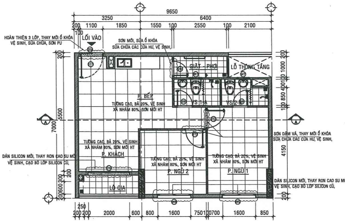
MẶT BẰNG SỬA CHỮA CĂN HỘ A - 06.01 - TL:1/50
