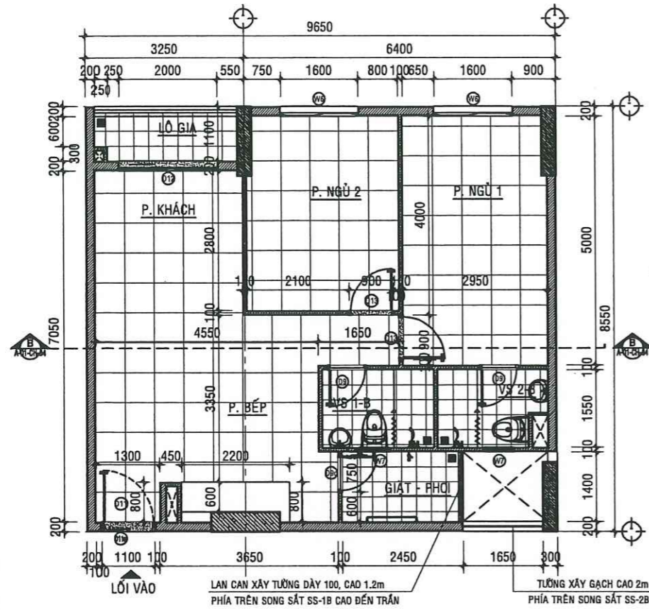
MẶT BẰNG HIỆN TRẠNG CĂN HỘ A - 05.04 - TL:1/50
