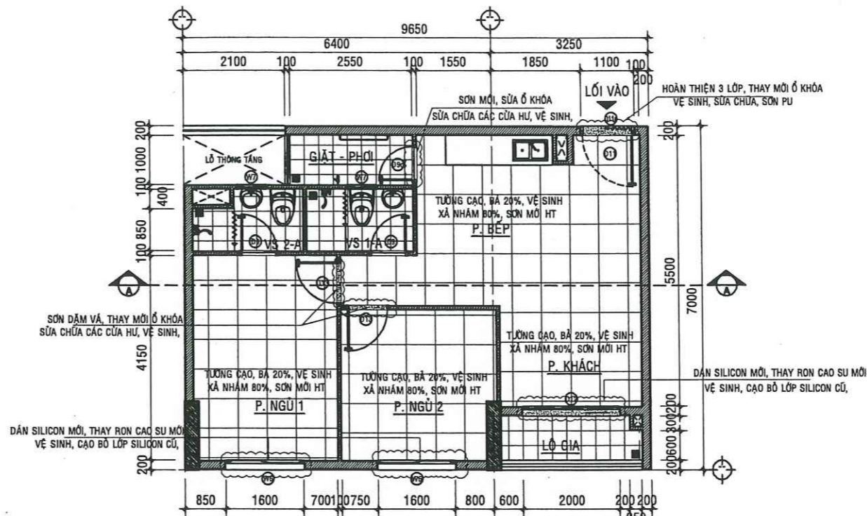
MẶT BẰNG SỬA CHỮA CĂN HỘ A - 06.09 - TL:1/50
