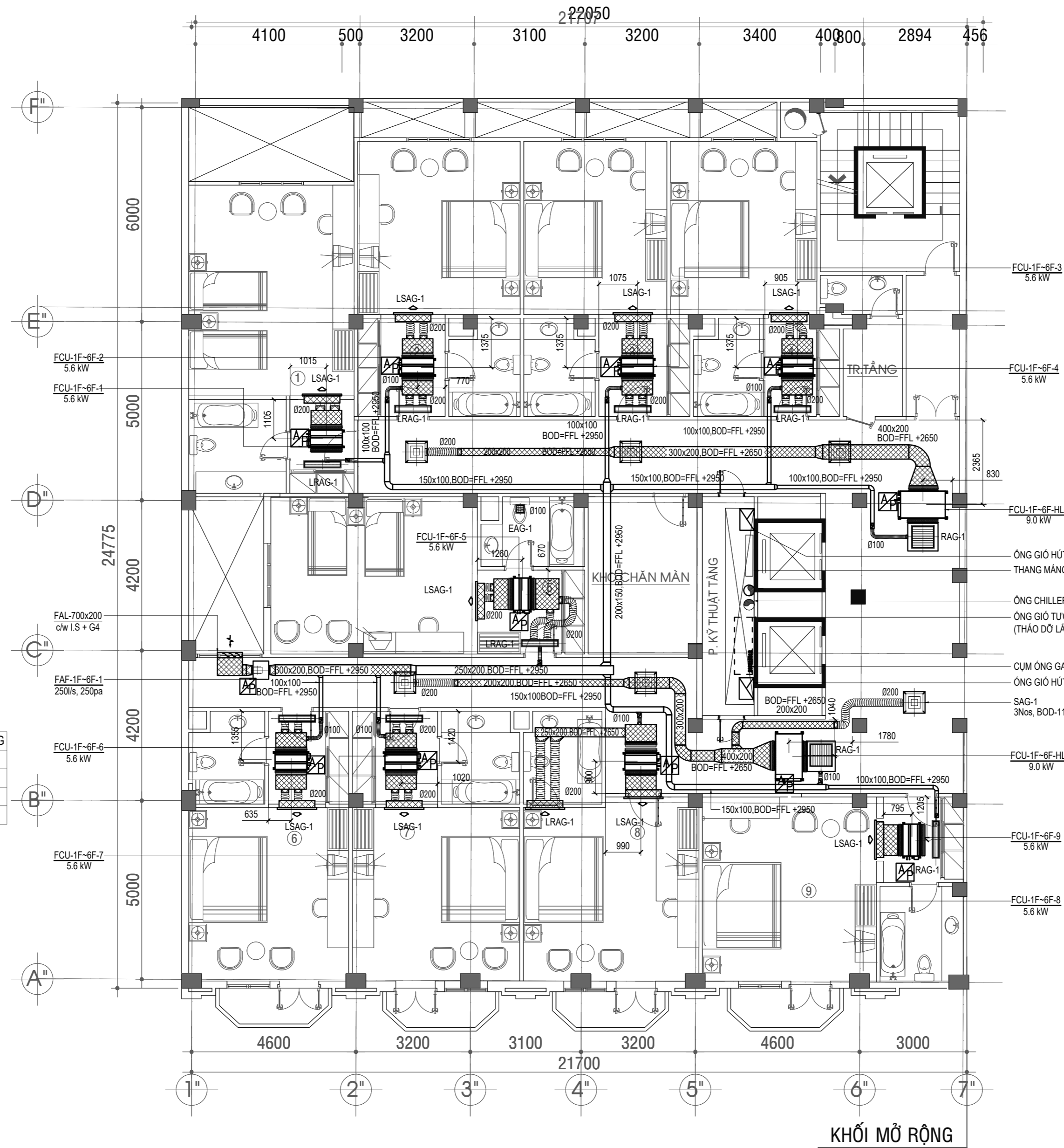
MẶT BẰNG CẢI TẠO ĐHKK & THÔNG GIÓ LẦU 1 ~ LẦU 6 TL: 1/100
