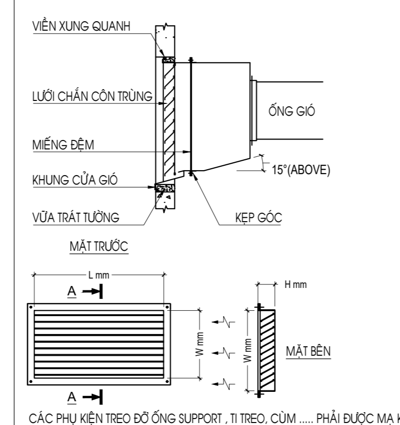
CHI TIẾT LẮP ĐẶT LOUVER
