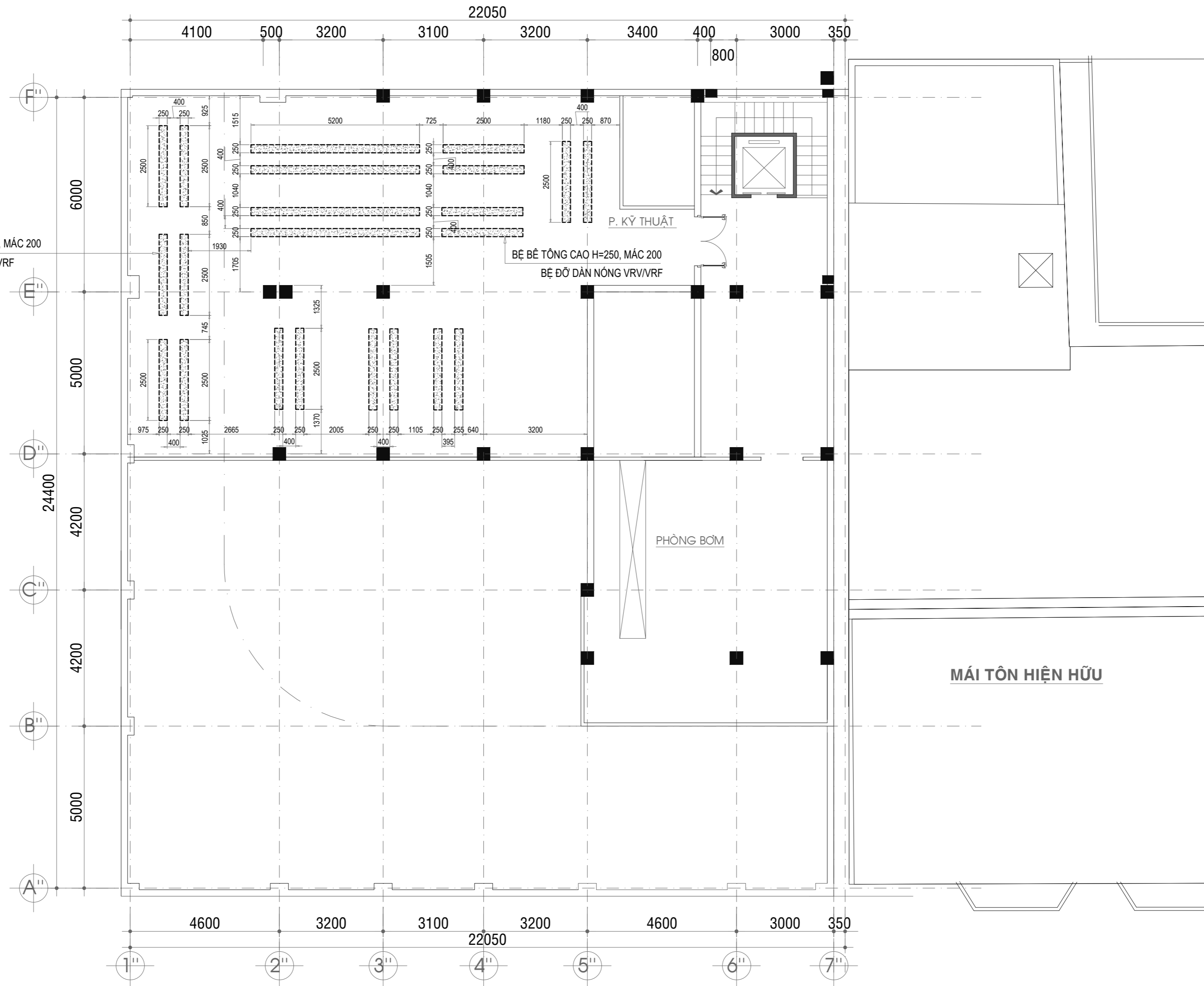
MẶT BẰNG BỐ TRÍ BỆ ĐỠ DÀN NÓNG TẦNG KỸ THUẬT TL: 1/100
