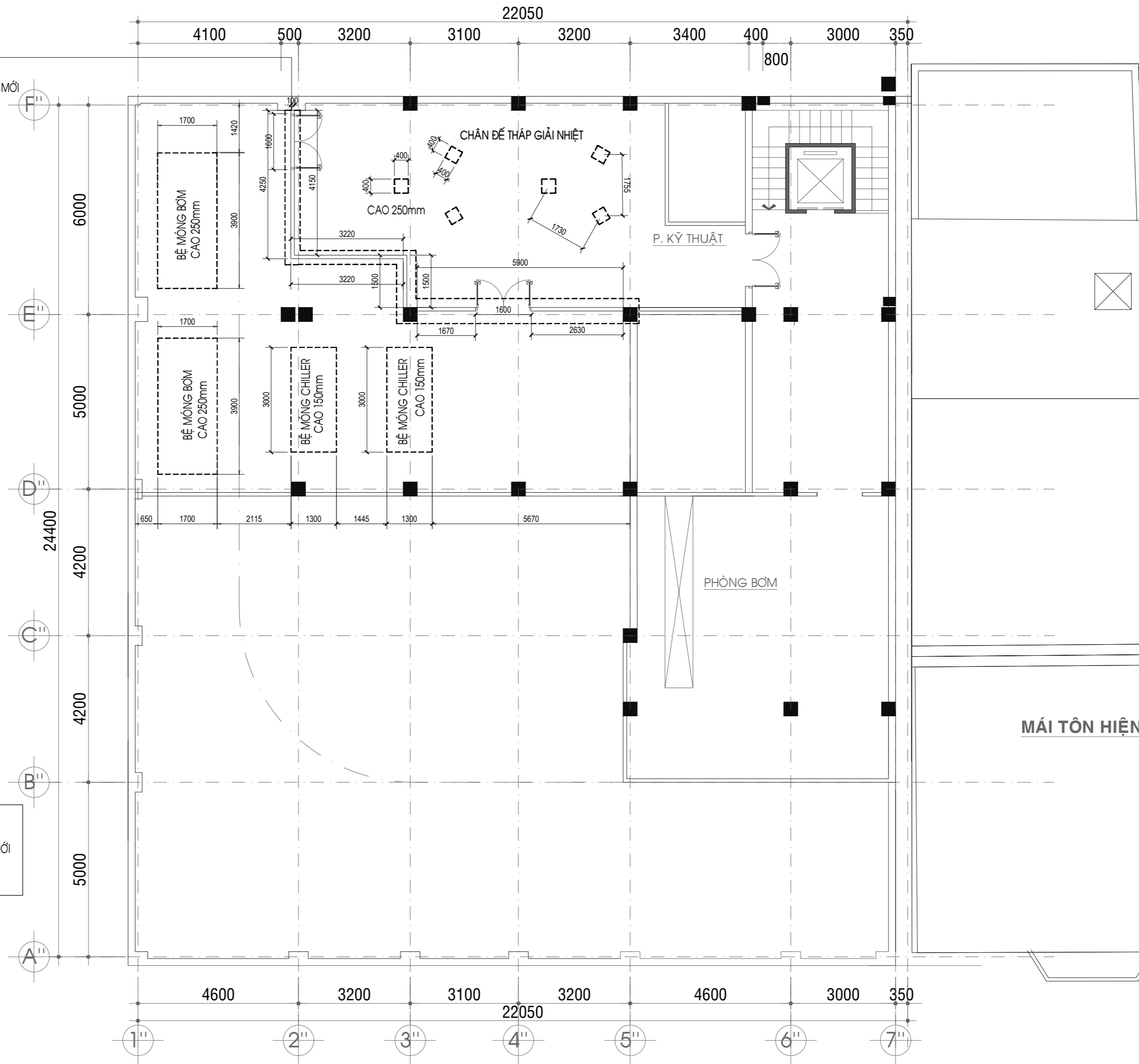
MẶT BẰNG THÁO DỠ TẦNG KỸ THUẬT TL: 1/100
