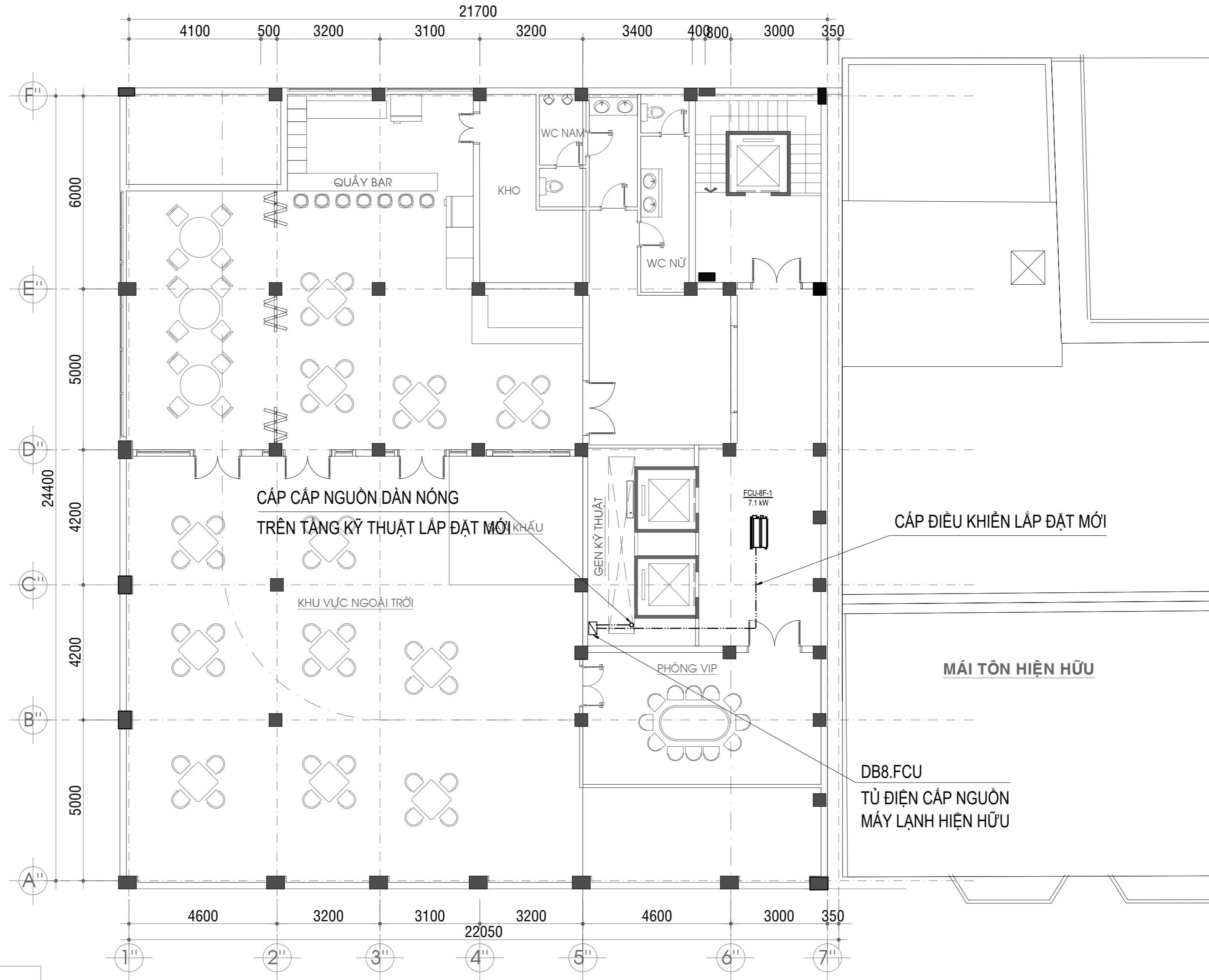
MẶT BẰNG CẤP NGUỒN ĐHKK & THÔNG GIÓ LẦU 8 TL: 1/100
