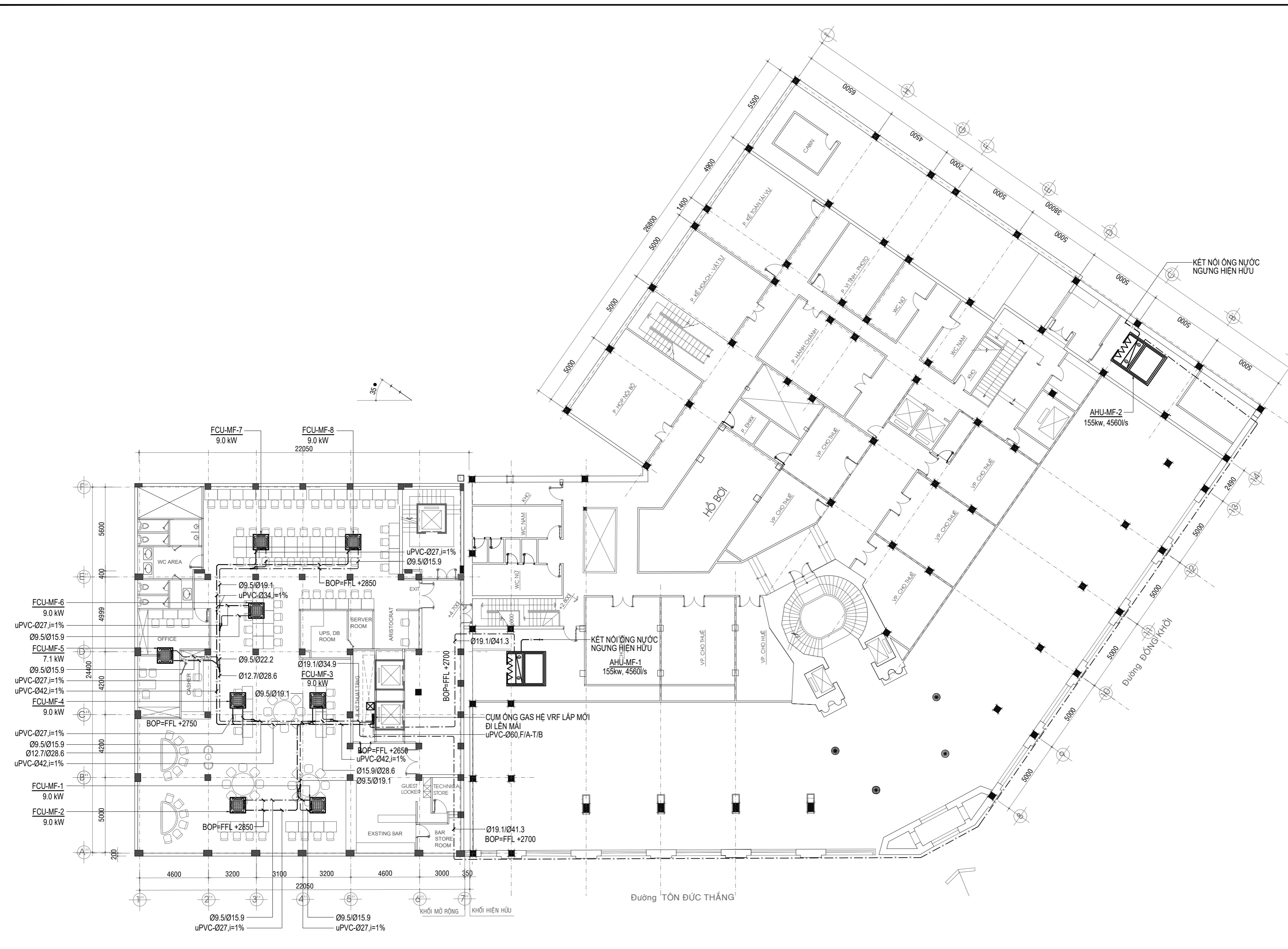
MẶT BẰNG CẢI TẠO ỚNG GAS, ỚNG NƯỚC NGƯNG TẦNG LỬNG TL: 1/200
