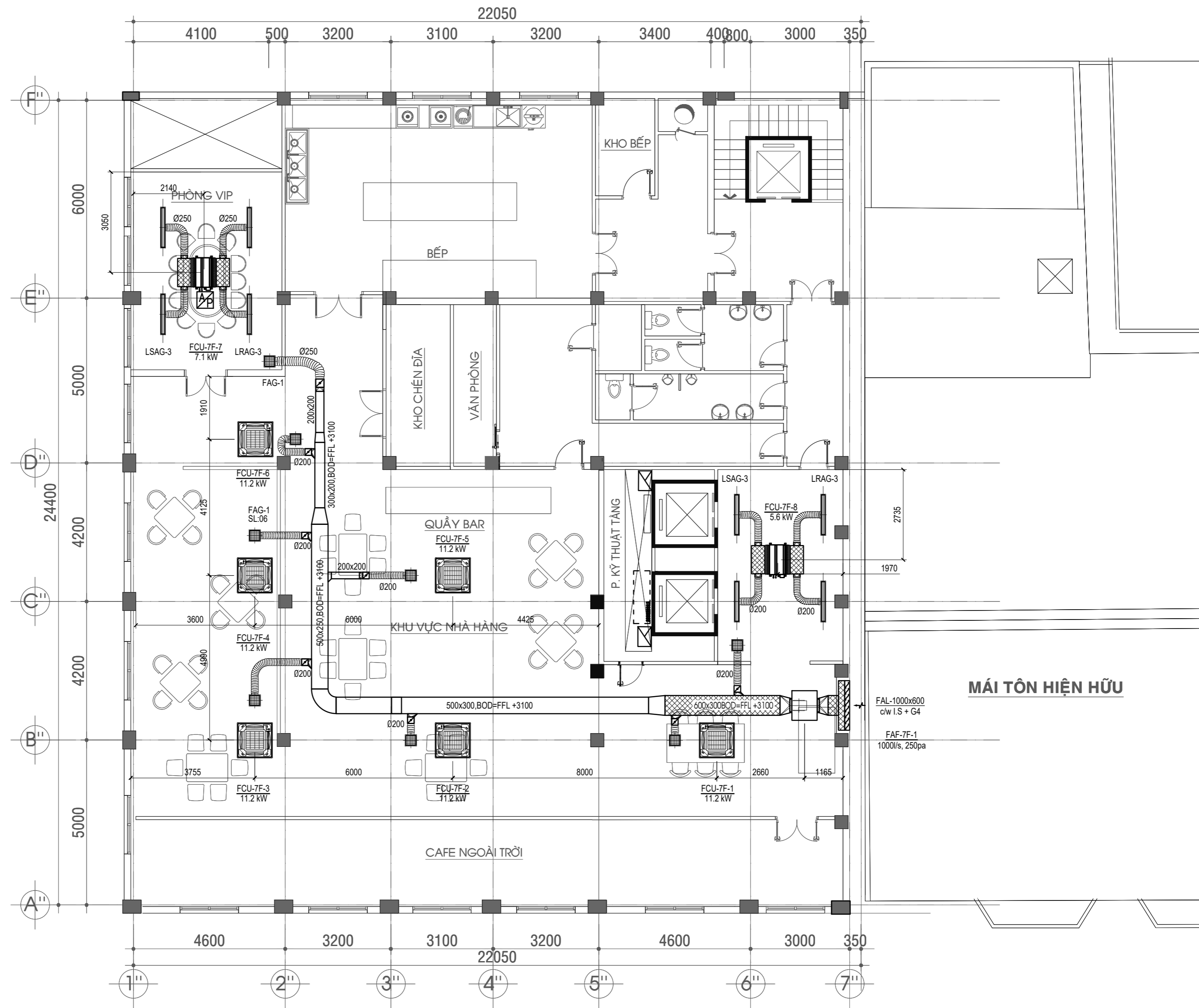
MẶT BẰNG CẢI TẠO ĐHKK & THÔNG GIÓ LẦU 7 TL: 1/100
