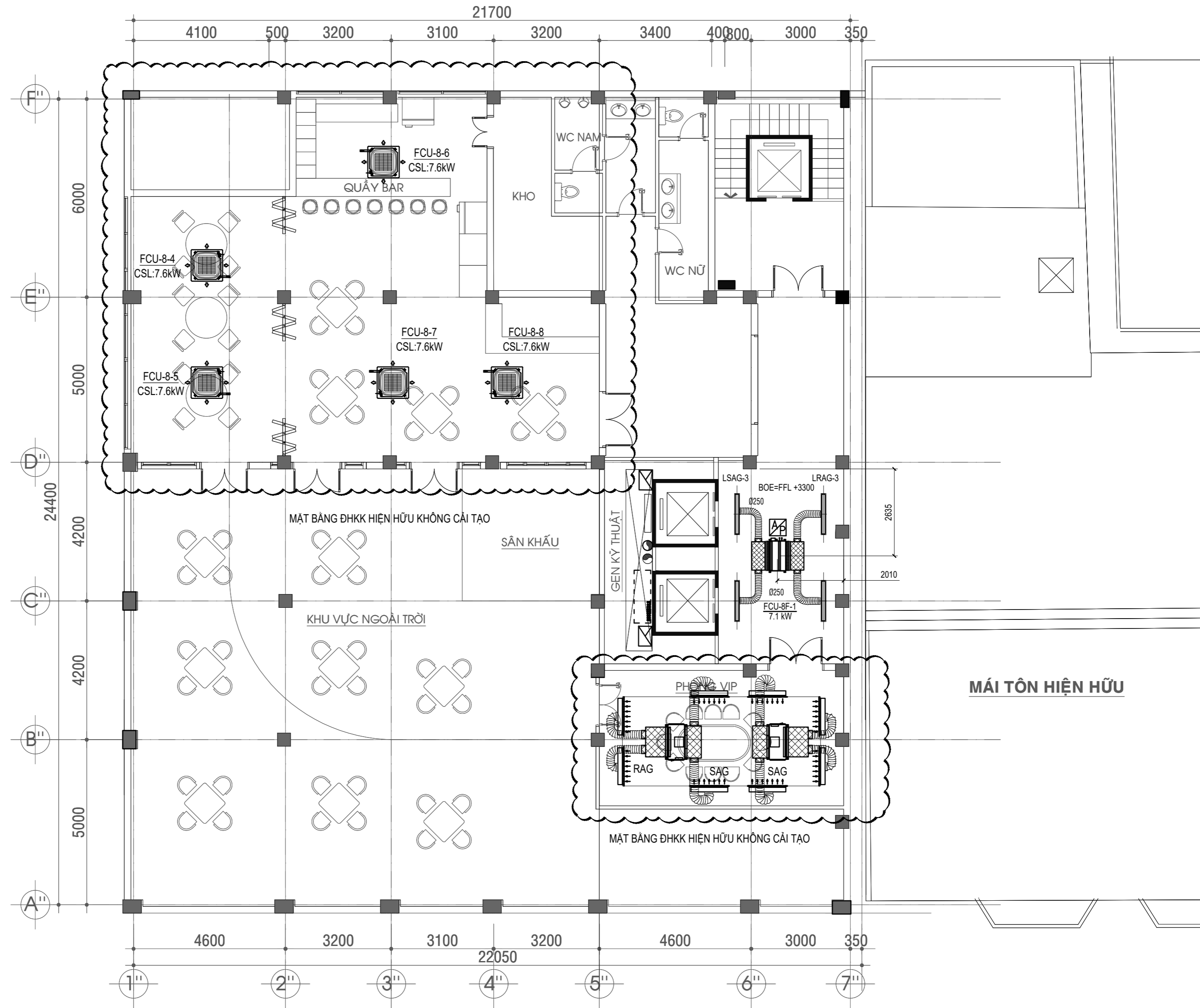
MẶT BẰNG CẢI TẠO ĐHKK & THÔNG GIÓ LẦU 8 TL: 1/100
