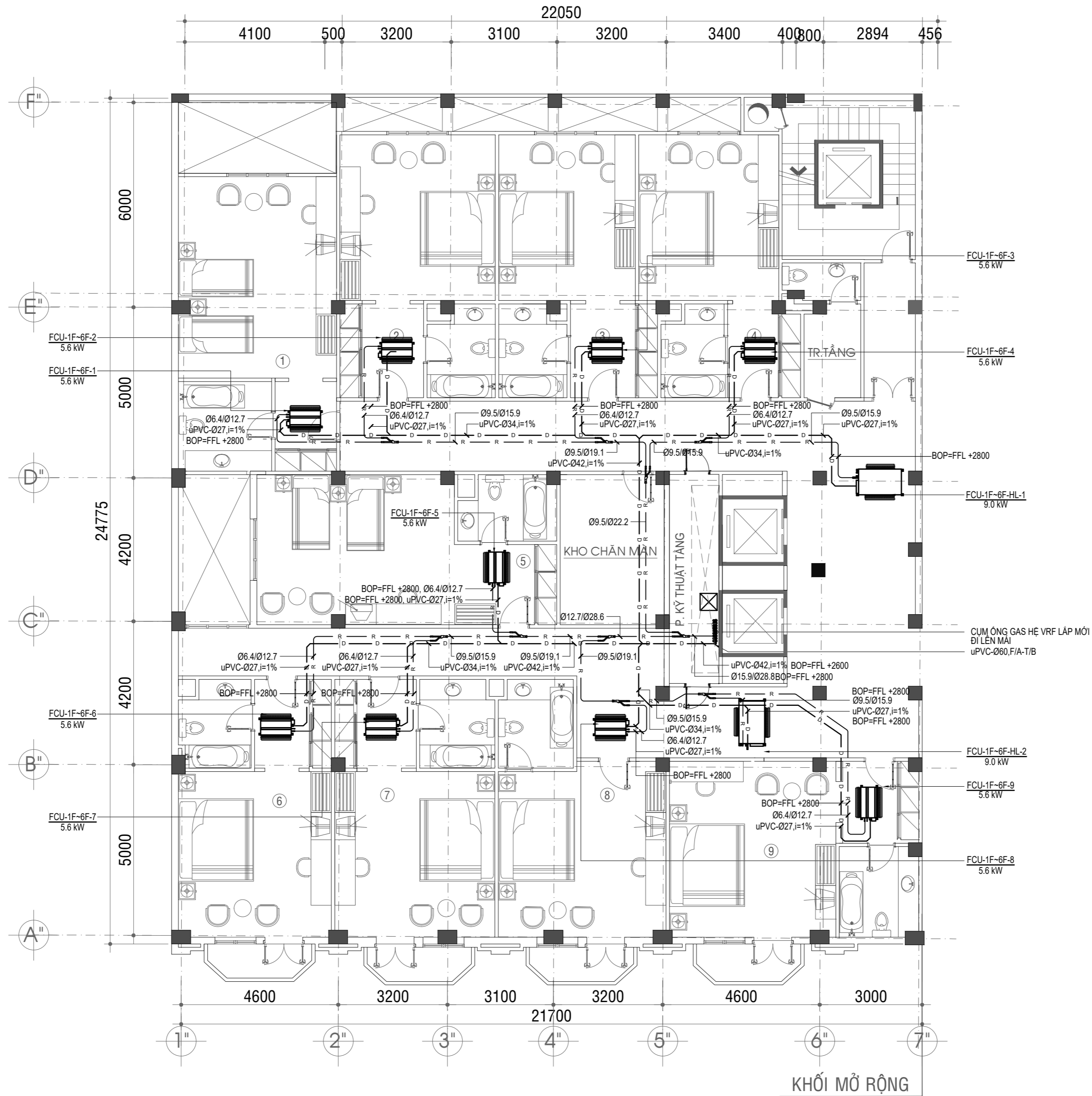
MẶT BẰNG CẢI TẠO ỚNG GAS, ỚNG NƯỚC NGƯNG LẦU 1~ LẦU 6 TL: 1/100
