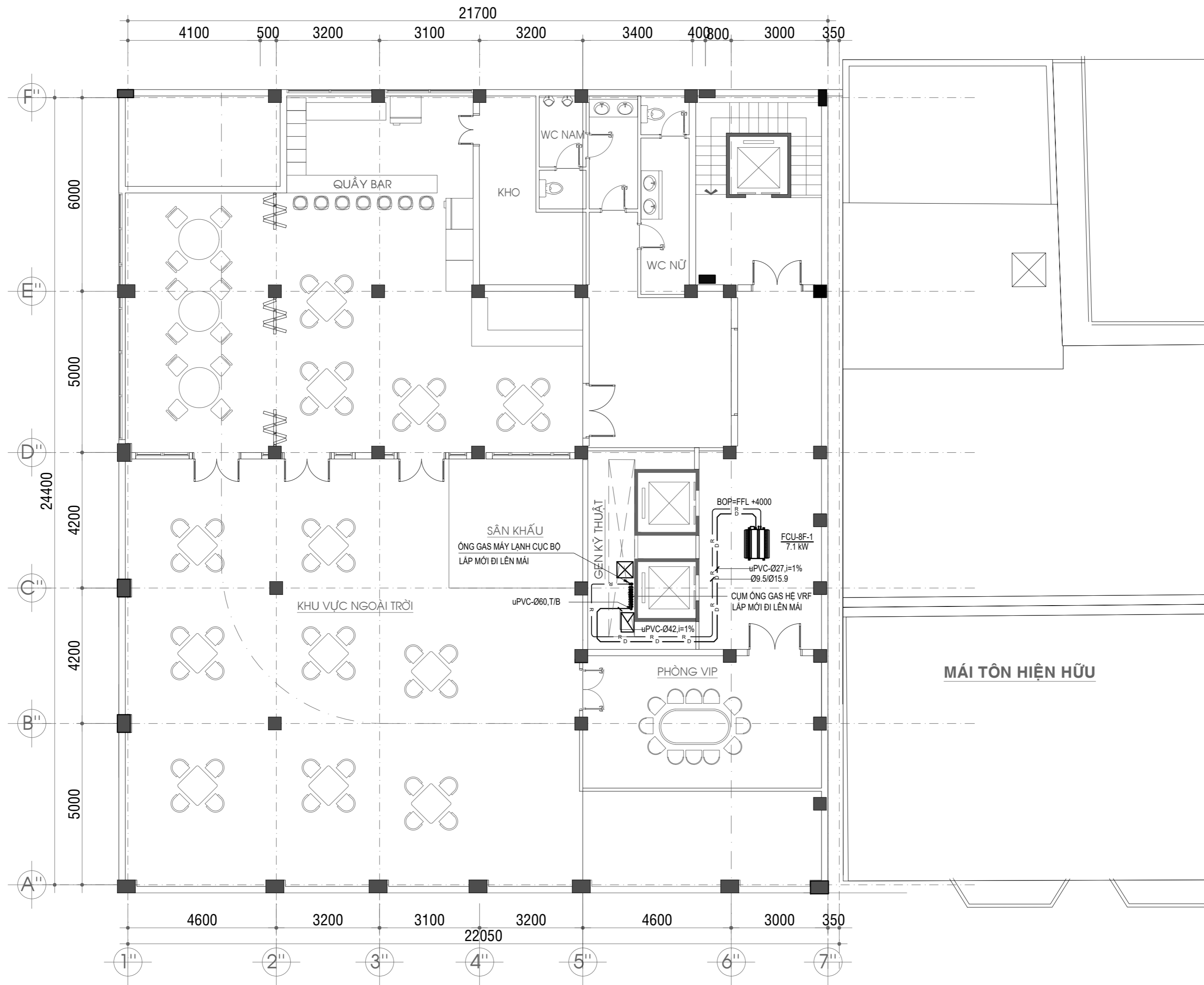
MẶT BẰNG CẢI TẠO ỚNG GAS, ỚNG NƯỚC NGƯNG LẦU 8 TL: 1/100
