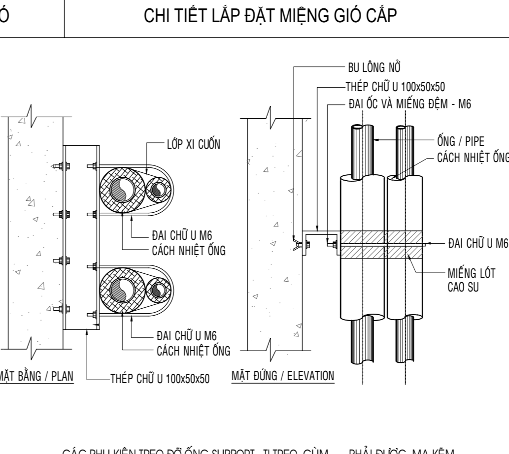
CHI TIẾT TREO ỚNG GAS TRỰC ĐỨNG
