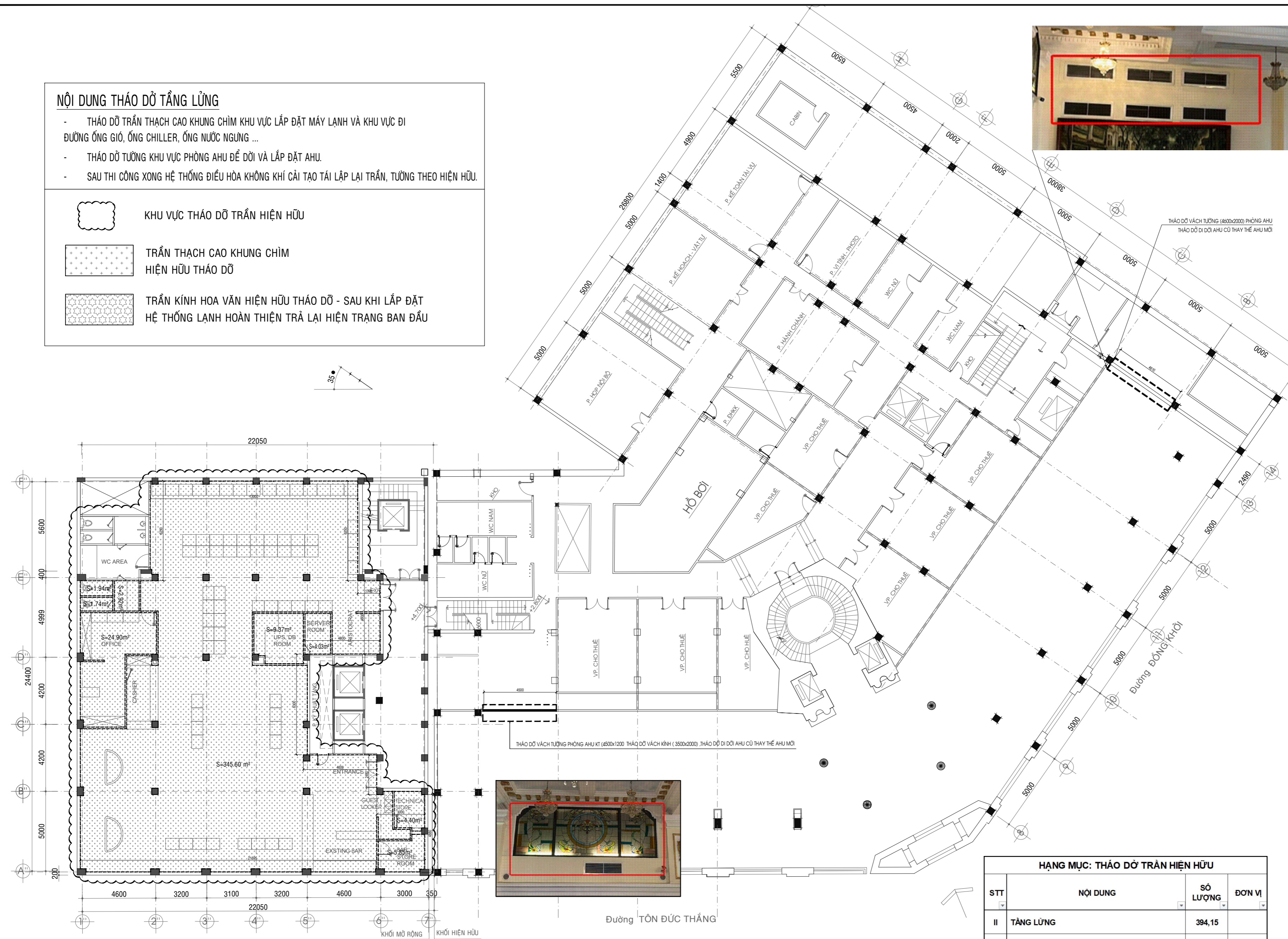
MẶT BẰNG THÁO DỠ TẦNG LỬNG TL: 1/100
