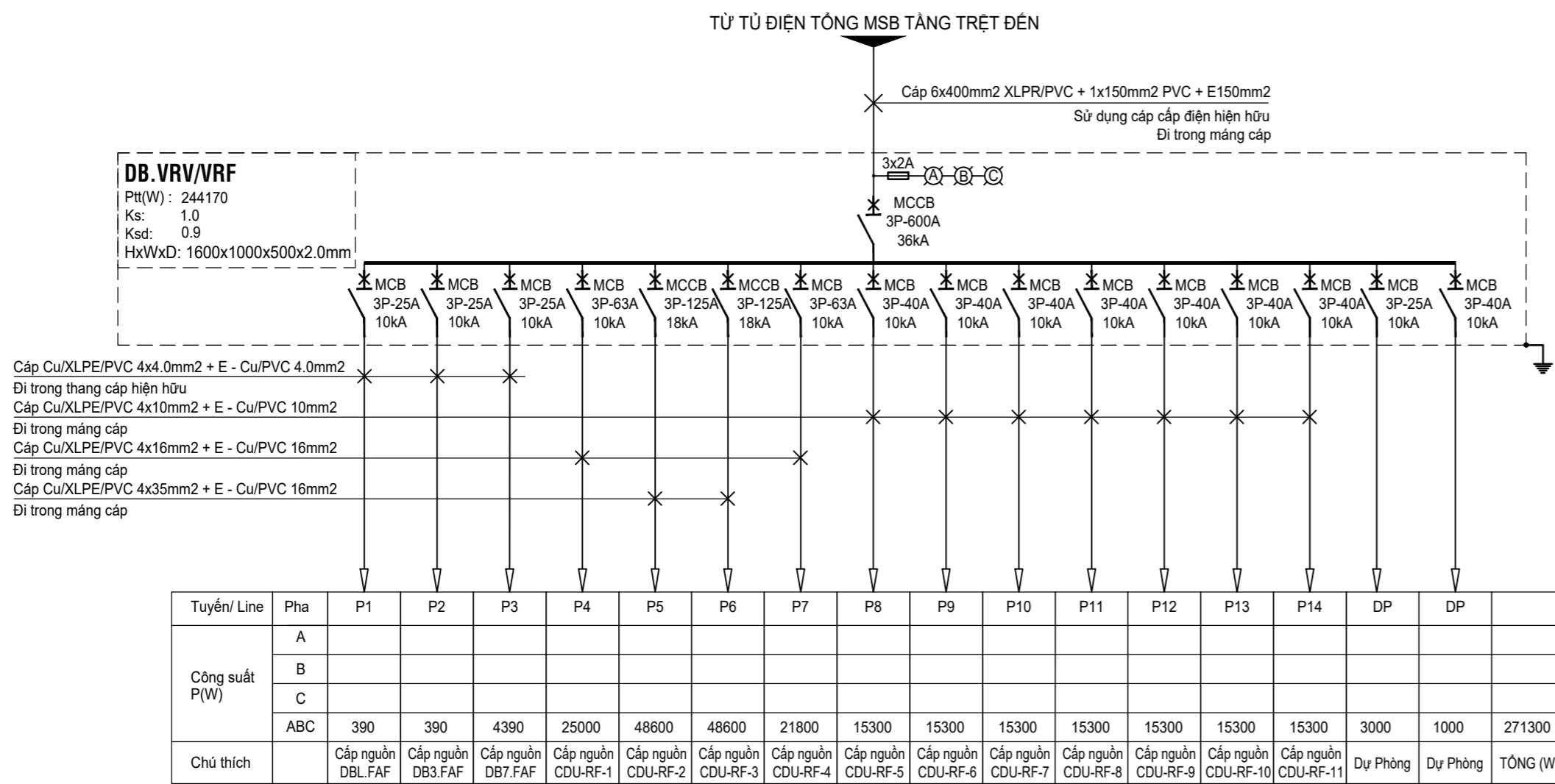
SƠ ĐỒ NGUYÊN LÝ TỦ ĐIỆN CHÍNH ĐHKK & THÔNG GIÓ (DB.VRV/VRF)
