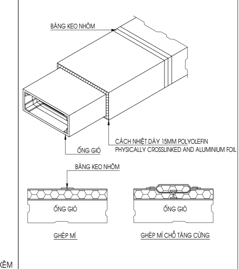
CHI TIẾT CÁCH NHIỆT ỚNG GIÓ
