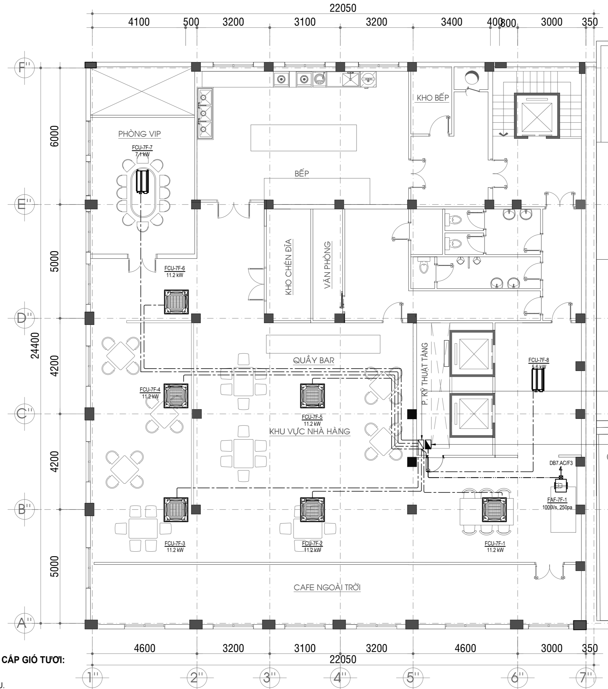
MẶT BẰNG CÁP NGUỒN ĐHKK & THÔNG GIÓ LẦU 7 TL: 1/100
