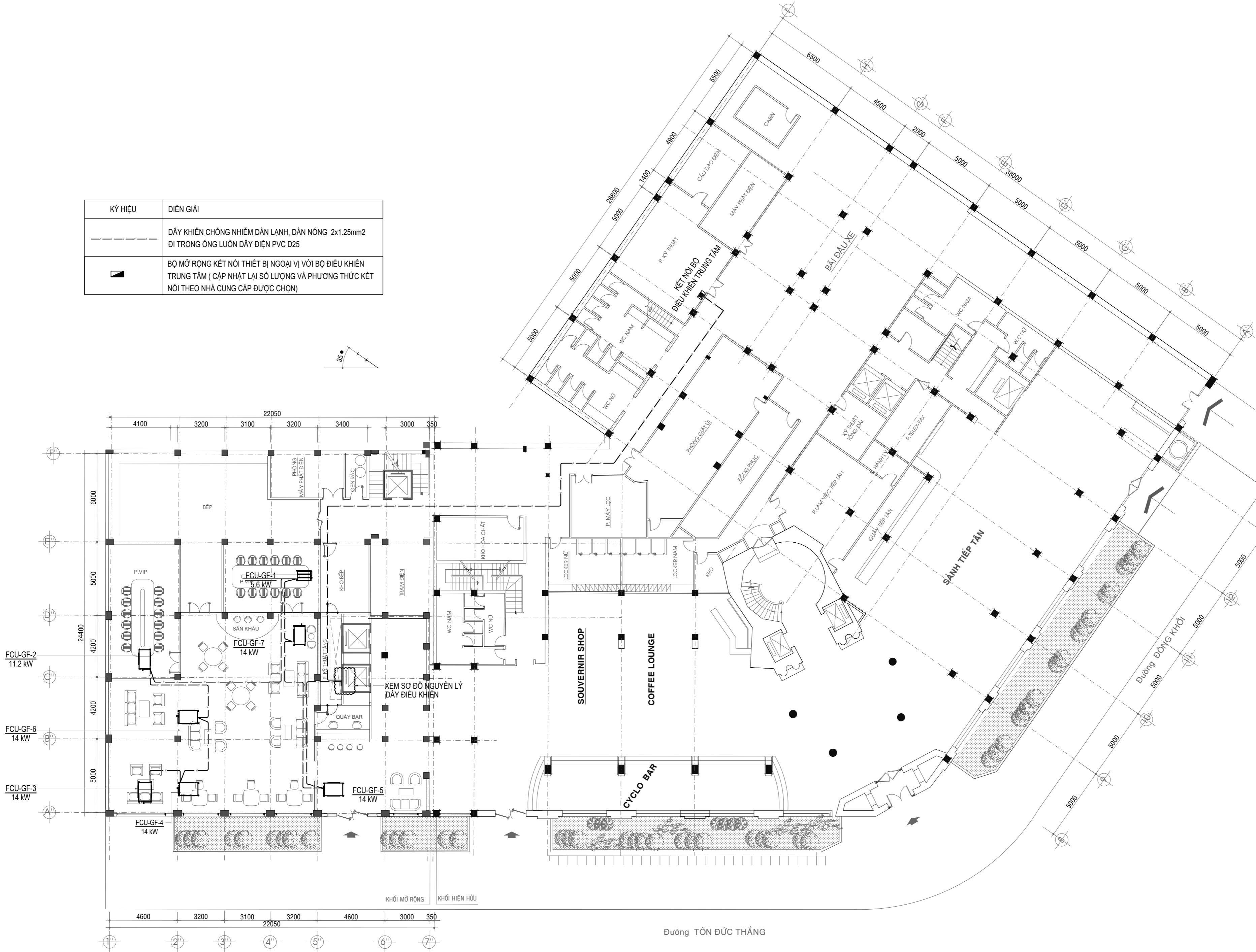
MẶT BẰNG CẢI TẠO DÂY ĐIỀU KHIỂN TẦNG TRỆT TL: 1/100
