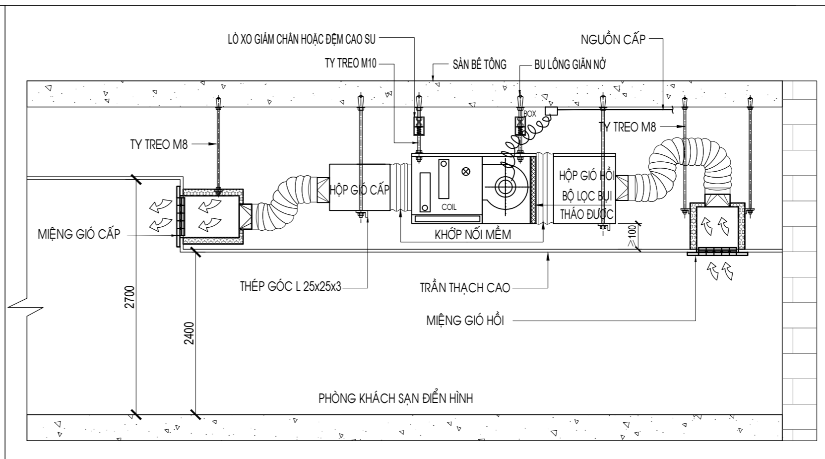
CHI TIẾT LẮP ĐẶT MIỆNG GIÓ PHÒNG KHÁCH SẠN ĐIỆN HÌNH
