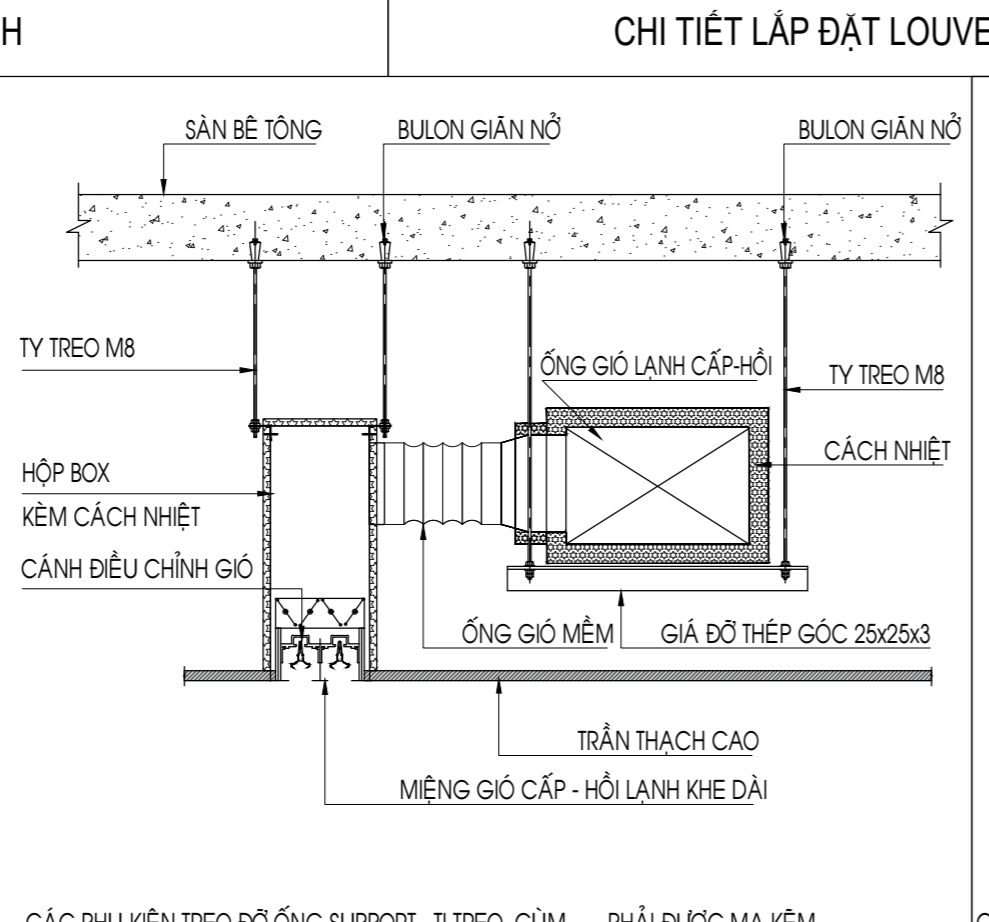
CHI TIẾT LẮP ĐẶT MIỆNG GIÓ CẤP- HỒI LẠNH KHE DÀI
