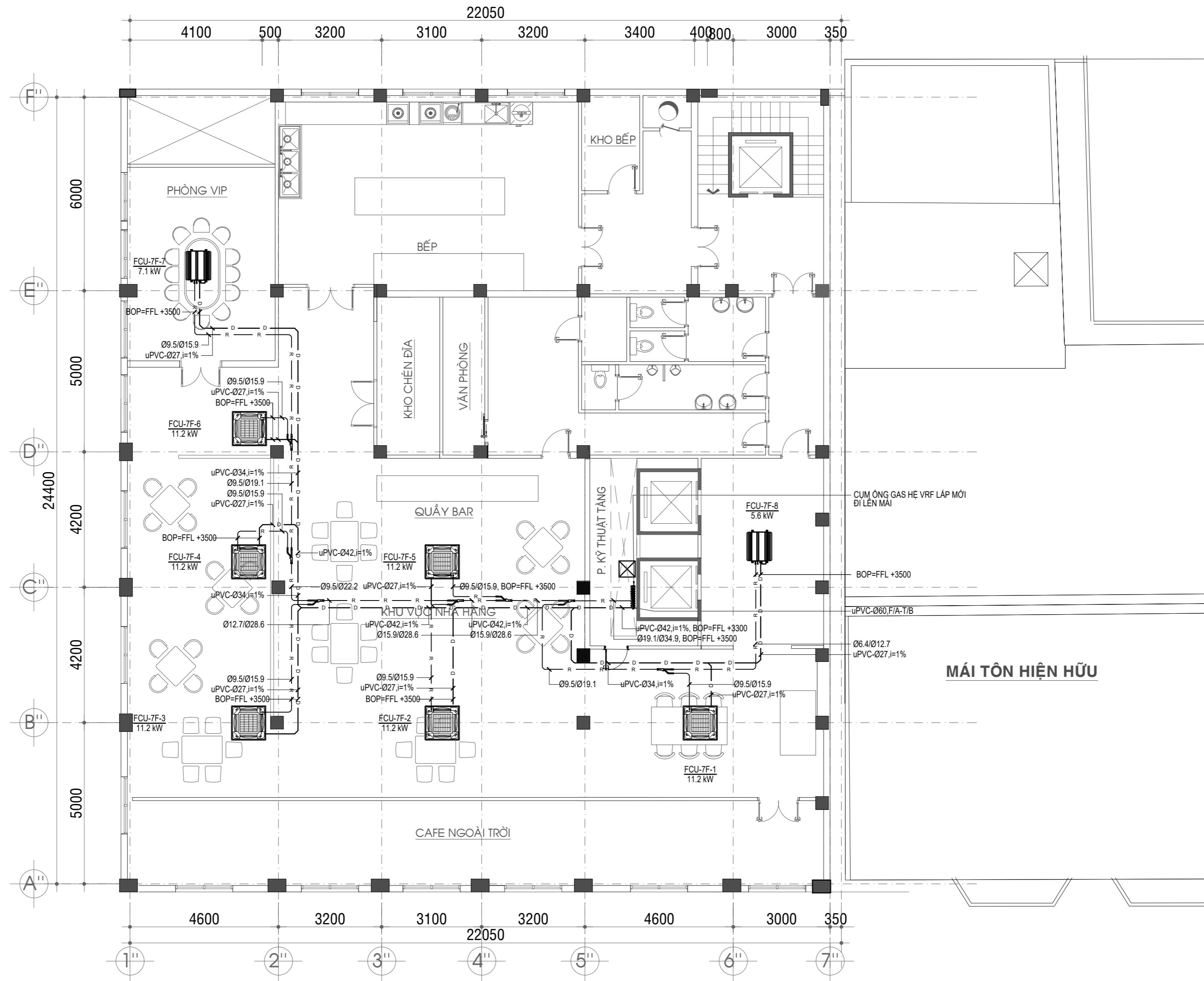
MẶT BẰNG CẢI TẠO ỚNG GAS, ỚNG NƯỚC NGƯNG LẦU 7 TL: 1/100
