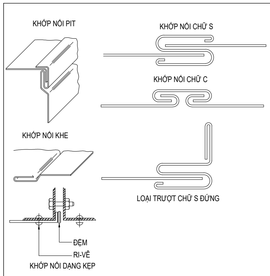
CHI TIẾT KHỚP NỐI
