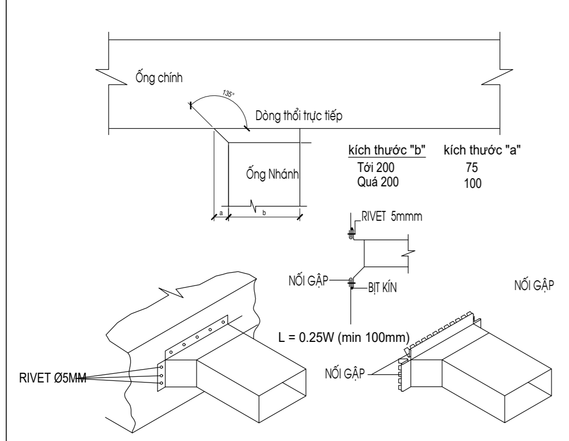
CHI TIẾT ỚNG GIÓ NHÁNH
