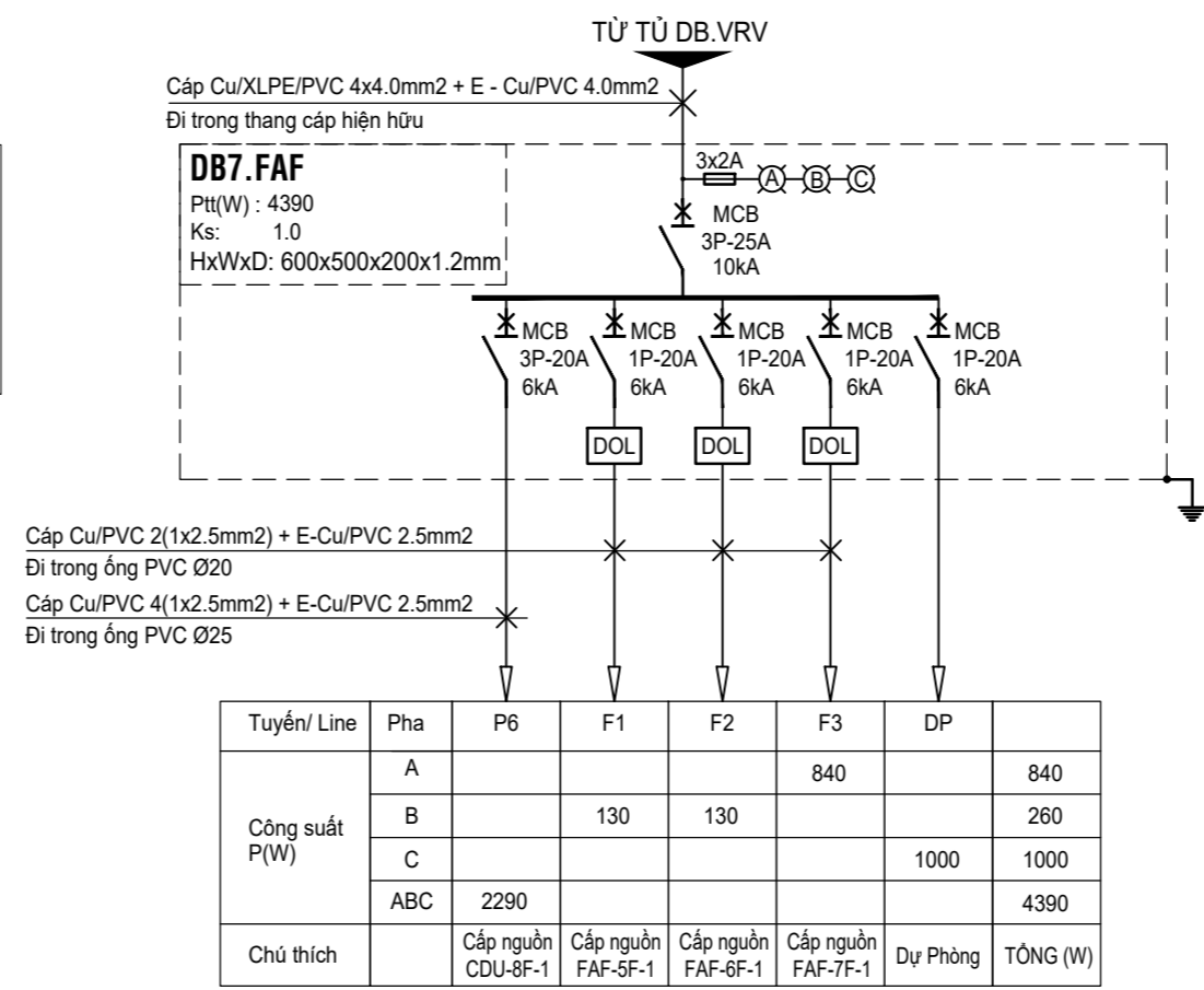
SƠ ĐỒ NGUYÊN LÝ TỦ ĐIỆN PHÂN PHỐI (DB7.FAF)
