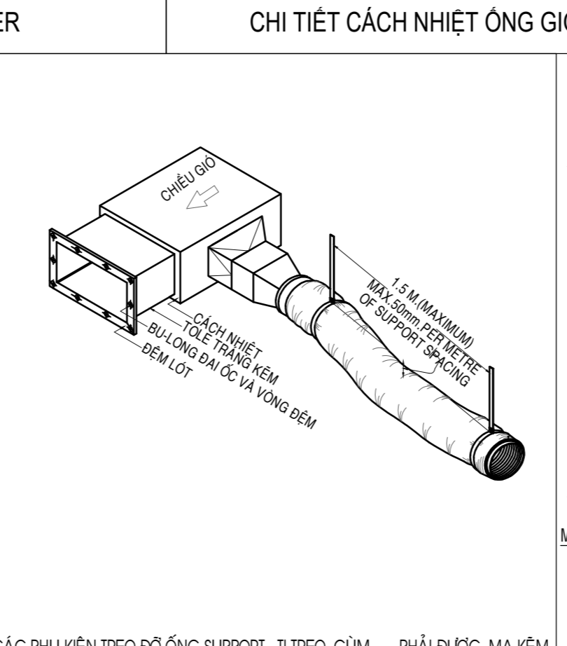
CHI TIẾT ỚNG NỐI MỀM VÀ RẺ NHÁNH
