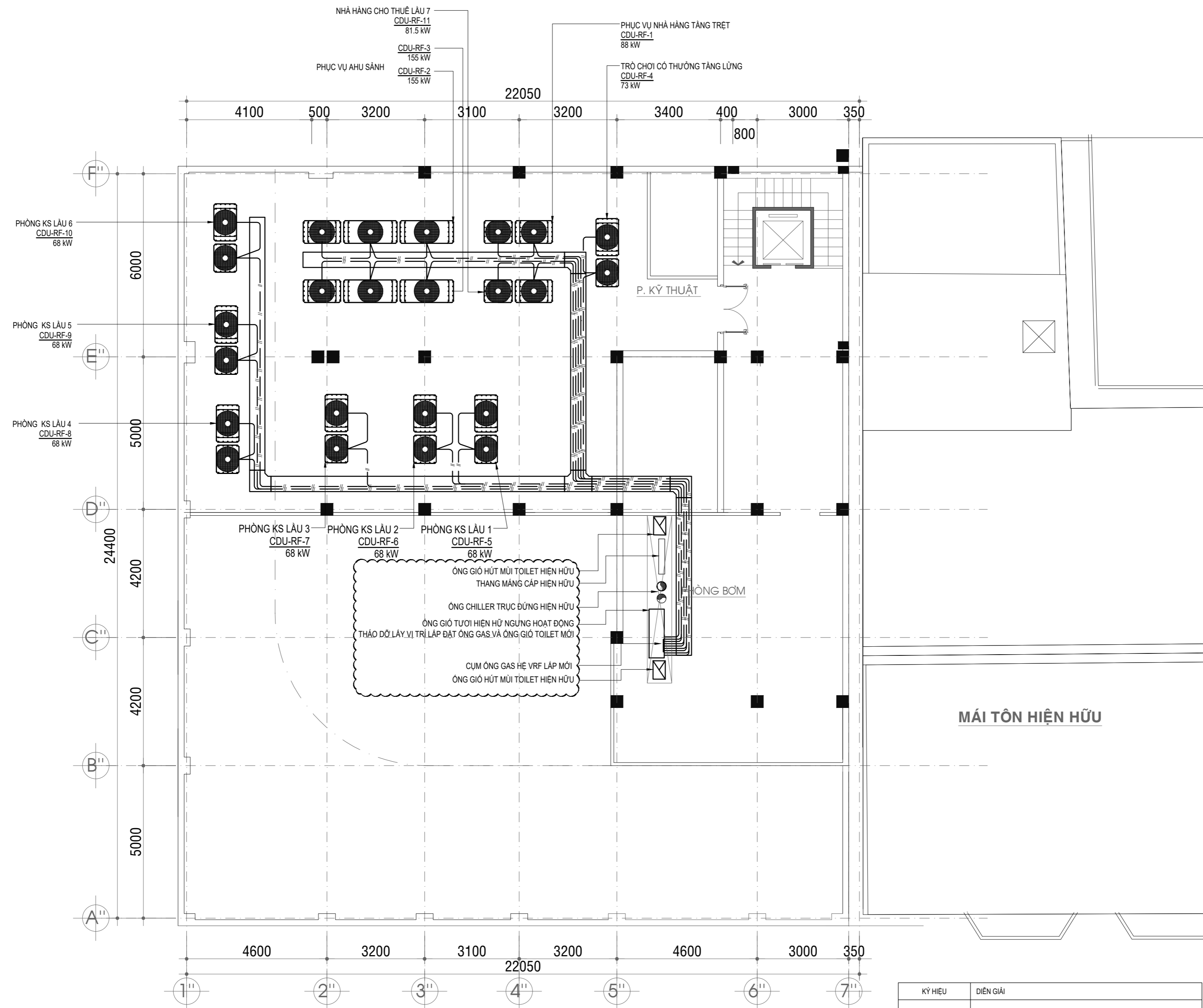
MẶT BẰNG CẢI TẠO DÂY ĐIỀU KHIỂN TẦNG KỸ THUẬT TL: 1/100
