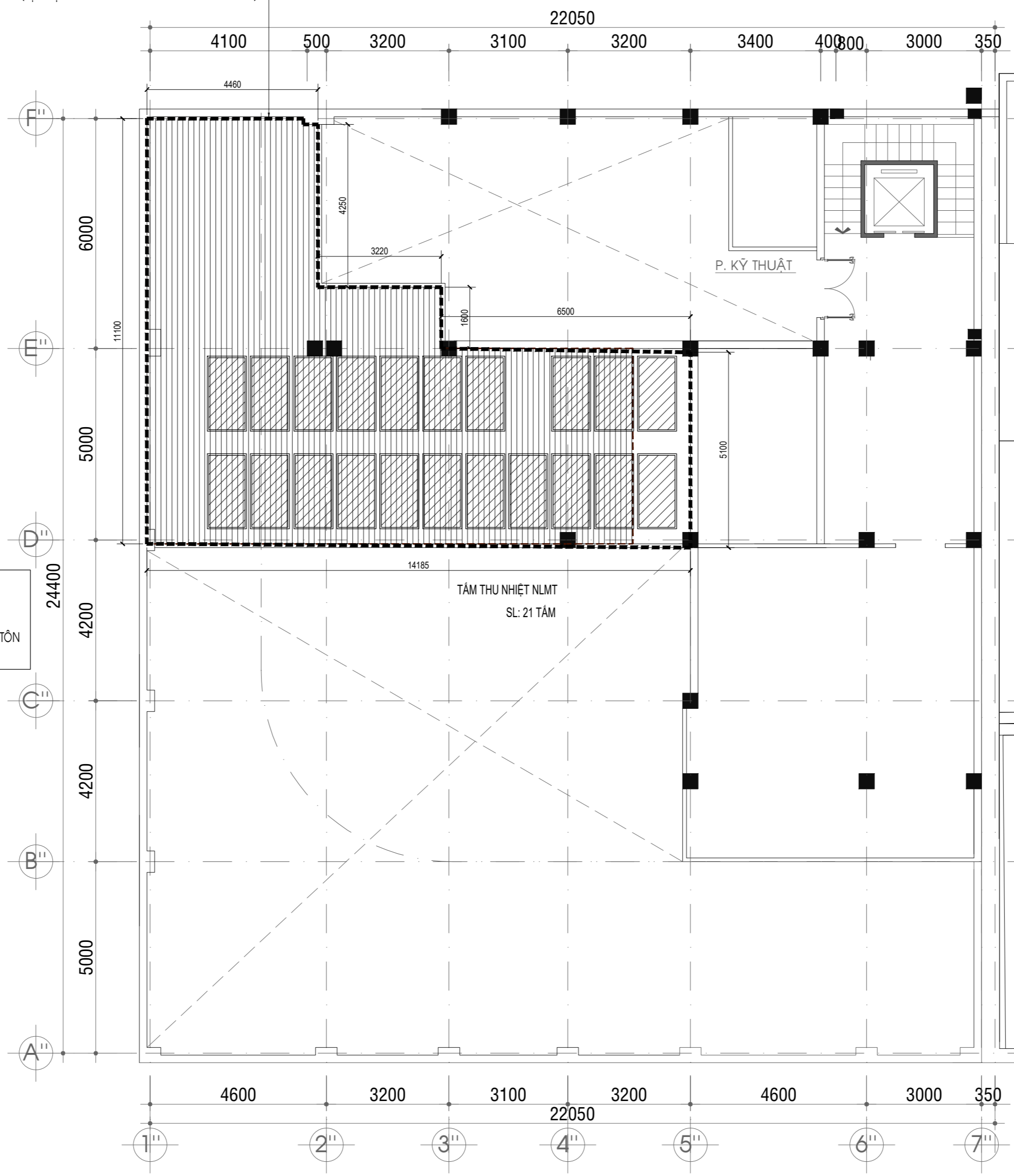
MẶT BẰNG THÁO DỠ TẦNG MÁI TL: 1/100
