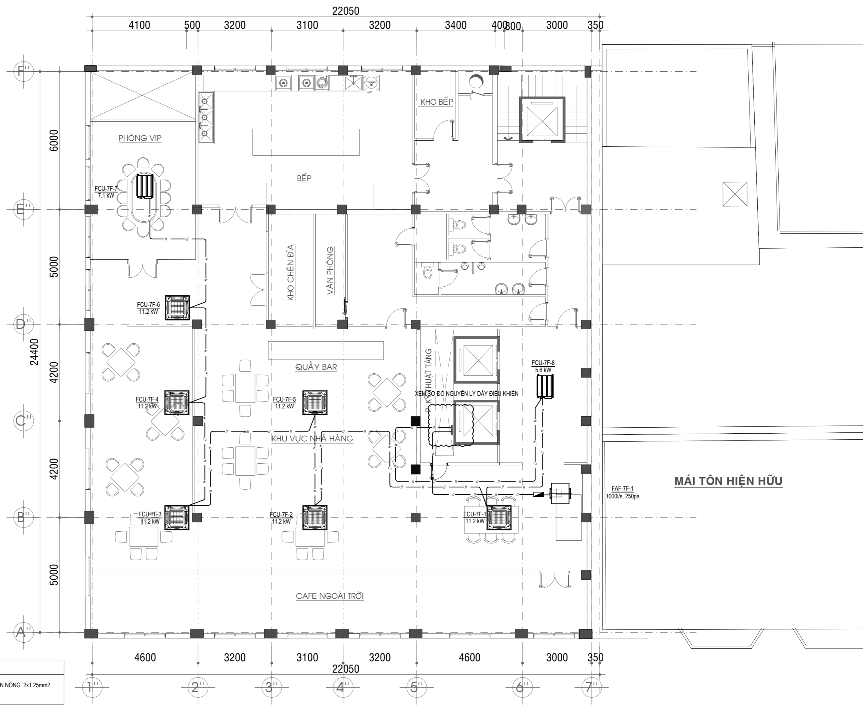
MẶT BẰNG CẢI TẠO DÂY ĐIỀU KHIỂN LẦU 7 TL: 1/100
