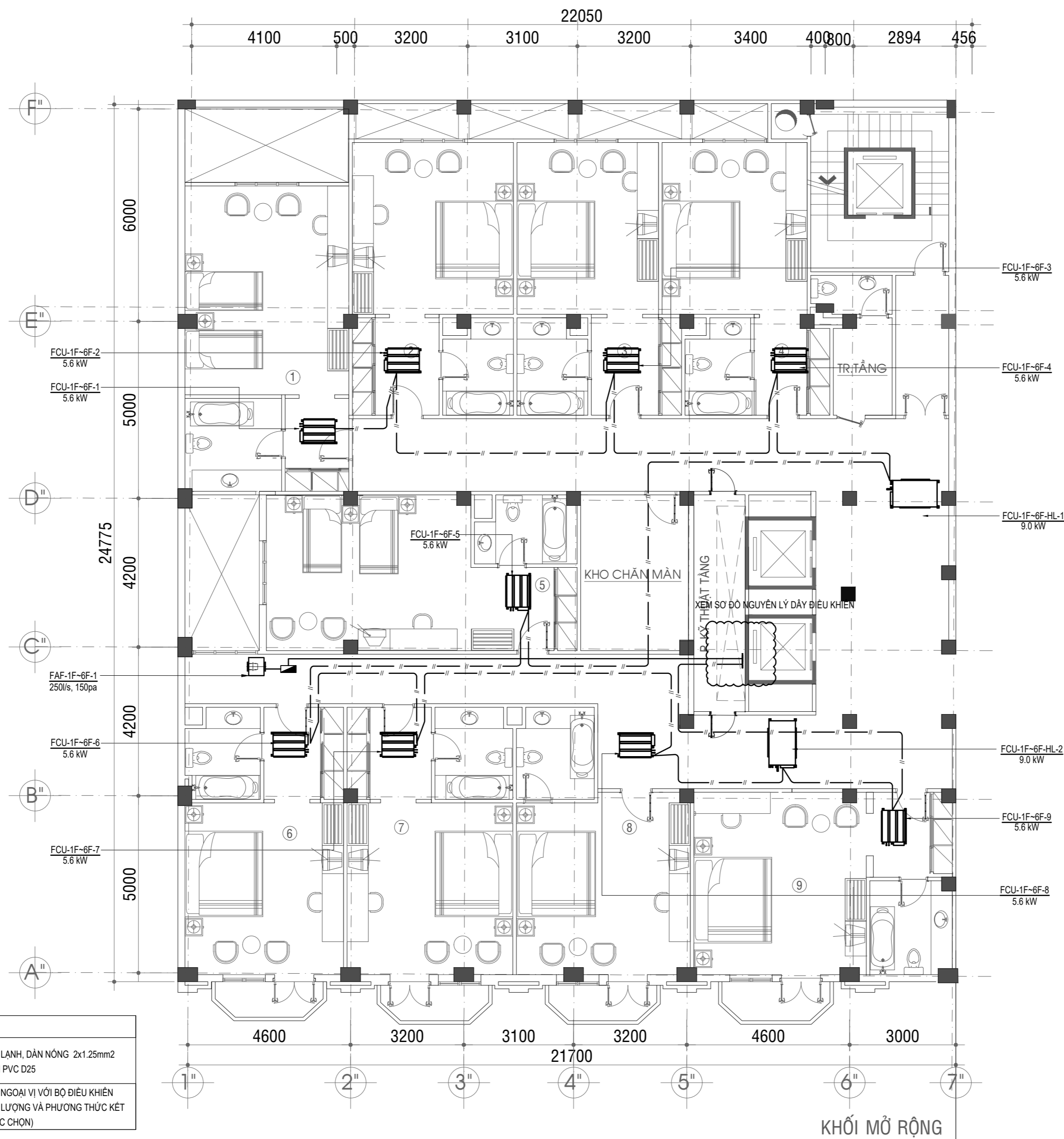
MẶT BẰNG CẢI TẠO DÂY ĐIỀU KHIỂN LẦU 1~ LẦU 6 TL: 1/100
