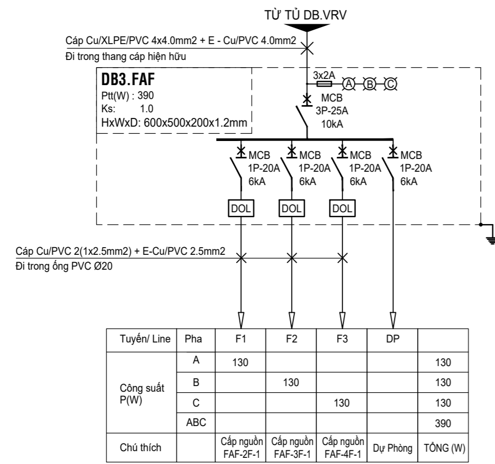
SƠ ĐỒ NGUYÊN LÝ TỦ ĐIỆN PHÂN PHỐI (DB3.FAF)
