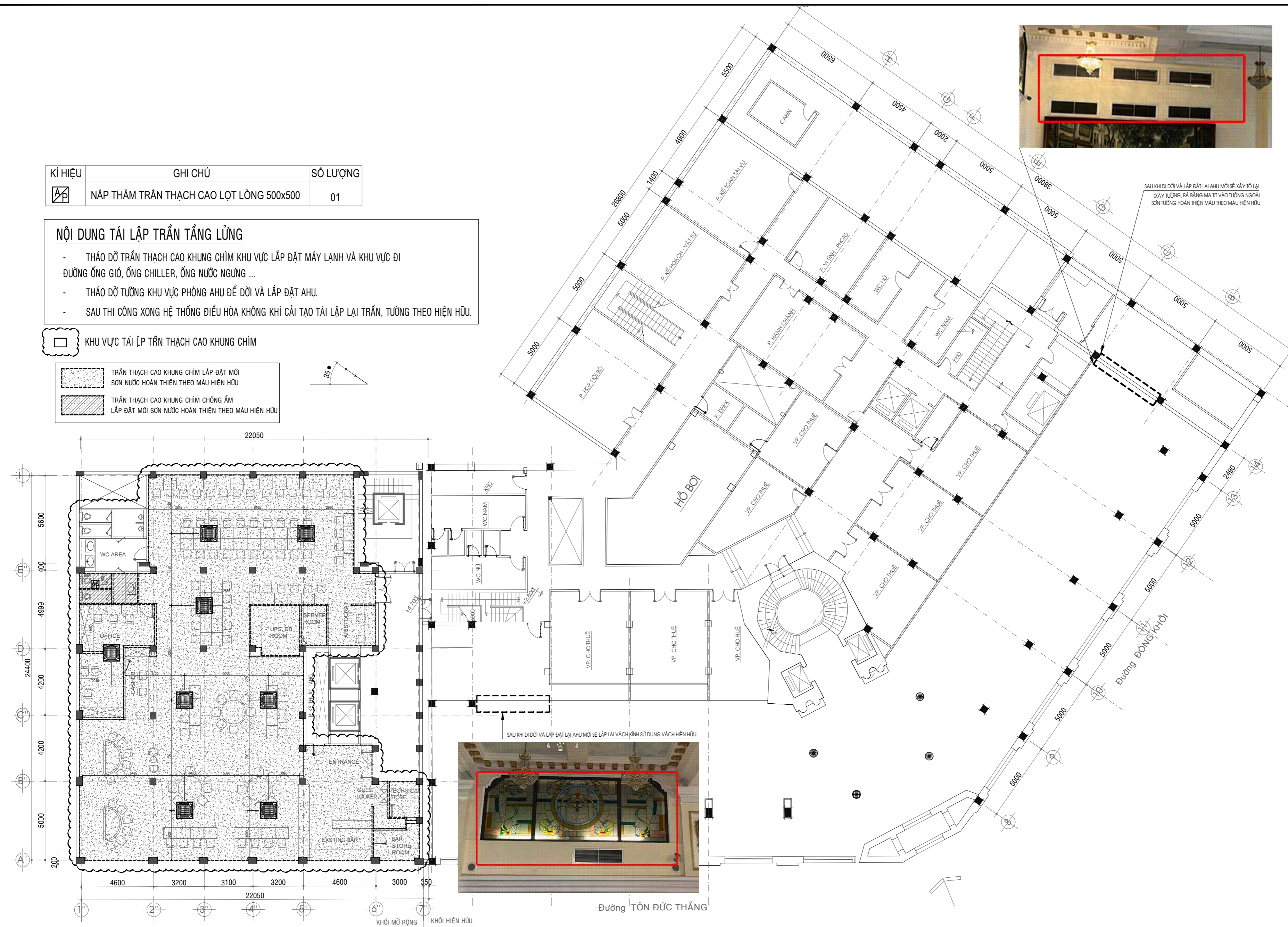
MẶT BẰNG TÁI LẬP TRẦN THẠCH CAO TẦNG LỬNG TL: 1/100
