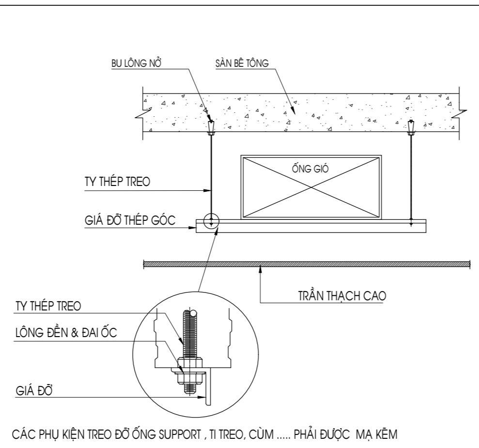
CHI TIẾT TREO VÀ ĐỠ ỚNG GIÓ ĐIỆN HÌNH
