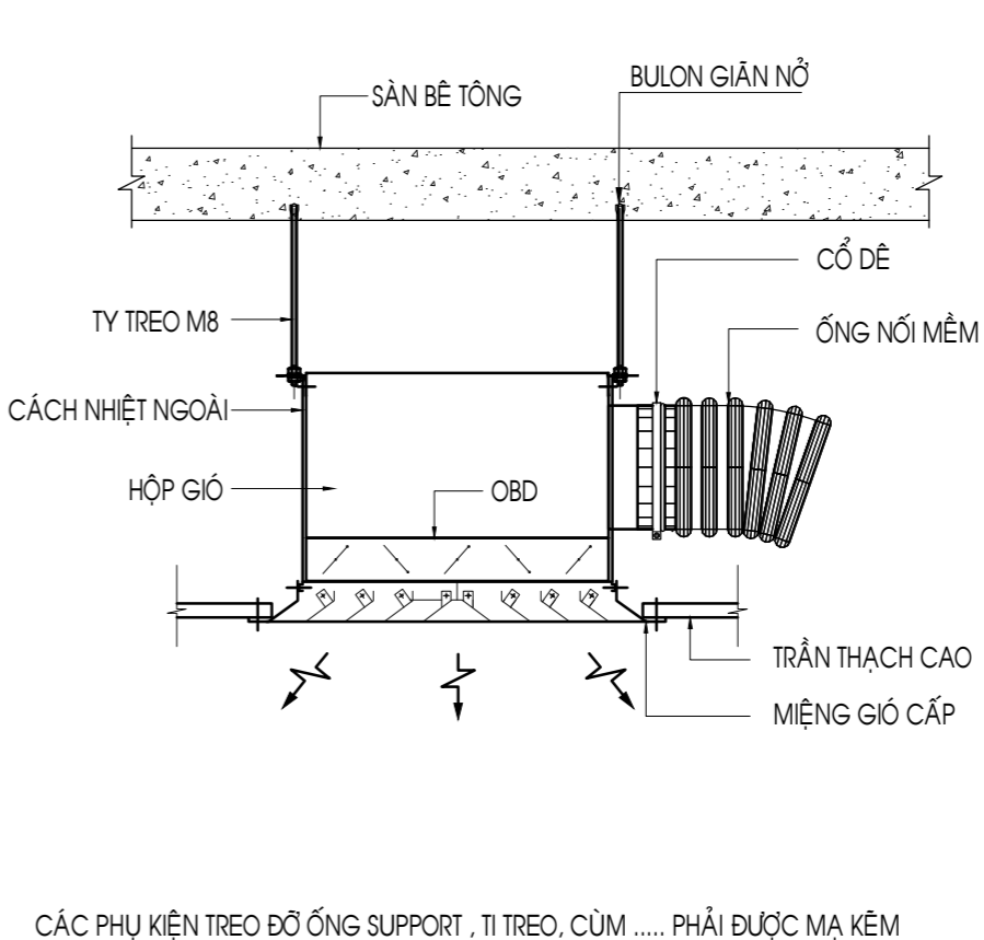
CHI TIẾT LẮP ĐẶT MIỆNG GIÓ CẤP
