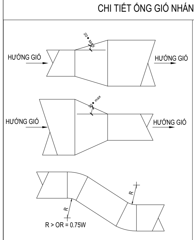
CHI TIẾT ỚNG GIẢM, ỚNG TĂNG
