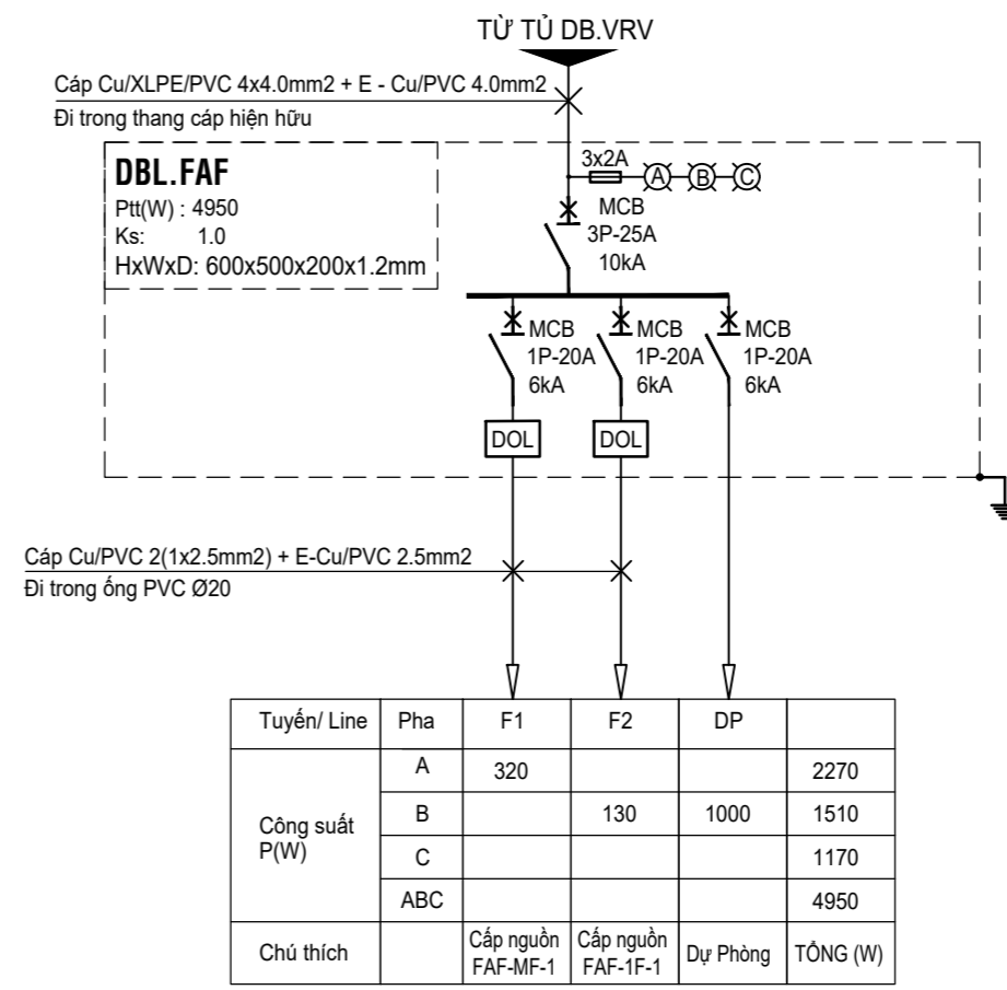
SƠ ĐỒ NGUYÊN LÝ TỦ ĐIỆN PHÂN PHỐI (DBL.AC)
