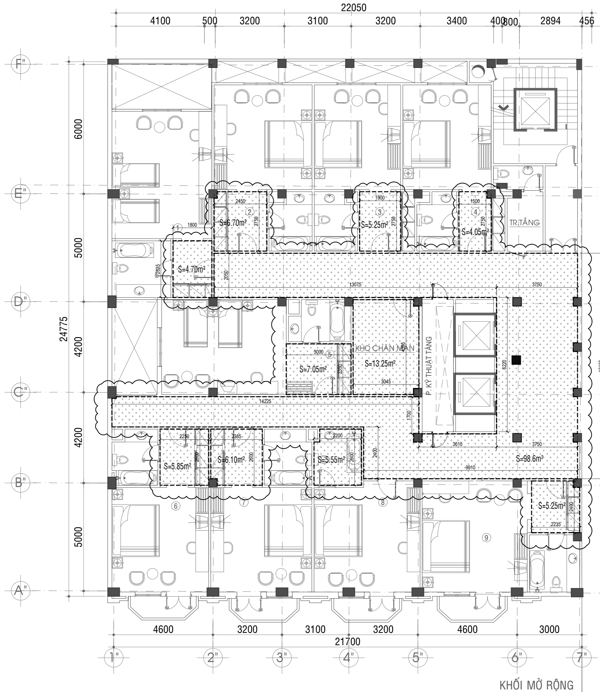
MẶT BẰNG THẢO DỜ LẦU 1 ~ LẦU 6 TL: 1/100
