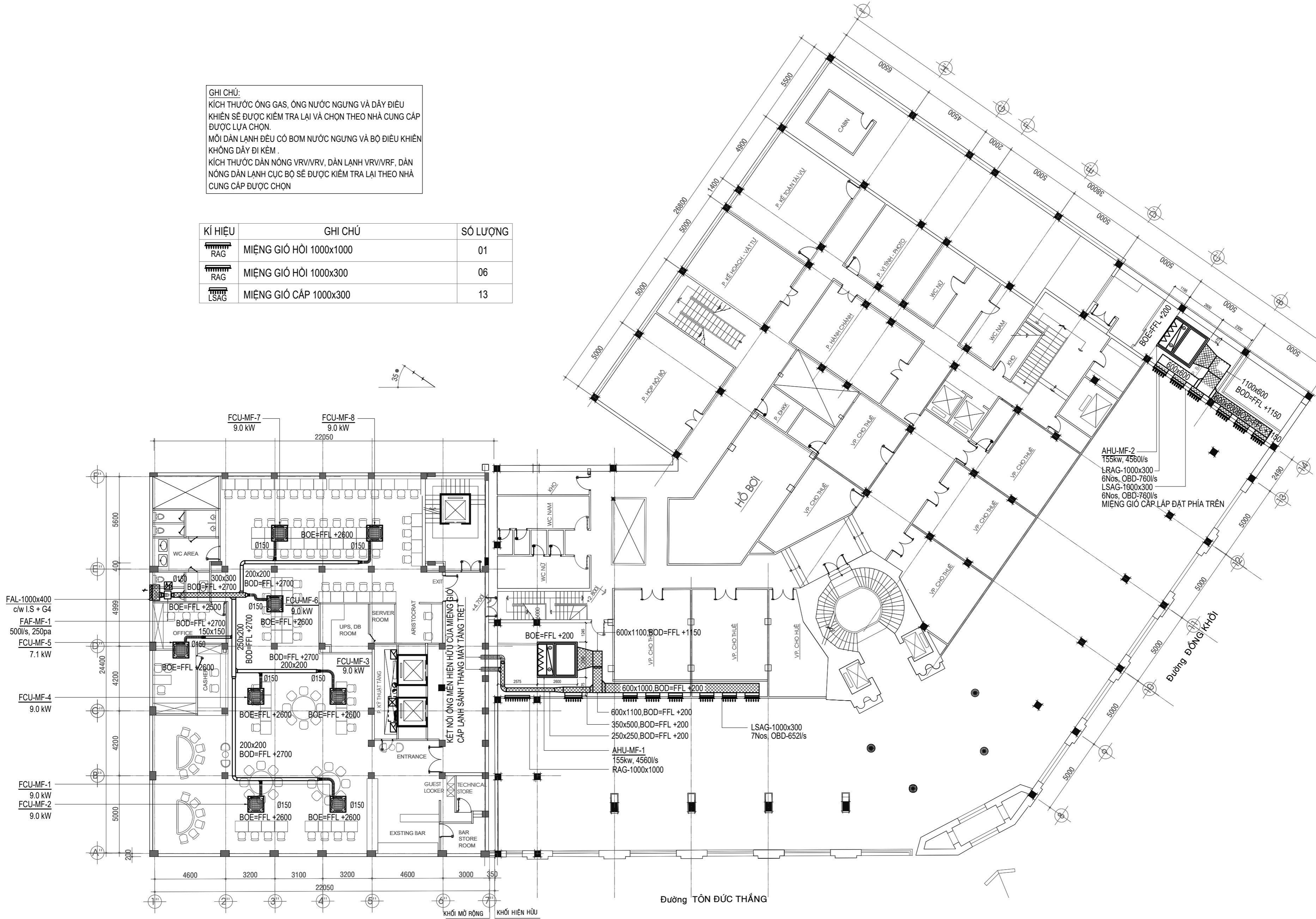
MẶT BẰNG CẢI TẠO ĐHKK & THÔNG GIÓ TẦNG LỬNG TL: 1/200
