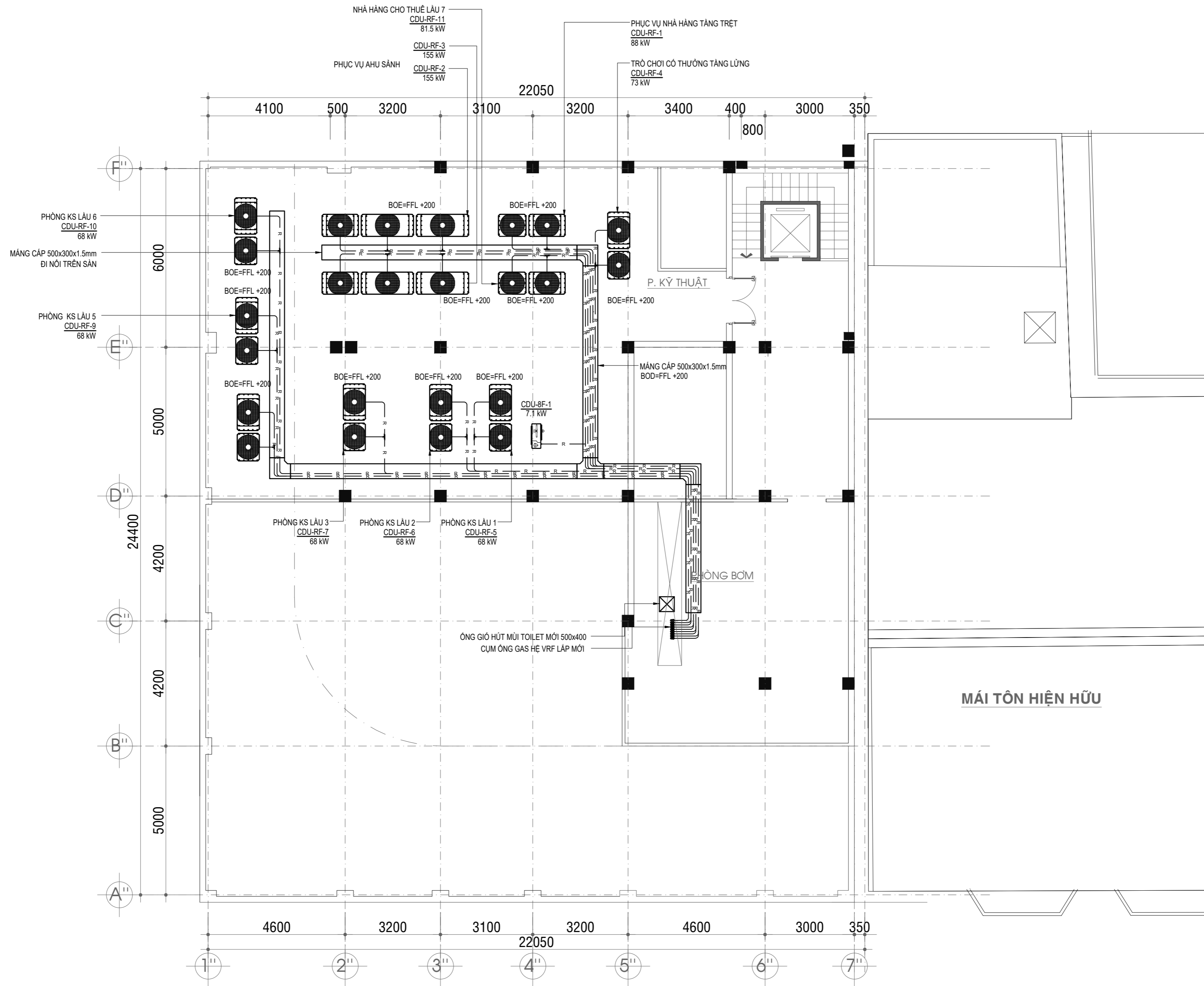
MẶT BẰNG CẢI TẠO ỚNG GAS, ỚNG NƯỚC NGỪNG TẦNG KỸ THUẬT TL: 1/100
