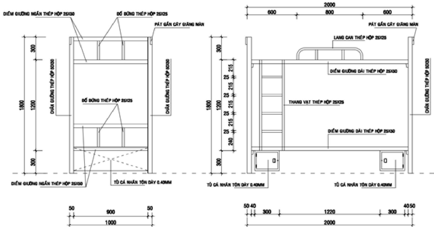
MẶT BÊN PHƯƠNG NGẮN GIƯỜNG SẮT 02 TẦNG TL 1/20
