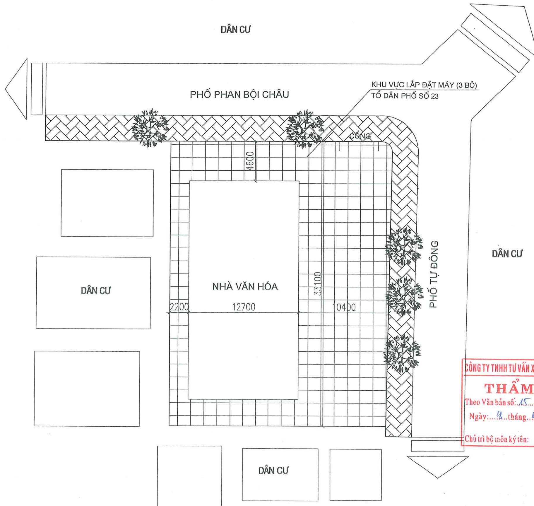
MẶT BẰNG BỐ TRÍ MÁY TẬP TỔ DÂN PHỐ SỐ 23 - SÂN NHÀ VĂN HÓA SỐ 8 PHAN BỘI CHÂU
