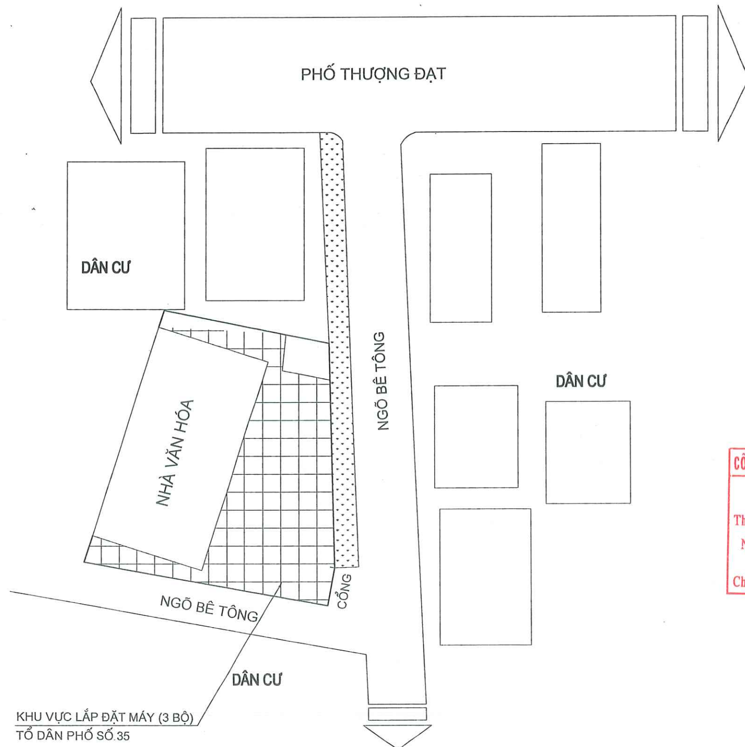
MẶT BẰNG BỐ TRÍ MÁY TẬP TỔ DÂN PHỐ SỐ 35 - SÂN NHÀ VĂN HÓA TỔ 35 CẦU HÀN, AN THƯỢNG
