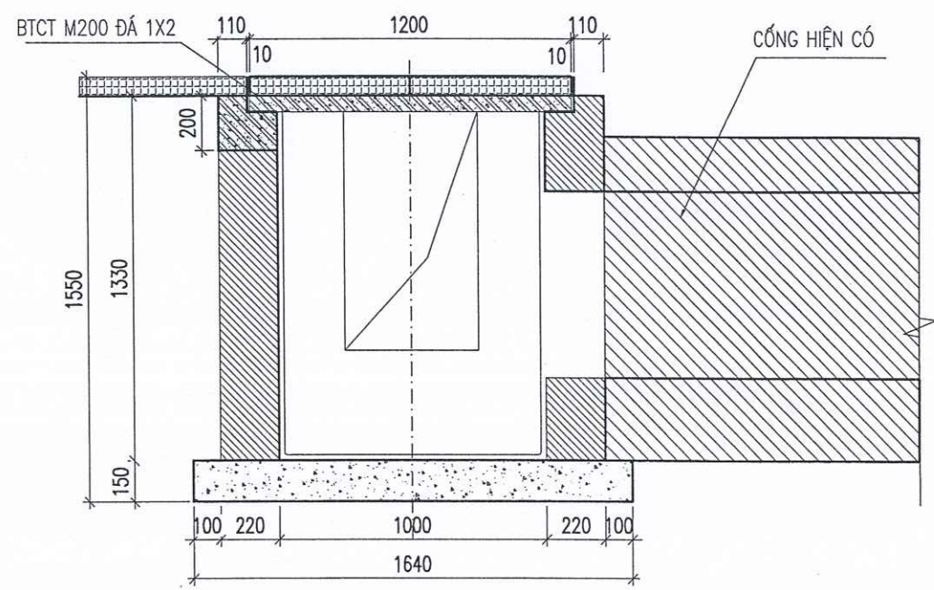
MẶT CẮT 1-1
