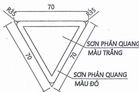
BIỂN SỐ W.208 TỈ LỆ: 1/20
