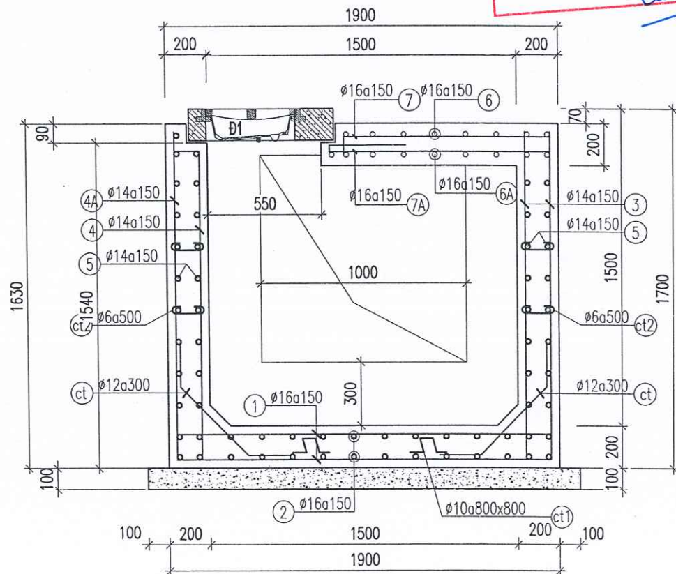
MẶT CẮT 1-1
