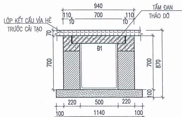
CỐNG THOÁT NƯỚC B = 500 HIỆN TRẠNG TRƯỚC KHI CẢI TẠO
