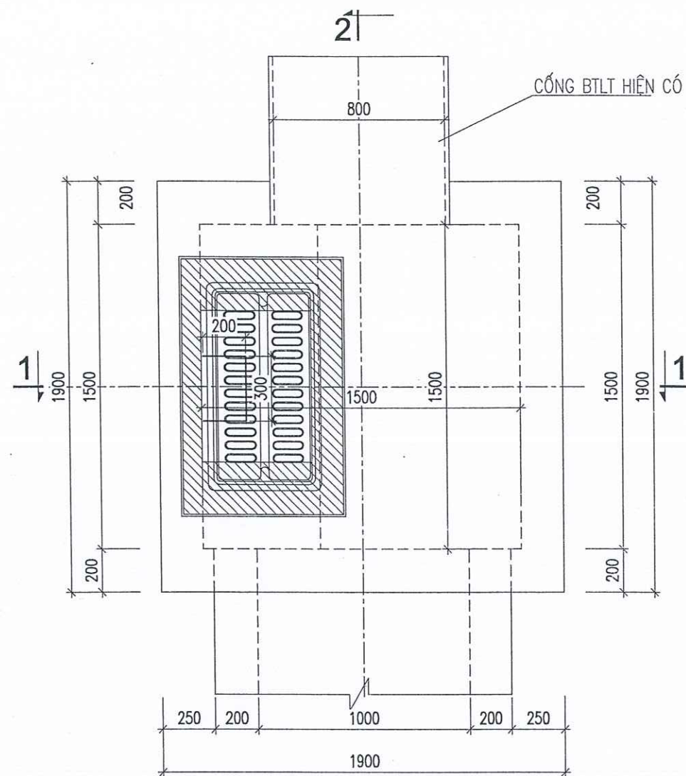
MẶT BẰNG HÓ GA G1
