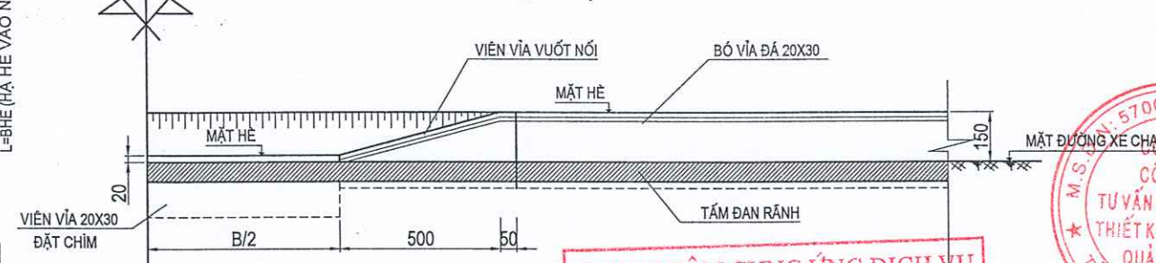
1/2 MẶT CẮT B-B
