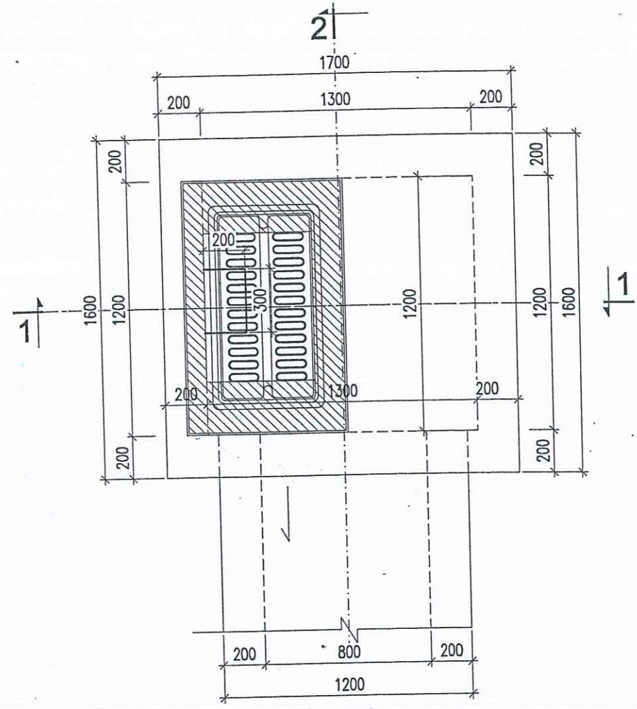
MẶT BẰNG HỒ GA G1
