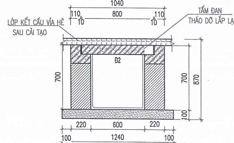
CỐNG THOÁT NƯỚC B = 600 HIỆN TRẠNG SAU KHI CẢI TẠO
