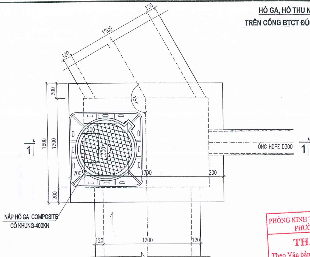
MẶT BẰNG HỒ GA TRÊN CỐNG 1200X1200
