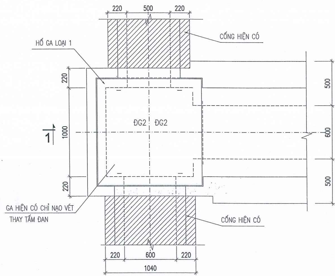
MẶT BẰNG HỐ GA K63
