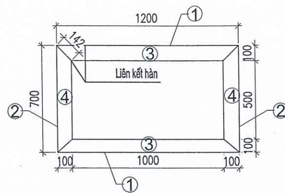
MẶT BẰNG THÉP BO MIỆNG ĐẠN HỐ THU ĐG1 (SL: 94 MIỆNG)
