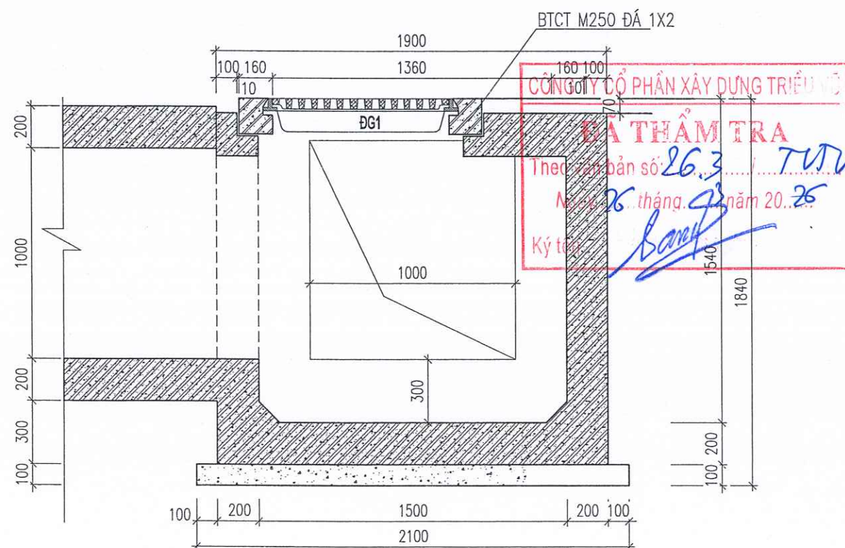
MẶT CẮT 2-2
