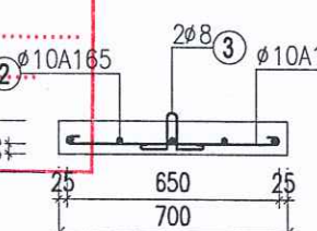
TẦM ĐÀN Đ1 (ĐẦY CỐNG B500 CỐNG THƯỜNG) Tận dụng : 70%
