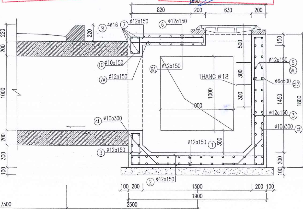
MẶT CẮT 1-1
