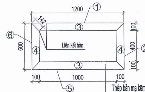
MẶT BẰNG THÉP BO MIỆNG ĐẠN HỐ ĐG2 (SL: 148 TẮM)
