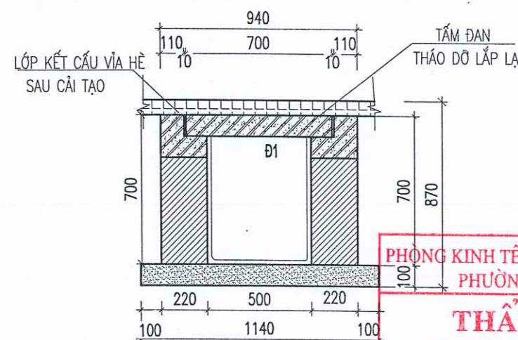
CỐNG THOÁT NƯỚC B = 500 HIỆN TRẠNG SAU KHI CẢI TẠO
