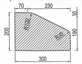
CẤU TẠO VIÊN VỈA 20X30X100
