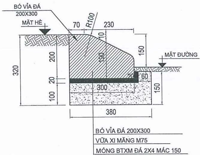
CHI TIẾT BÓ VỈA 200X300X1000MM KHÔNG ĐẠN RÃNH
