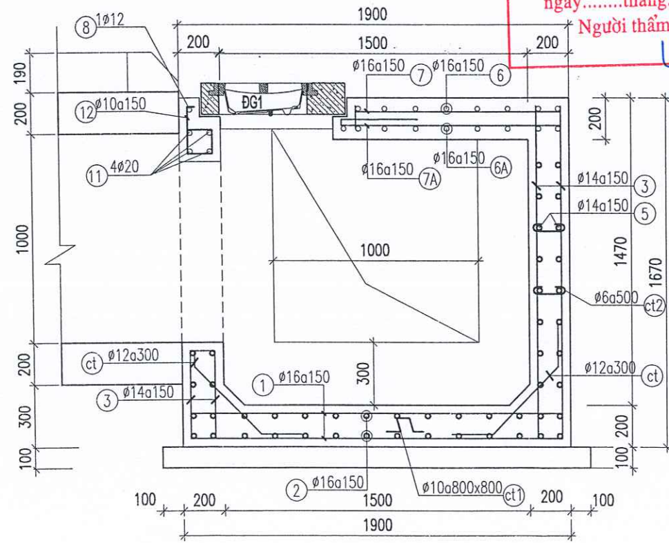
MẶT CẮT 1-1
