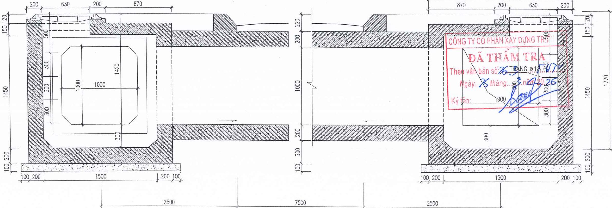
MẶT CẮT 1-1
