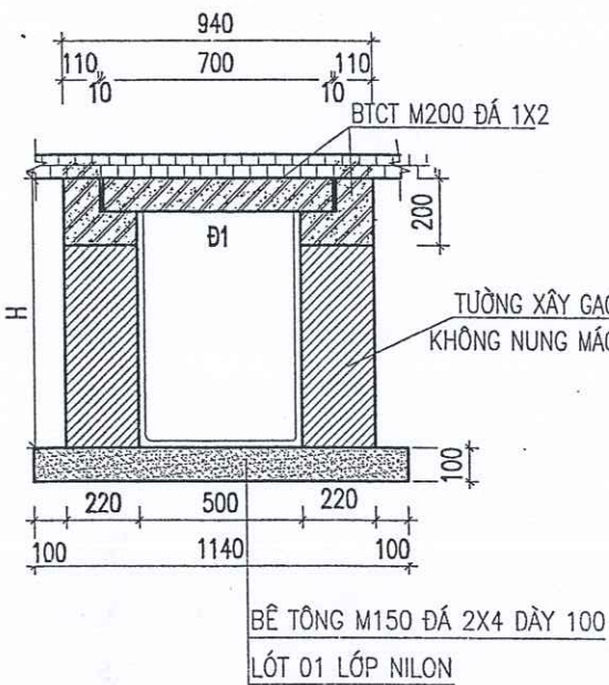
MẶT CÁT CỐNG XÂY MỚI B = 500 CHIỀU DÀI : 216.50 MÉT
