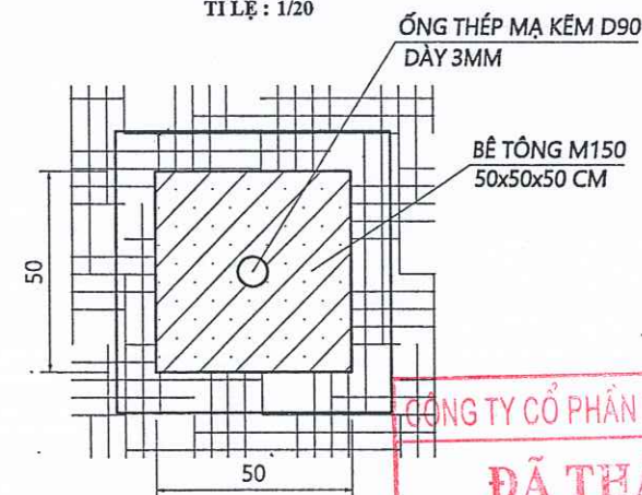
A - A TỈ LỆ: 1/20
