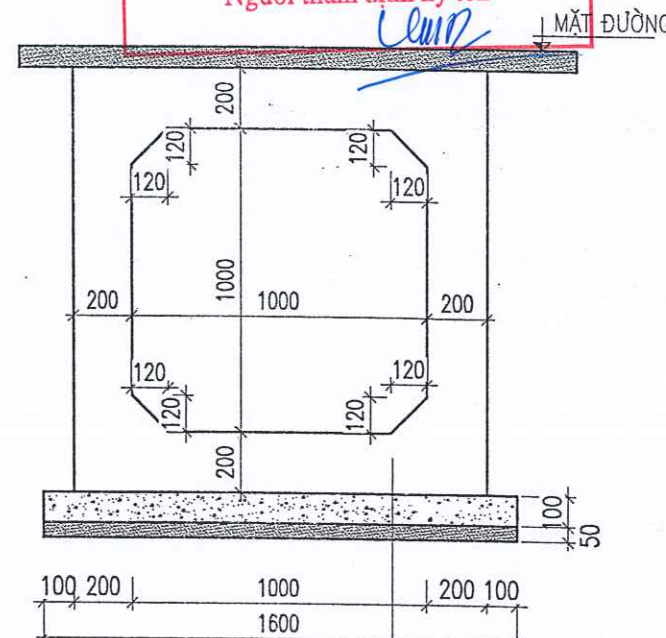
CỐNG BTCT ĐỔ TẠI CHỖ 1000X1000 CHIỀU DÀI : 85.8 MÉT
