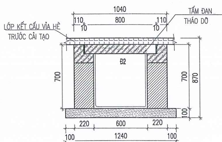
CỐNG THOÁT NƯỚC B = 600 HIỆN TRẠNG TRƯỚC KHI CẢI TẠO
