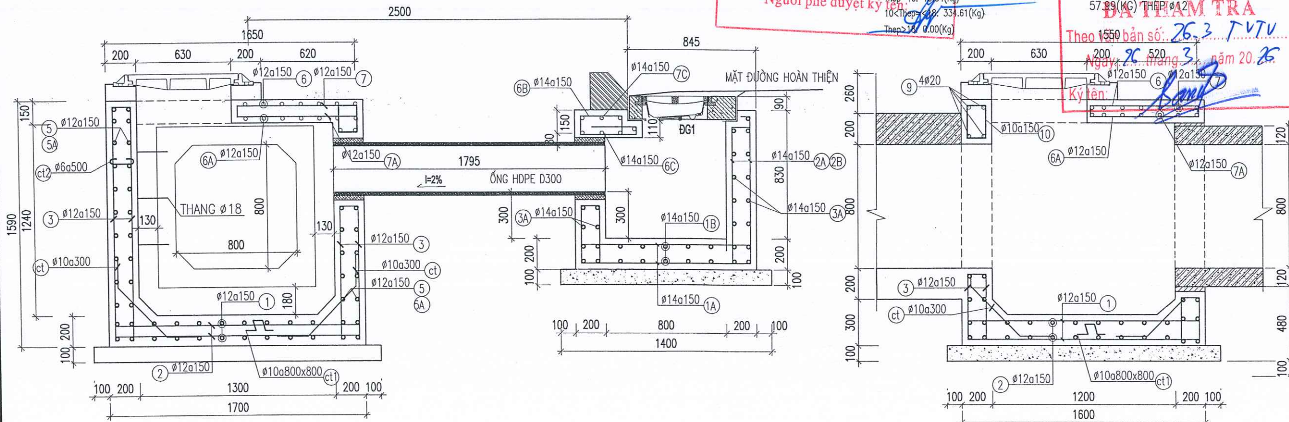
MẶT CẮT 1 - 1
