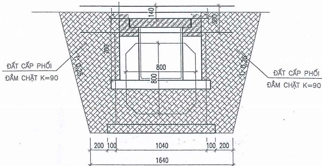
MẶT CẮT PHẢ DỜ CỐNG HIỆN CÓ THI CÔNG CỐNG BTCT ĐÚC SẴN KT : 800X800 DIỆN TÍCH D= 1.87 M2
