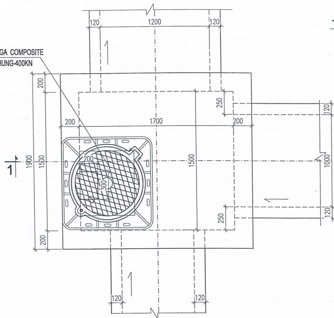
MẶT BẰNG HỐ GA G12
