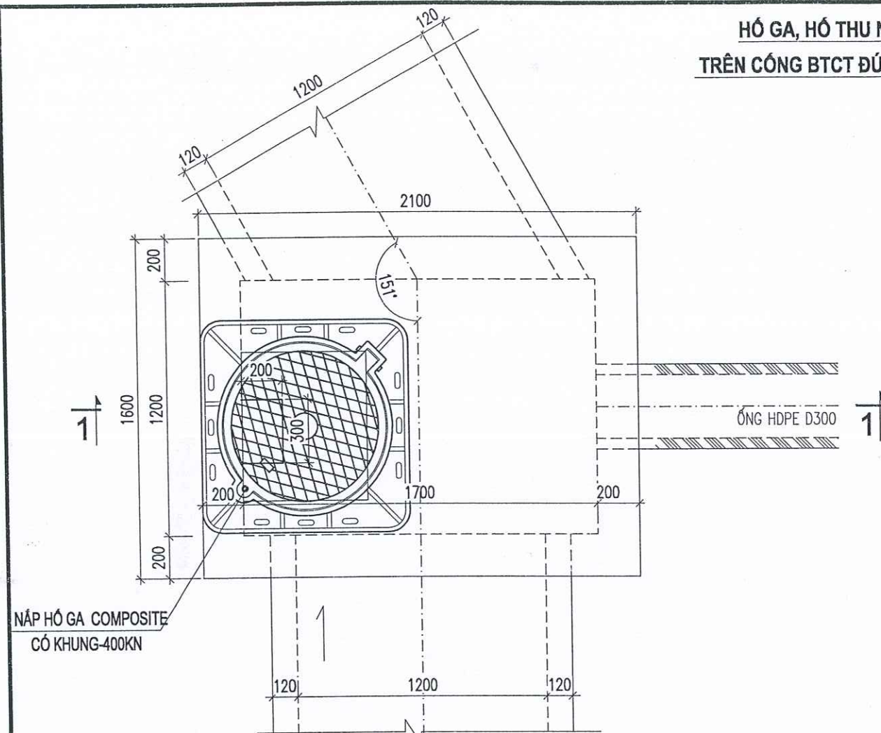
MẶT BẰNG HỒ GA TRÊN CÔNG 1200X1200
