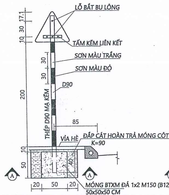
CẤU TẠO CỘT BIÊN BẢO TỈ LỆ: 1/40
