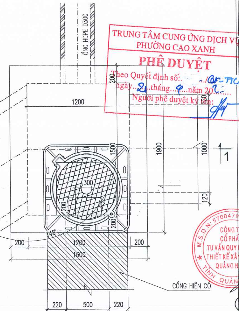
MẶT BẰNG HỒ GA G11
