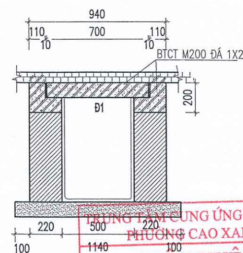
PHÁ ĐỠ CỐNG B500 HIỆN TRẠNG CHIỀU DÀI : 344.20 MÉT
