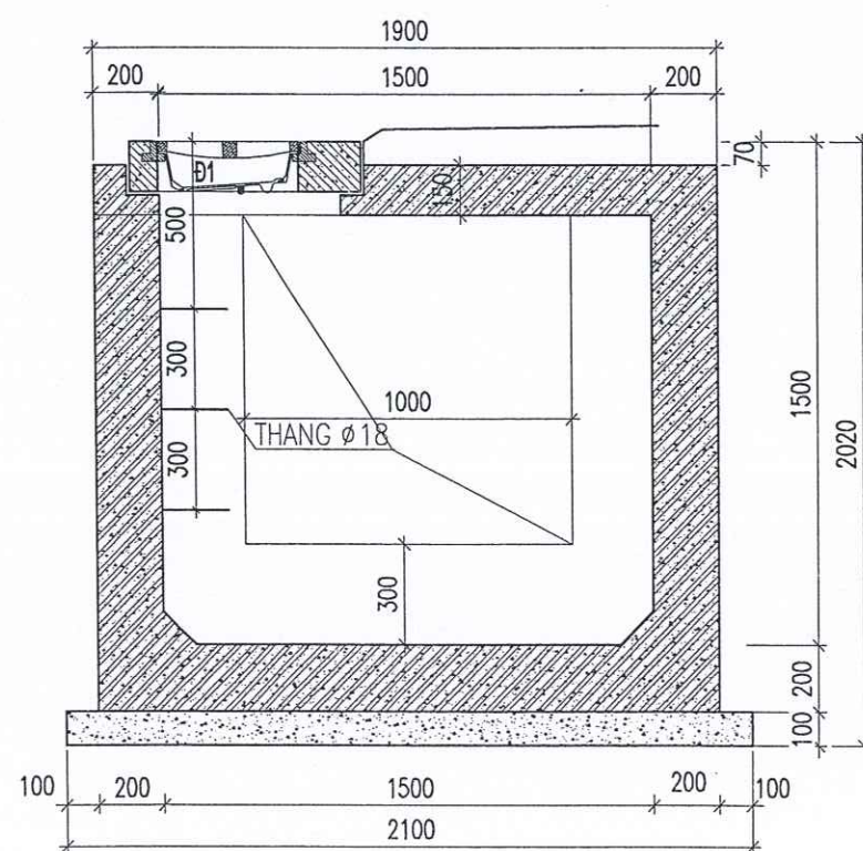
MẶT CẮT 1-1
