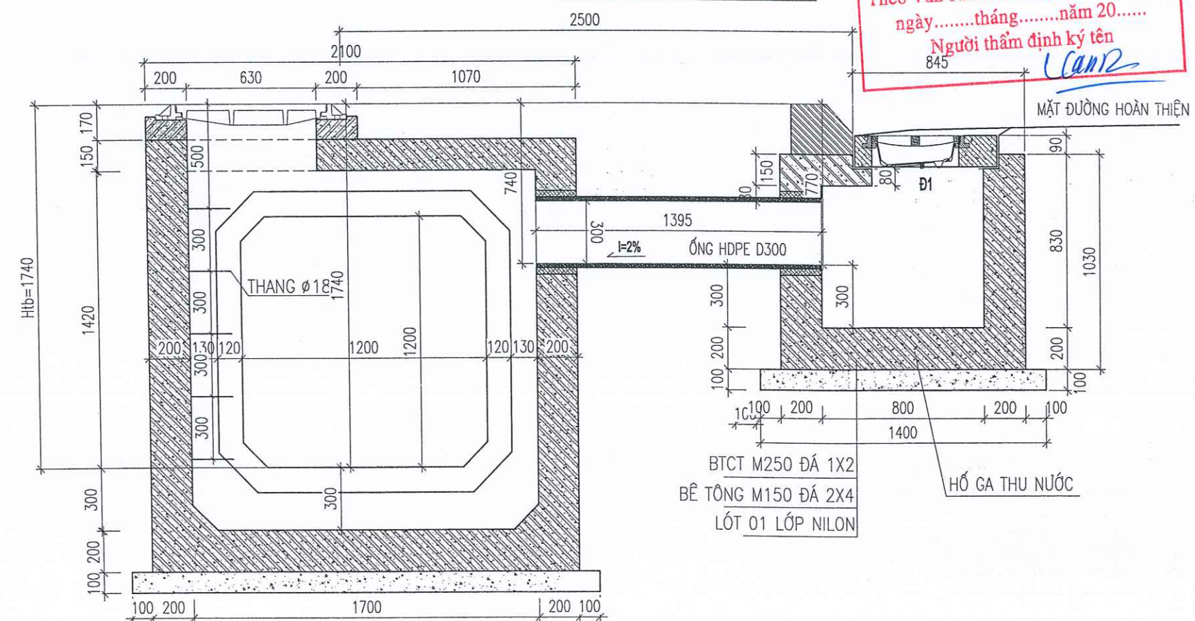
MẶT CẮT 1-1
