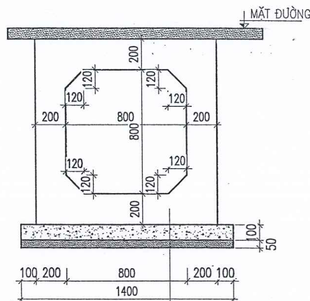
CỐNG BTCT ĐỔ TẠI CHỖ 800X800 CHIỀU DÀI : 15.0 MÉT
