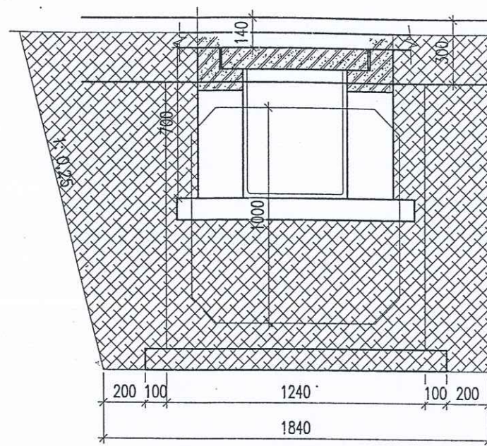
MẶT CẮT PHẢ DỜ CỐNG HIỆN CÓ THI CÔNG CỐNG BTCT ĐÚC SẴN KT : 1000X1000 DIỆN TÍCH D= 2.66M2
