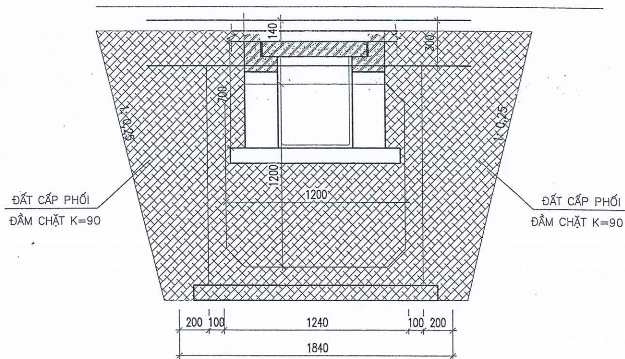
MẶT CẮT PHẢ DỜ CỐNG HIỆN CÓ THI CÔNG CỐNG BTCT ĐÚC SẴN KT : 1200X1200 DIỆN TÍCH D= 2.66M2
