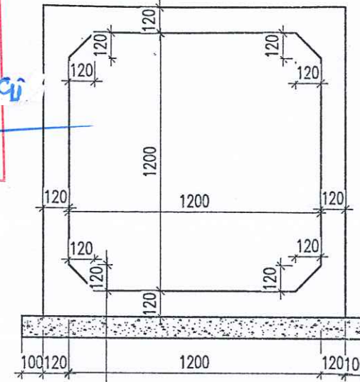
CỐNG HỘP BTCT MẮC 200 ĐÚC SẴN BÊ TÔNG M150 ĐÁ 2X4 DÀY 100 LỚT 01 LỚP NILON ĐẤT NỀN ĐẦM CHẶT TỪNG LỚP ĐẾN K=0.90
