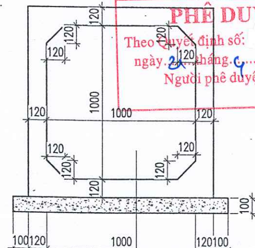
CỐNG HỘP BTCT MẮC 200 ĐÚC SẴN BÊ TÔNG M150 ĐÁ 2X4 DÀY 100 LỚT 01 LỚP NILON ĐẤT NỀN ĐẦM CHẶT TỪNG LỚP ĐẾN K=0.90
