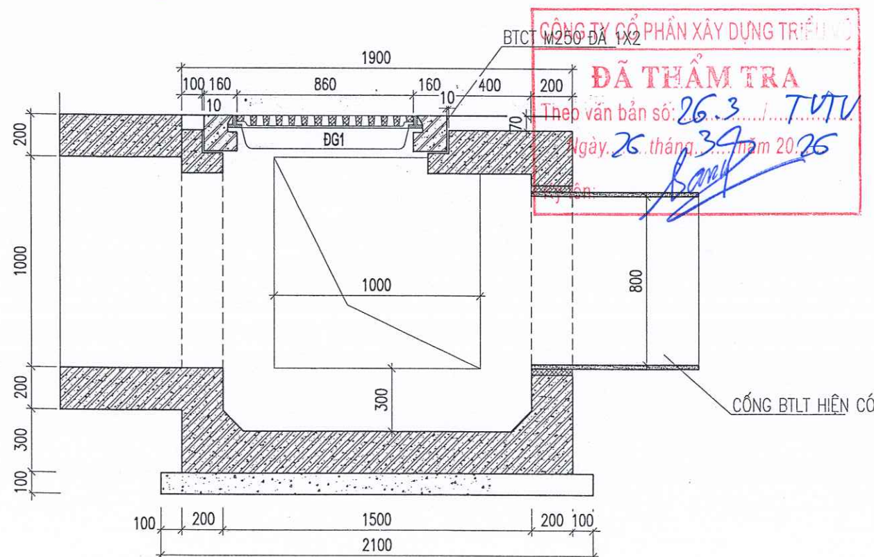
MẶT CẮT 2-2
