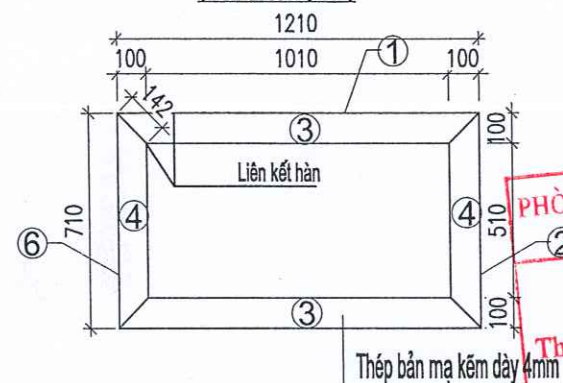
MẶT BẰNG THÉP BO MIỆNG HỐ THU (SL: 94 TẮM)
