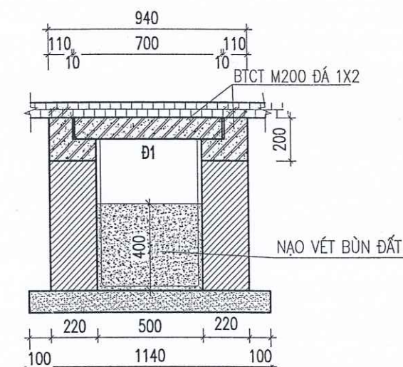
NAO VẾT CỐNG B = 500 HIỆN TRẠNG CHIỀU DÀI : 1366.70 MÉT
