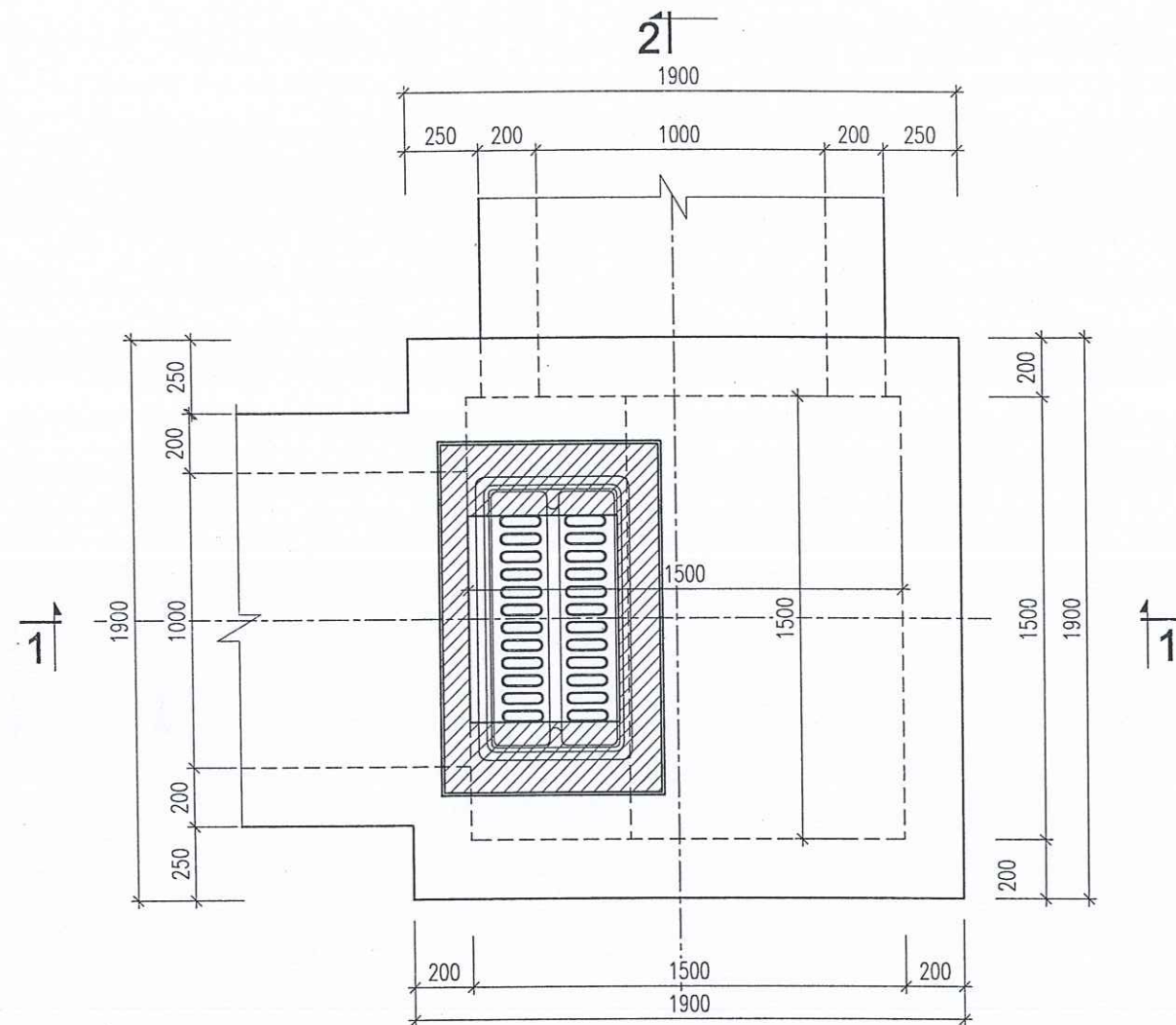
MẶT BẰNG HỒ GA G2
