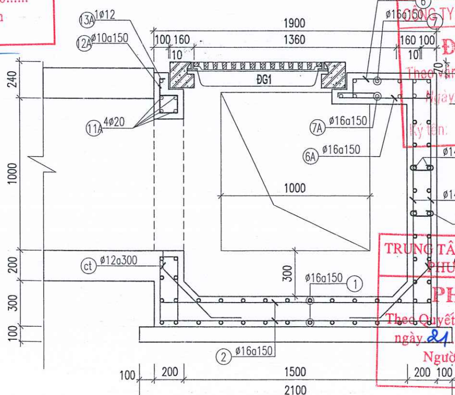
MẶT CẮT 2-2
