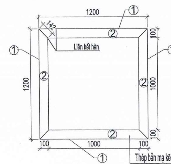
MẶT BẰNG THÉP BO MIỆNG HỐ GA (SL: 65+6+3= 74 MIỆNG)
