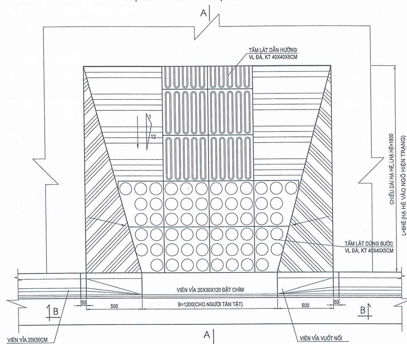
CHI TIẾT HẠ HÈ (HÈ ĐƯỜNG DỪNG CHO VỈA ĐÁ 20X30 CM)
