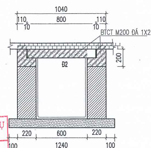
PHÁ ĐỠ CỐNG B600 HIỆN TRẠNG CHIỀU DÀI : 118.30 MÉT
