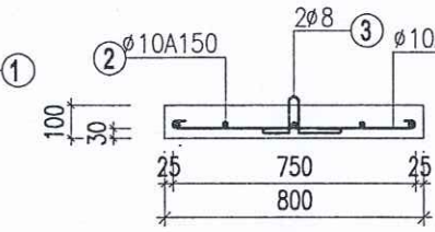
TẦM ĐÀN Đ2 (ĐẦY CỐNG B600 CỐNG THƯỜNG) Tận dụng : 70%
