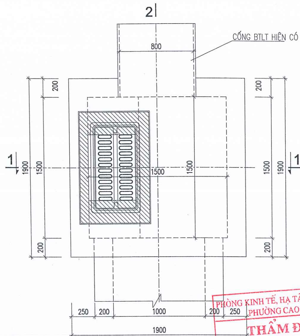
MẶT BẰNG HỒ GA G1
