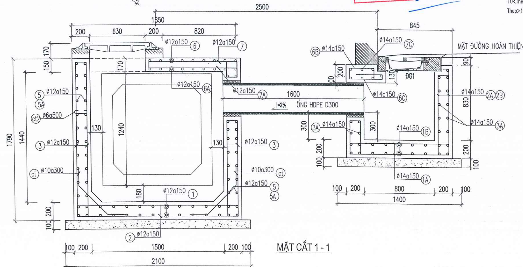
MẶT BẰNG HỒ GA TRÊN CÔNG 1000X1000 G6 (01 HỒ)
