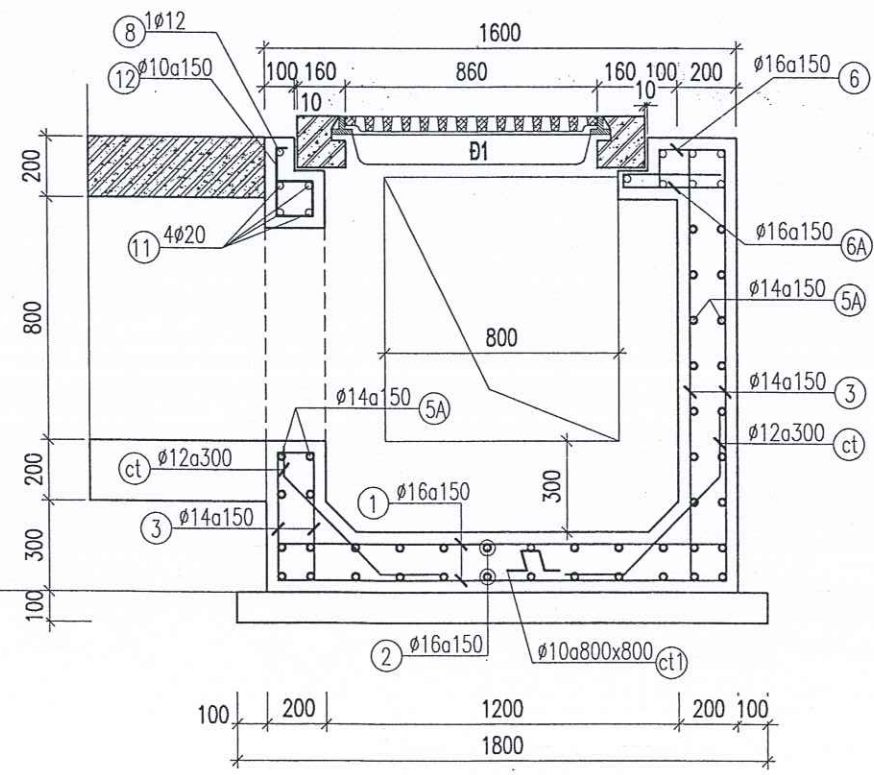
MẶT CẮT 1-1
