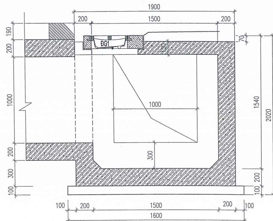
MẶT CẮT 1-1
