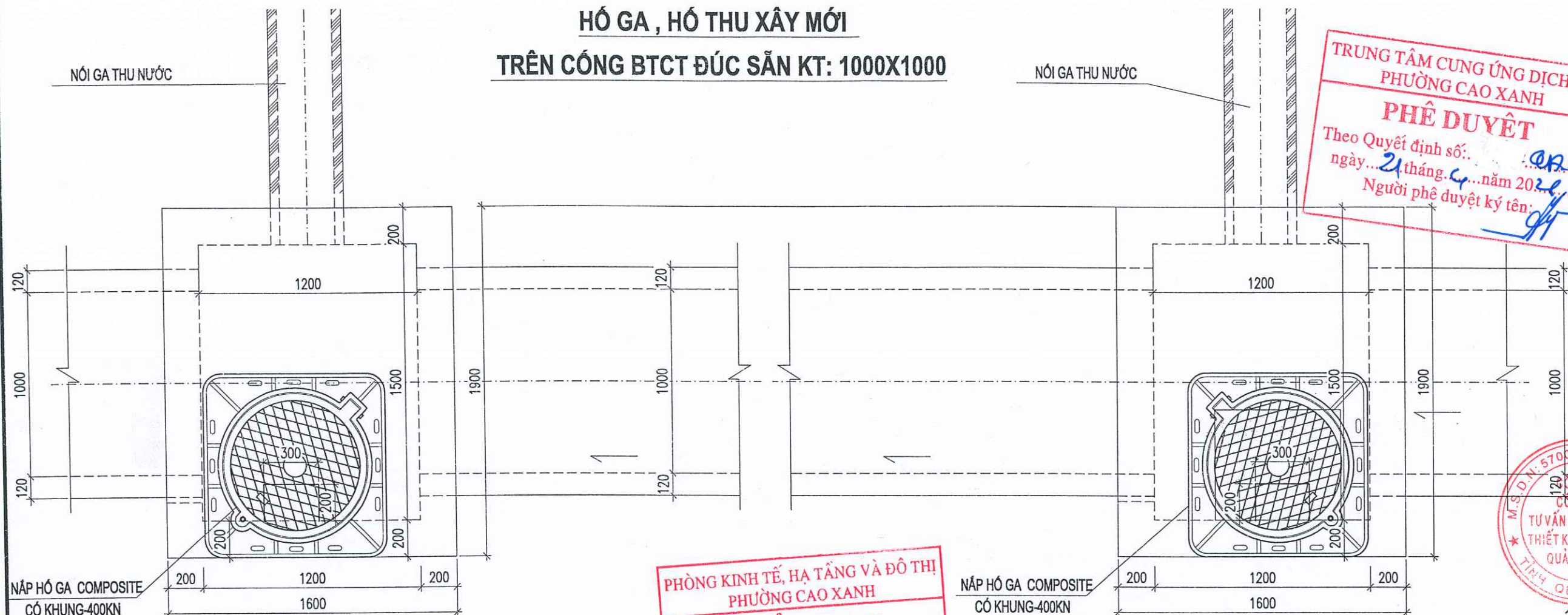
MẶT BẰNG HỒ GA G9
