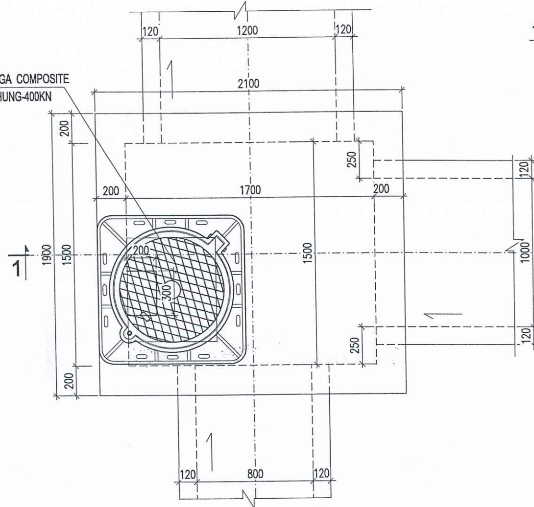
MẶT BẰNG HỒ GA G12
