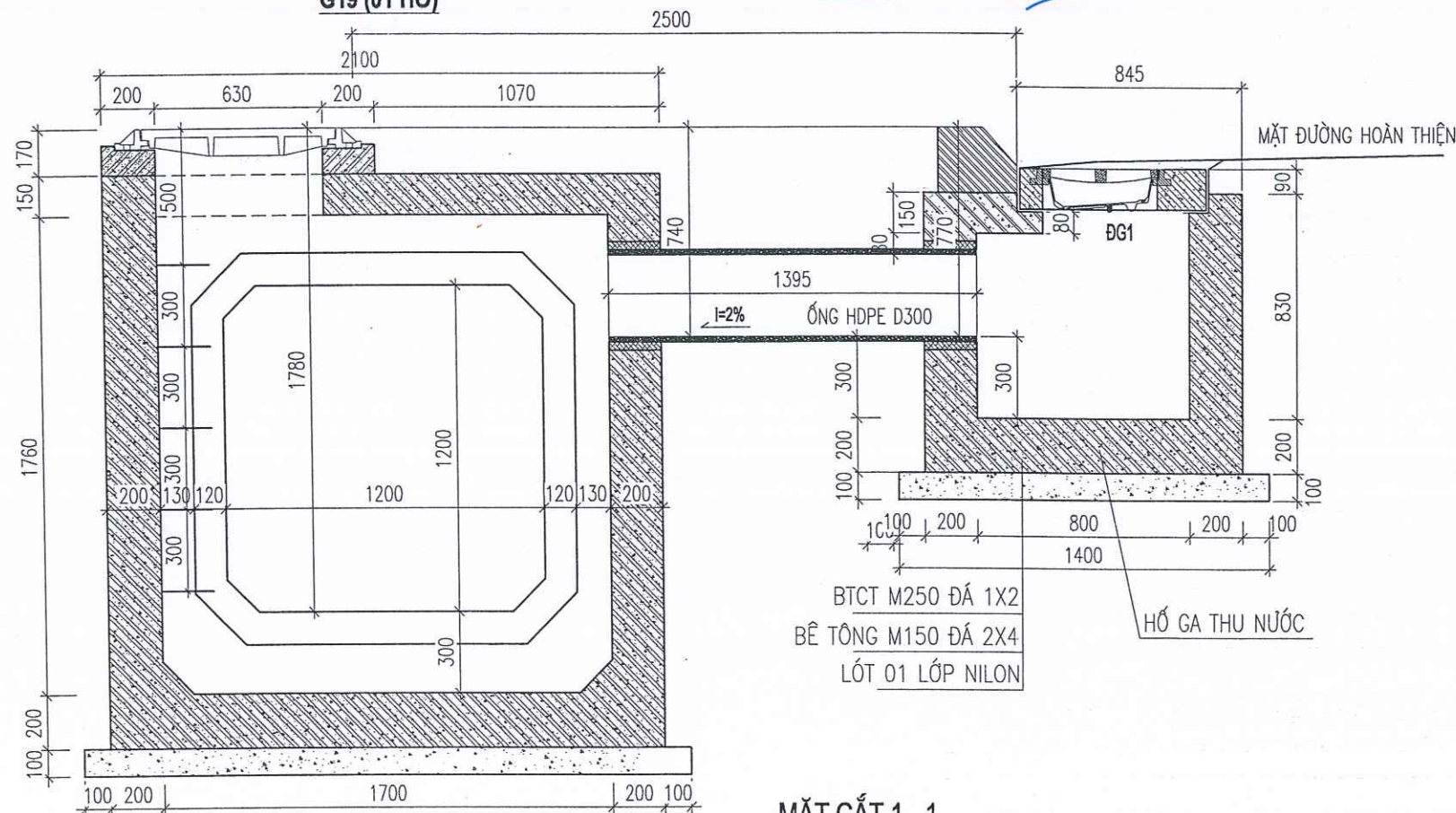
MẶT CẮT 1-1
