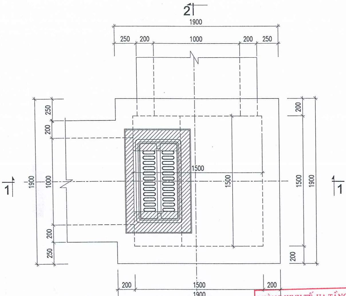
MẶT BẰNG HỒ GA G2
