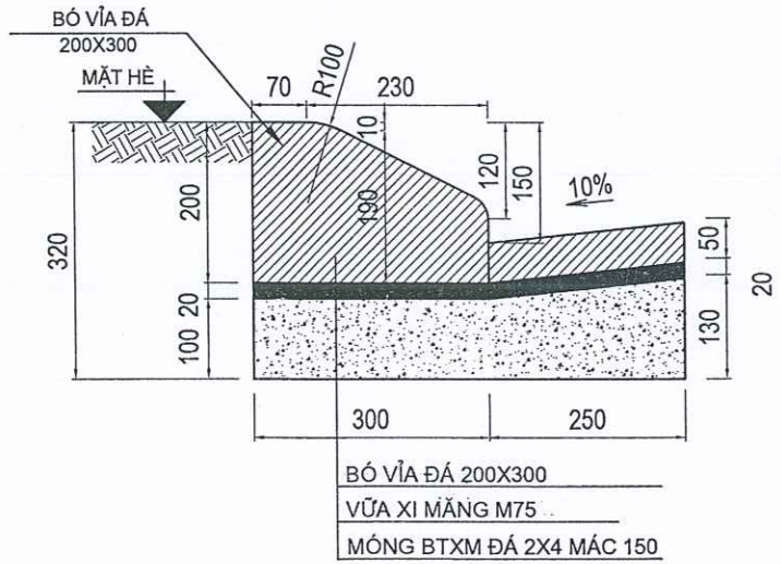
CHI TIẾT BÓ VỈA 200X300X1000MM CÓ ĐẠN RÃNH
