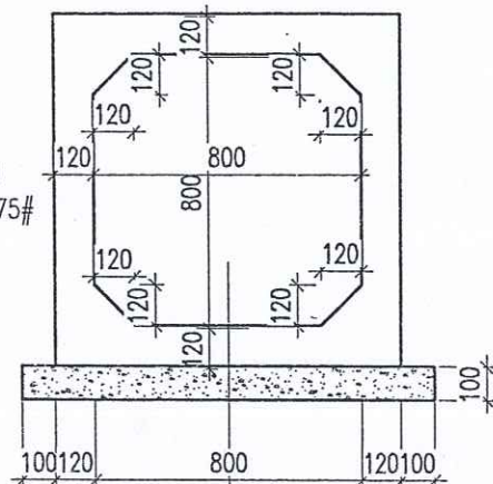
CỐNG HỘP BTCT MẮC 200 ĐÚC SẴN BÊ TÔNG M150 ĐÁ 2X4 DÀY 100 LỚT 01 LỚP NILON ĐẤT NỀN ĐẦM CHẶT TỪNG LỚP ĐẾN K=0.90
