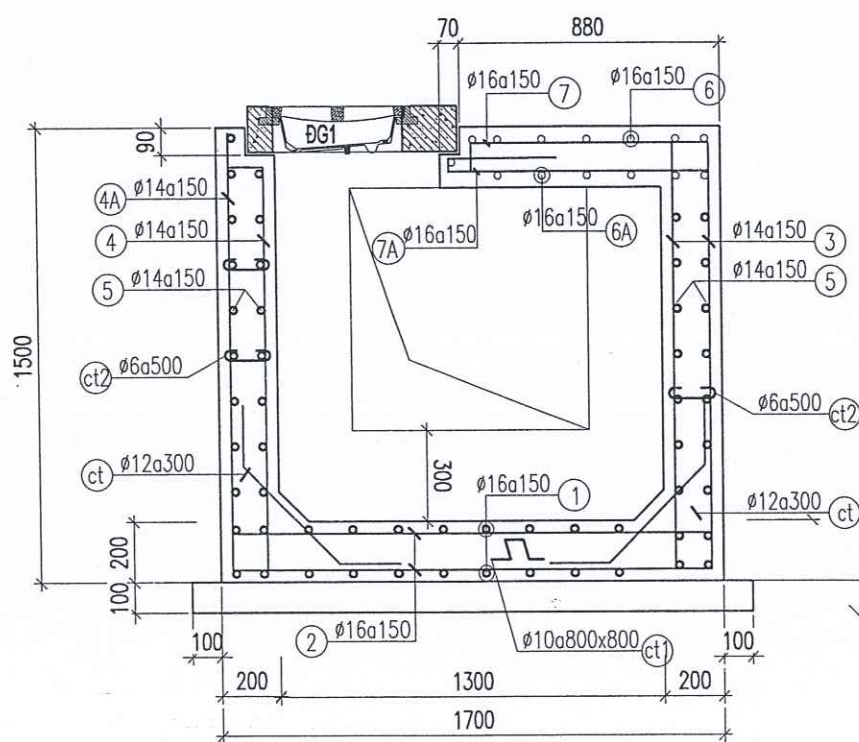
MẶT CẮT 1-1
