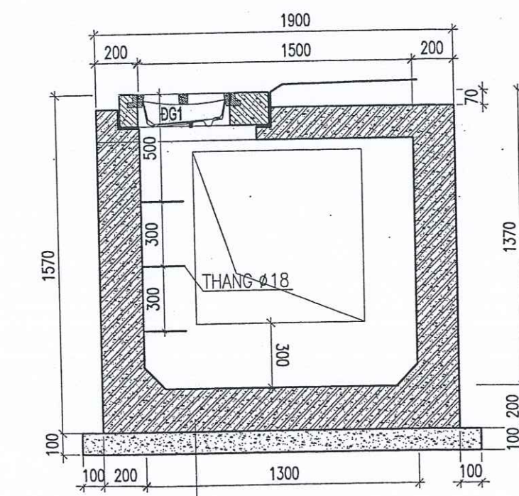
MẶT CẮT 1-1
