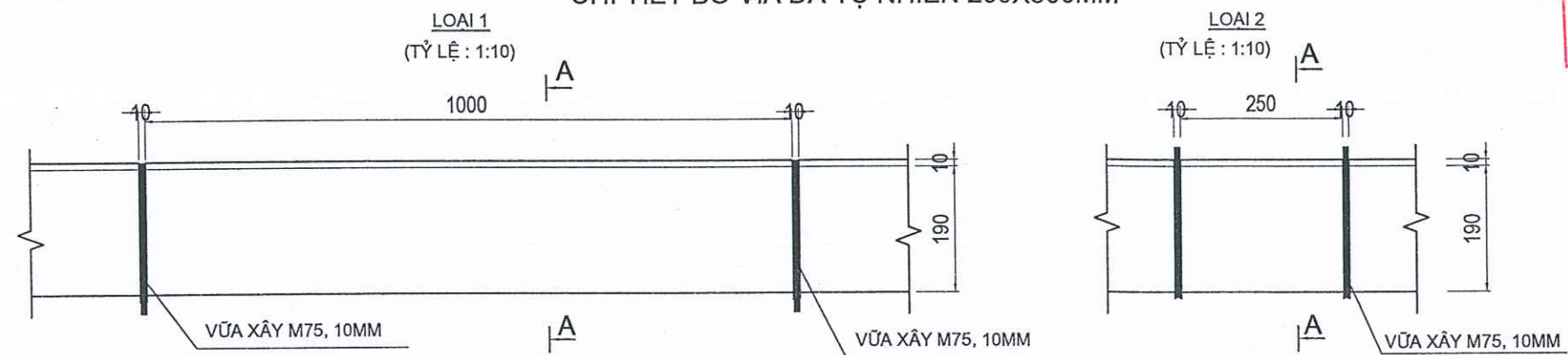
CHI TIẾT BÓ VỈA ĐÁ TỰ NHIÊN 200X300MM
