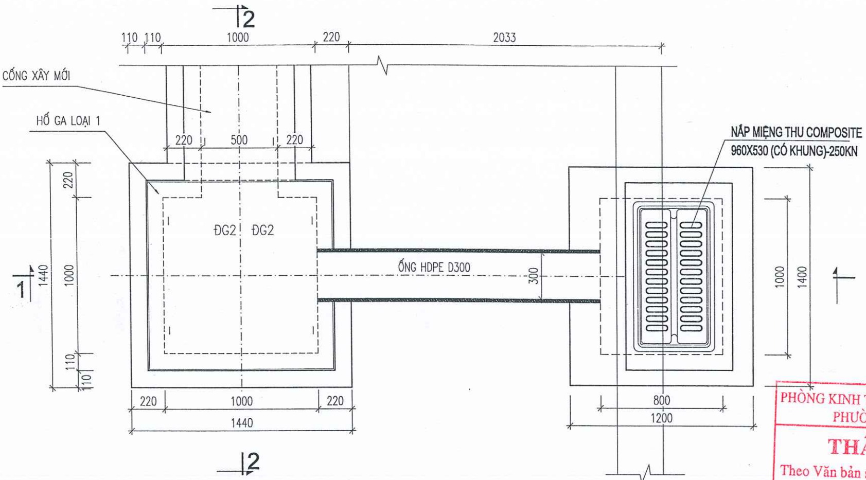
MẶT BẰNG HỒ GA TRÊN CỐNG XÂY MỚI B=500 K7; K29; K36; G22; G29; G32 (06 HỒ)
