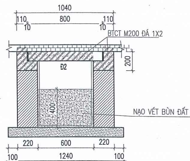
NAO VẾT CỐNG B = 600 HIỆN TRẠNG CHIỀU DÀI : 283.60 MÉT
