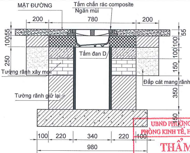
CHI TIẾT RĂNG CẢI TẠO
