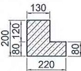
CHI TIẾT CỔ RÃNH
