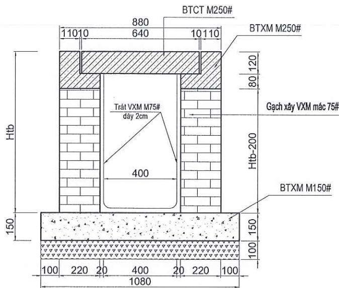
CHI TIẾT RÃNH THOÁT NƯỚC B400
