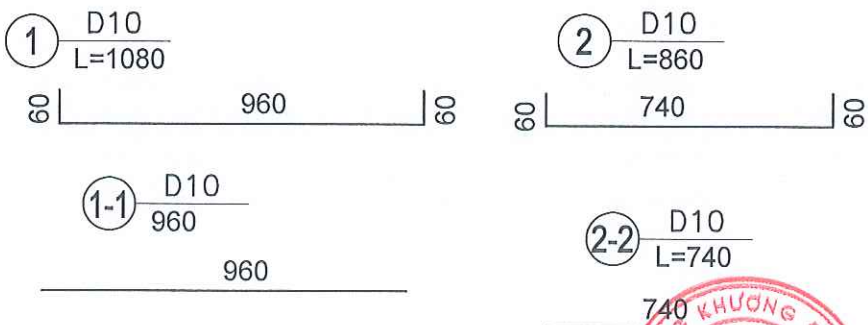
QUY CÁCH CỐT THÉP
