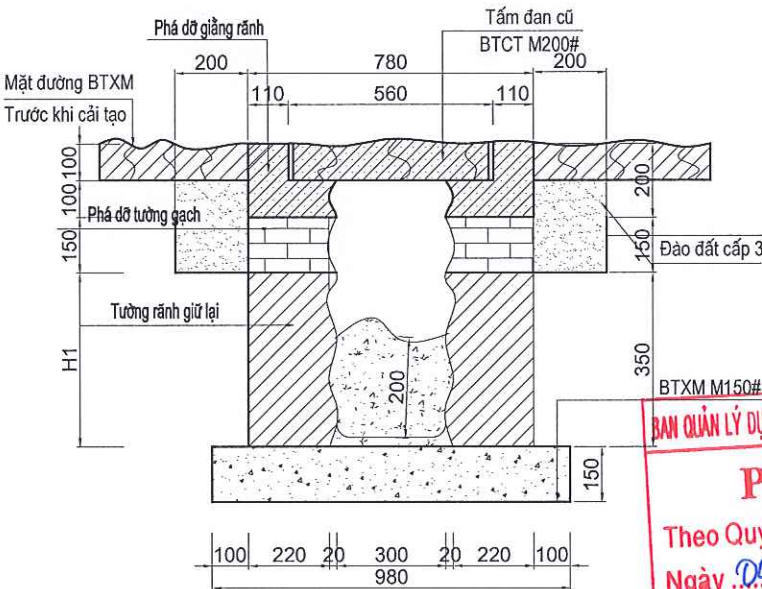
CHI TIẾT RÃNH THOÁT NƯỚC HIỆN TRẠNG
