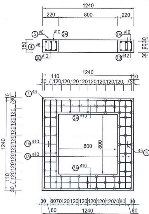
BỐ TRÍ CỐT THÉP TẮM ĐAN NẮP GA D1
