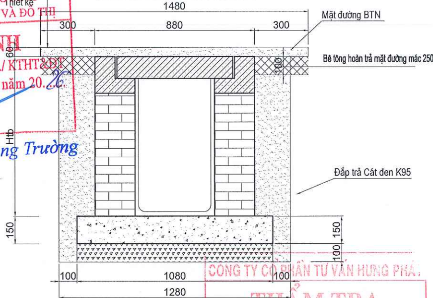
MẶT CẮT ĐÀO ĐẮP RÃNH
