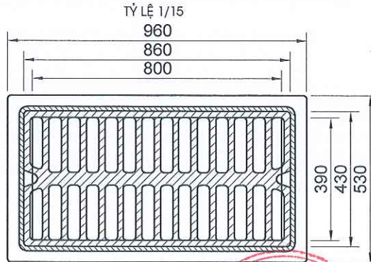
SONG CHÂN RÁC TẢI TRỌNG 250KN
