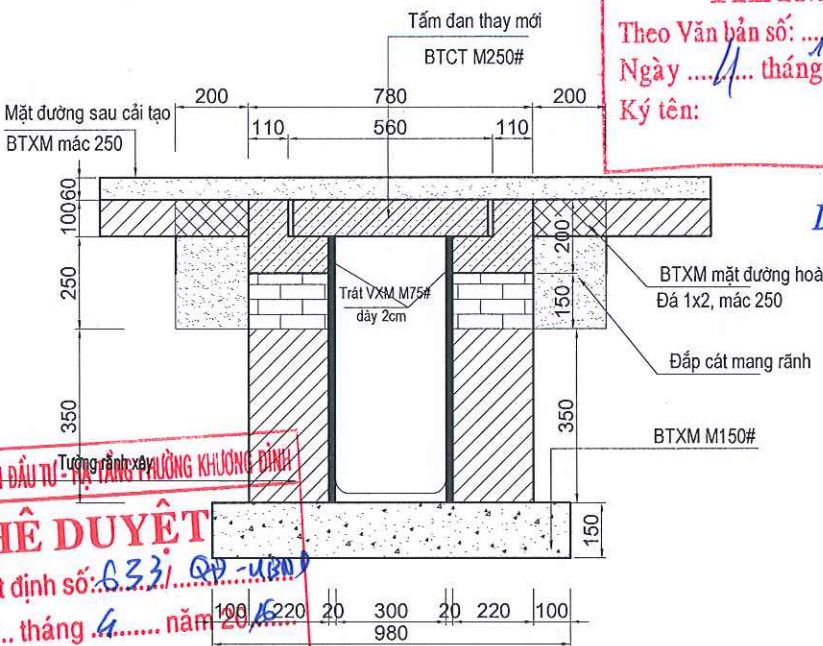
CHI TIẾT RÃNH THOÁT NƯỚC CẢI TẠO
