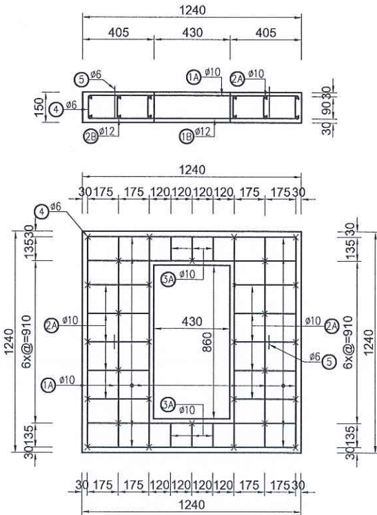
BỐ TRÍ CỐT THÉP TẤM ĐÀN NẮP GA D1
