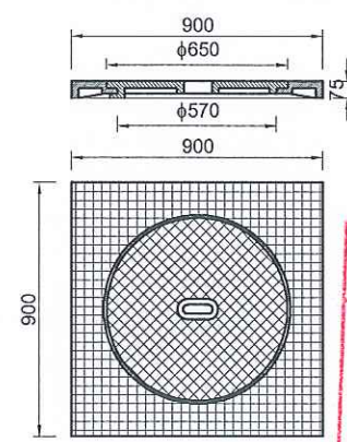
CẤU TẠO NẮP GA GANG TRÒN
