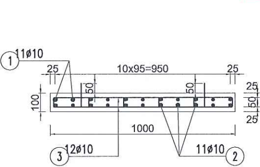
CHI TIẾT CỔ RÃNH
