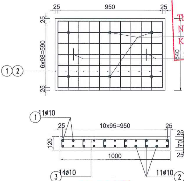
CHI TIẾT TẤM ĐAN RÃNH
