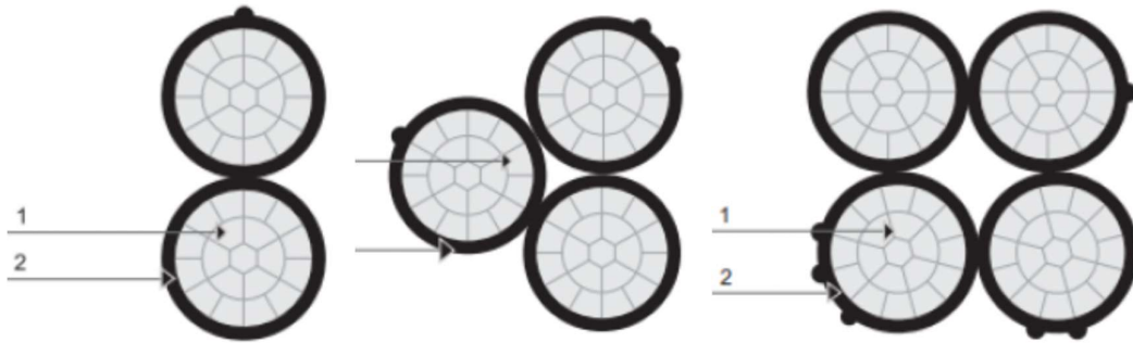
Hình: Mặt cắt 3 loại cáp vặn xoắn điển hình (2 lõi, 3 lõi, 4 lõi) với lõi trung tâm là kiểu tron không gân.
