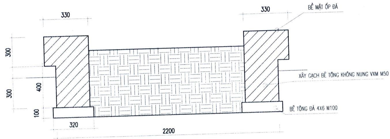
CHI TIẾT BỐN HOA SL:02 CK
