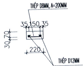
CẮT NGANG GIÀNG MÓNG
