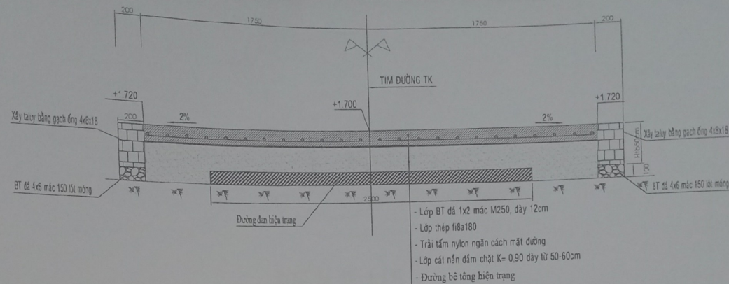
MẶT CẮT NGANG ĐẠI DIỆN ĐOẠN XÂY TALUY TỪ ĐCT -C1 TL: 1/25
