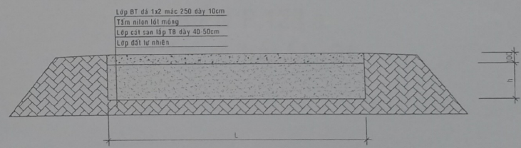
MC 1-1: TỶ LỆ 1/25
