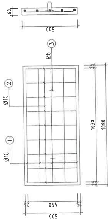
TẮM ĐẠN TĐ1 (SL=30 TẮM)
