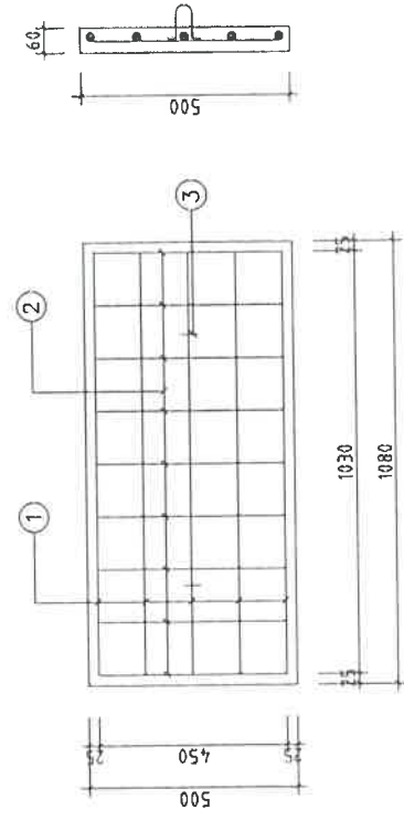
TẦM ĐẠN TĐ1 THẢO DỠ (SL=30 TẦM)
