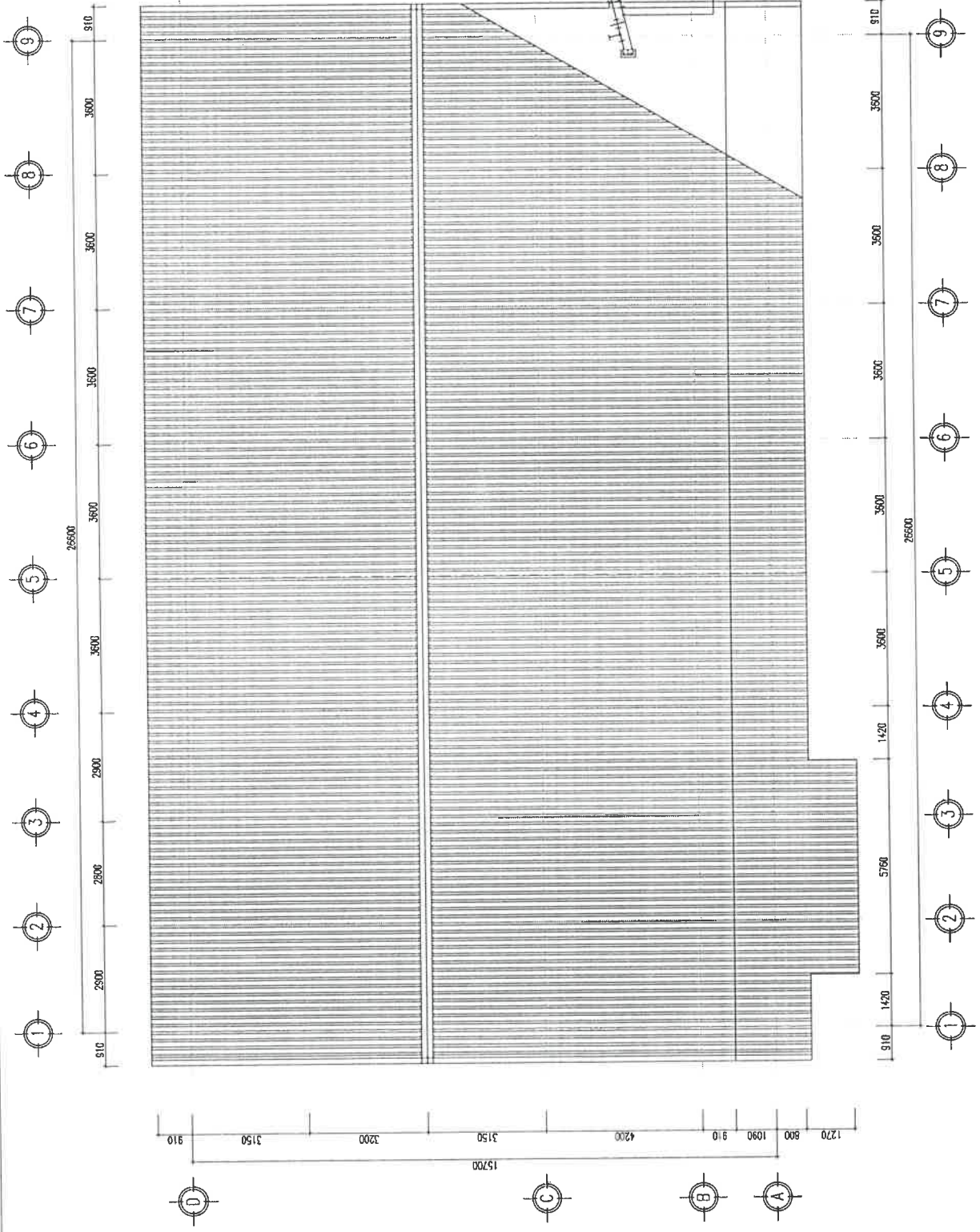
MẶT BẰNG MÁI NHÀ ĐKPP SỬA CHỮA
