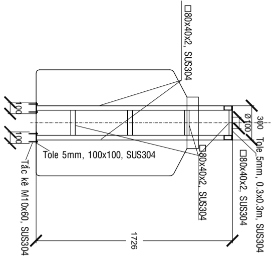
MẶT CẮT I - I
