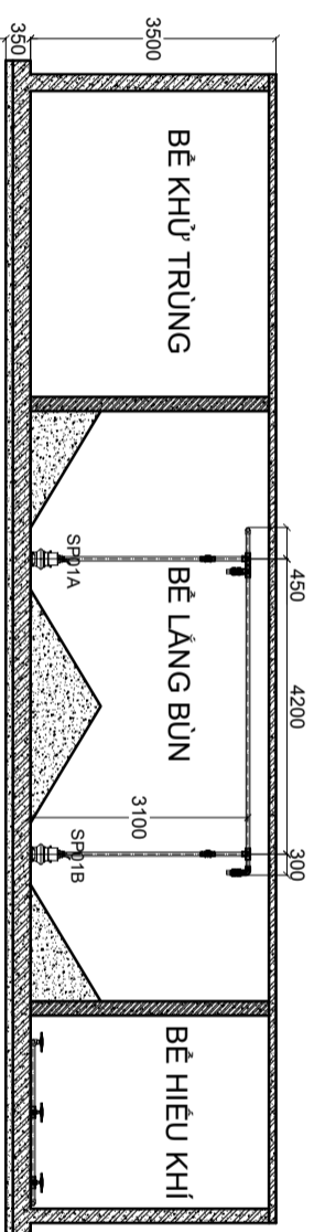
MẶT CẮT ĐỨNG B-B
