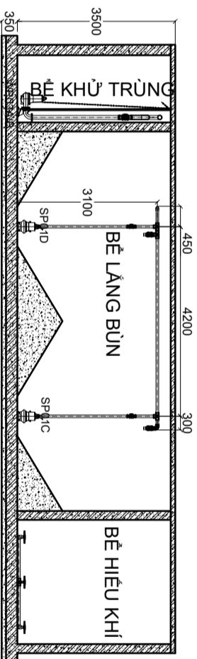
MẶT CẮT ĐỨNG A-A
