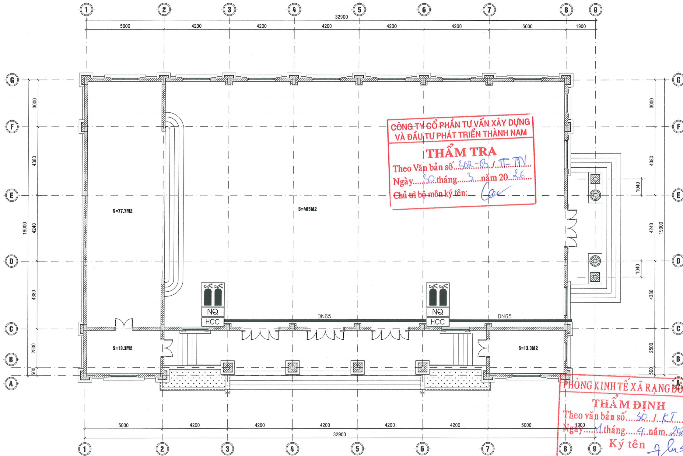
MẶT BẰNG HỆ THỐNG CHỮA CHÁY NHÀ ĐA NĂNG (VỊ TRÍ 3 TRÊN TMB)
