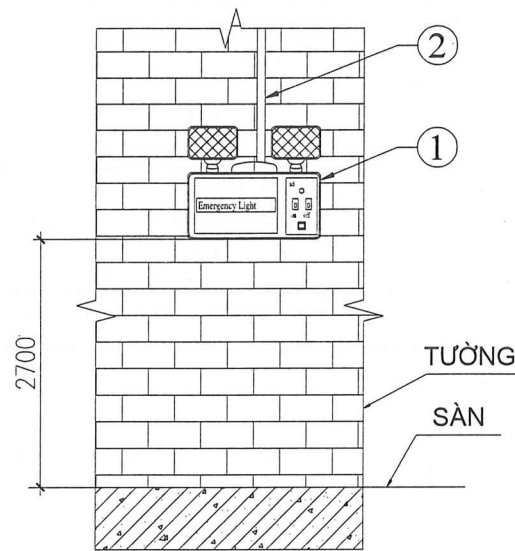
MẶT ĐỨNG/FRONT VIEW
