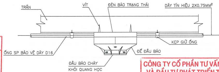
CHI TIẾT LẮP ĐẶT ĐẦU BÁO KHỐI
