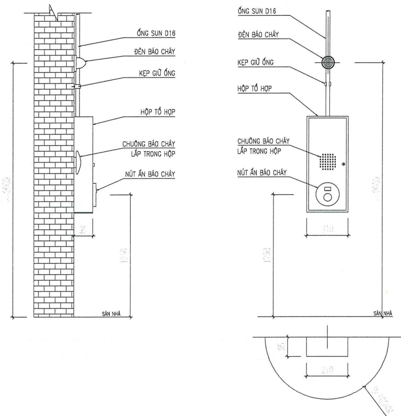
CHI TIẾT LẮP ĐẶT HỘP TỔ HỢP CHUÔNG, ĐÈN, NÚT ẮN BÁO CHÁY
