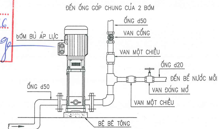
CHI TIẾT LẮP ĐẶT BƠM BÙ ÁP LỰC
