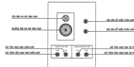
CHI TIẾT TỦ TÍN HIỆU GIÁM SÁT TRẠM BƠM
