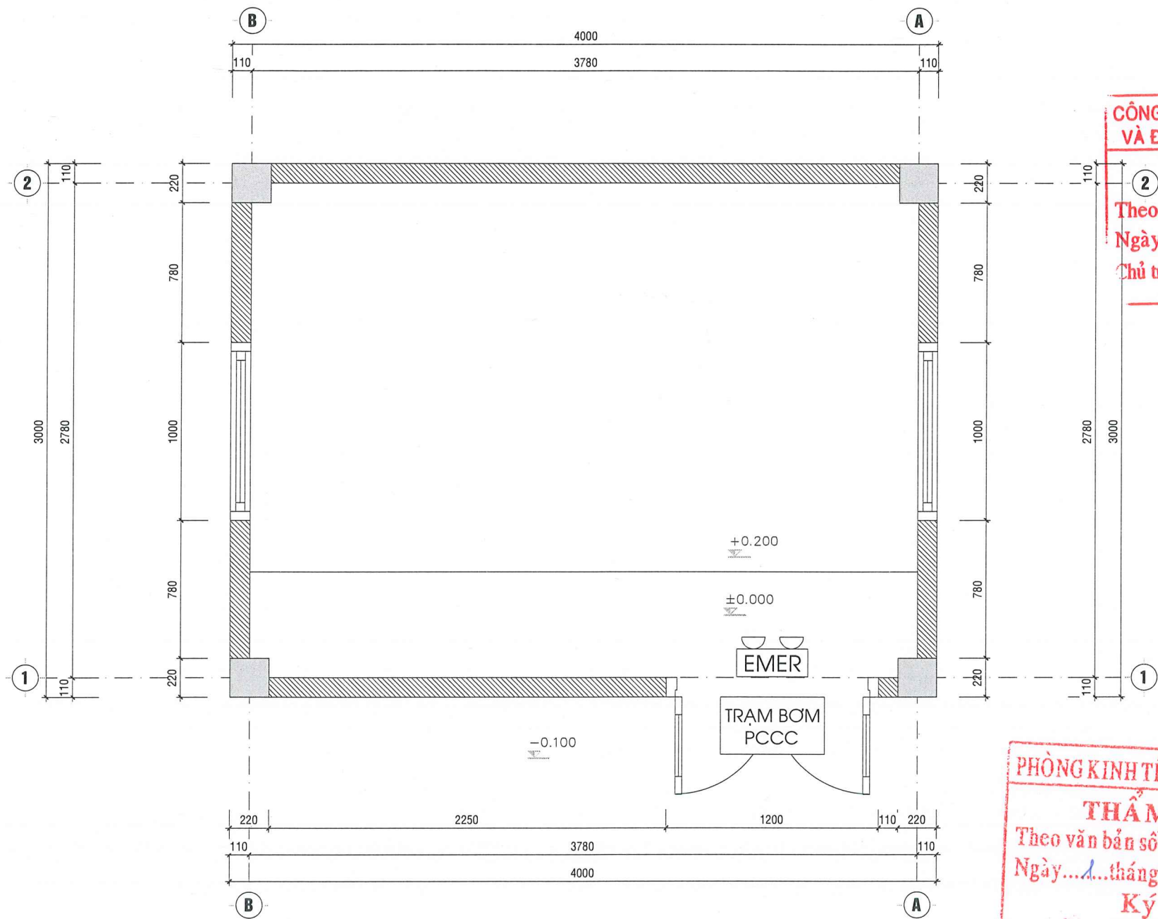
MẶT BẰNG HỆ THỐNG ĐÈN EXIT VÀ ĐÈN SỰ CỐ NHÀ TRẠM BƠM (VỊ TRÍ 10 TRÊN TMB)
