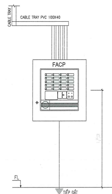
CHI TIẾT LẮP ĐẶT TỦ BÁO CHÁY TRUNG TÂM
