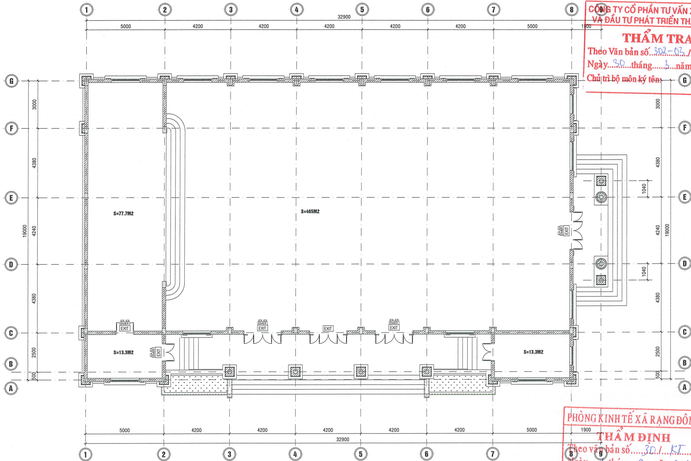
MẶT BẰNG HỆ THỐNG ĐÈN EXIT VÀ ĐÈN SỰ CỐ NHÀ ĐA NĂNG (VỊ TRÍ 3 TRÊN TMB)
