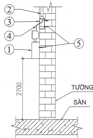
MẶT CẠNH/SIDE VIEW
