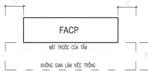
CHI TIẾT BỐ TRÍ KHÔNG GIAN TRỐNG XUNG QUANG TRƯỚC MẶT CỦA TỦ TRUNG TÂM BÁO CHÁY
