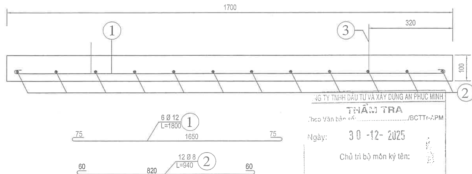
MẶT CẮT A - A
