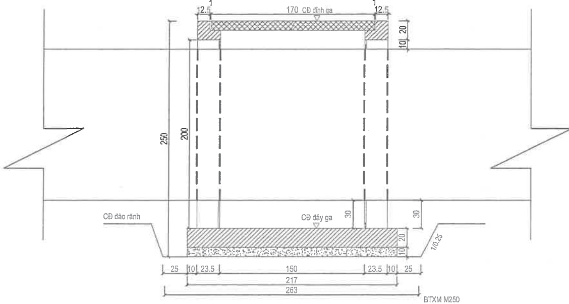
MẶT CẮT 2-2
