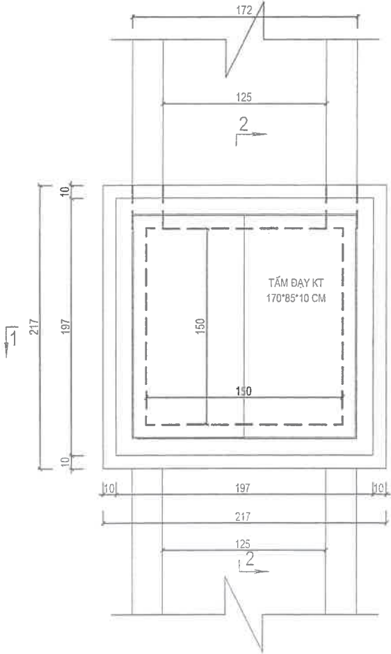
MẶT BẰNG
