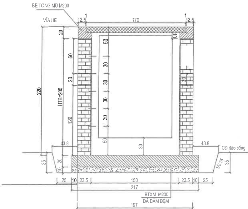
MẶT CẮT 1-1
