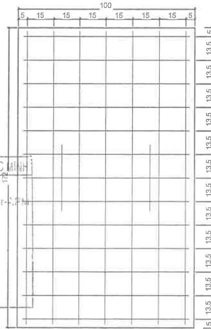
CẤU TẠO TẤM ĐAN KT100X77X15CM
