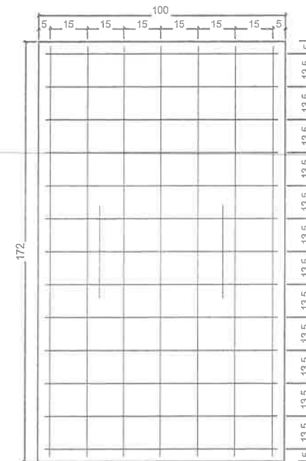
CẤU TẠO TẤM ĐAN KT100X77X15CM
