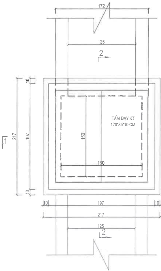
MẶT BẰNG
