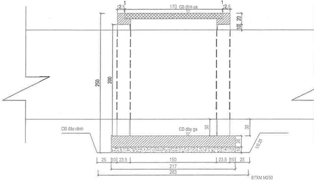
MẶT CẮT 2-2
