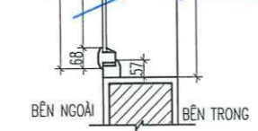
MẶT CẮT 1 - 1
