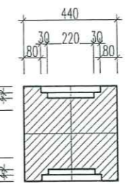
MẶT CẮT 3-3
