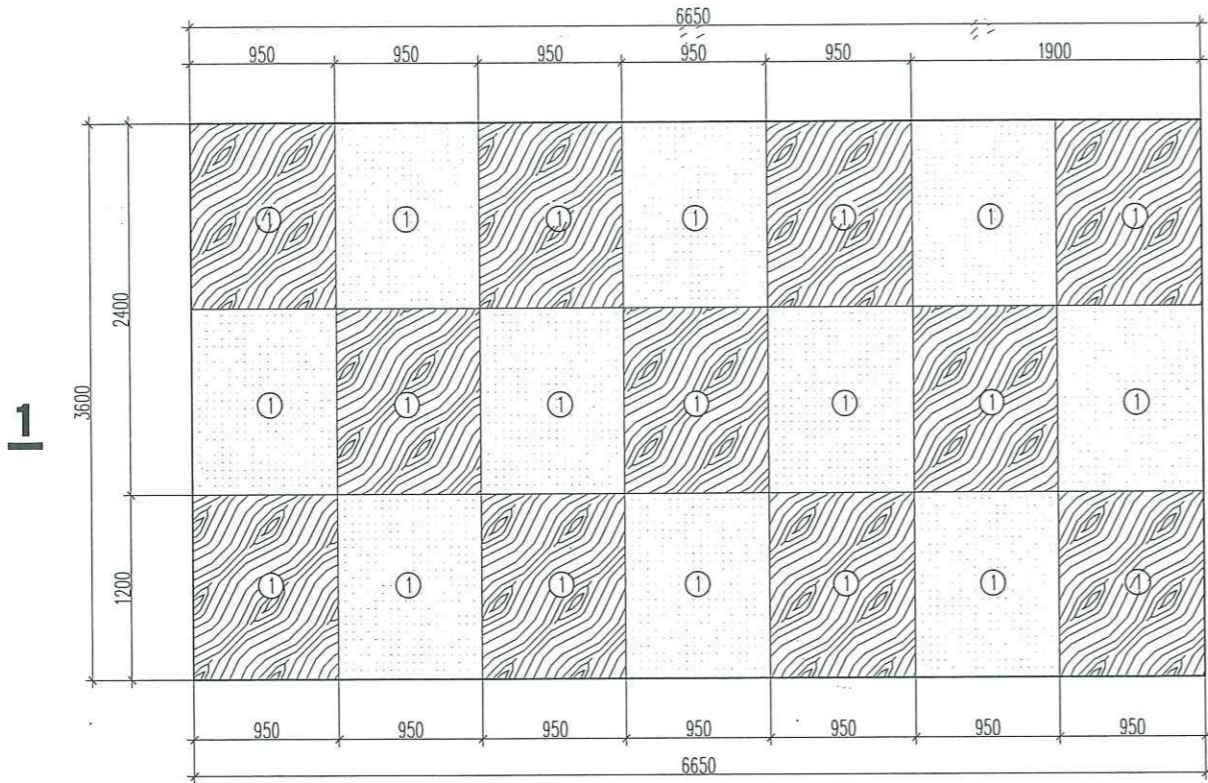
MẶT BẰNG BUC SÂN KHẤU PHÒNG HỘI TRƯỜNG (SL=01CK)
