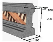
MẶT CẮT
