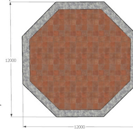
CỘT NHÀ
