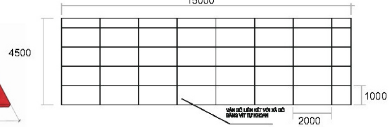
SƠ ĐỒ TRẢI SẮT HỘP 40MM X 80MM X 1.4MM DÀY
