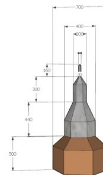
HỌA TIẾT TRANG TRÍ ĐỈNH MÁI
