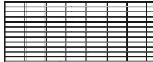
SƠ ĐỒ TRẢI SẮT HỘP 40MM X 80MM X 1.4MM DÀY
