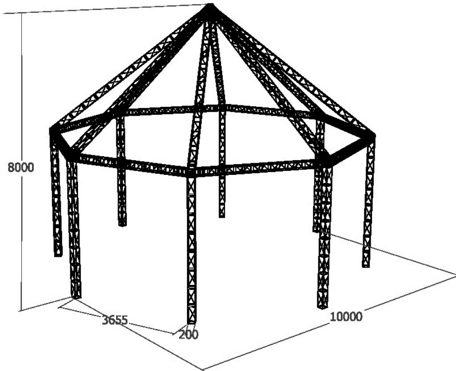
KÍCH THƯỚC CHI TIẾT CỦA KHUNG NHÀ
