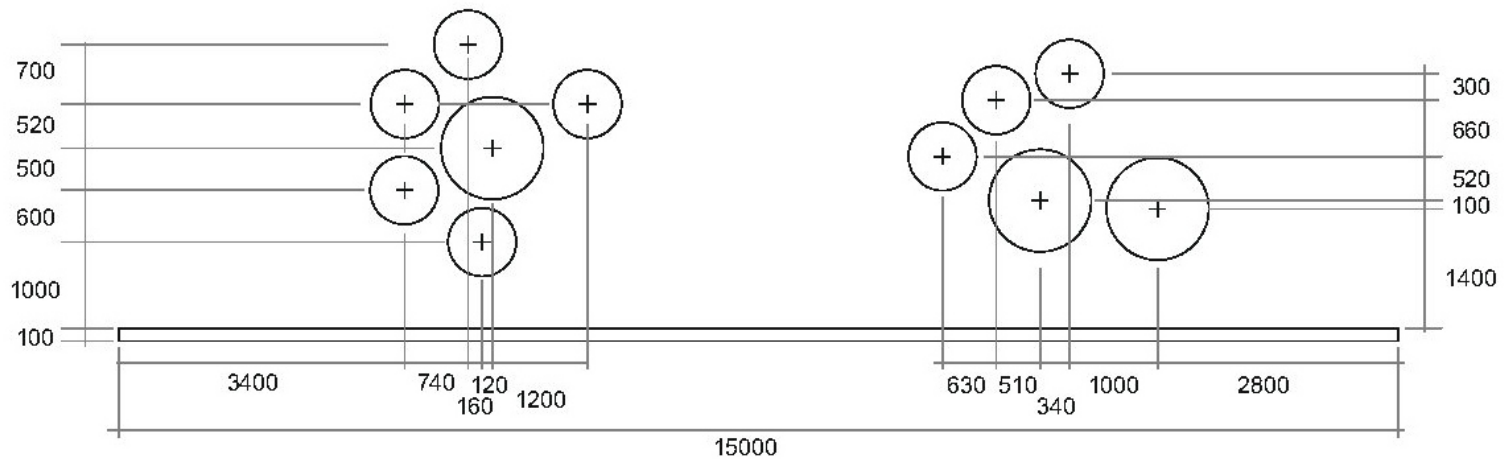
VỊ TRÍ VÀ KHOẢNG CÁCH TREO MỆT TRE
