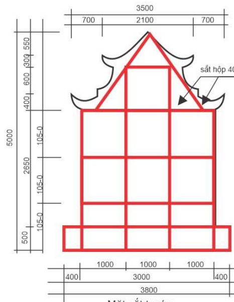
Mặt cắt trước Mặt cắt bên Khung Nhà mái đình ( SL: 2 bộ)
