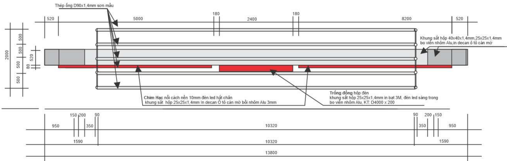
MẶT BẰNG ( đơn vị tính mm)
