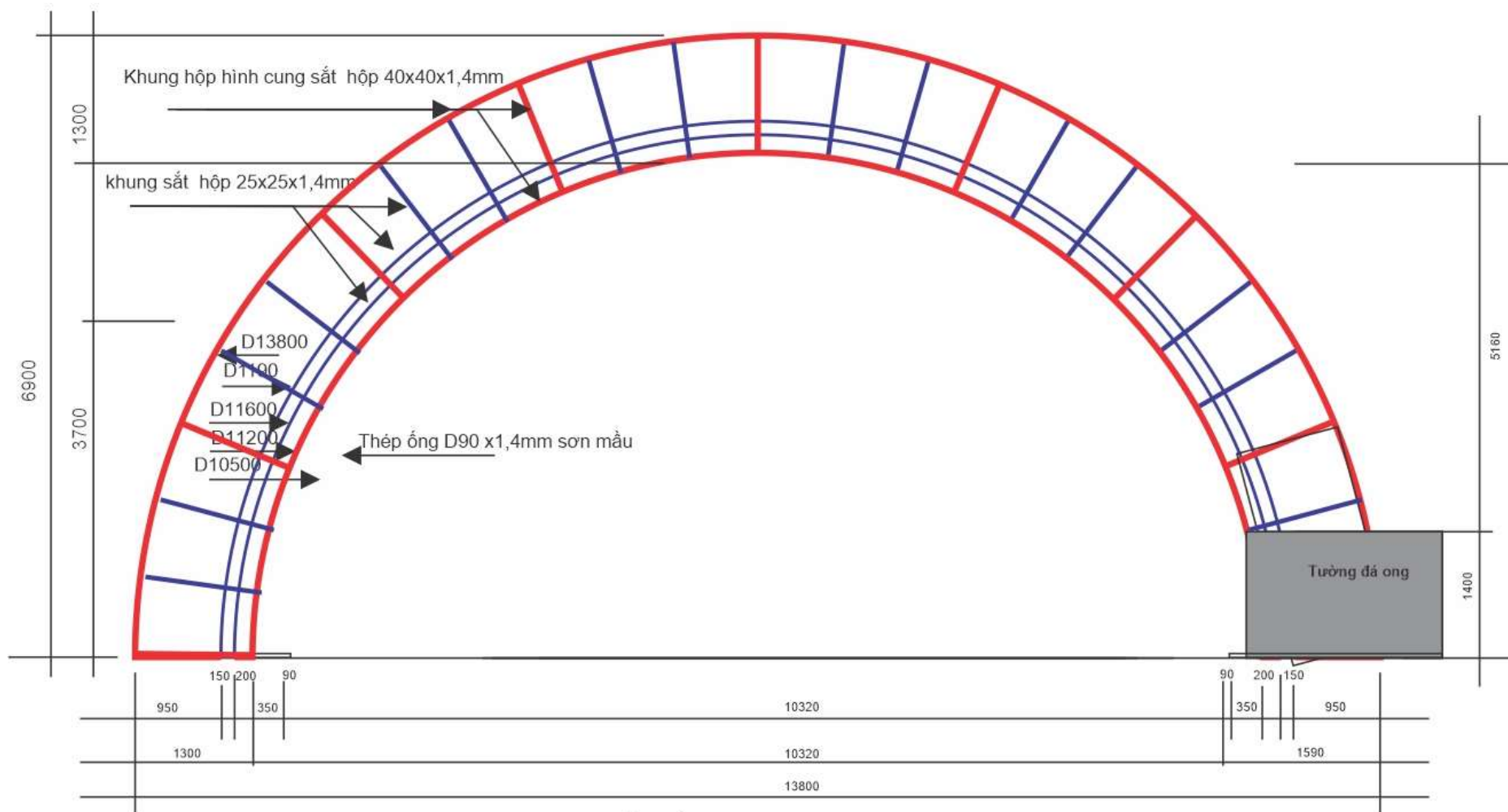
MẶT CẮT KHUNG ( đơn vị tính mm)
