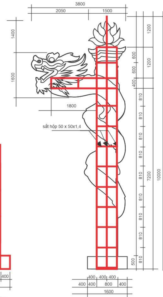
Khung tròn cột RỒNG ( SL: 2 bộ)
