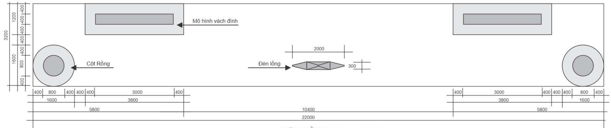
MẶT BẰNG (đơn vị tính mm)
