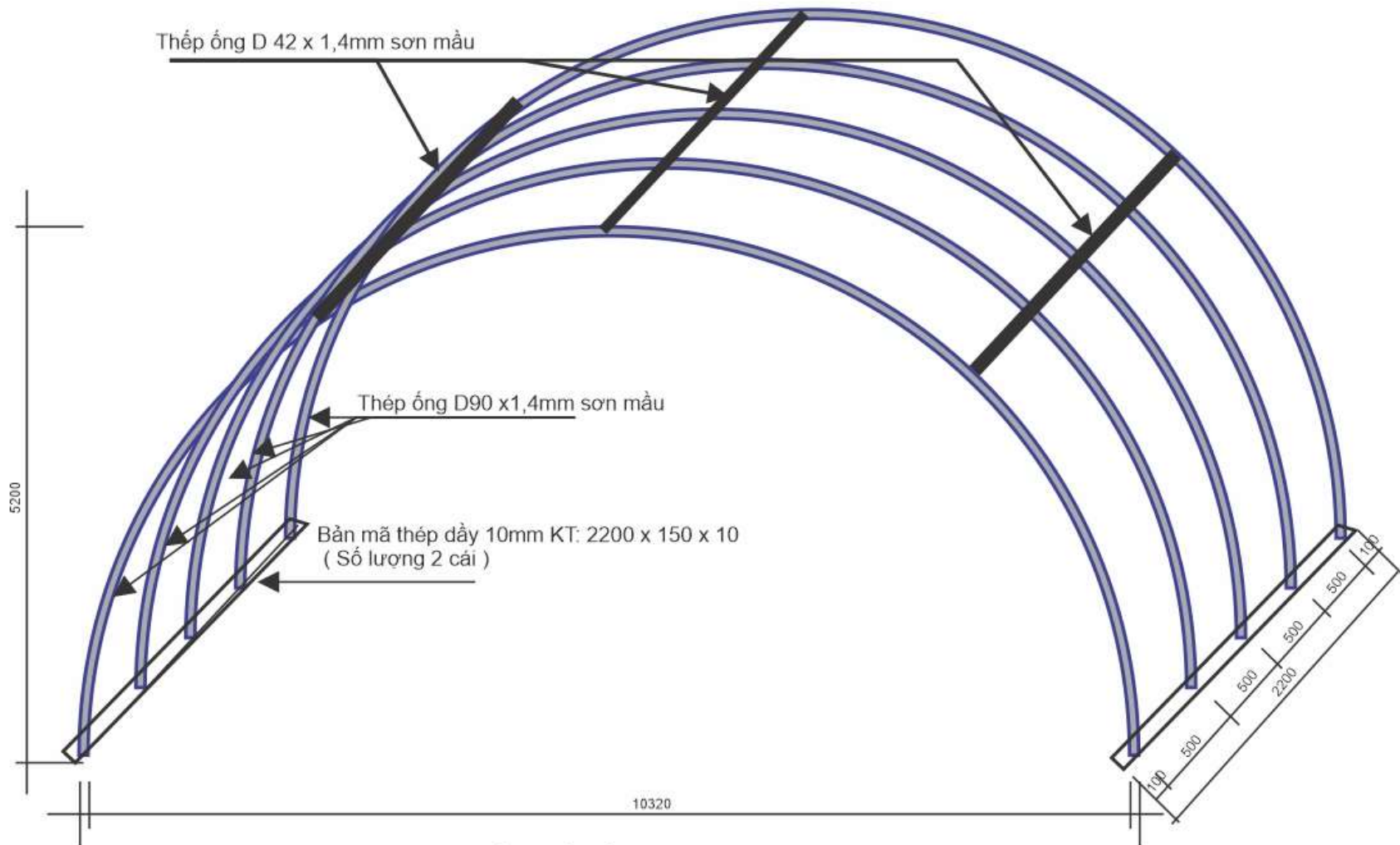
KHUNG VÒM SẮT ỚNG ( đơn vị tính mm)
