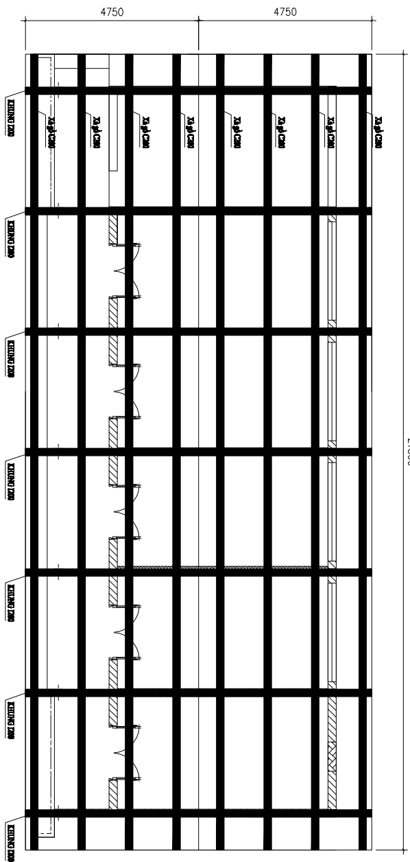
MẶT BẰNG KHUNG & XÀ GỖ NHÀ GIAO CA
