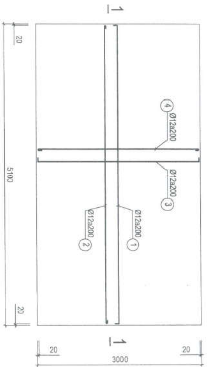
MẶT BẰNG THẸP DÂY BÊ
