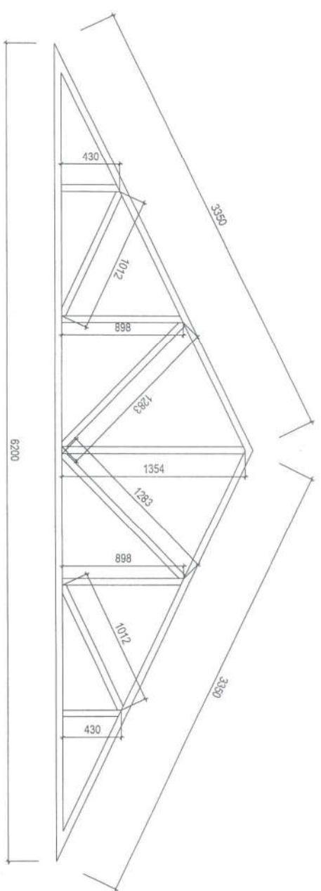
VỊ KÈO HIỆN TRẠNG TRỤC 6 ĐOẠN B-C THÉP HỘP (01 CK)
