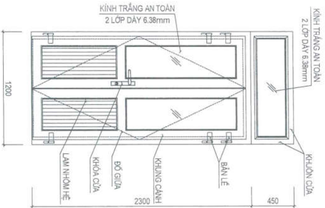
CHI TIẾT CỬA ĐI D1CT (5BỘ)
