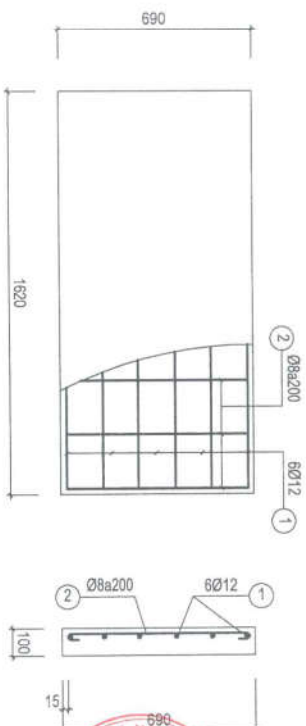
ĐAN D2 (04CK)
