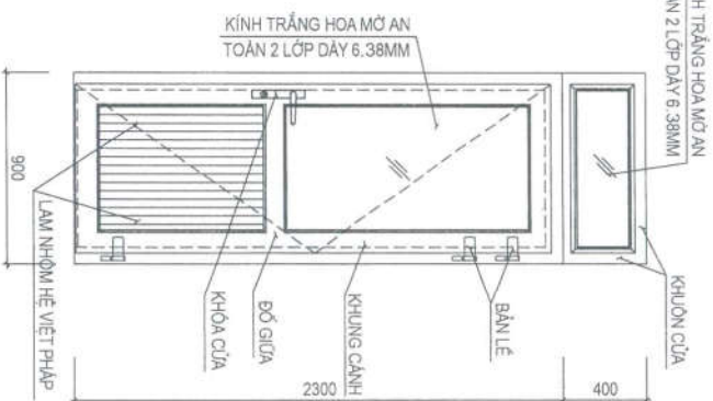
CHI TIẾT CỬA ĐI D2 (1B)
