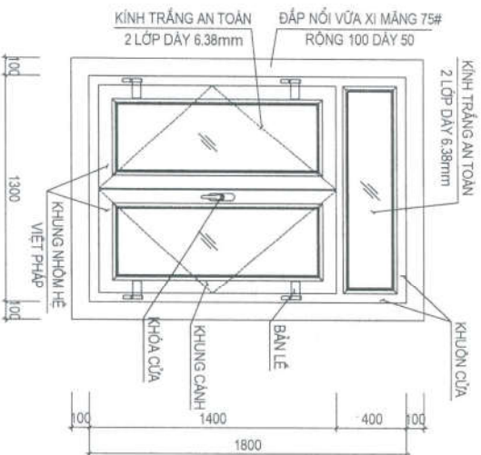
CHI TIẾT CỬA SỎ S1 (12B)
