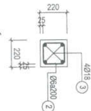
CẮT 3-3
