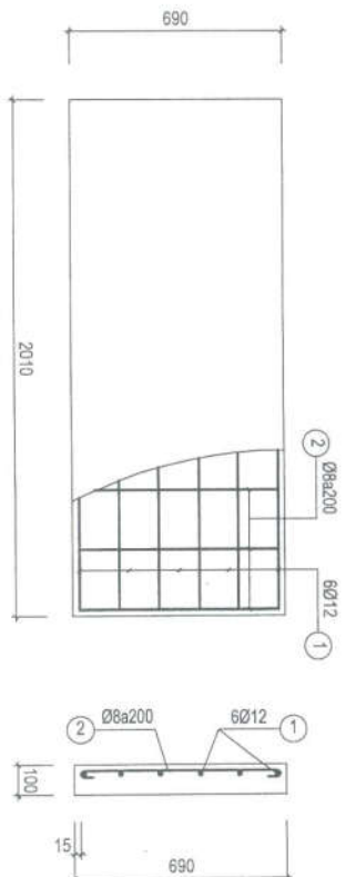
ĐAN D1 (04CK)
