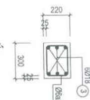
CẮT 4-4
