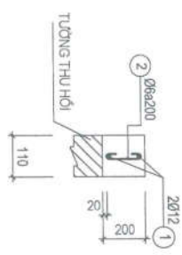
CẮT 3-3
