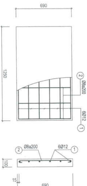
ĐAN D3 (04CK)
