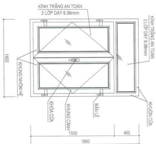
CHI TIẾT CỬA SỔ S1CT (2BỘ)
