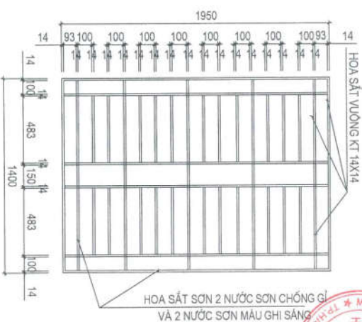
CHI TIẾT HOA SẮT CỬA SỔ S1CT (2 BỘ)
