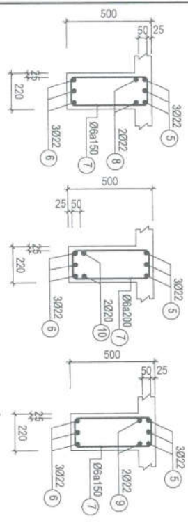
CẮT 7-7
