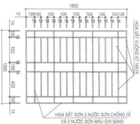
CHI TIẾT HOA SẮT CỬA SỎ S1 (12B)
