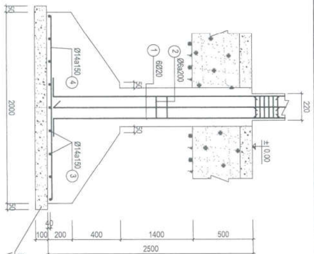
CẮT 1-1
