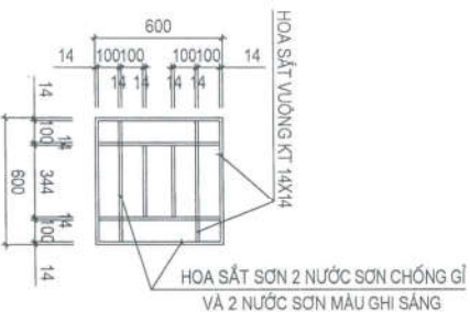
CHI TIẾT HOA SẮT CỬA SỔ S2LM (5 BỘ)
