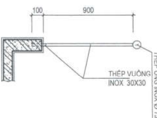
CẮT 2-2
