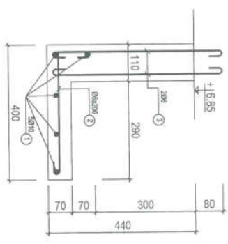
CẮT 2-2
