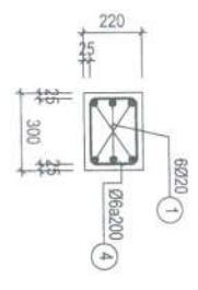
CẮT 2-2
