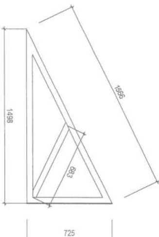
BÀN KÈO HIỆN TRẠNG THÉP HỘP (05 CK)
