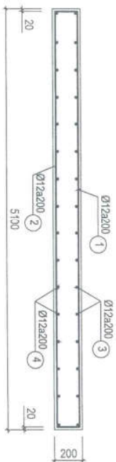
MẶT CẮT 1-1
