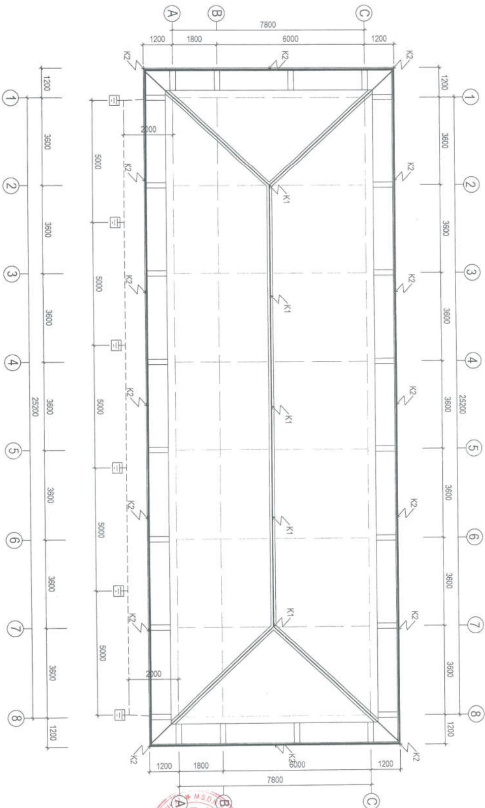
MẶT BẰNG BỐ TRÍ HỆ THỐNG CHỐNG SÉT MÀI
