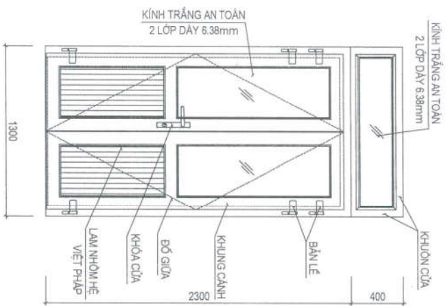
CHI TIẾT CỬA ĐI D1 (12B)
