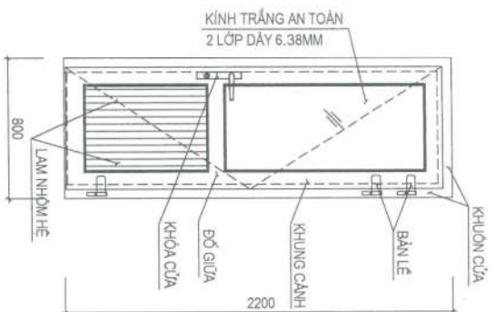
CHI TIẾT CỬA ĐI D2CT (1BỘ)
