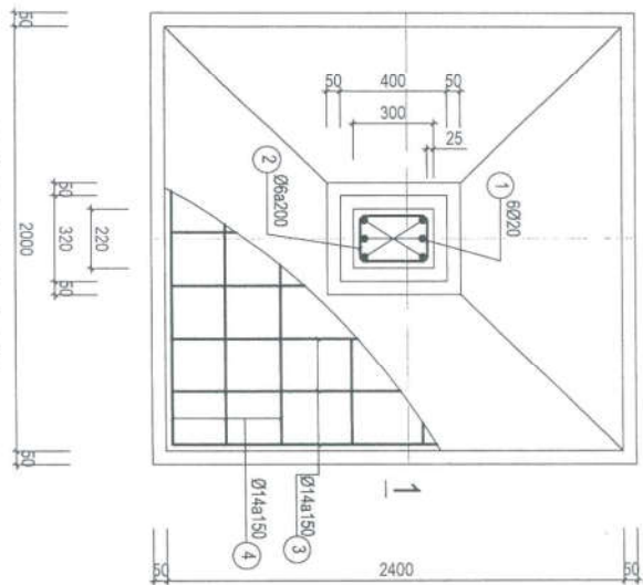
MÔNG MT1 (8CK)
