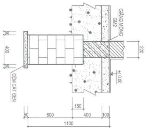
MÓNG M1
